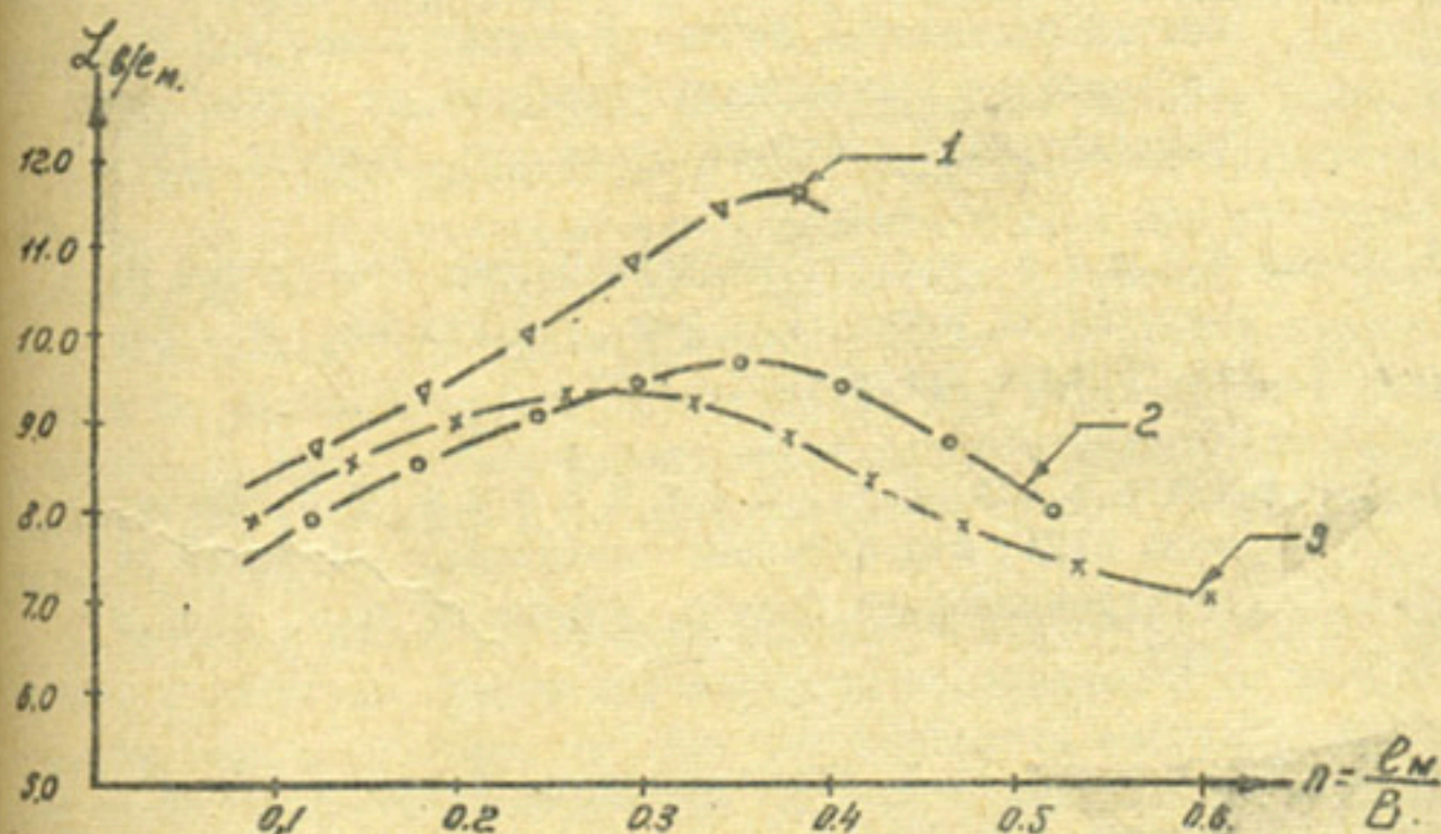
Рис. 2. График L B / e_m = f(n) : 1 — по Бакиеву М.Р. и др.; 2 — по автору (метод ЭГДА); 3 — по Баланину В.В. и др.
