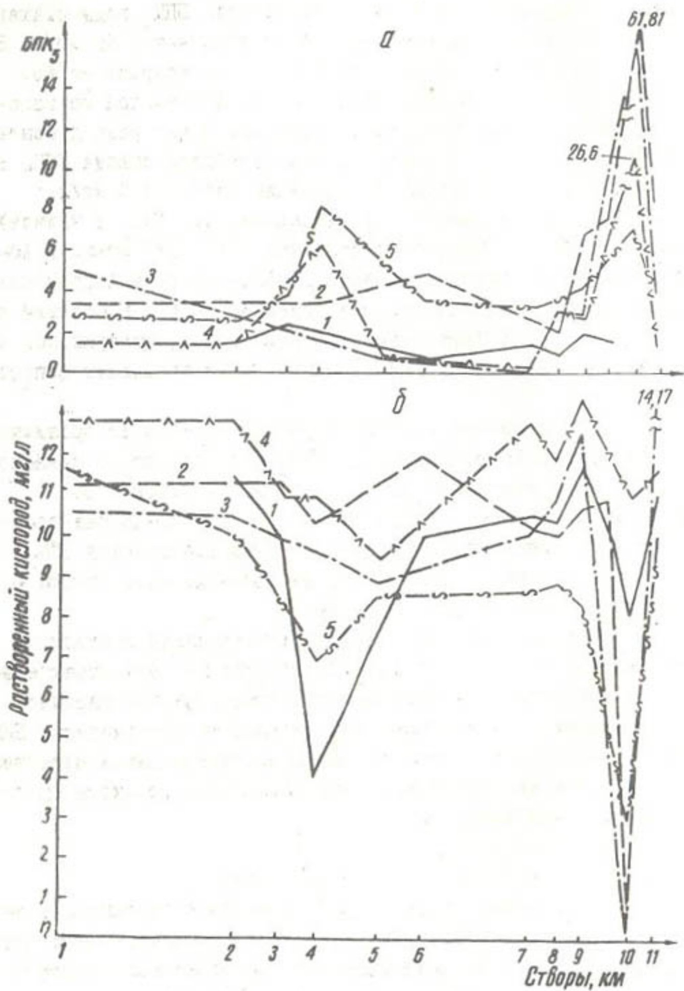
Рис. 4. БПК 5 (а) и растворенный кислород (б) в воде ДАХАНГАРАН. 1-зима; 2-весна; 3- лето; 4-осень; 5-ср. год 1964.
