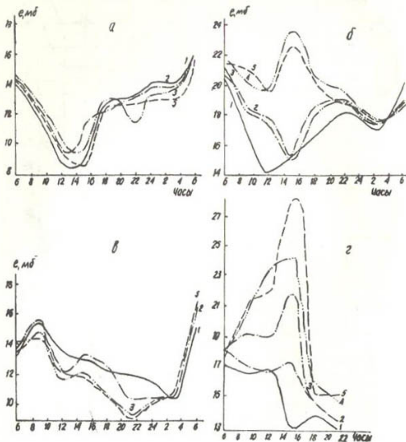
Рис.3.Суточный ход абсолютной влажности воздуха на хлопковом поле: а-22-23.УІ до полива; б-І-2.УІІ после полива; в-І3-І4.УІ до полива; г-3.УІІ после полива. І-3м; 2-І; 3-0,5; 4-0,2; 5-0,1м.
