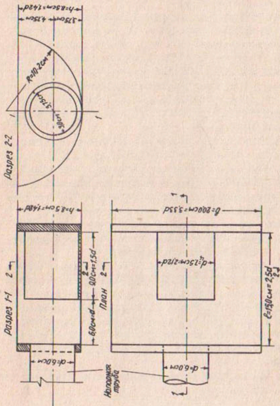
Рис. I. Односекционный гаситель-растекатель для \frac{Q^2}{D^3} < 10,0 \text{ м/сек}^2 .
