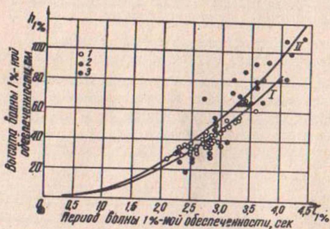
Рис. 4. Кривые связи между высотой и периодом волны 1%-ной обеспеченности. Данные натуре: I—по Каттакурганскому; 2—Южносурханскому; 3—Кайраккумскому водохранилищам. Кривые: I—для Ташкентского водохранилища; II—для Кайраккумского.
