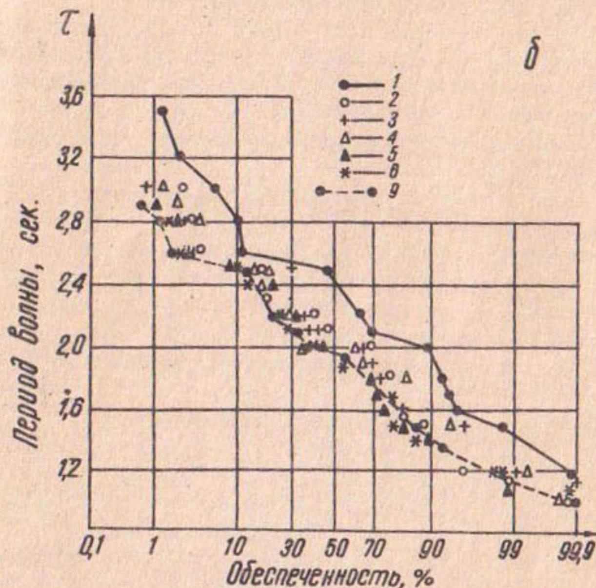
Рис.4. Изменение периодов волн при их движении в сторону уменьшающихся глубин на Кайраккумском водохранилище: а- изменение \tau/\tau_0 с увеличением h/H ( \tau_0 - период глубоководной волны; h - высота волны; H - глубина воды; б- изменение кривых обеспеченностей периодов волн по мере движения волн к берегу (1-6, 9 - номера датчиков-волнографов).
