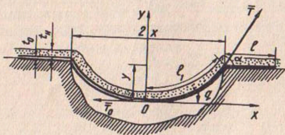
Рис. 2. Схематический продольный разрез гибкого тьюка, провисающего над ковшом.
