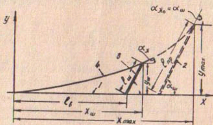
Рис.2. Расчетная схема для определения l_b ; x_{max} ; y_{max} .
