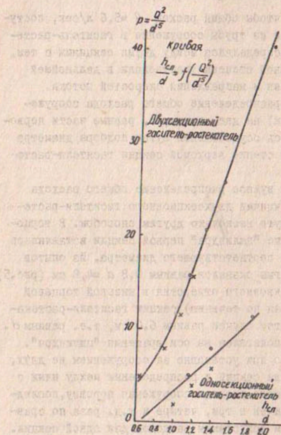
Рис. 5. Кривые \frac{h_{сл}}{d} = f\left(\frac{Q^2}{d^5}\right) для односекционного и двухсекционного гасителя-растекателя.
