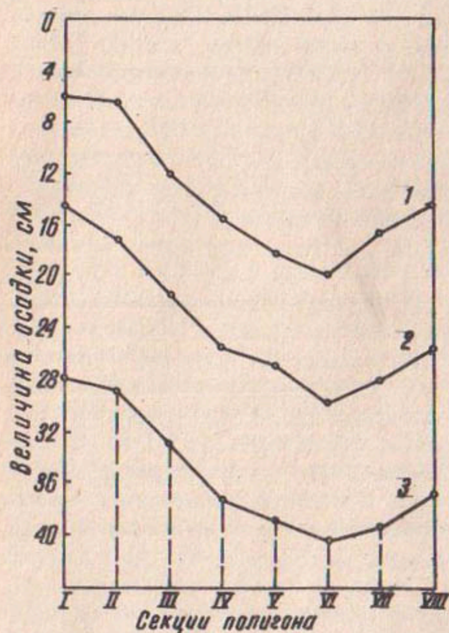
Рис.3. График изменения средней величины осадки креплений по секциям опытного полигона на пло- тине Ташкентского водохранилища: I-с I4.IY-6Iг. по I9.X-6Iг.; 2-с 20.X-6Iг. по I6.X-62г.; 3-с I6.X-62г. по I8.X-64г.
