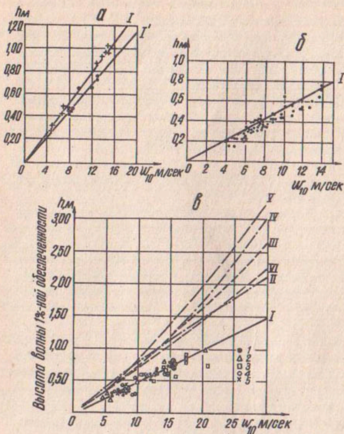
Рис.5. Зависимость h_{1\%} = f(w_{10}, D) : а-для Каттакурганского водохранилища (I-при юго-западном направлении ветра и длине разгона D=9 км; I'-то же при юго-восточном направлении и D=7 км); б-для Такентского водохранилища ( D=6 км); в-обобщенная зависимость h = f(w) для D=5 км. Расчетные кривые: I-по формуле, рекомендуемой САНИИРИ; II-по Лабзовскому; III-IV-по Браславскому (III-для H < 0,5 , IV-для H > 0,5 ) У-по Андриянову; VI-ТУСН 92-60. Данные натурных наблюдений: I-3 на Каттакурганском водохранилище (I-по данным волнографов, 2-по максимально-минимальным вехам, 3-по станции УГМС); 4-на Тедженском водохранилище; 5-на озере Часкак.
