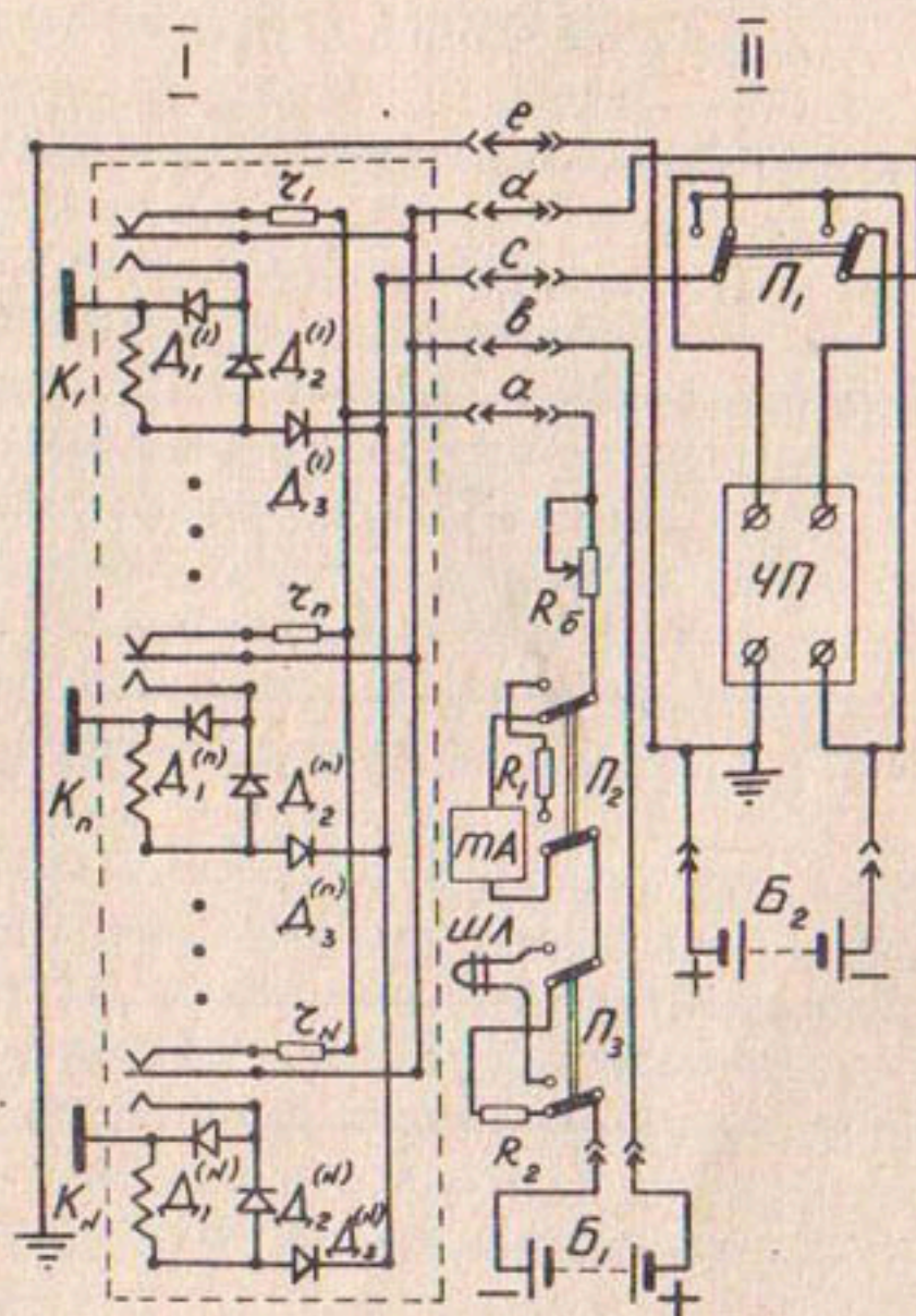
Рис. I. Электрическая схема релейного волномера-волнографа:
