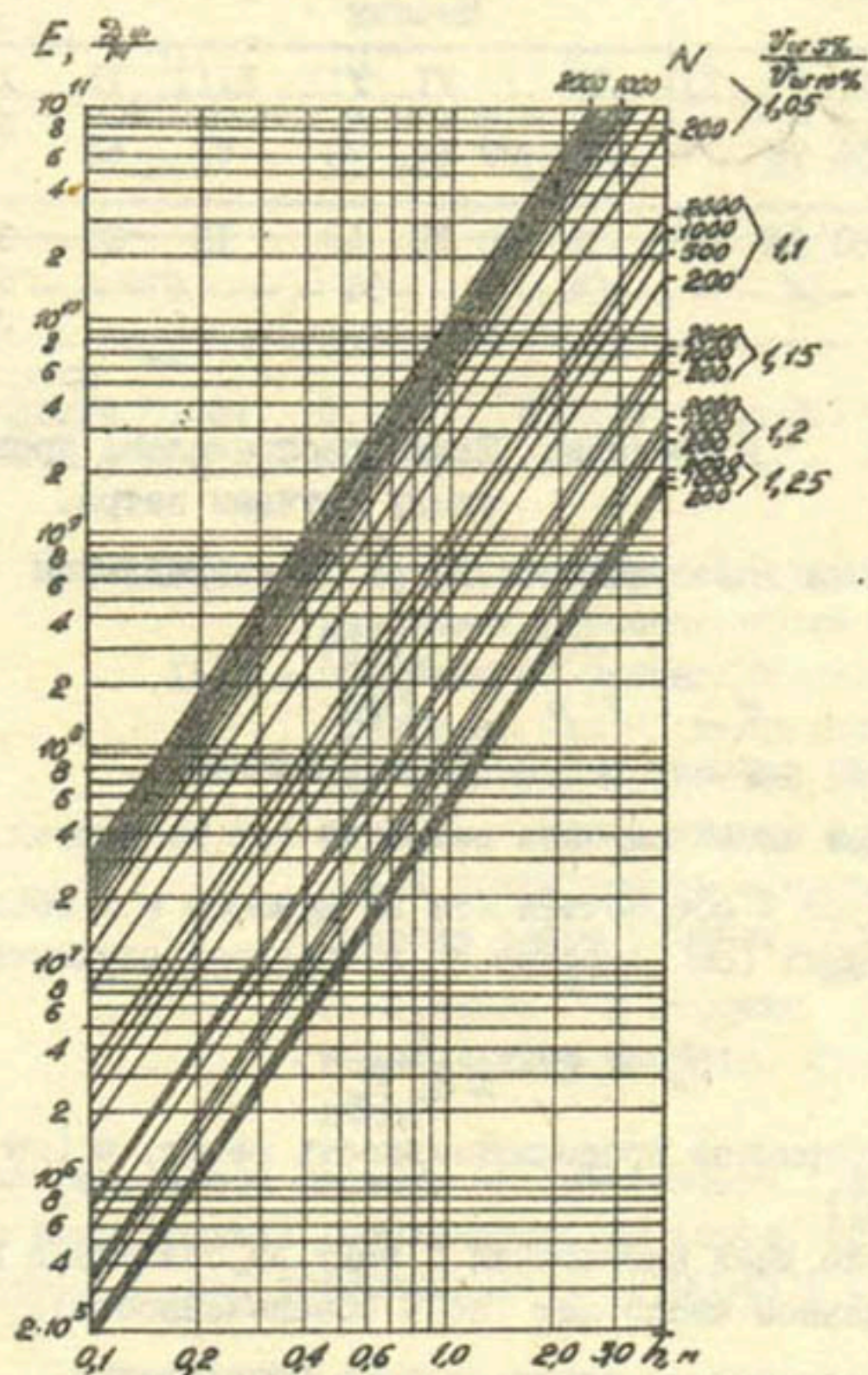
Рис. I. График для определения суммарной годовой энергии волн.
