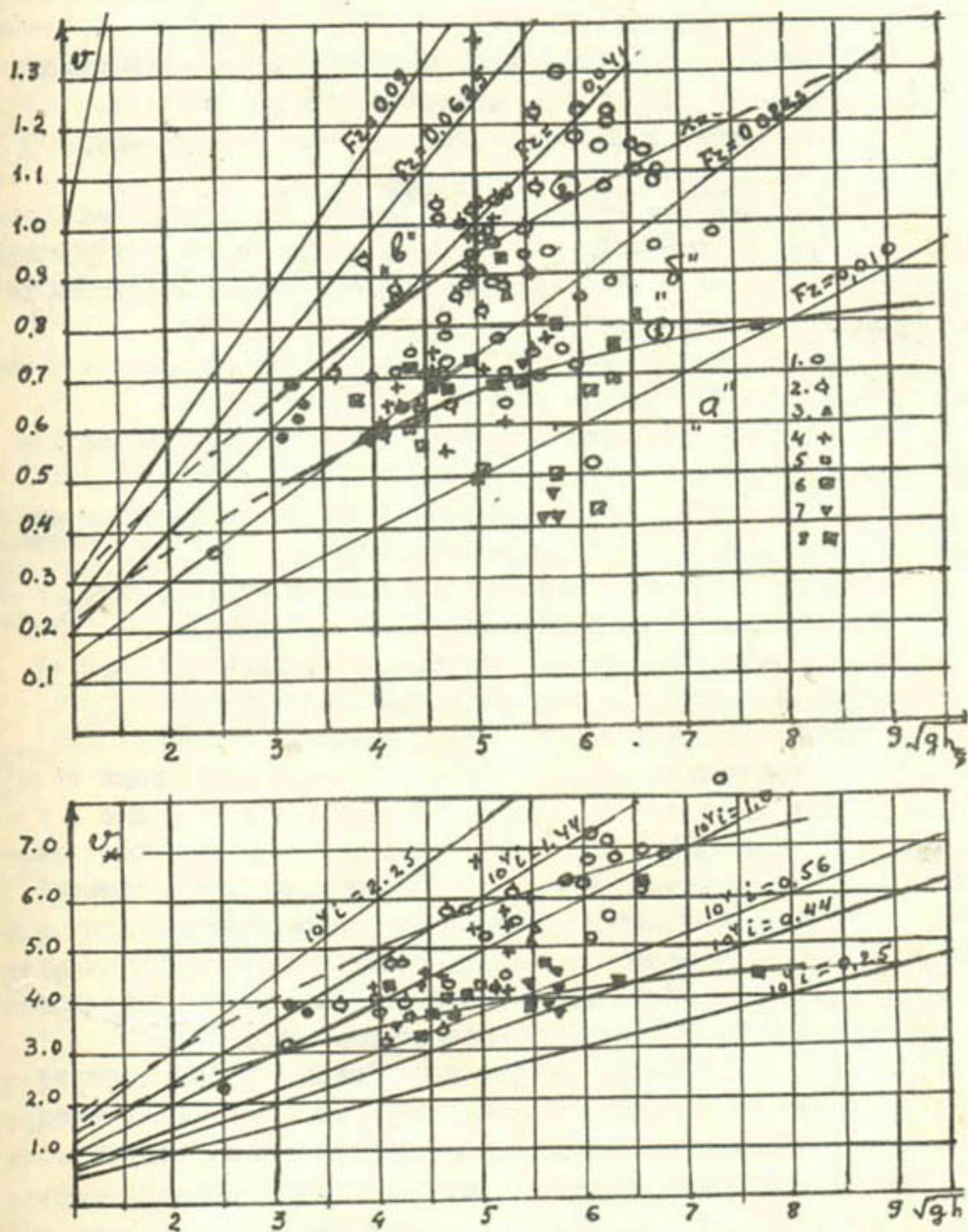
Рис. 2. График зависимости средней и динамической скоростей потока от \sqrt{qh} (обозначения те же, что на рис. 1): а) зона грядового движения наносов; б) переходная зона от начала срыва гряд к сплошному влечению наносов; в) зона сплошного движения наносов (зона гладкого дна).
