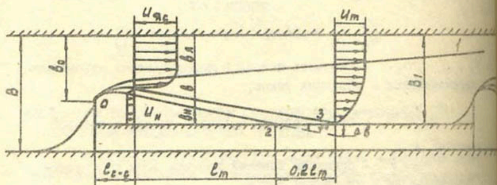
Рис. I. План растекания потока в междомоном пространстве.
