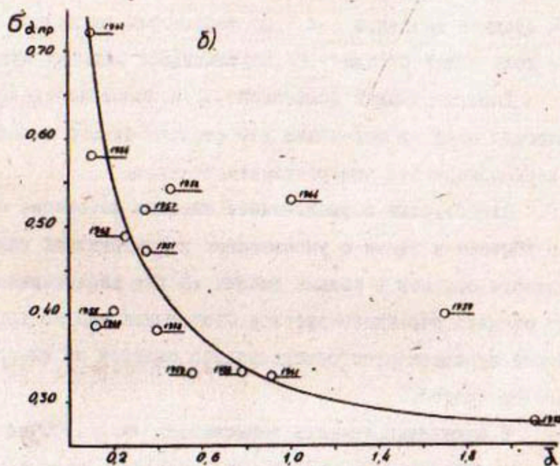
Рис. I Зависимость характеристики пространственной изменчивости осадков от степени увлажнения года.
