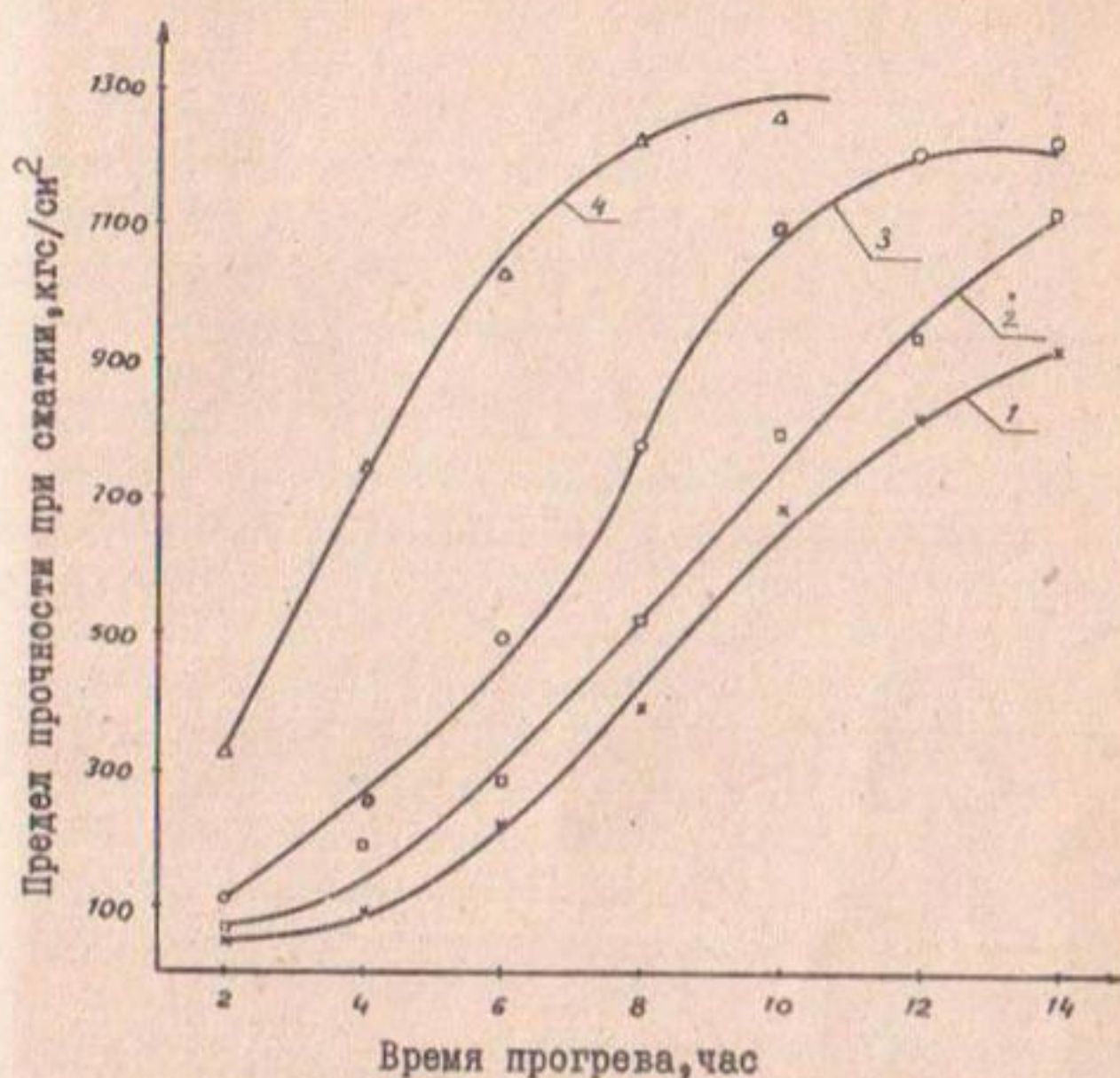
Рис. I. Влияние термообработки на прочность полимербетона на смоле ФД: 1—прогрев при 40°С; 2—прогрев при 60°С; 3—прогрев при 80°С; 4—прогрев при 100°С.
