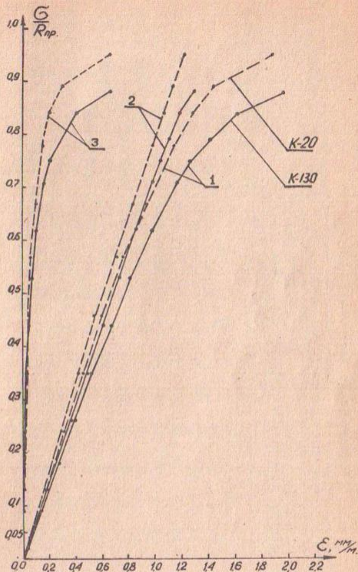
Рис.5. Зависимость \varepsilon = f\left(\frac{\sigma}{R_{np}}\right) для кернов : K - 20 (ступенчатое нагружение) и K - 130 (циклично-ступенчатое нагружение). 1 - полная деформация; 2 - упругая деформация; 3 - пластическая деформация.
