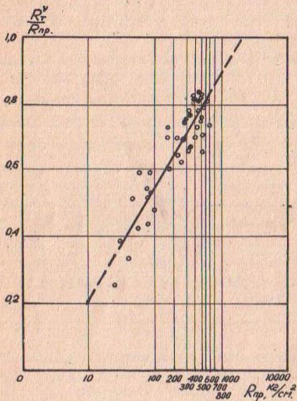
Рис.7. Граница образования микротрещин при сжатии R_T :
