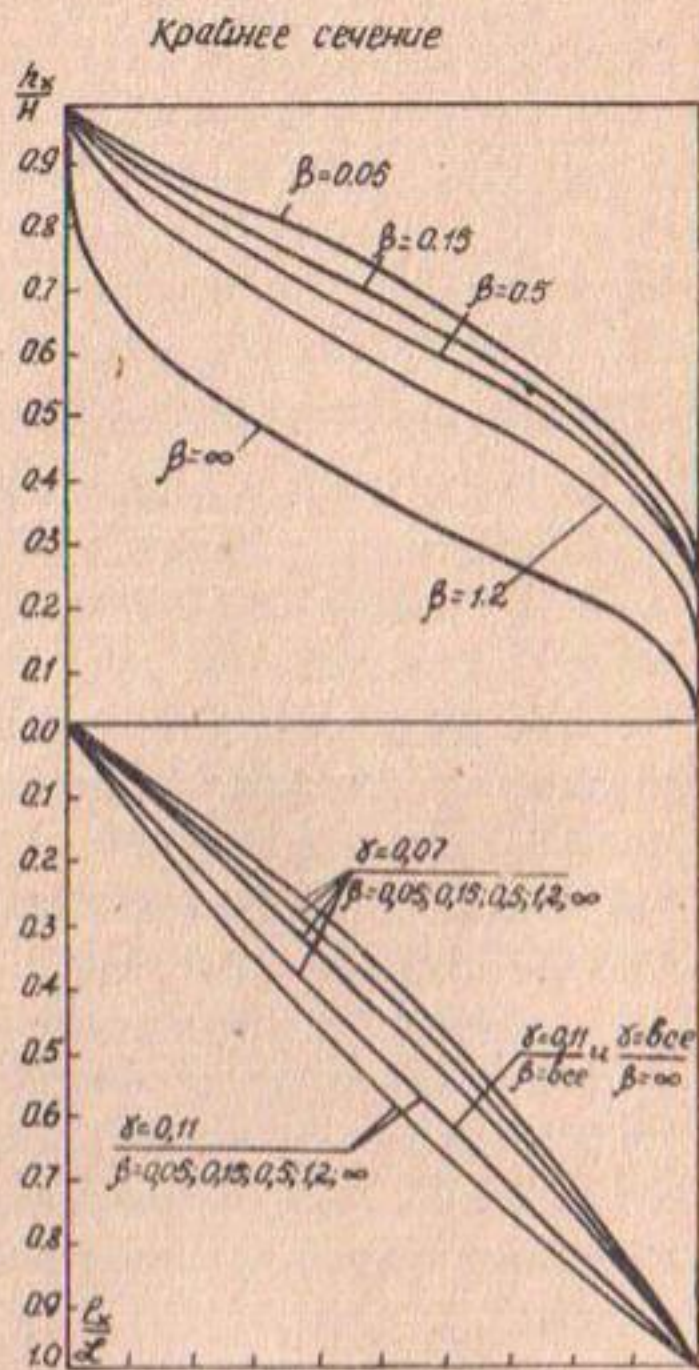
Рис. 1. Зависимости \frac{h}{H} = f_{\alpha}(\frac{l_x}{L}) по осевым и крайним сечениям водовыпусков при \alpha = 1:10 .
