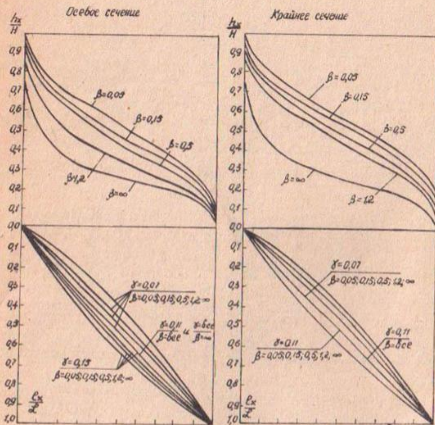
Рис. 3. Зависимости \frac{h_x}{H} = f_{\alpha} \left( \frac{l_x}{L} \right) осевым и крайним сечениям водовыпусков при \alpha = 1:100 .
