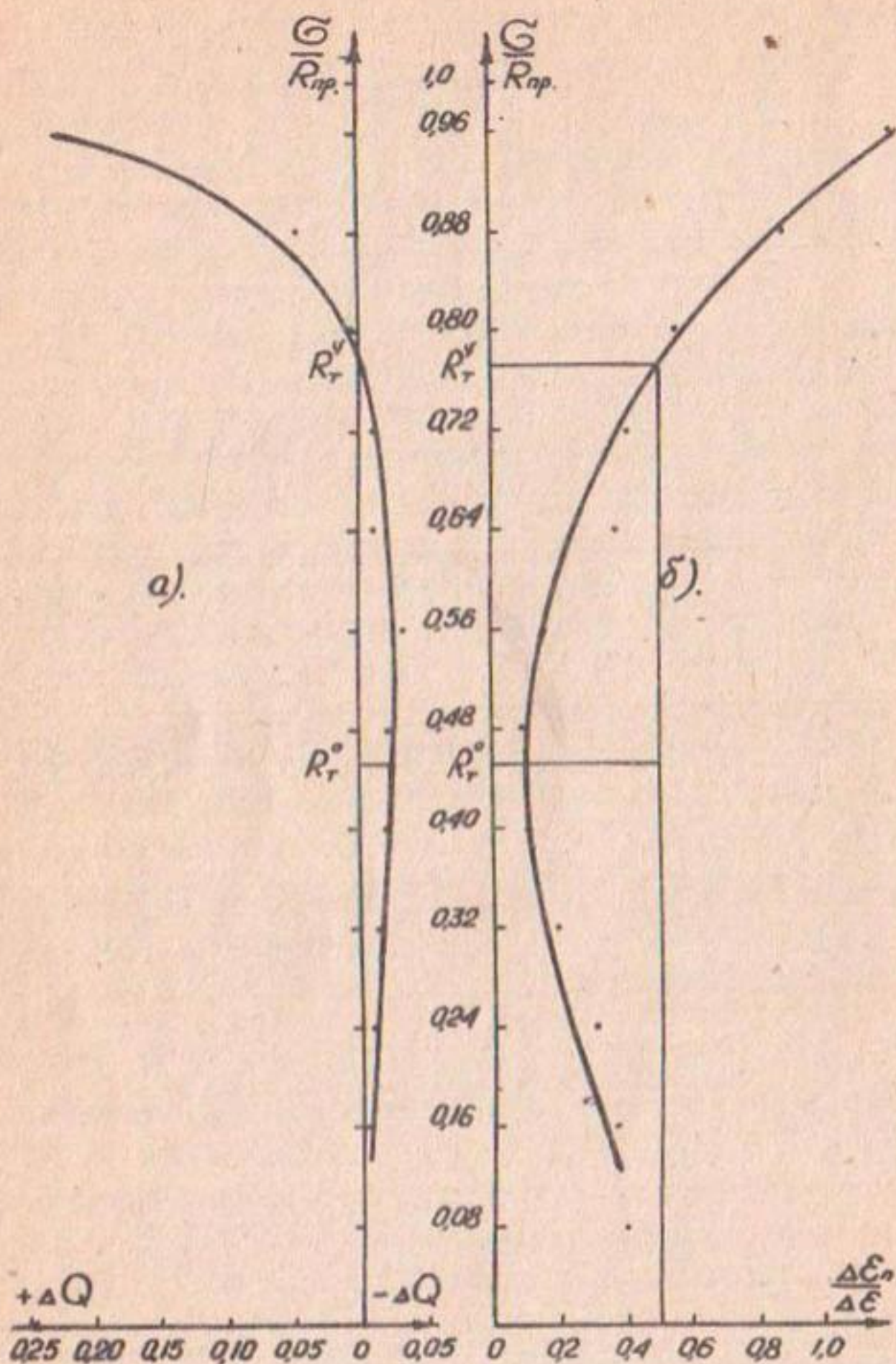
Рис.6. Зависимость от нагрузки : \alpha - приращения внешнего объема зерна K = 208 ; \delta - величины отношения \frac{\Delta \epsilon_n}{\Delta \epsilon} .
