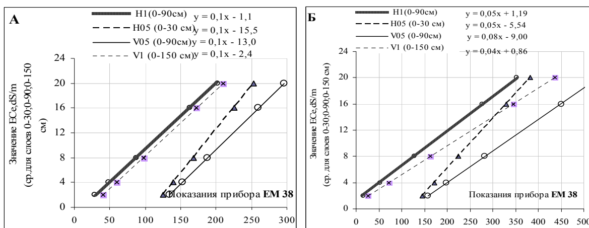
Рис. 2 - Графики для определения значений ЕС по показаниям EM38 в слоях почвы
