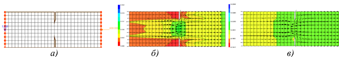
Рис. 1 - Прямоугольный участок русло с сужением
