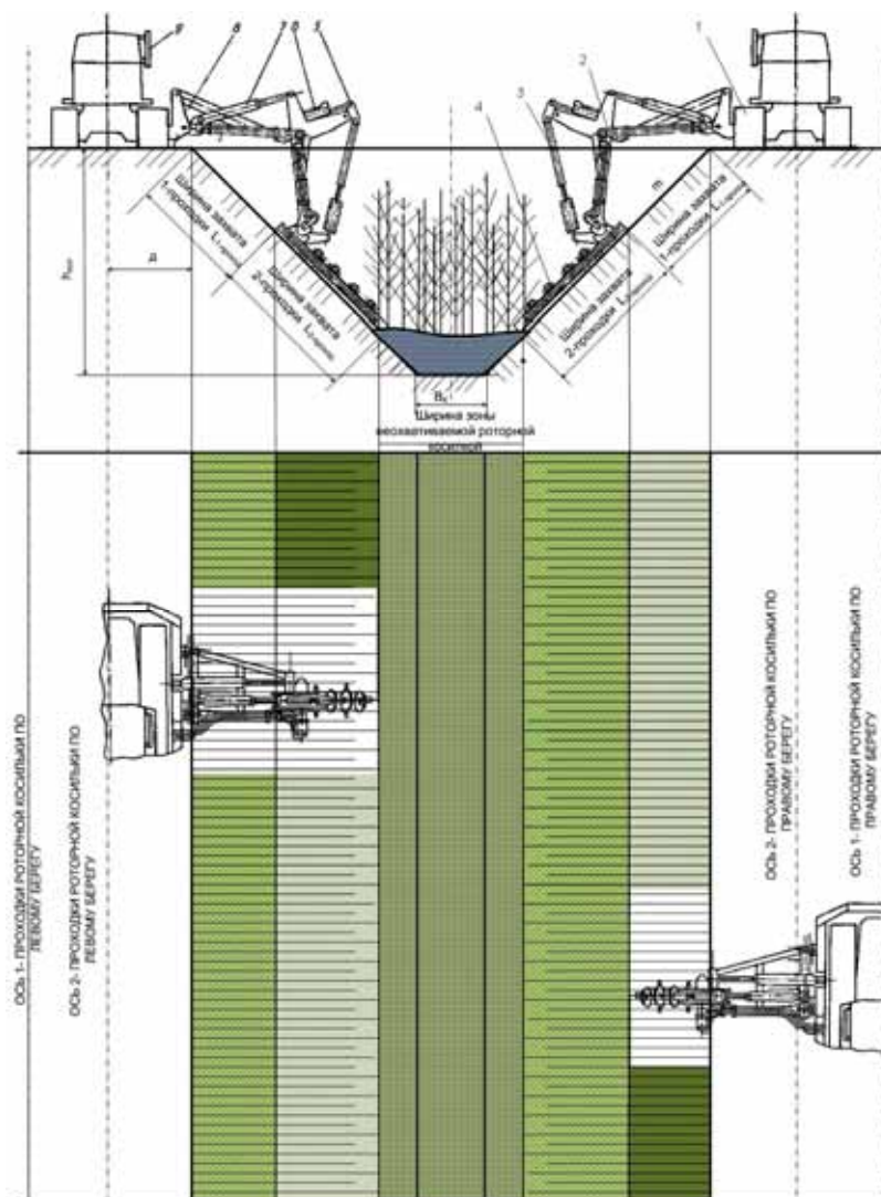
Рис. 1 - Технологическая карта окашивания коллектора навесной косилкой
