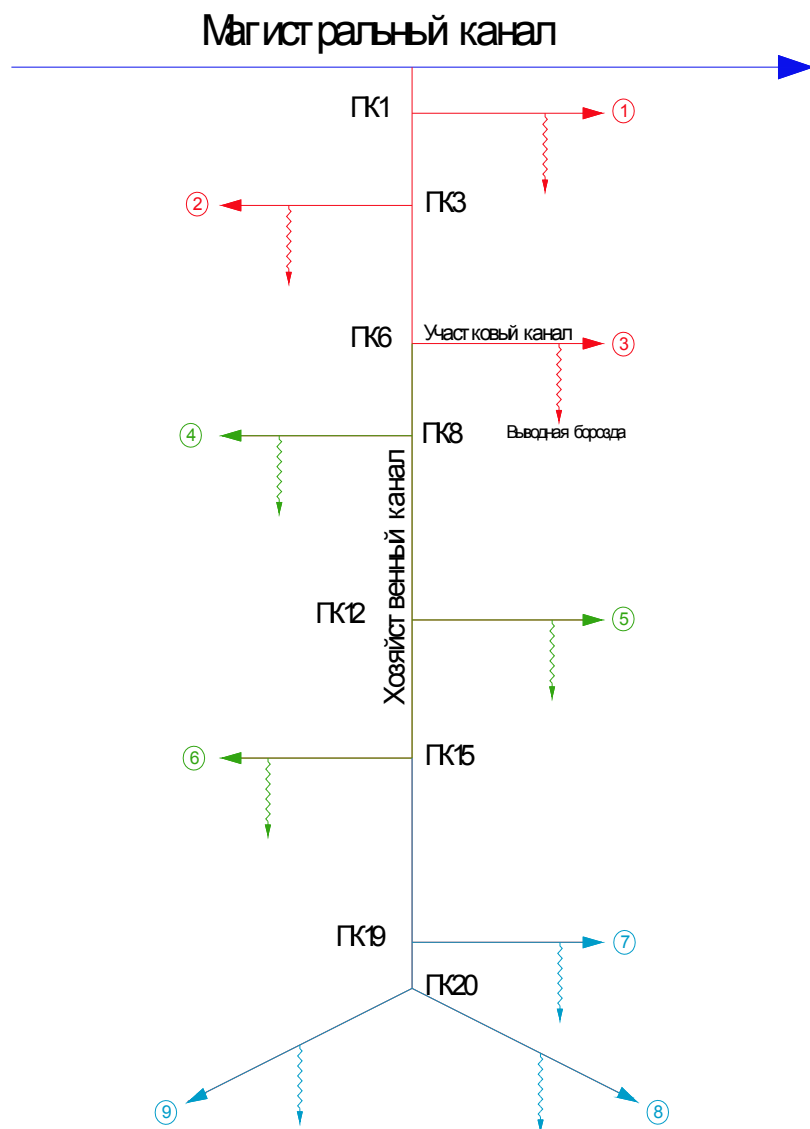
Линейная схема хозяйственного канала
