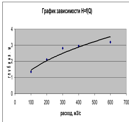
Рис. 1 - Графики зависимости H=f(Q) для левой протоки
