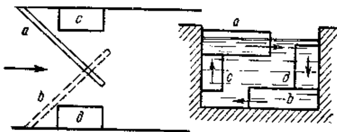
Рис. 1 - Комбинированные направляющие системы на водозаборе
