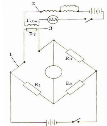
Рис. 1 - Схема измерителя скорости течения с полупроводниковым термосопротивлением
