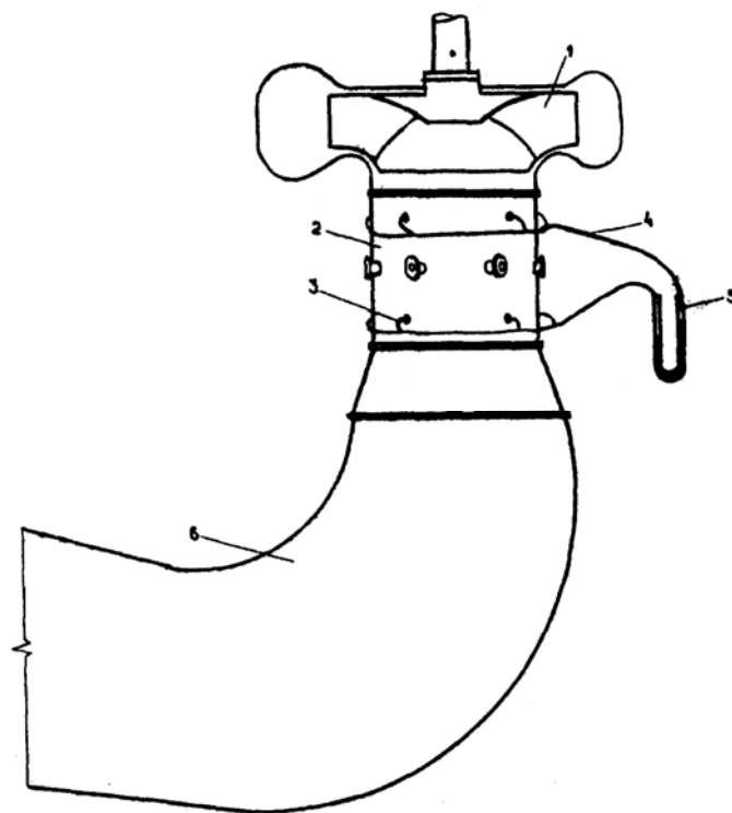
Рис.2 - Измерение давления в проточной части и всасывающей трубе насоса 2600BP 25/25:
