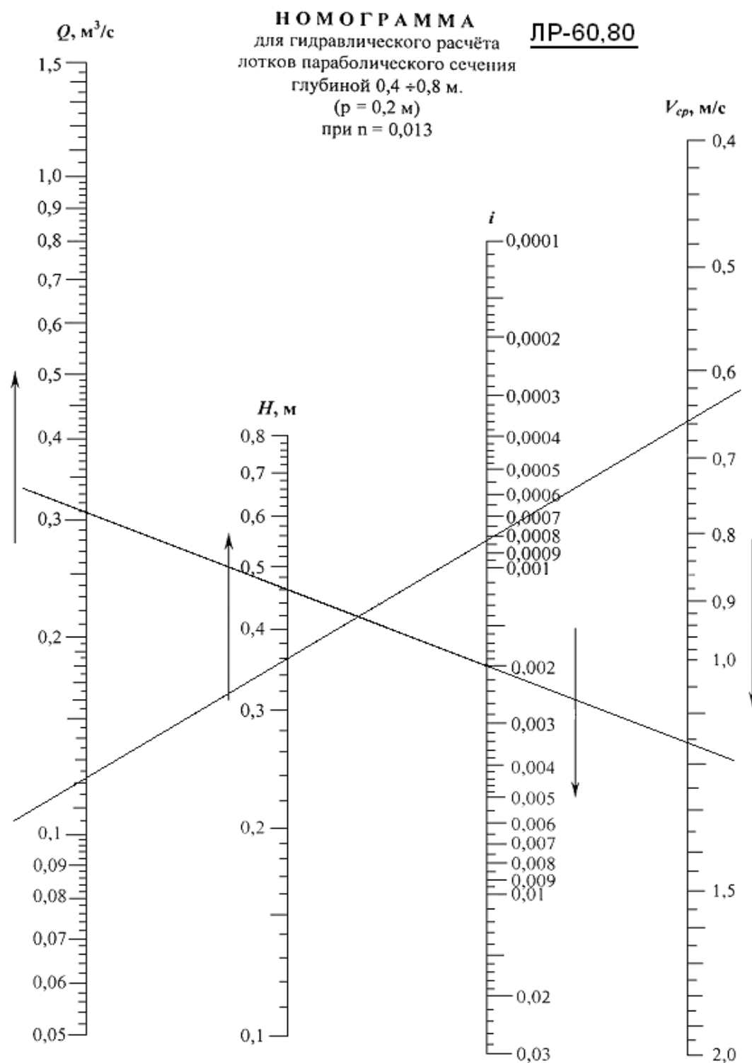
Рис. 1 - Номограмма для гидравлического расчёта параболических лотков ЛР-60 и ЛР-80.
