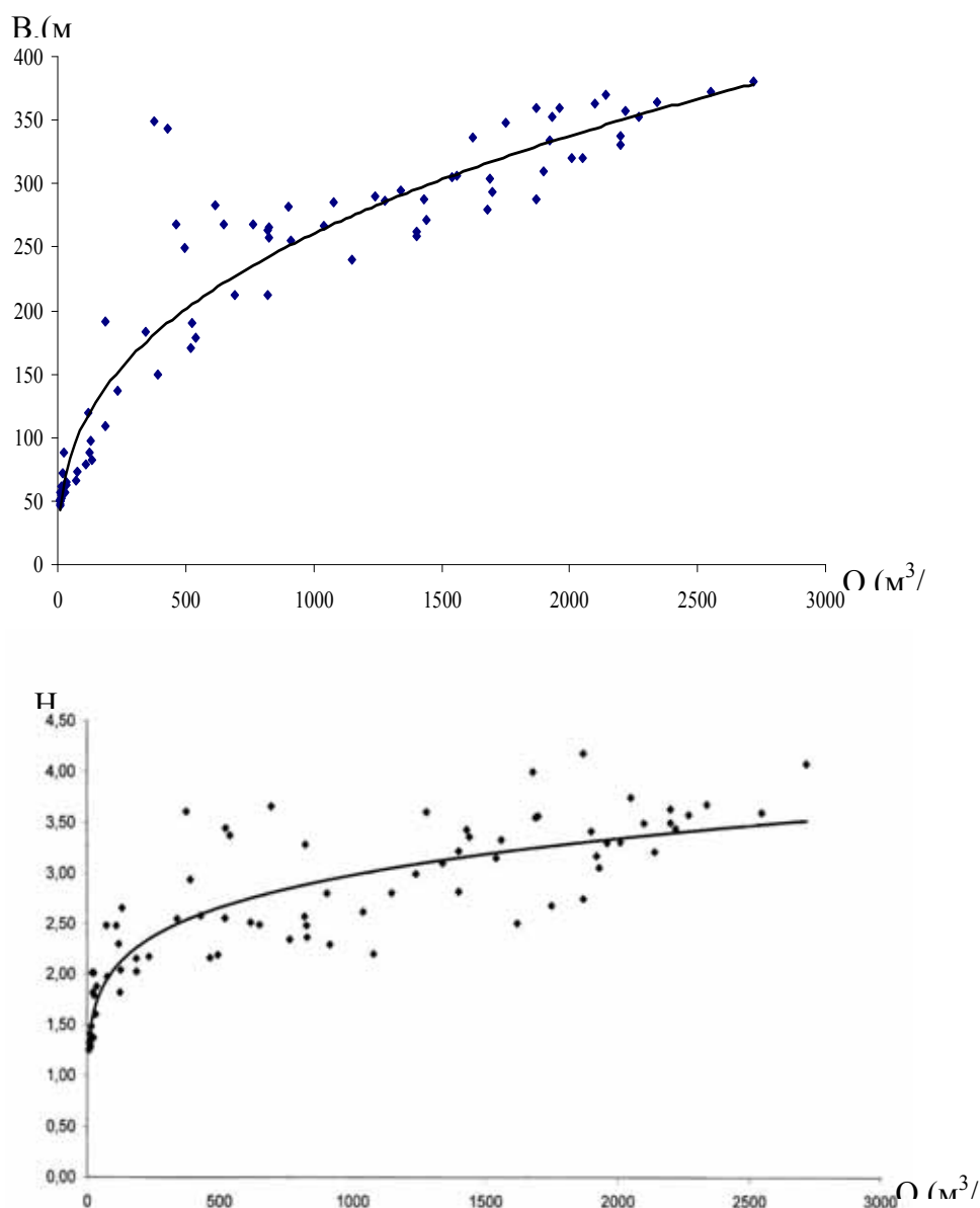
Рисунок-1. Графики B=f(Q) , H=f(Q) для нижнего течения р. Амударьи в условиях зарегулированного стока воды.
