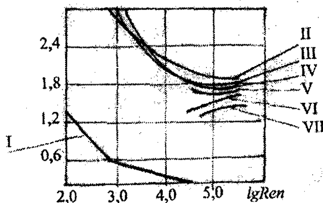
Рис. 2 - Зависимость коэффициента гидравлического сопротивления от Re для русел:
