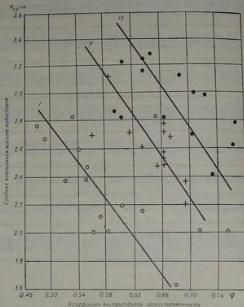
Рис. 75. Зависимость коэффициента внутригодовой зарегулированности стока \varphi от средней высоты водосборов H_{cp} . I — реки североферганского района, II — реки верхнечирчикского района, III — реки южноферганского района.
