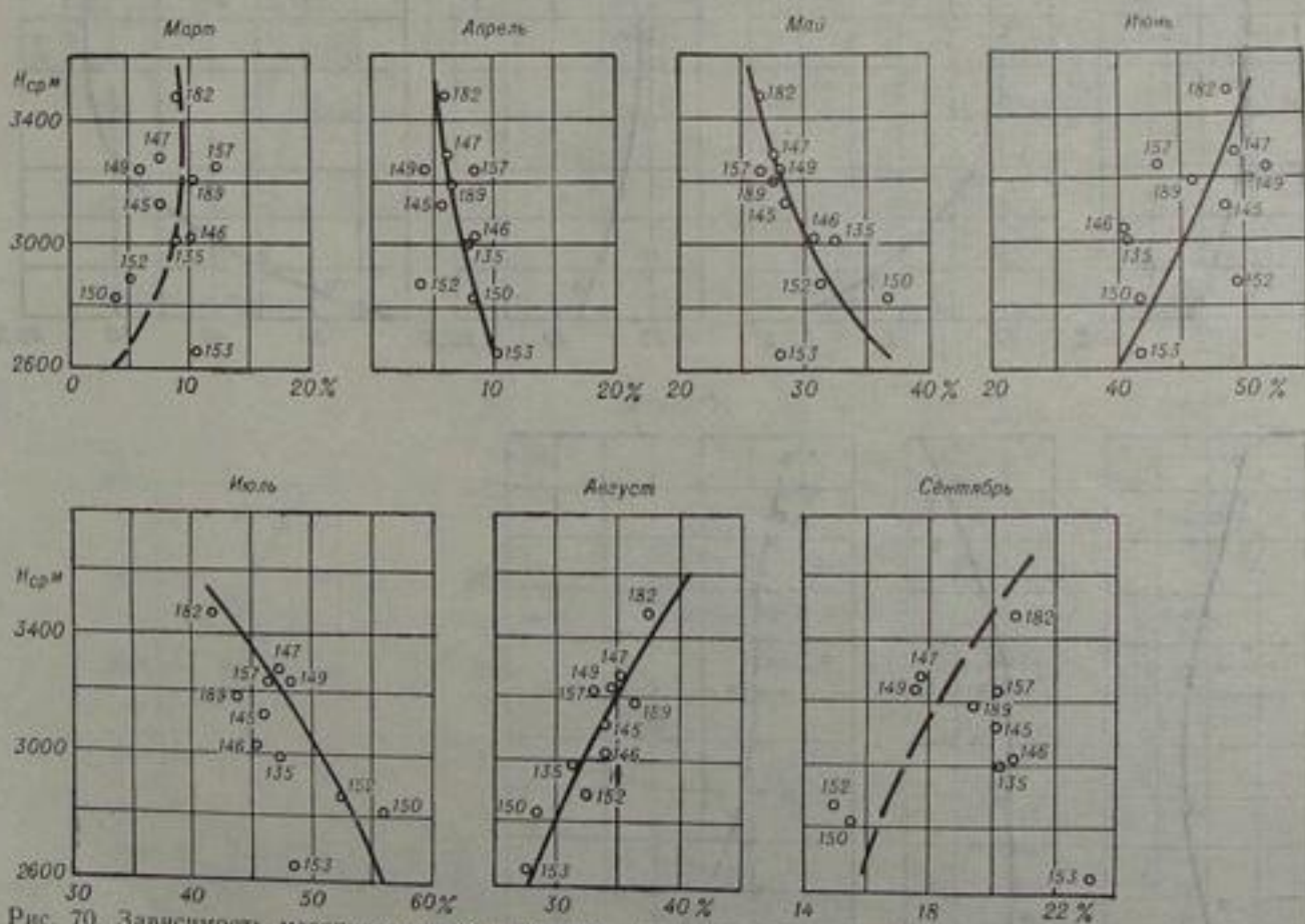
Рис. 70. Зависимость месячного стока весеннего и летнего сезонов (в % от сезонного) от средневзвешенной высоты водосбора H_{cp} для рек III района.
