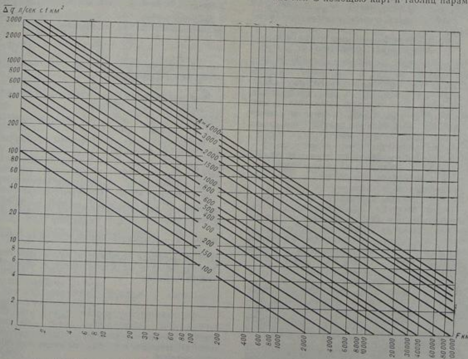
Рис. 95. Номограмма для вычисления дождевой надбавки \Delta \bar{q} к наибольшим расходам талых вод.
