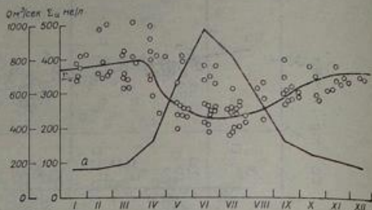
Рис. 156. Внутригодовое изменение минерализации ( \Sigma\text{и} ) и расходов воды ( Q ) р. Нарына по посту у кишла. Учкурган по многолетним данным.
