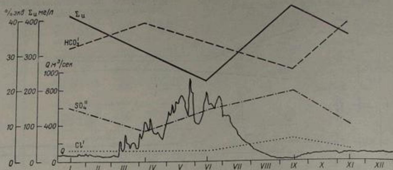
Рис. 167. Внутригодовое изменение минерализации ( \Sigma_a ) и содержания главных анионов в воде р. Чирчик у с. Чиназ за 1942 г.
