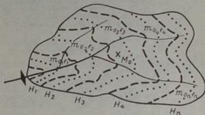
Рис. 43. Схема разбивки горного речного бассейна на высотные зоны для вычисления зональных модулей стока ( m_0 ).
