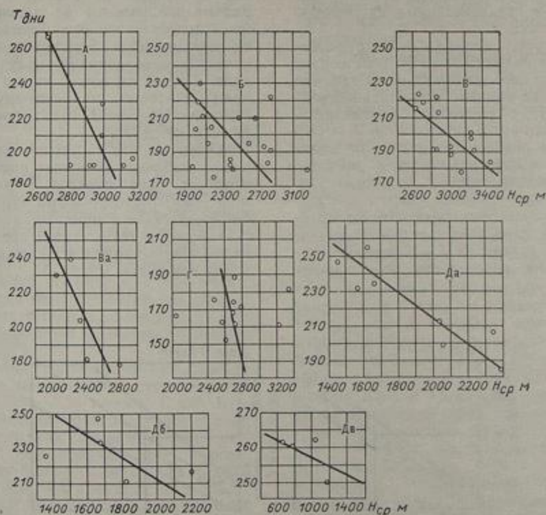
Рис. 100. Зависимость средней продолжительности меженного периода ( I ) от средней высоты водосборов ( H_{ср} ).
