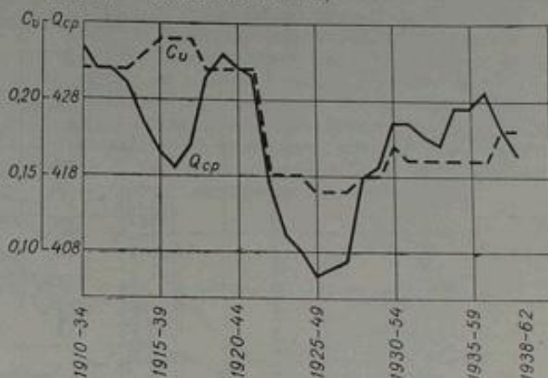
Рис. 35. Графики колебания среднегодовых расходов воды и их коэффициентов вариации по р. Нарын в створе кишл. Учкурган по скользящим 25-летиям за 1910—1962 гг.
