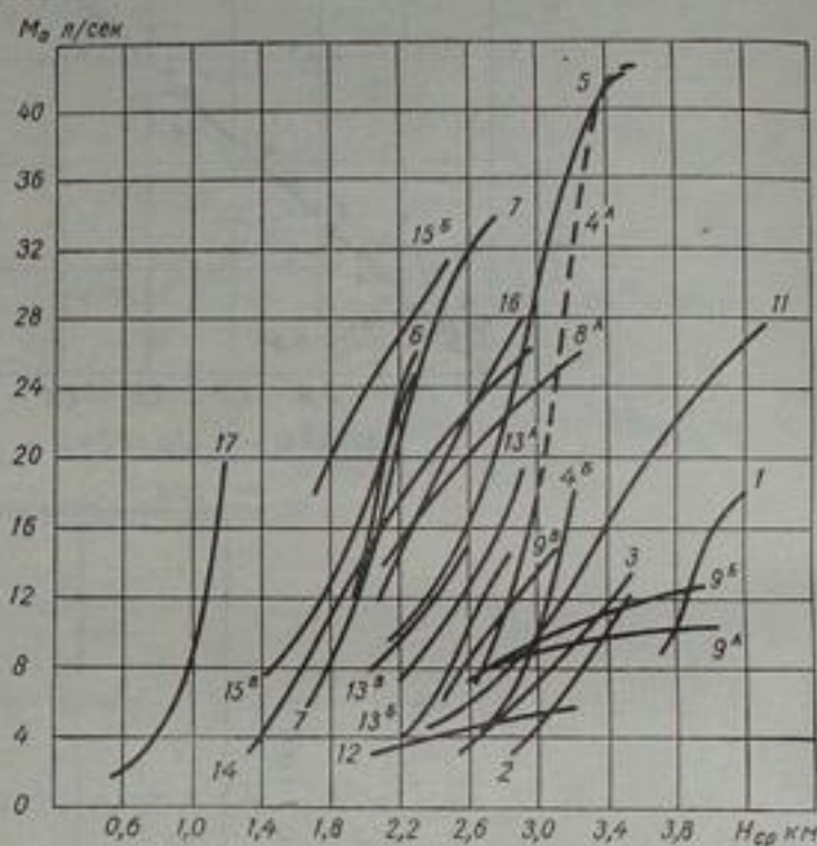
Рис. 42. Зависимости модуля стока M_0 от средней взвешенной высоты водосборов по рекам бассейна Сыр-Дарьи. Цифры у кривых — номера районов.
