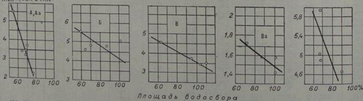
Рис. 103. Зависимость месячного модуля минимального стока ( M_{min} ) от относительной площади водосбора, сложенной слабо водопроницаемыми горными породами.
