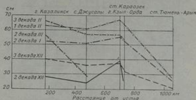
Рис. 126. Изменение средней многолетней толщины льда по длине р. Сыр-Дарья.
