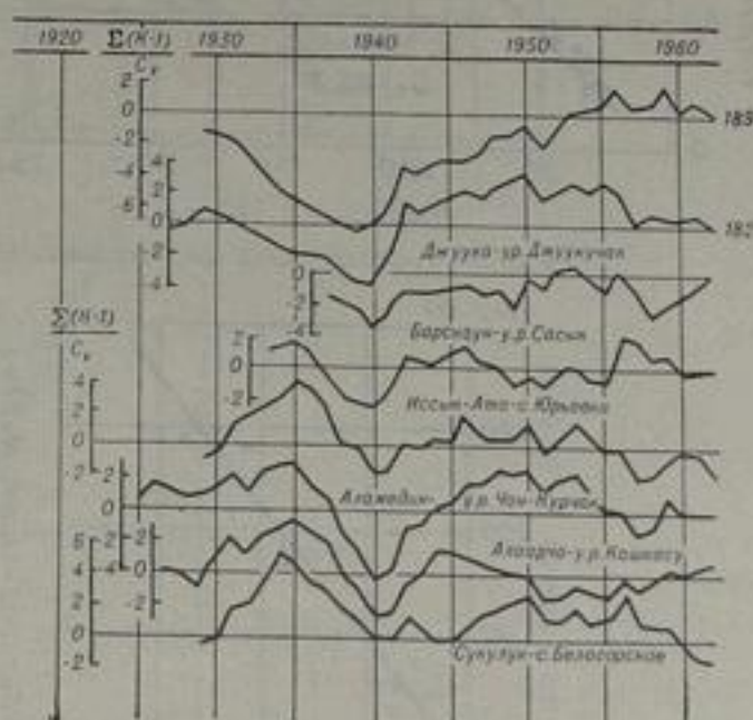
Рис. 38. Разностные интегральные кривые колебаний годового стока воды по рекам III группы с показателем типа питания \delta более 2.
