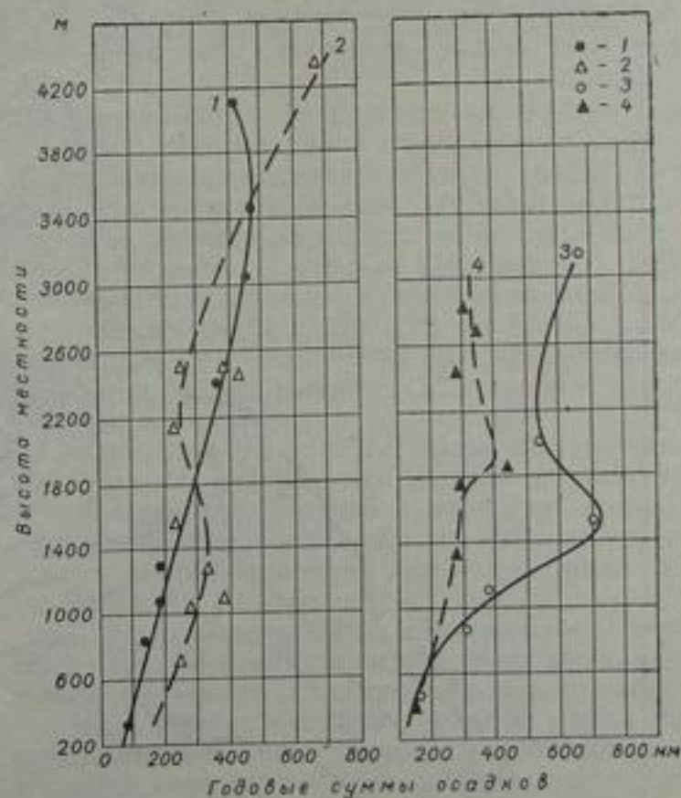
Рис. 6. Зависимость средней годовой суммы осадков от высоты местности на профилях по долинам рек.
