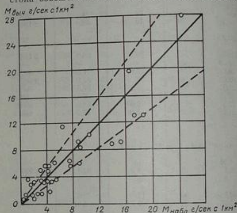
Рис. 133. Связь модулей стока взвешенных наносов, вычисленных по формуле и по данным фактических наблюдений.
