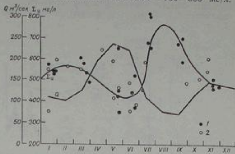
Рис. 157. Внутригодовое изменение минерализации и расходов воды в нижнем течении р. Карадарья по многолетним данным.
