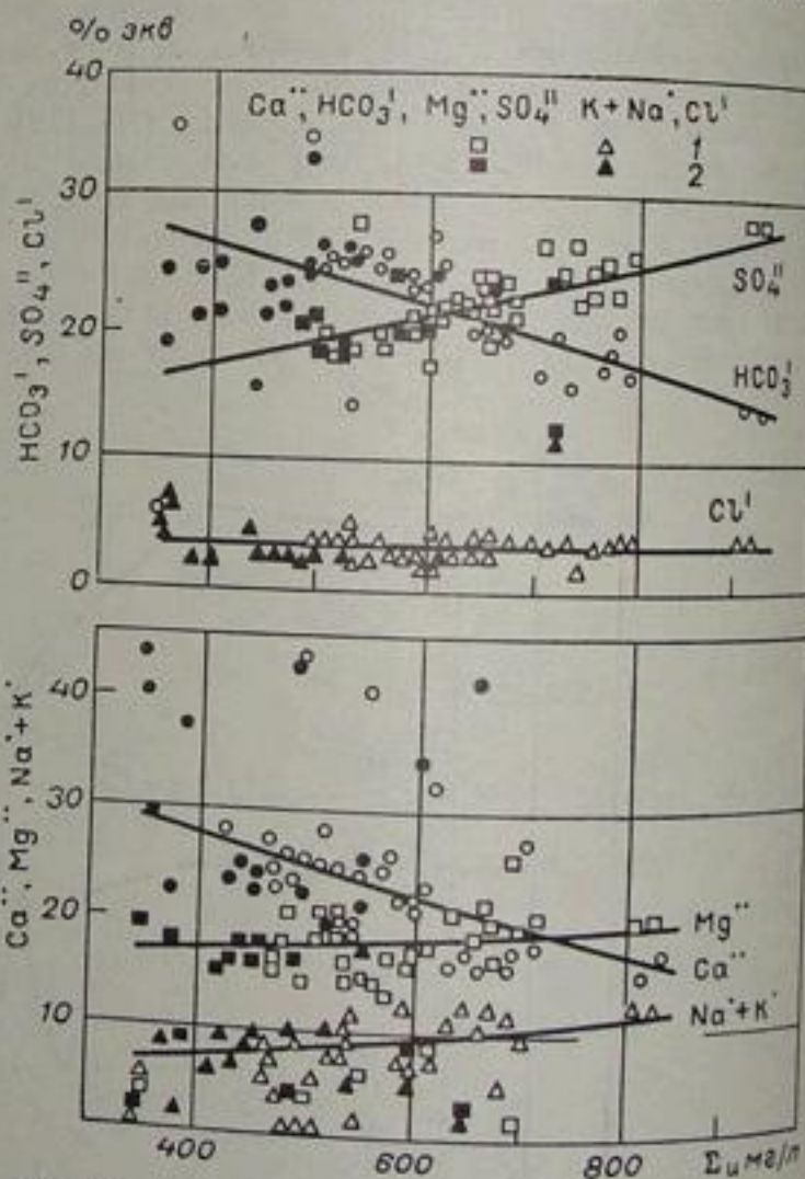
Рис. 160. Характер связи между величиной минерализации воды ( \Sigma_{и} ) и содержанием главных анионов и катионов (% экв) по р. Карадарье у кишл. Учтепе. 1 — для периода межени, 2 — для периода половодья.
