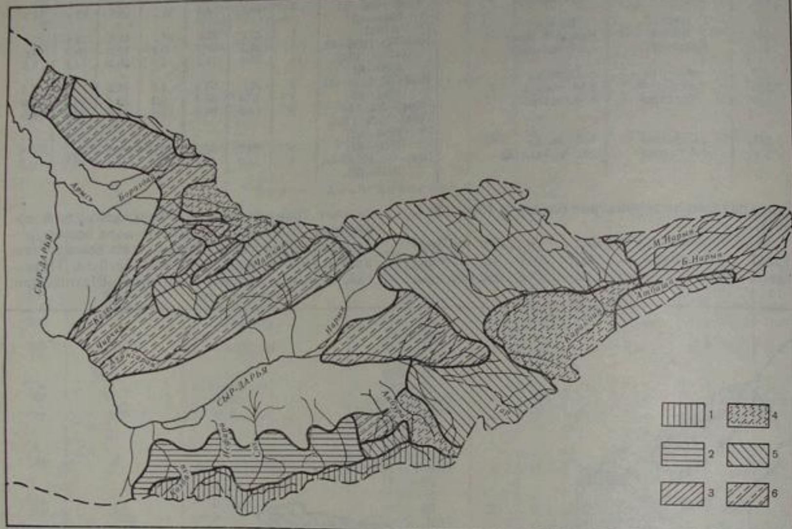
Рис. 140. Схематическая карта распределения стока взвешенных наносов за март—июнь (в % от годового). 1 — 10—20%, 2 — 20—30%, 3 — 30—40%, 4 — 40—60%, 5 — 60—80%, 6 — 80—100%.
