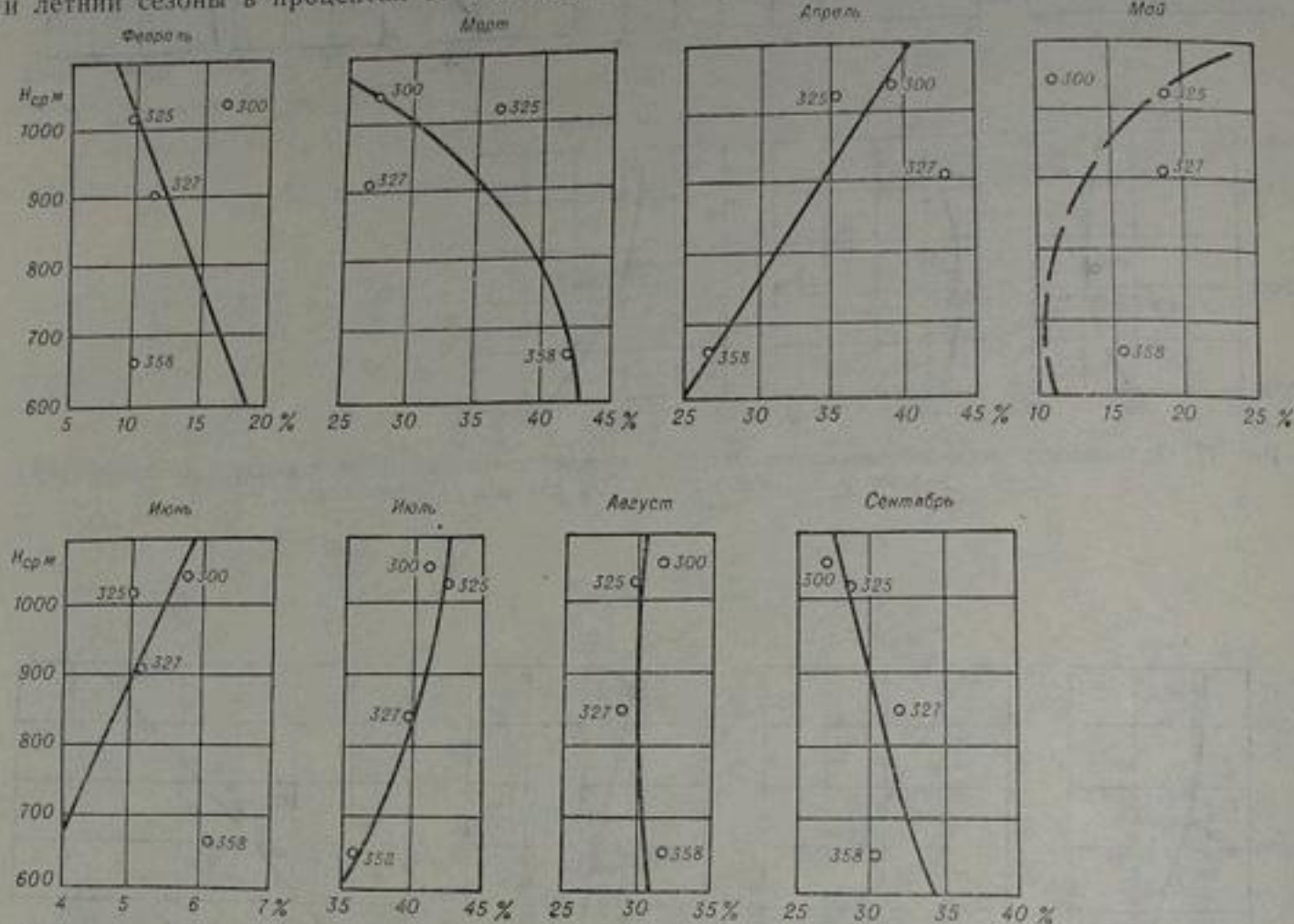
Рис. 73. Зависимость месячного стока весеннего и летнего сезонов (в % от сезонного) от средневзвешенной высоты водосбора H_{ср} для рек VI района.
