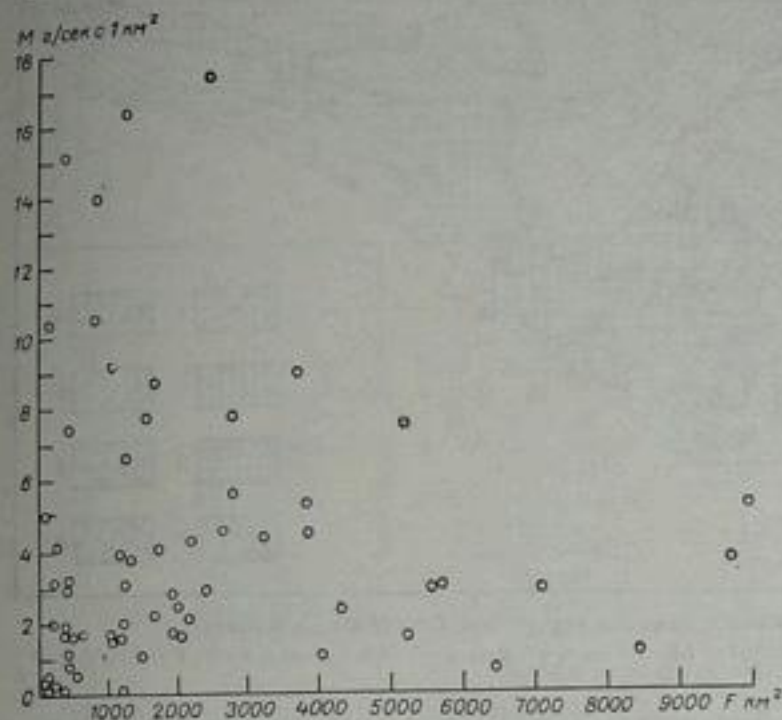
Рис. 134. Зависимость модуля стока взвешенных наносов (М) от площади бассейна.
