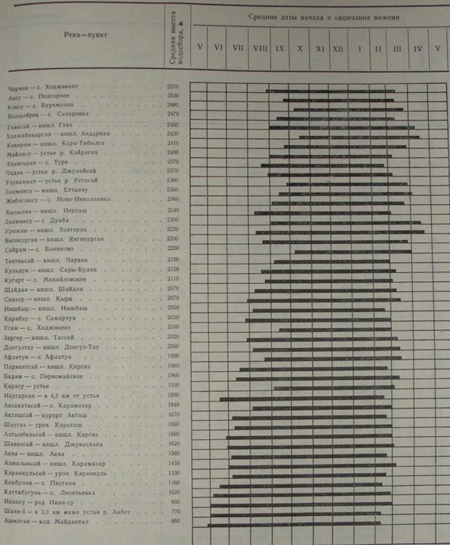
Рис. 96. Средние даты начала и окончания межени.
