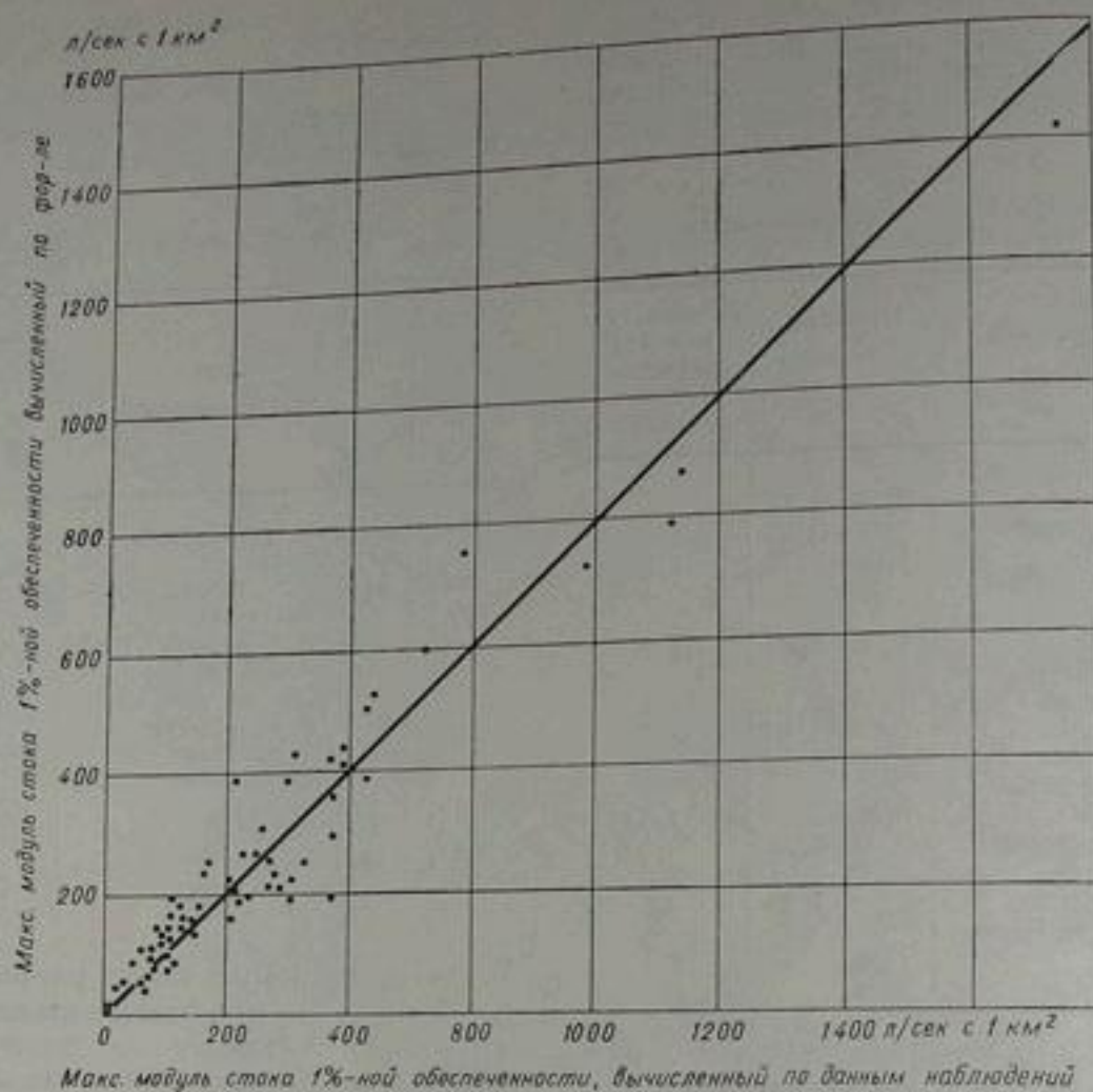
Рис. 92. Связь максимальных модулей стока, вычисленных по формулам и по данным наблюдений.
