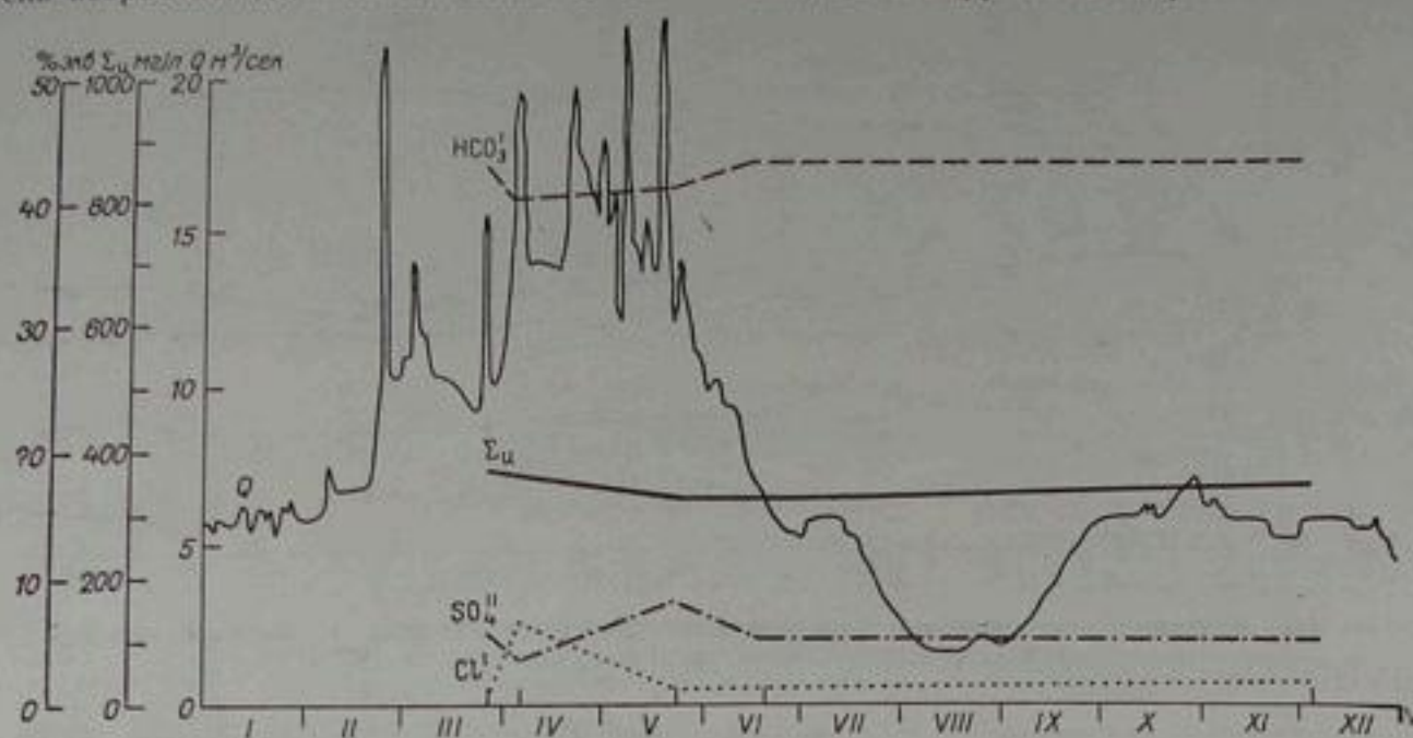
Рис. 170. Внутригодовое изменение минерализации ( \Sigma_{и} ) и содержания главных анионов в воде р. Арысь у с. Балыкчи за 1960 г.
