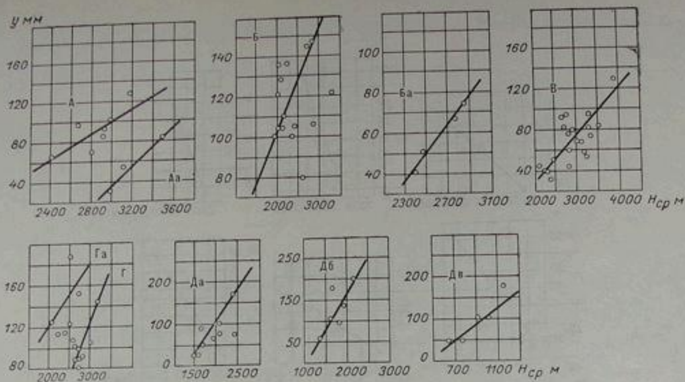
Рис. 101. Зависимость слоя стока воды за меженный период ( y ) от средней высоты водосборов ( H_{cp} ).
