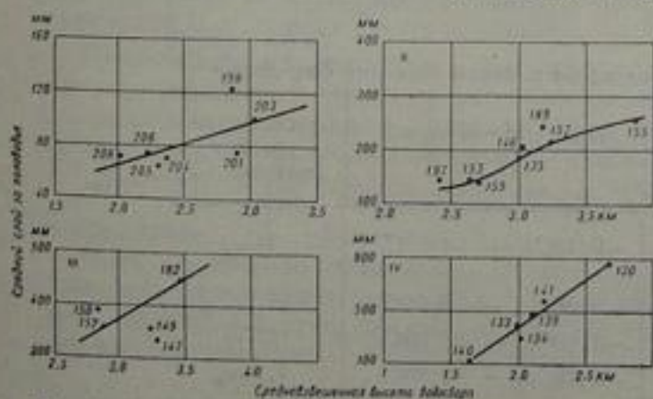
Рис. 81. Зависимость среднего многолетнего слоя стока за половодье от высоты водосборов для рек Туркестано-Алайского и Ферганского хребтов (I—IV районы).
