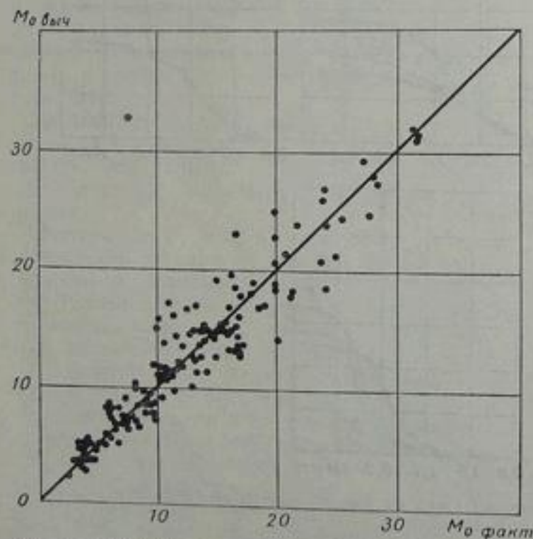
Рис. 47. Сравнение вычисленных на основе зависимостей m_0 = f(H) значений M_0 с фактически наблюдаемыми.
