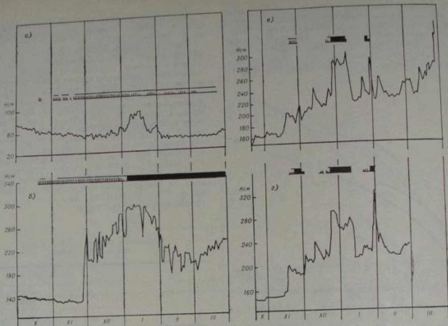
Рис. 31. Ход уровня воды на реках в период осенне-зимней межени 1957-58 г., искаженный ледовыми явлениями. а — р. Нарын — г. Нарын; б — р. Большой Нарын — устье; в — р. Армыс — с. Шаульдер; г — р. Бугунь — Красный мост.
