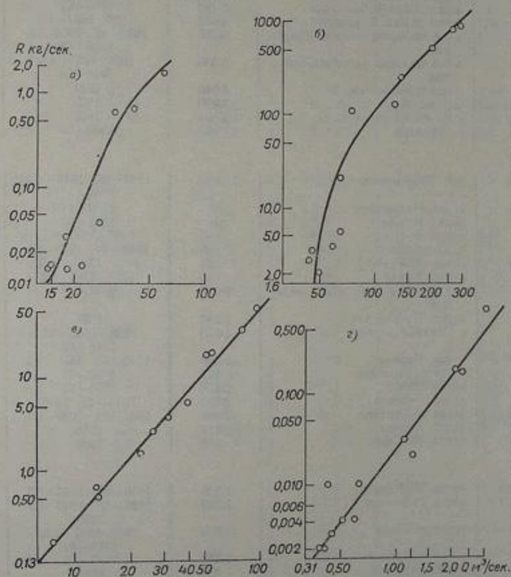
Рис. 132. Зависимость среднемесячных средних многолетних расходов наносов от расходов воды.
