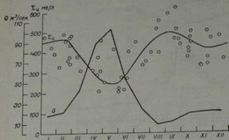
Рис. 163. Внутригодовое изменение минерализации ( \Sigma_{и} ) и расходов воды ( Q ) в р. Ахангаран у с. Самарское по данным многолетних наблюдений.
