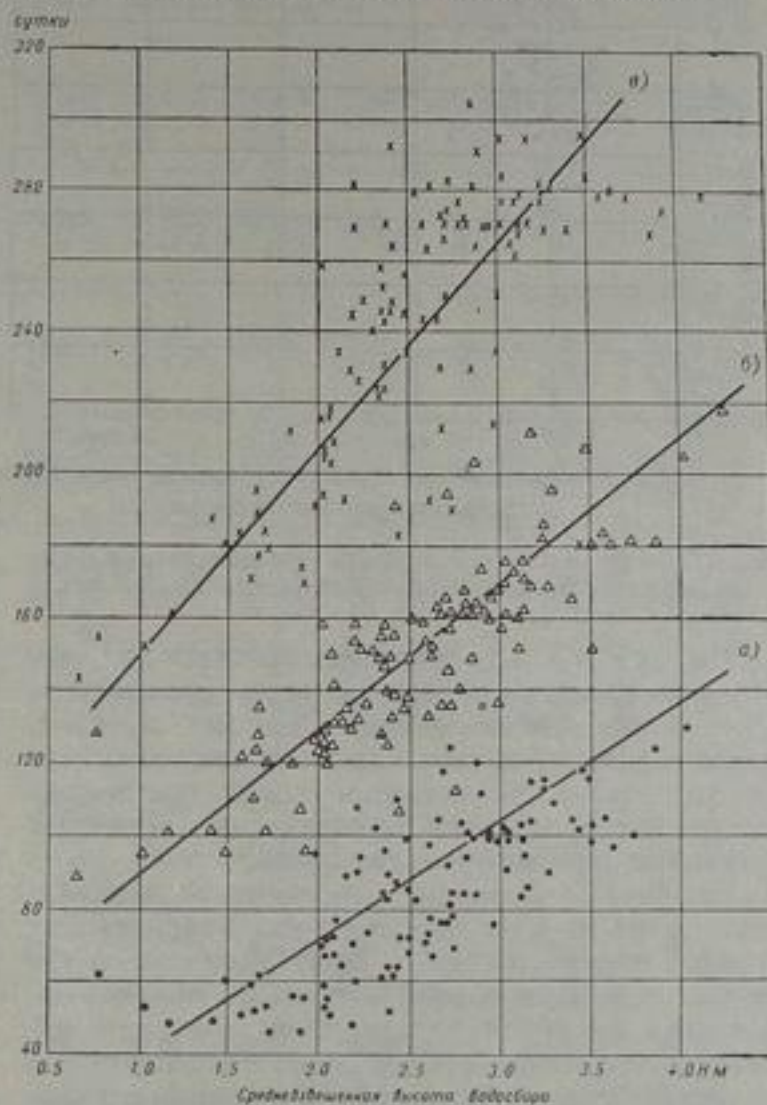
Рис. 76. Зависимость времени прохождения половодья от средней высоты водосборов. а — среднее время (отсчитываемое от 1/1) начала половодья, б — то же наибольшего расхода, в — то же конца половодья.
