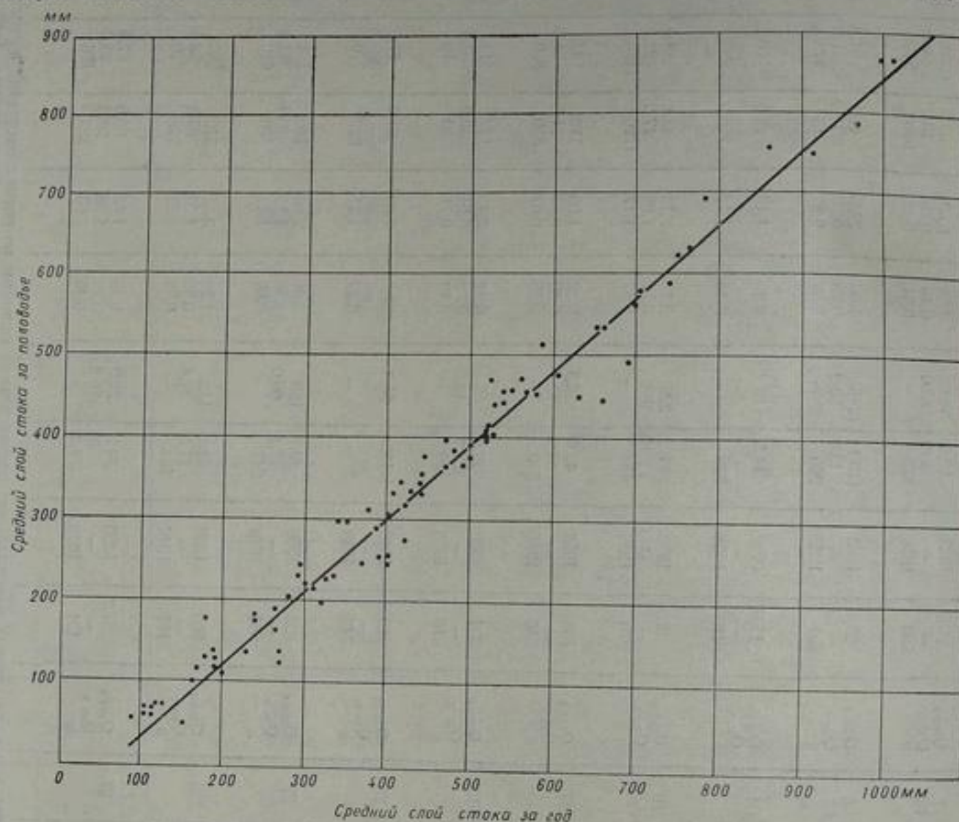
Рис. 79. Связь между нормой стока за половодье и нормой годового стока.
