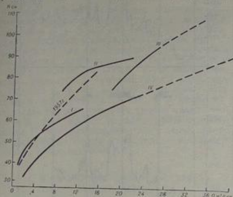
Рис. 29. Кривые расходов р. Падшаата — устье р. Тосту за 1958 г.
