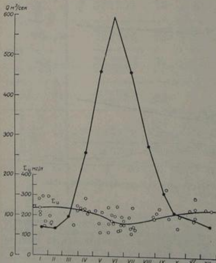
Рис. 168. Внутригодовое изменение минерализации ( \Sigma_a ) и расходов воды (Q) в р. Чирчик у с. Ходжикент по многолетним данным.
