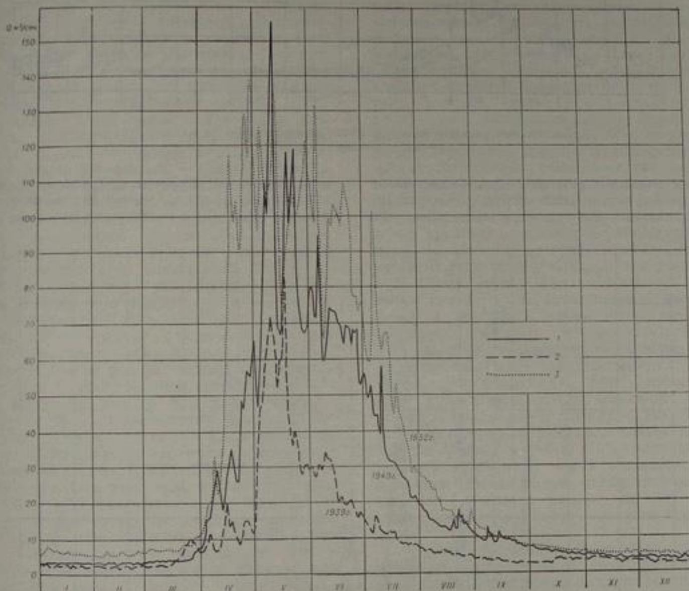
Рис. 17. Гидрографы стока р. Ясы за характерные по водоносности годы. 1 — 1940 г., 2 — 1939 г., 3 — 1952 г.
