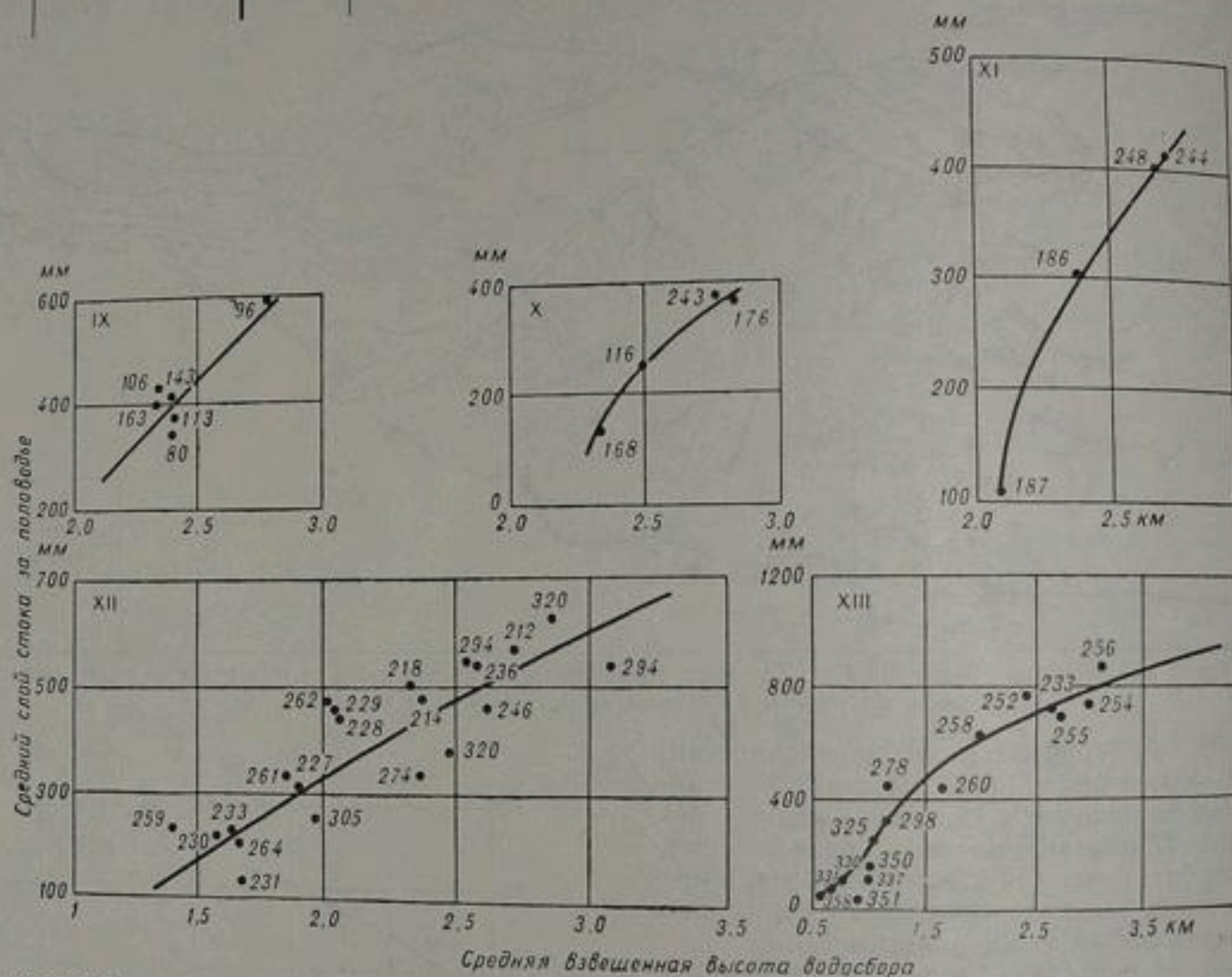
Рис. 83. Зависимость среднего многолетнего слоя стока за половодье от средней высоты водосборов для рек IX—XIII районов.
