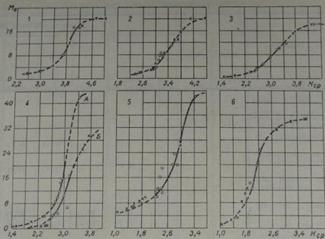
Рис. 48. Районные зависимости модуля стока M_0 от средней высоты водосборов ( H_{cp} ) по рекам бассейна Нарына. 1-6 — номера районов.
