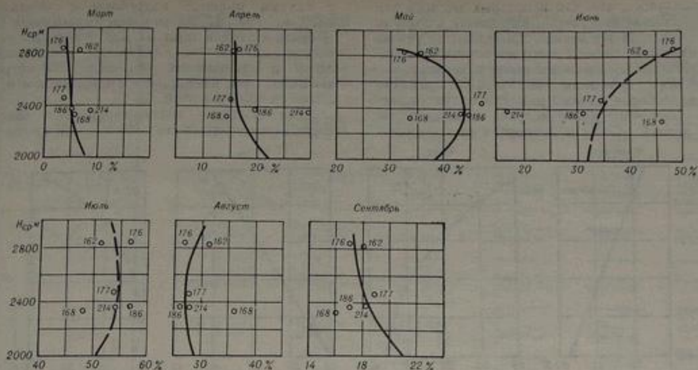
Рис. 71. Зависимость месячного стока весеннего и летнего сезонов (в % от сезонного) от средневзвешенной высоты водосбора H_{cp} для рек IV района.
