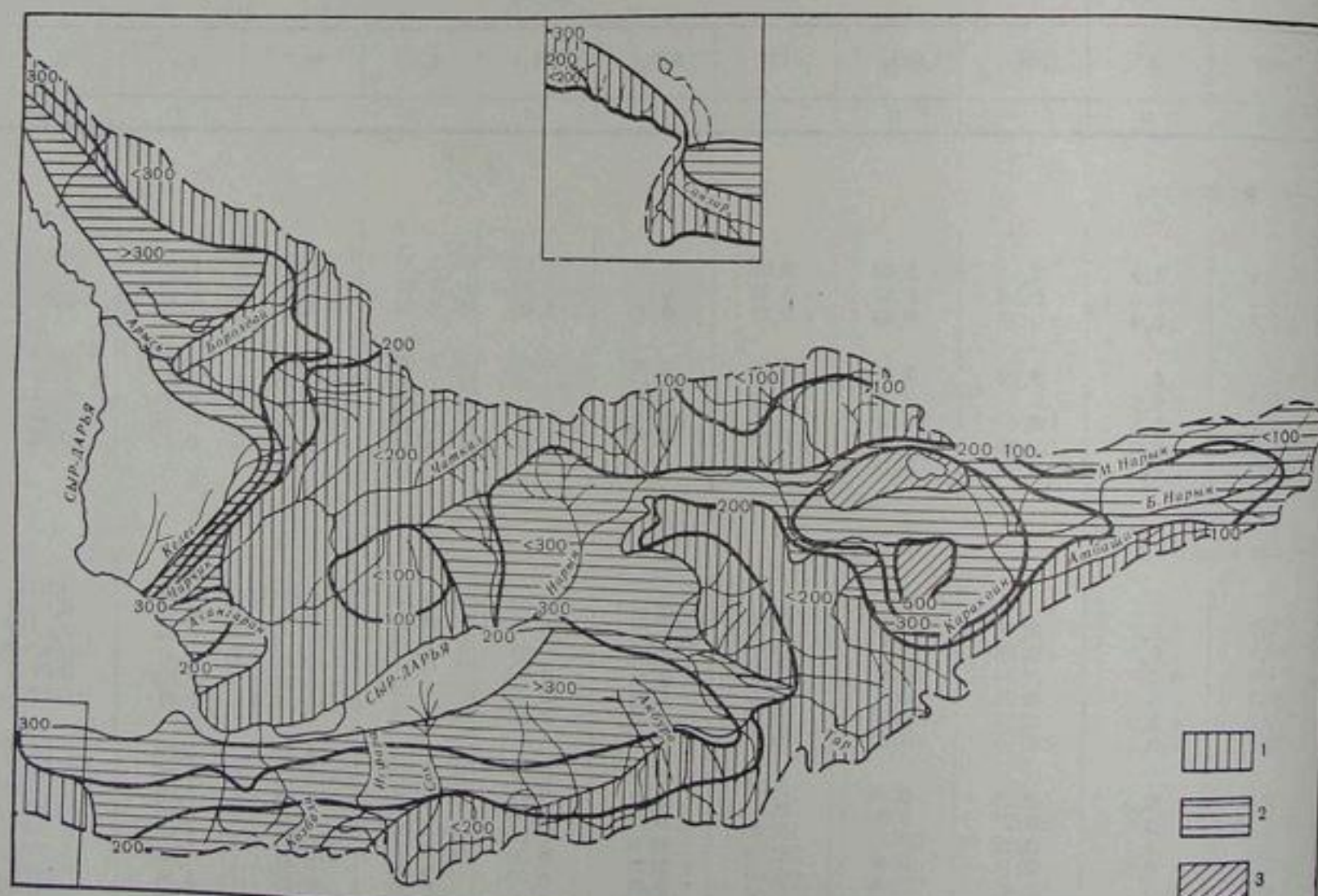
Рис. 151. Минерализация воды и содержание HCO 3 ' в реках бассейна Сыр-Дарьи в период половодья. 1 — 44—36% экв HCO 3 ', 2 — 36—28% экв HCO 3 ', 3 — <28% экв HCO 3 '.
