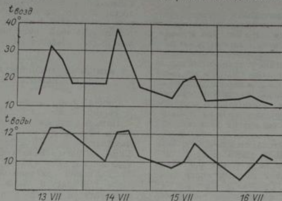
Рис. 112. Суточный ход температуры воды и воздуха на посту р. Большой Нарын — устье, 13—16/VII 1958 г.
