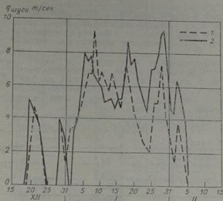
Рис. 129. Совмещенный график ежедневных расходов шуги ( q_{\text{шуги}} ) по постам на р. Нарын за зиму 1959-60 г. 1 — кишл. Учкурган, 2 — ст. Верхне-Учкурганская.
