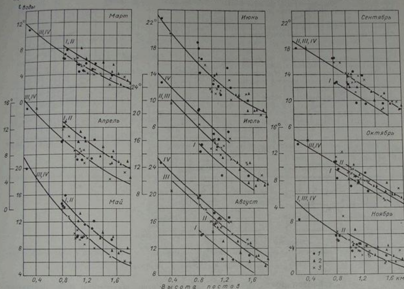
Рис. 116. Графики зависимости многолетней среднемесячной температуры воды от высоты постов по рекам Ферганской долины и бассейна р. Ахангаран.
