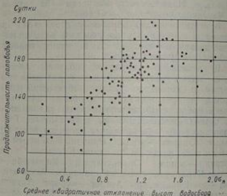
Рис. 78. Зависимость продолжительности половодья от среднего квадратичного отклонения высот водосбора.
