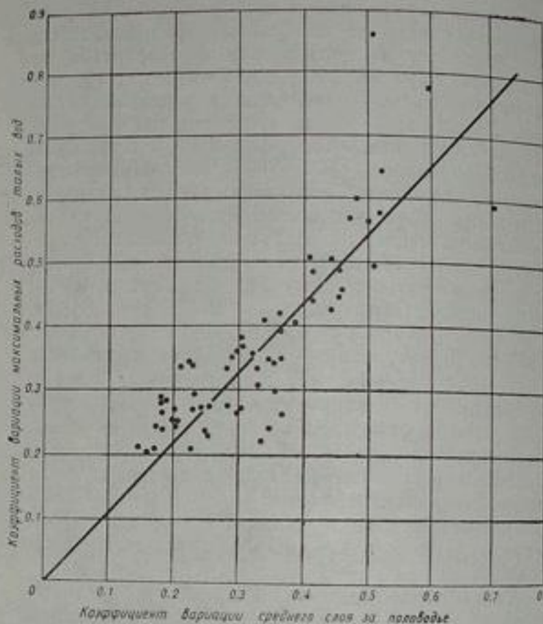
Рис. 86. Зависимость коэффициентов вариации наибольших расходов талых вод от коэффициентов вариации расхода за половодье.
