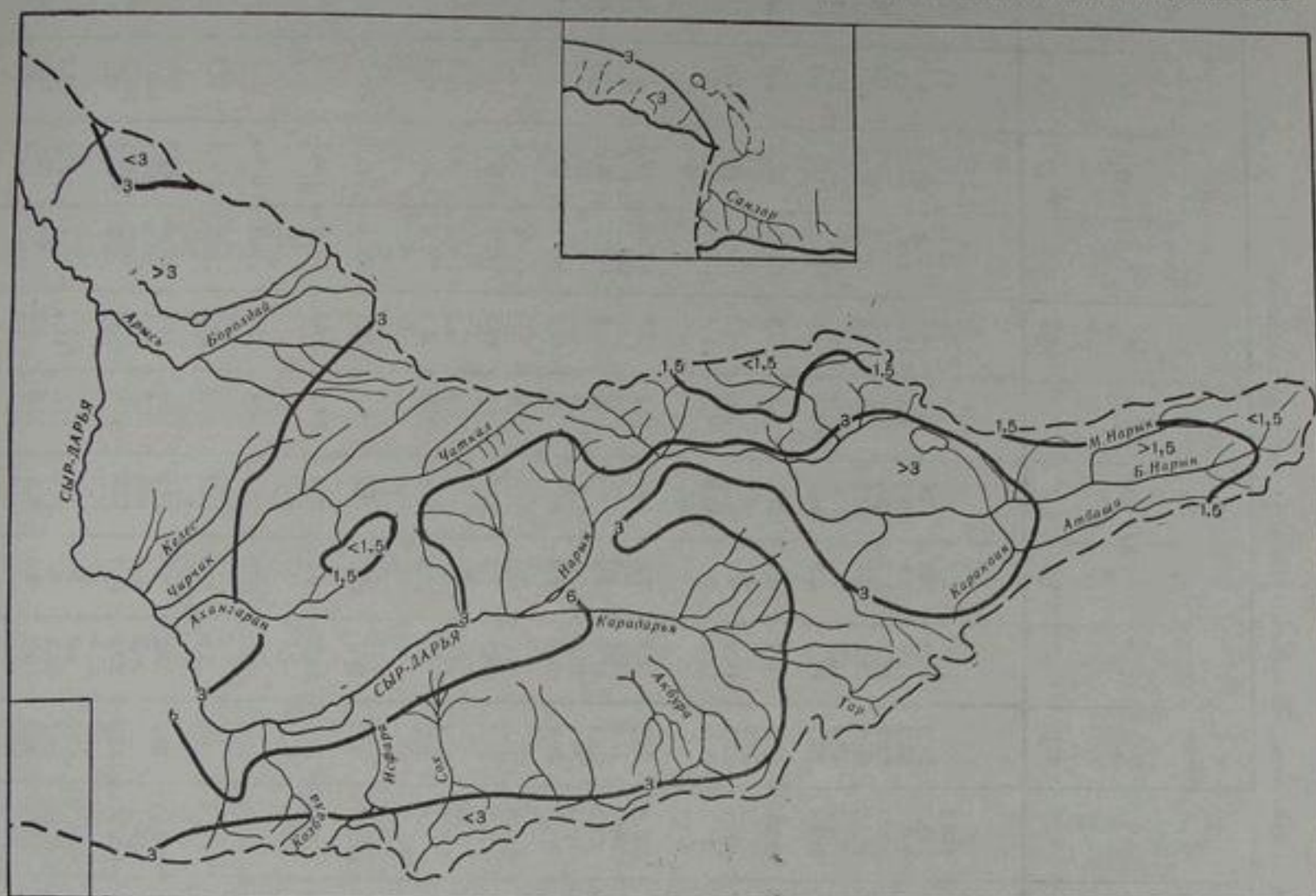
Рис. 154. Величина общей жесткости речной воды (мг-экв/л) в бассейне р. Сыр-Дарьи в период межени.
