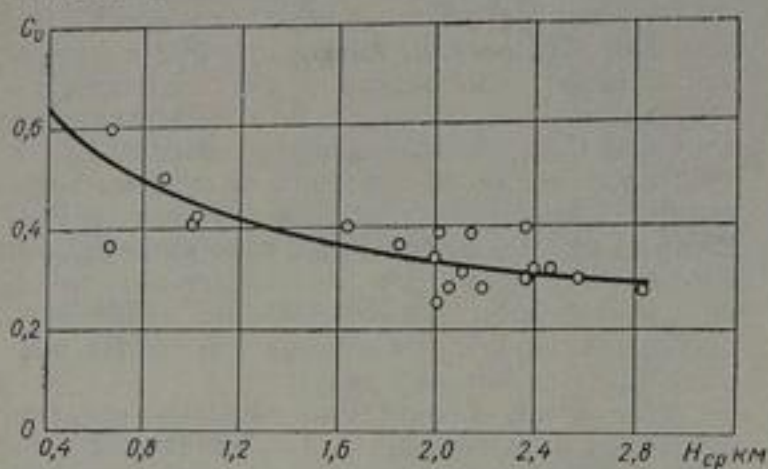
Рис. 60. Зависимость коэффициента вариации годового стока ( C_v ) от средневзвешенной высоты водосбора H_{ср} для рек с показателем типа питания \delta < 0,4 .
