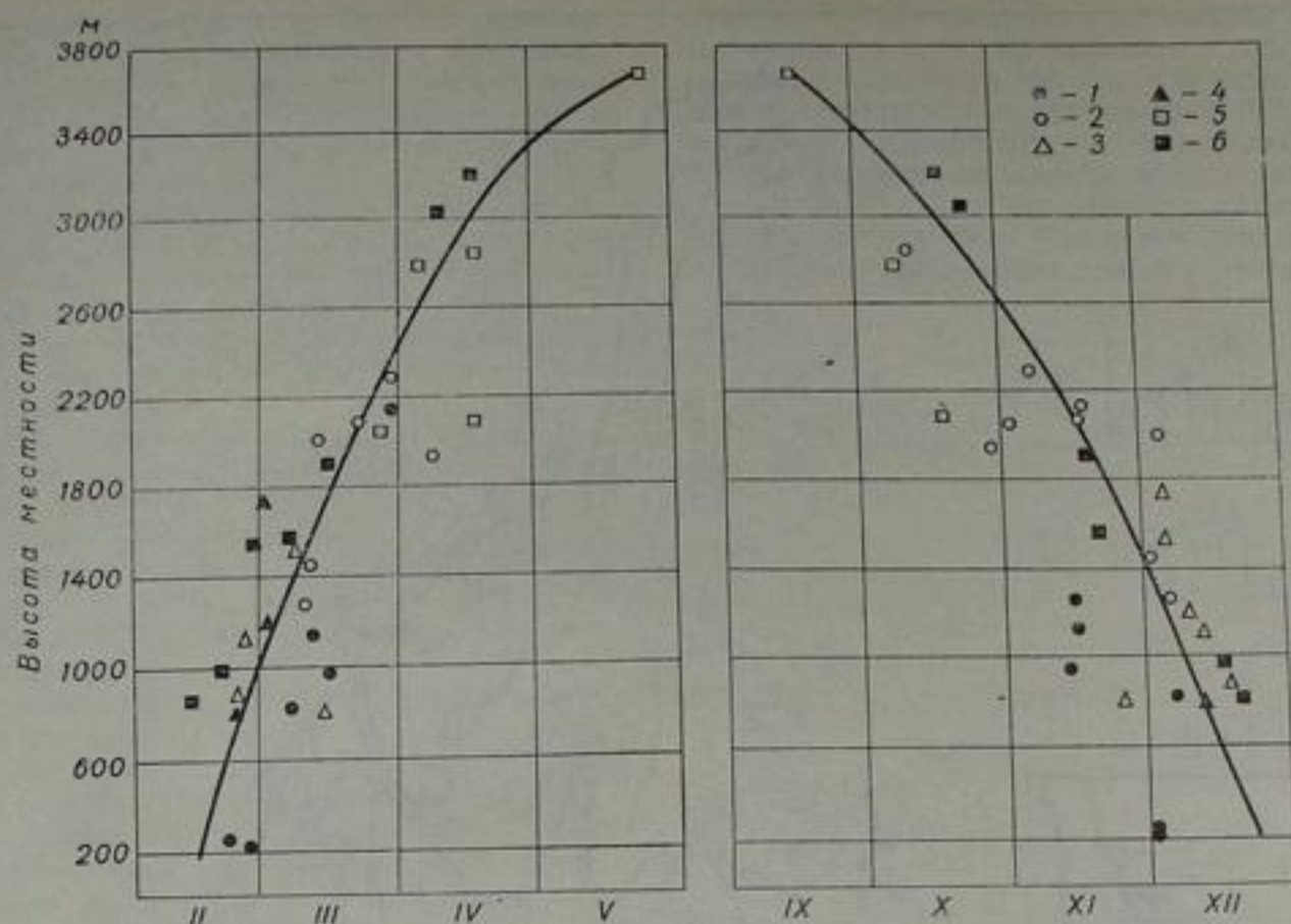
Рис. 5. Зависимость времени перехода средней суточной температуры воздуха через 0^{\circ} от высоты местности.
