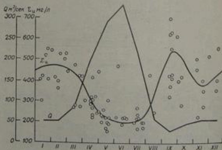
Рис. 169. Внутригодовое изменение минерализации ( \Sigma_a ) и расходов воды (Q) в р. Чирчик у с. Чиназ по многолетним данным.
