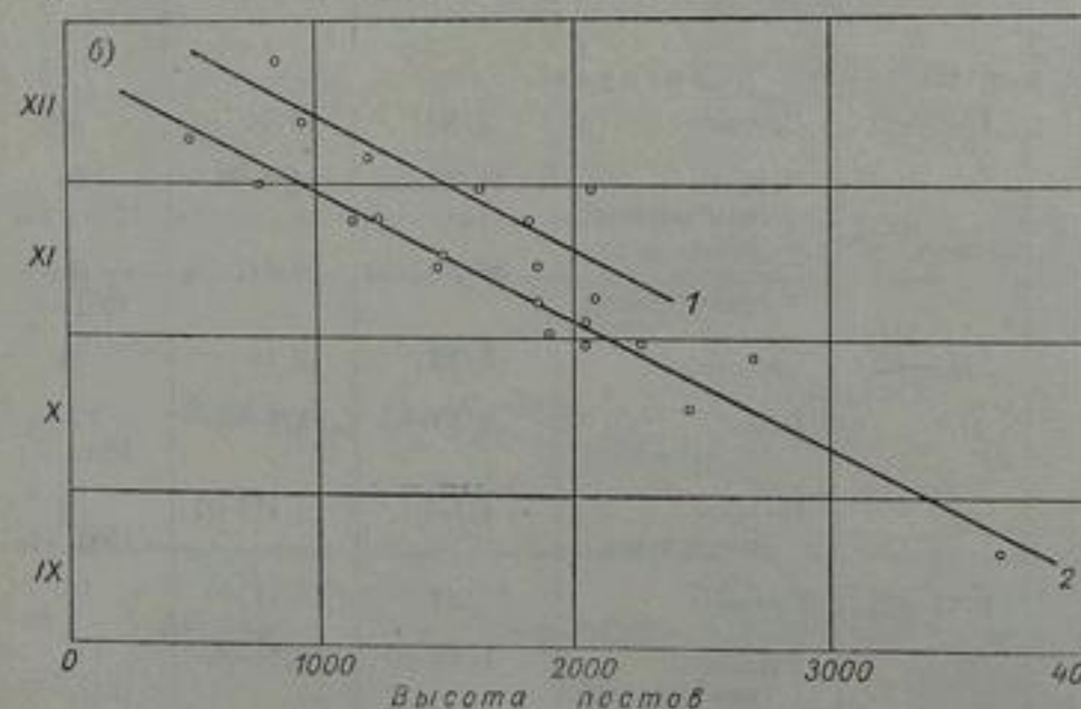
Рис. 119. Зависимость средних дат начала ледовых явлений от высоты постов.
