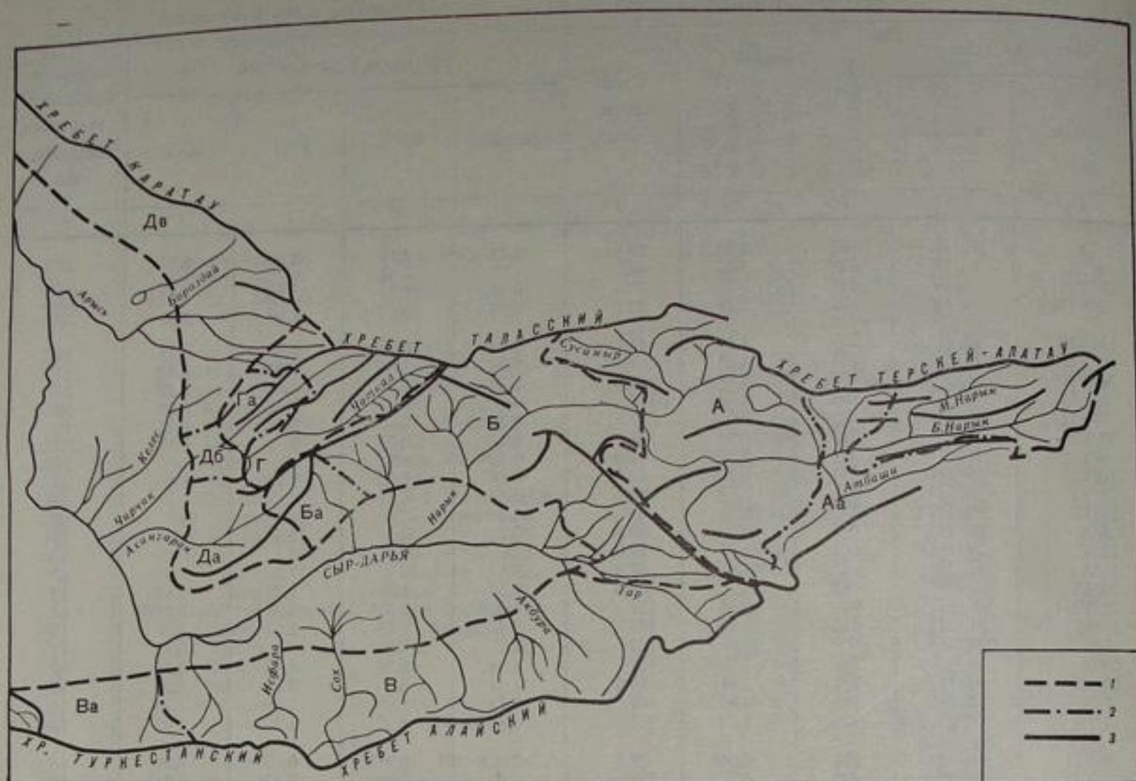
Рис. 97. Схема районирования бассейна р. Сыр-Дарьи по характеру зависимости меженного стока от средней высоты водосбора.
