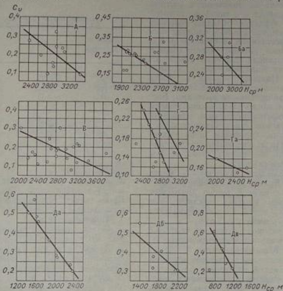
Рис. 109. Зависимость коэффициента вариации минимального стока ( C_{v \min} ) от средней высоты водосборов ( H_{cp} ).
