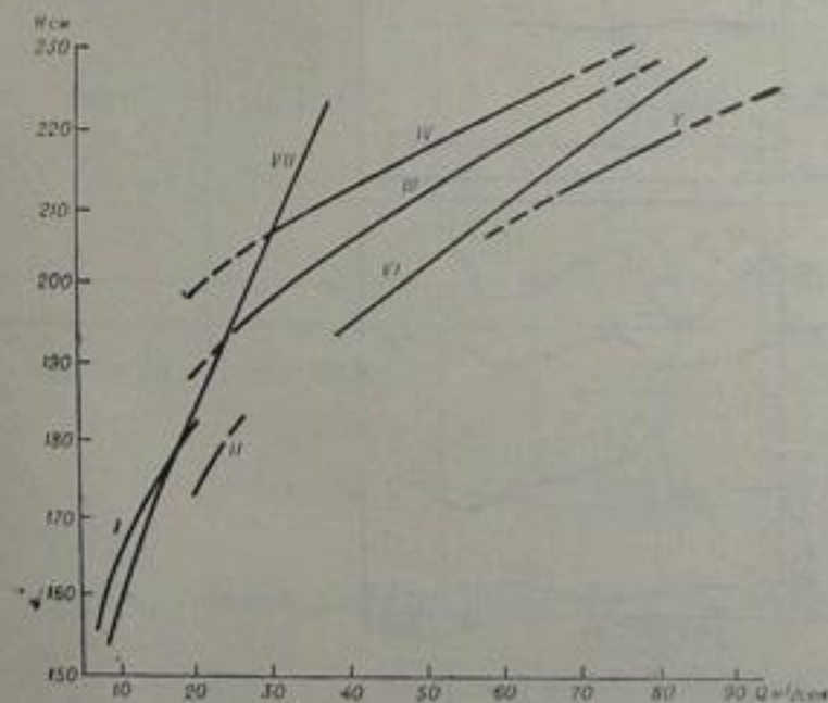
Рис. 30. Кривые расходов р. Куршаб — с. Гульча за 1958 г.
