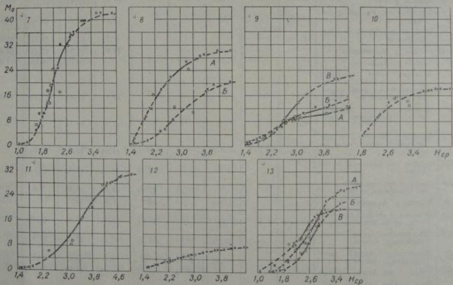
Рис. 49. Районные зависимости модуля стока M_0 от средней высоты водосборов по рекам Ферганской долины. 7-13 — номера районов.
