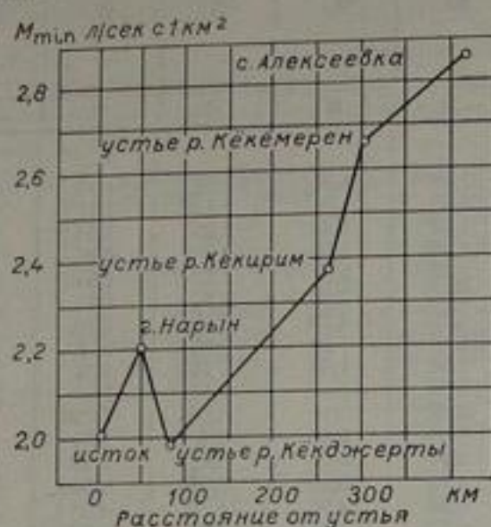
Рис. 105. Изменение модуля месячного минимального стока ( M_{min} ) по длине р. Нарын. За исток принято место слияния рек Большого и Малого Нарына.
