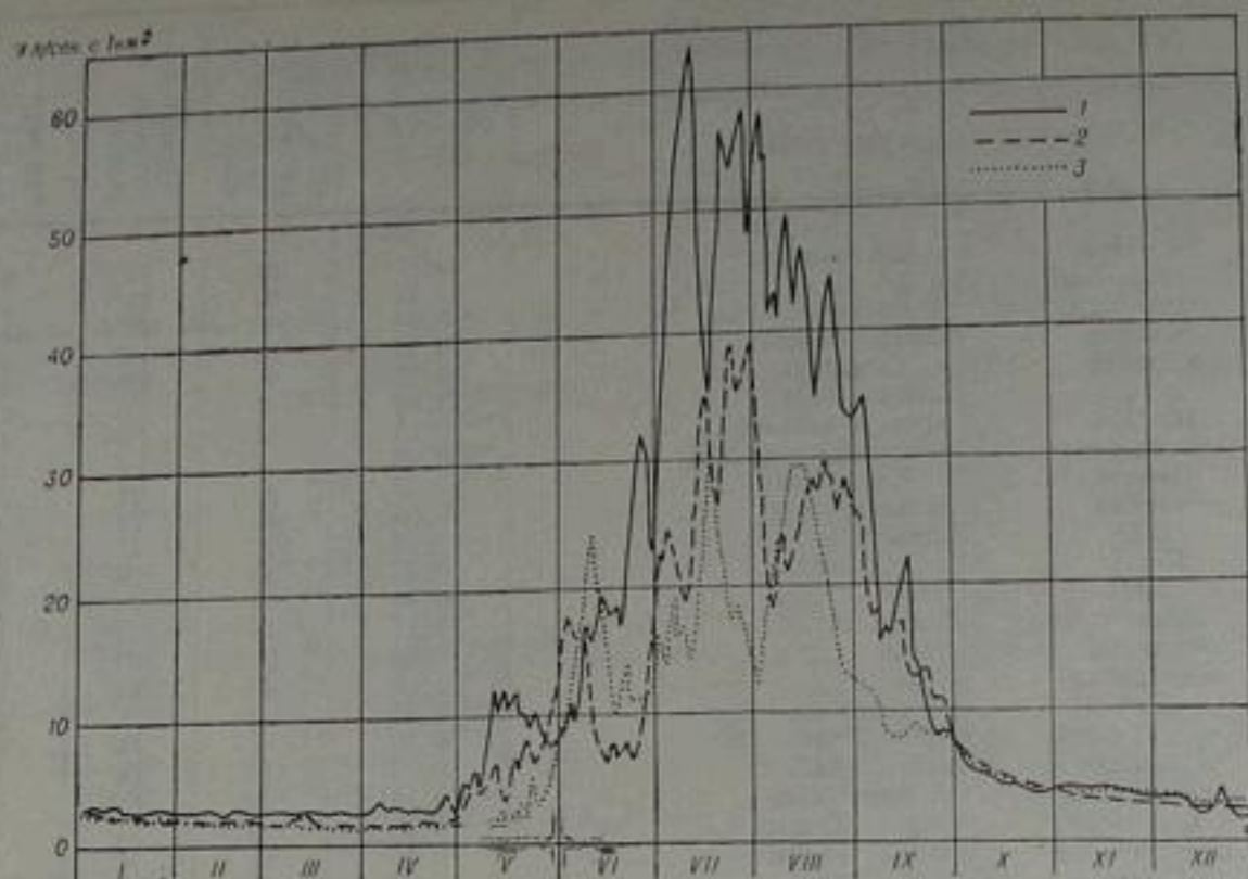
Рис. 15. Гидрографы стока по р. Исфара у кишла. Таш-Курган за характерные по водоносности годы. 1 — 1942 г., 2 — 1961 г., 3 — 1957 г.
