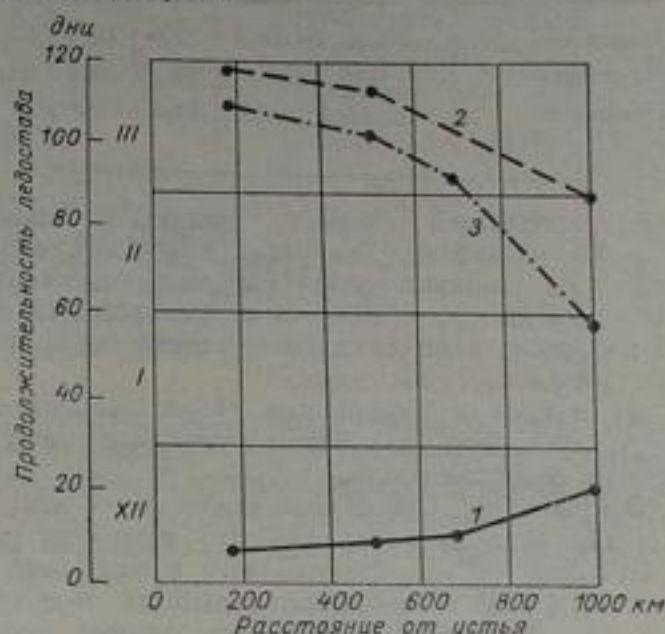
Рис. 124. Изменение дат начала (1), конца (2) и продолжительности (3) ледостава по длине р. Сыр-Дарьи.
