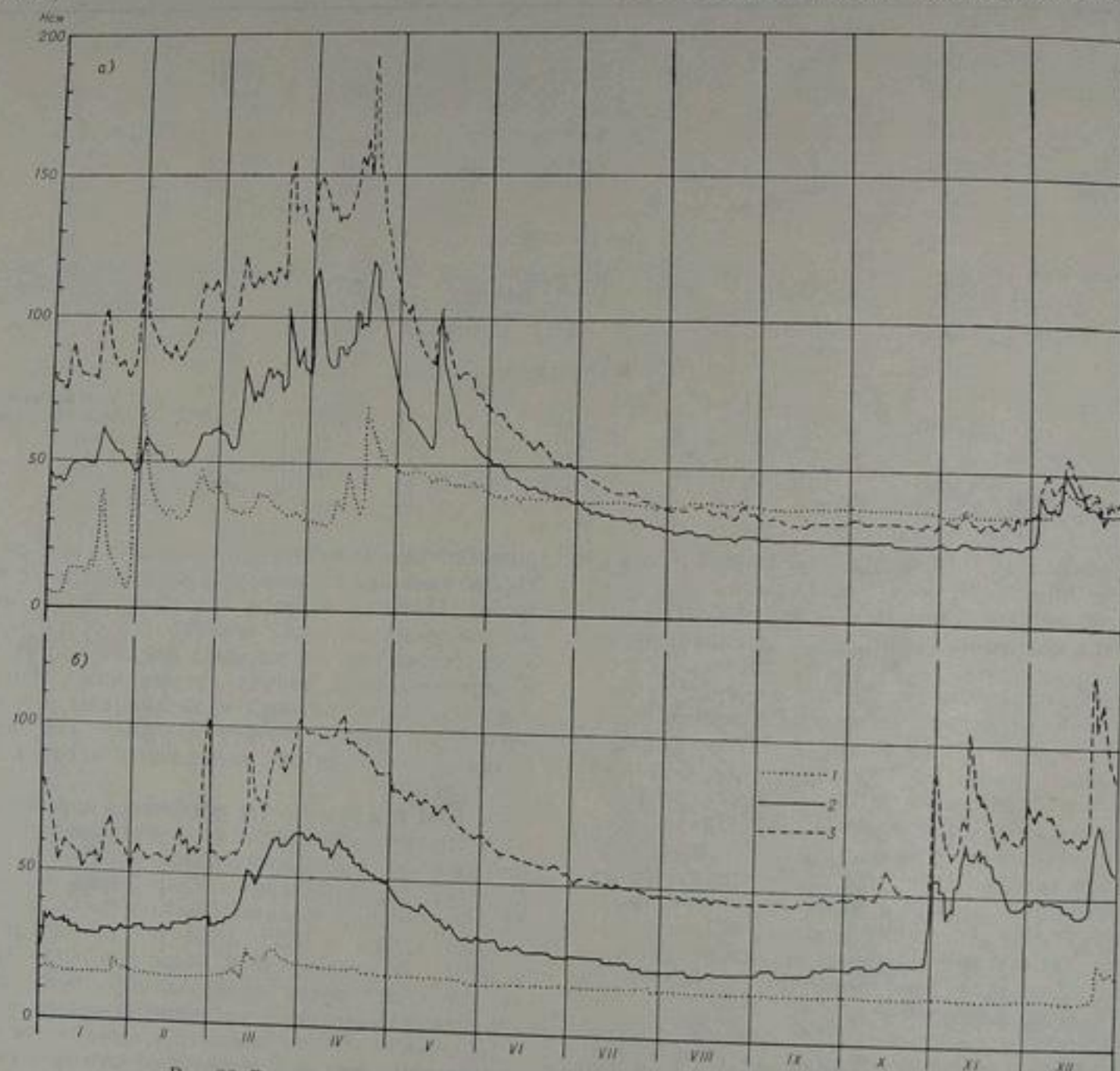
Рис. 26. Годовой ход уровня на низкогорных реках снего-дождевого питания. а — многоводный 1958 г., б — маловодный 1951 г.; 1 — р. Ашилган — клх Майдантал, 2 — р. Кокбулак — с. Пистелли, 3 — р. Боралдай — клх им. Карла Маркса.
