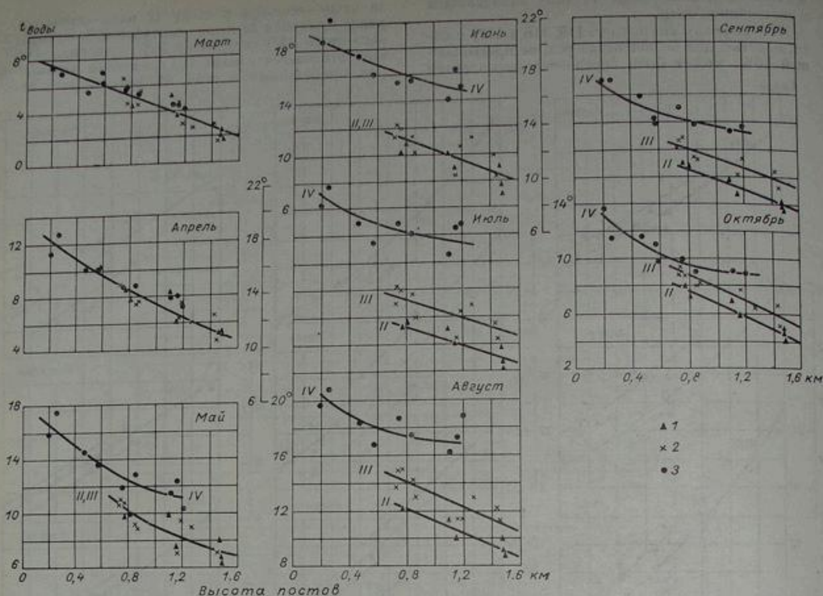
Рис. 117. Графики зависимости многолетней среднемесячной температуры воды от высоты постов в реках бассейнов Чирчика и Арыси.
