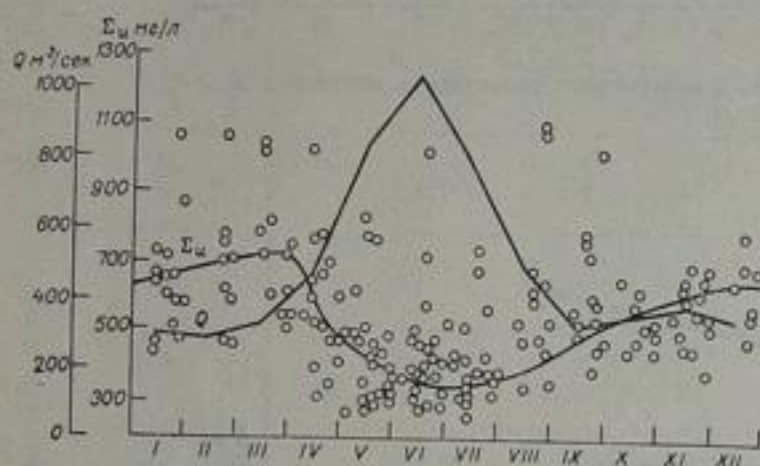
Рис. 174. Внутригодовое изменение минерализации ( \Sigma_{и} ) и расходов воды ( Q ) в р. Сыр-Дарье у кишла. Каль.
