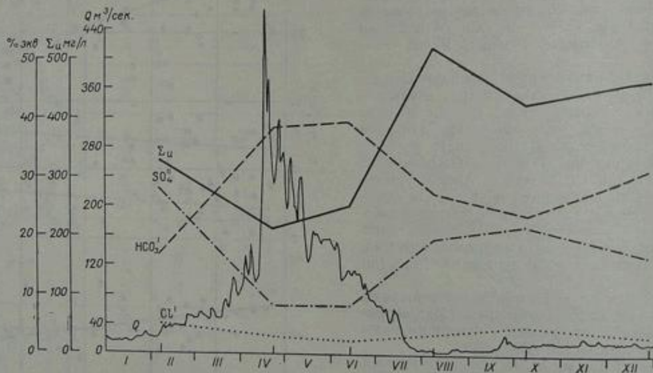
Рис. 164. Внутригодовое изменение минерализации ( \Sigma_{и} ) и содержания главных анионов в воде р. Ахангаран у с. Самарское за 1952 г.
