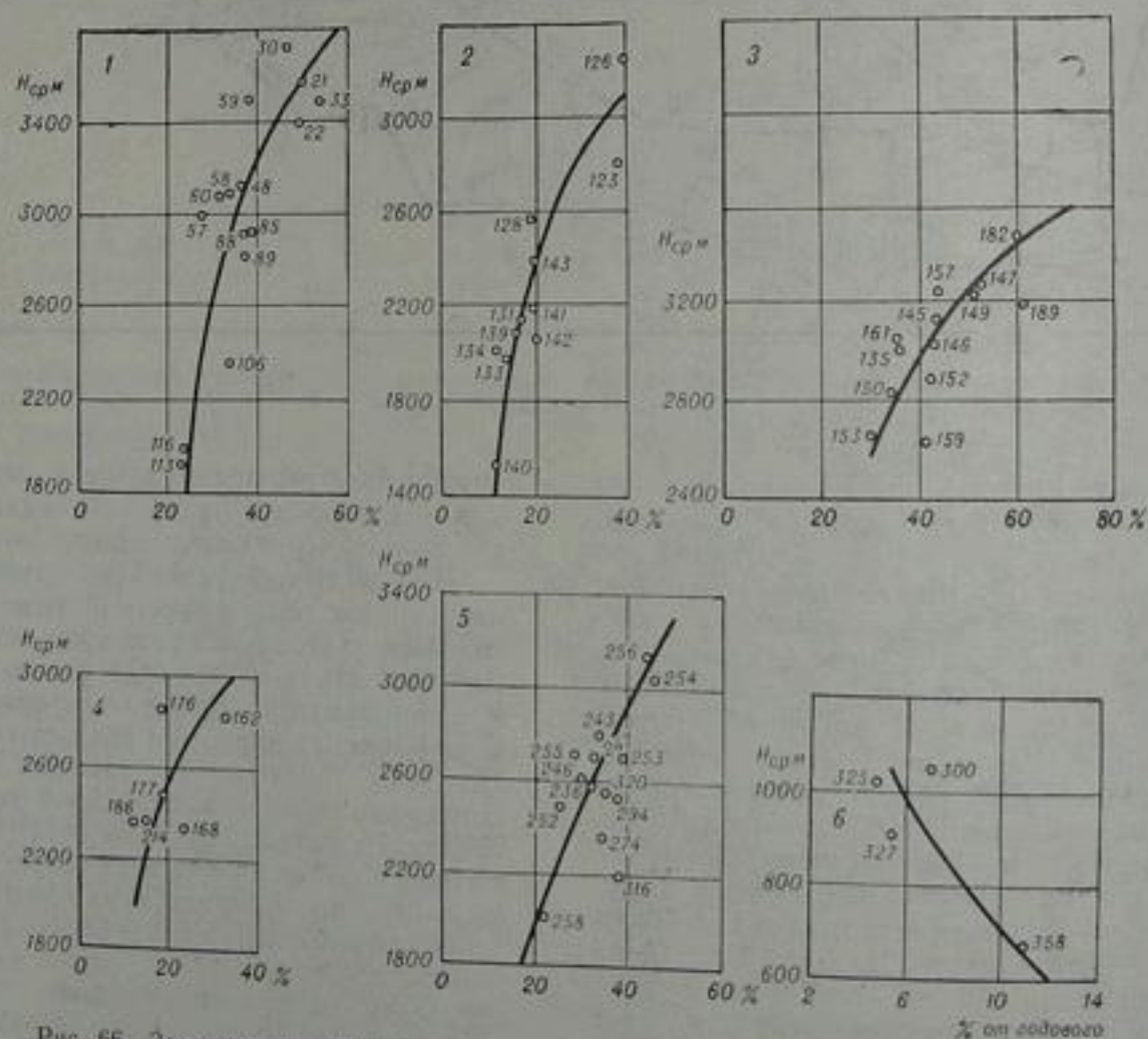
Рис. 66. Зависимость летнего стока рек бассейна Сыр-Дарьи (в % от годового) от средневзвешенной высоты водосборов H_{cp} . Усл. обозначения см. рис. 65.
