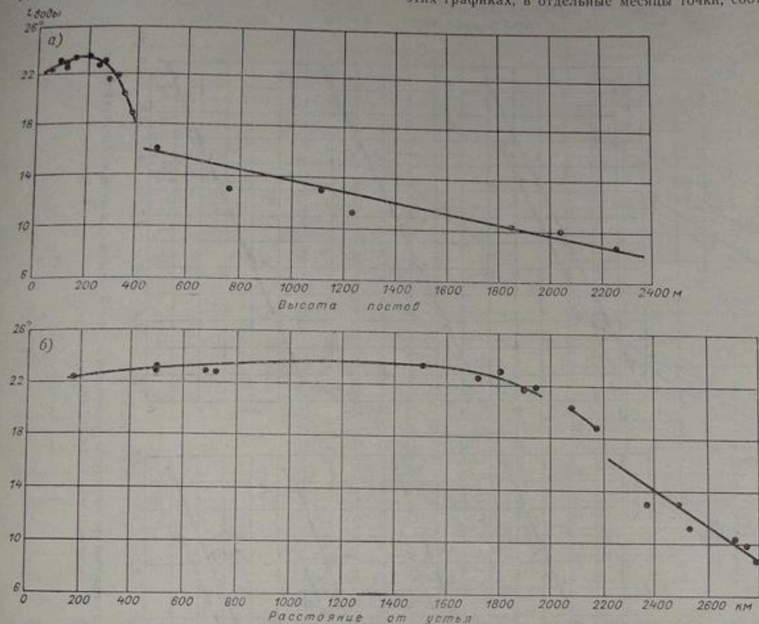
Рис. 114. Изменение средней многолетней температуры воды в р. Сыр-Дарье (с. Нарыном) за июнь в зависимости от высоты постов над уровнем моря (а) и расстояния от устья (б).
