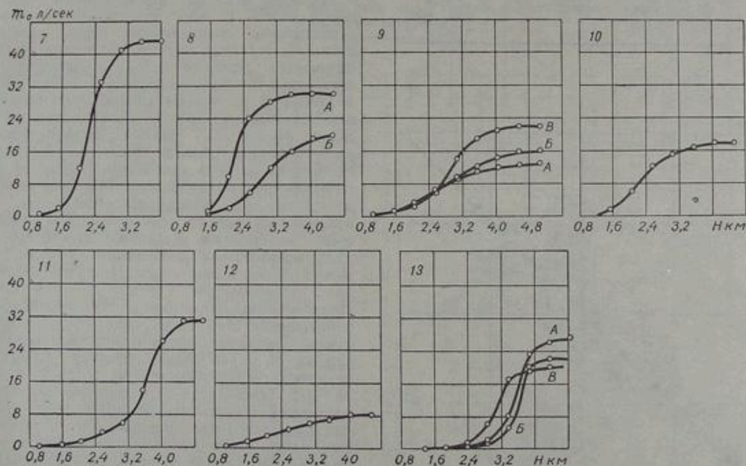
Рис. 45. Районные зависимости зональных модулей нормы годового стока от высоты водосборов m_0 = f(H) для рек Ферганской долины. 7-13 — районы.
