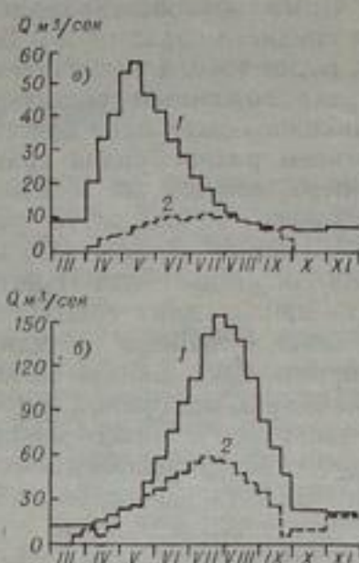
Рис. 62. Графики внутригодового распределения стока (1) и водопотребления на орошение (2) по типичным рекам бассейна Сыр-Дарьи.
