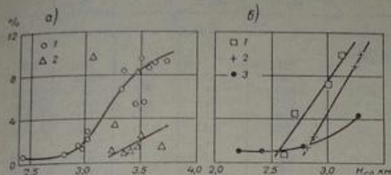
Рис. 148. Зависимость коэффициента (процента) оледенения речных водосборов от их средней высоты ( H_{cp} ).
