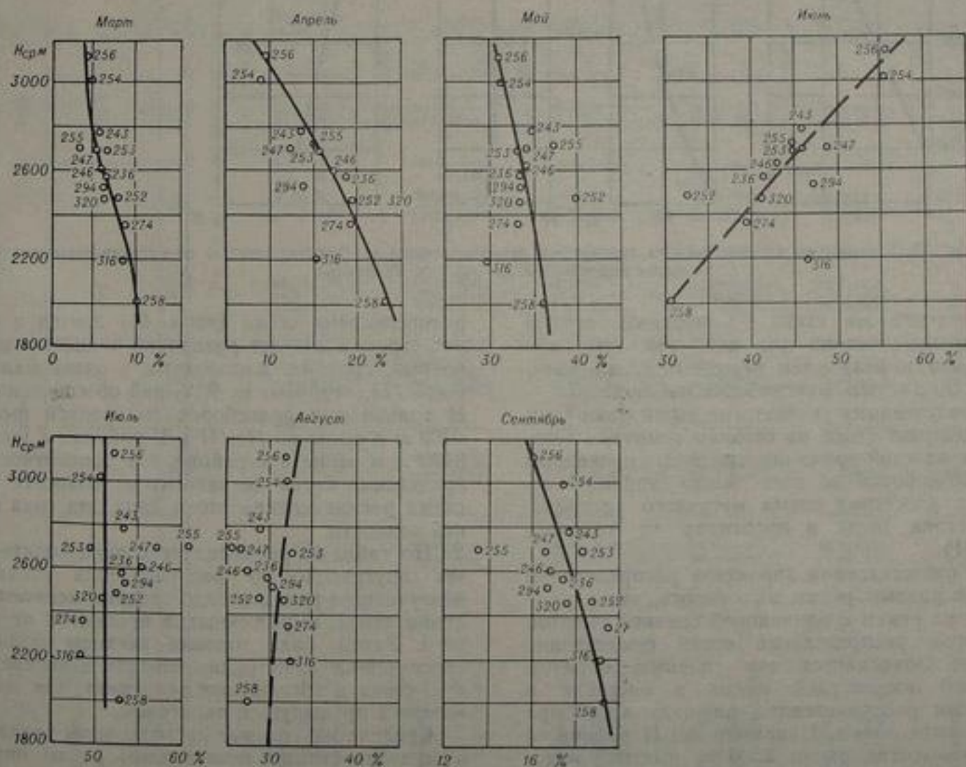
Рис. 72. Зависимость месячного стока весеннего и летнего сезонов (в % от сезонного) от средневзвешенной высоты водосбора H_{cp} для рек V района.
