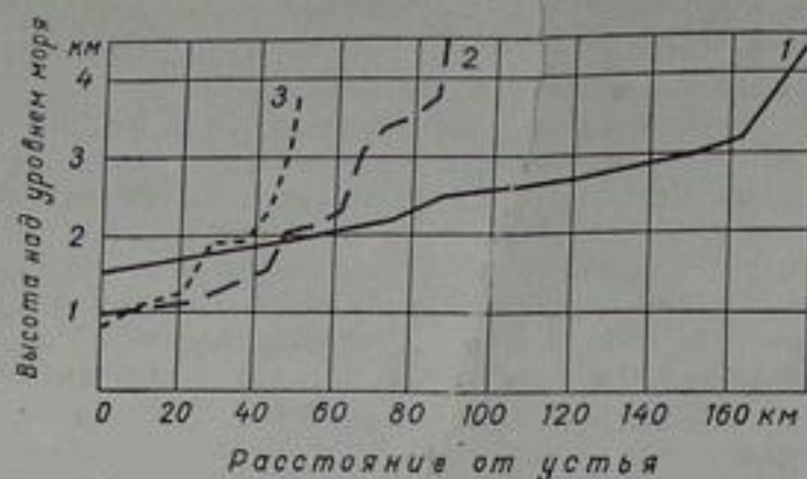
Рис. 13. Продольные профили русел рек с характерным ступенчатым строением.
