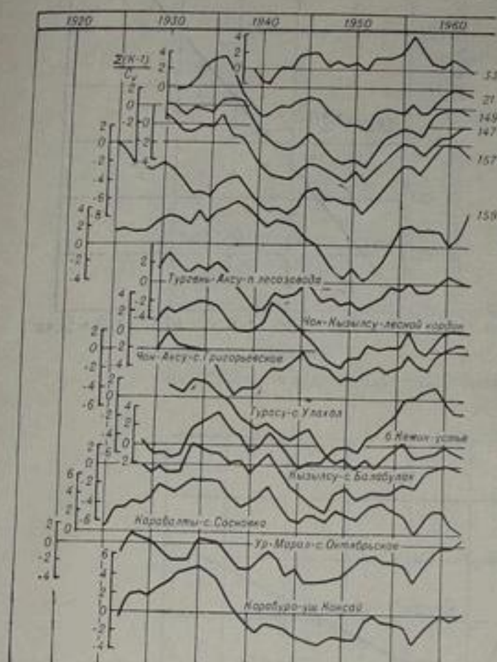
Рис. 37. Разностные интегральные кривые колебаний годового стока воды по рекам II группы с показателем типа питания \delta , равным от 1,2 до 2.
