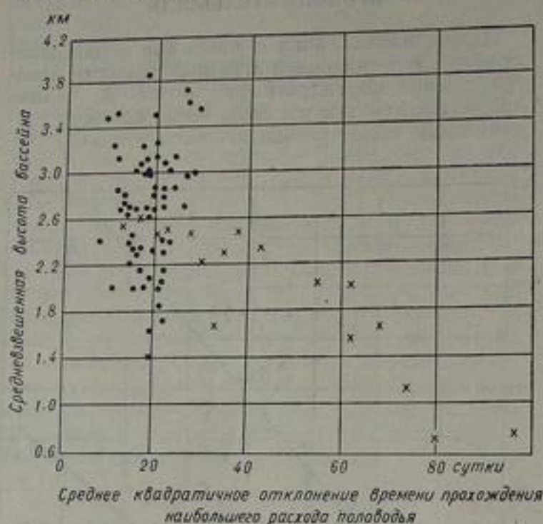
Рис. 77. Зависимость изменчивости времени прохождения наибольшего расхода половодья от высоты водосборов.
