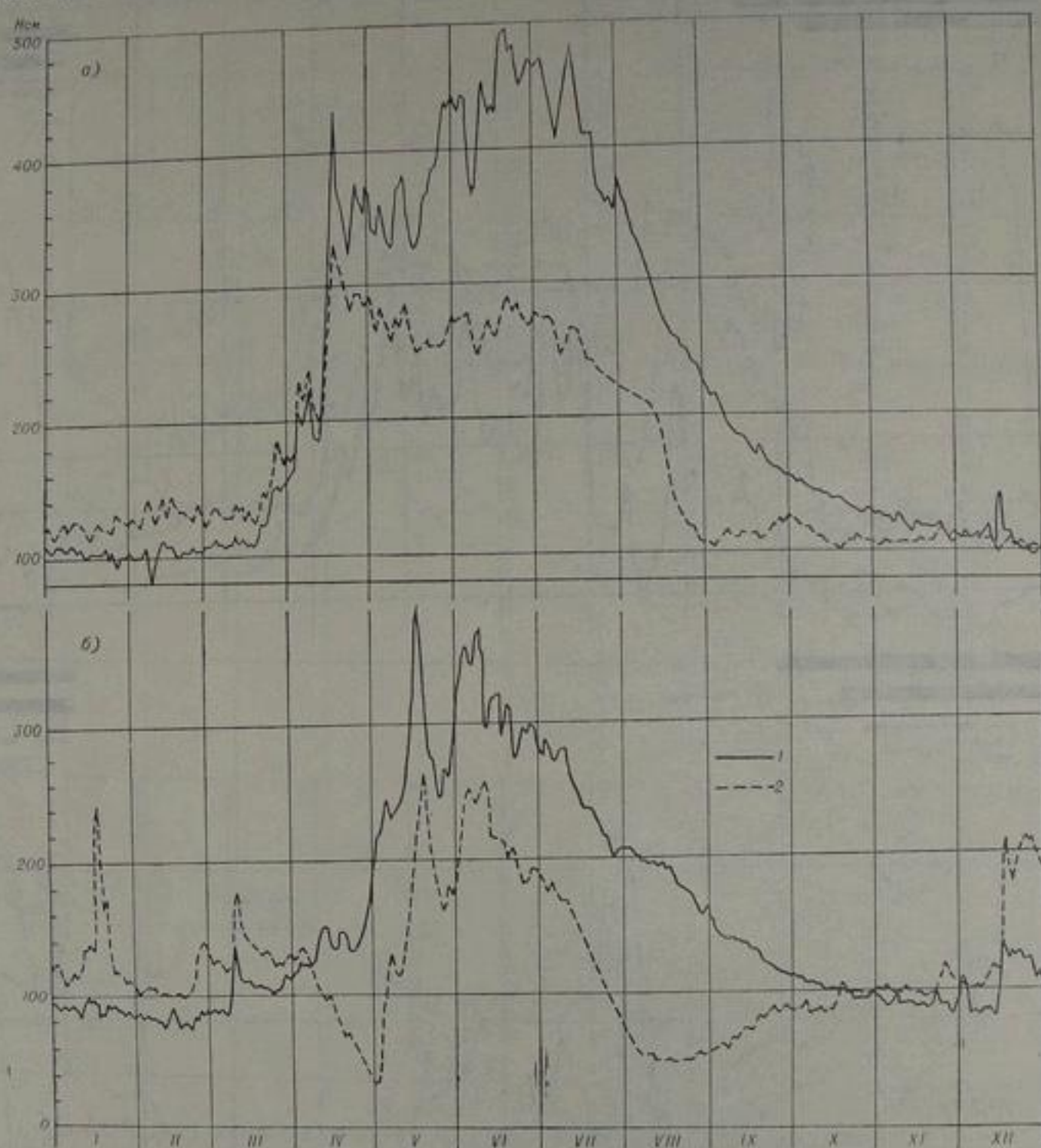
Рис. 28. Годовой ход уровня воды в р. Чирчик в створе на выходе из гор у с. Ходжикент и в устье у с. Чиназ.
