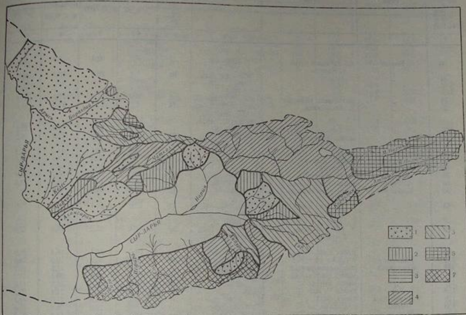
Рис. 141. Схематическая карта распределения стока взвешенных наносов за июль—сентябрь (в % от годового). 1 — 0—5%, 2 — 5—10%, 3 — 10—20%, 4 — 20—30%, 5 — 30—50%, 6 — 50—70%, 7 — 70—85%.
