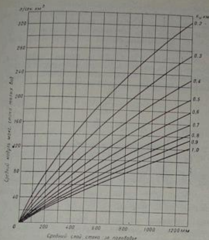
Рис. 94. Номограмма для вычисления модулей максимального стока талых вод. \bar{H} мм — среднее квадратичное отклонение высот водосбора.
