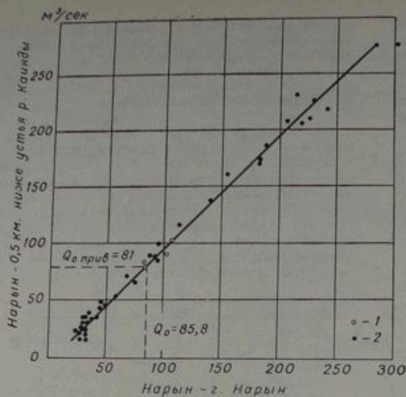
Рис. 39. Графики связи среднегодовых (1) и среднемесячных (2) расходов воды р. Нарын.
