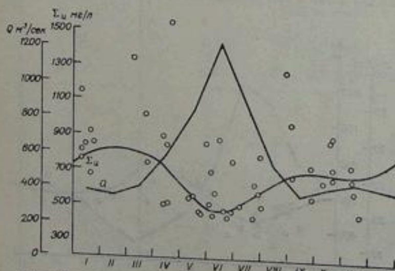
Рис. 175. Внутригодовое изменение минерализации ( \Sigma_{и} ) и расходов воды ( Q ) в р. Сыр-Дарье у кишла. Акджар.
