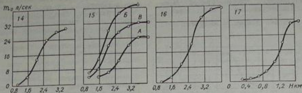
Рис. 46. Районные зависимости зональных модулей нормы годового стока от высоты водосборов m_0 = f(H) для бассейнов рек Ахангаран, Чирчик, Арысь и рек юго-западных склонов хр. Каратау.
