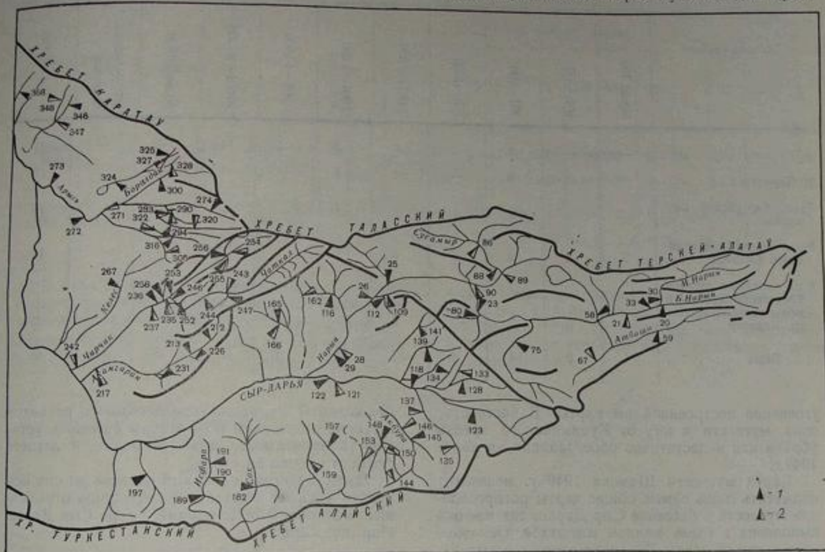
Рис. 131. Схема расположения пунктов наблюдений за стоком взвешенных наносов в бассейне Сыр-Дарьи. 1 — посты, действующие на 1/1 1963 г., 2 — посты закрытые.
