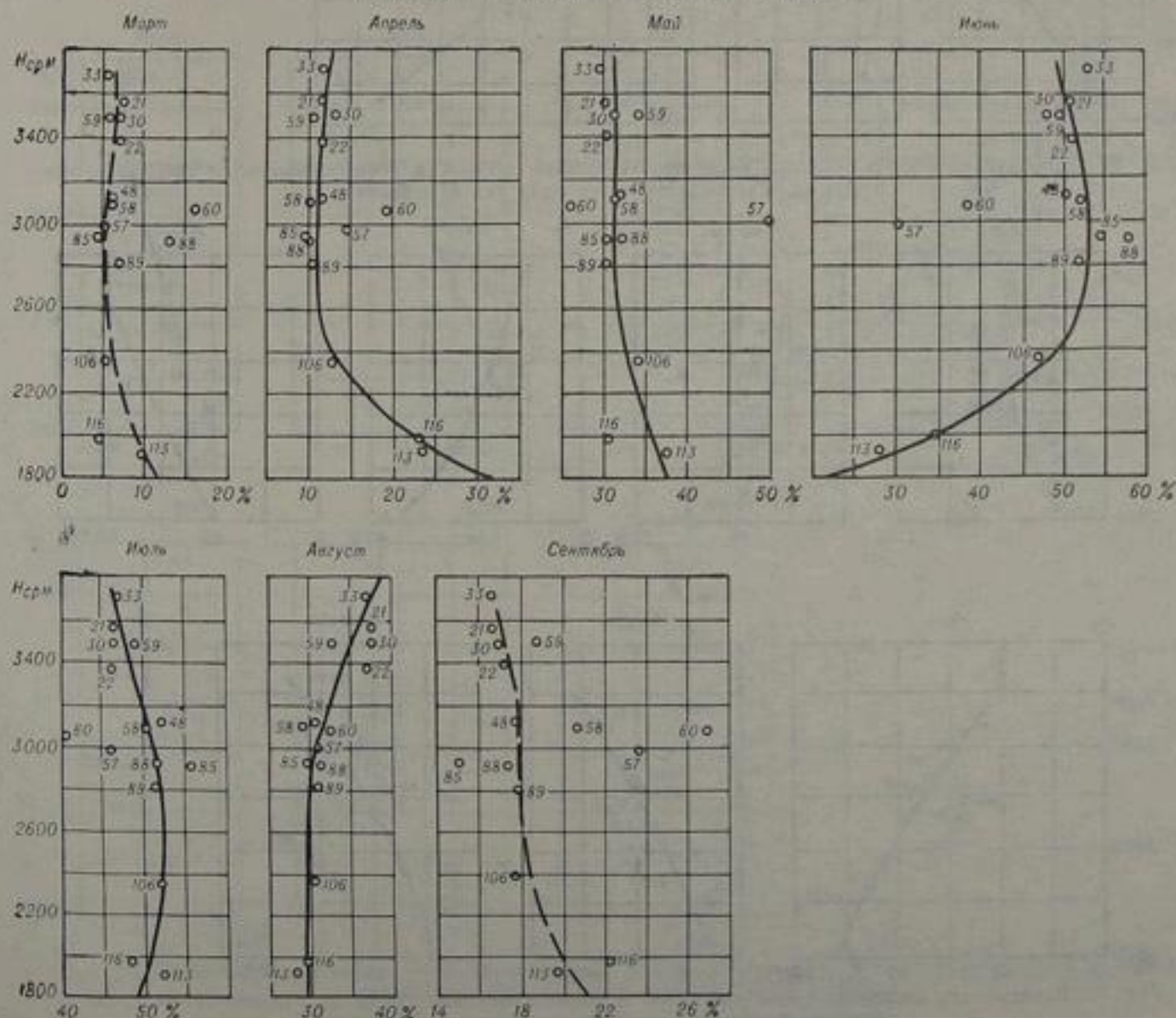
Рис. 68. Зависимость месячного стока весеннего и летнего сезонов (в % от годового) от средневзвешенной высоты водосбора H_{\text{ср}} для рек I района.
