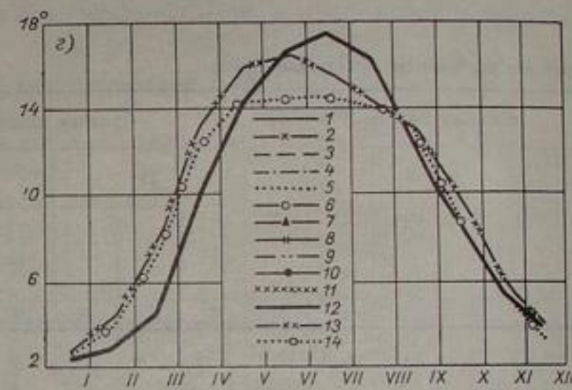
Рис. 110. Годовой ход средней многолетней температуры воды.
