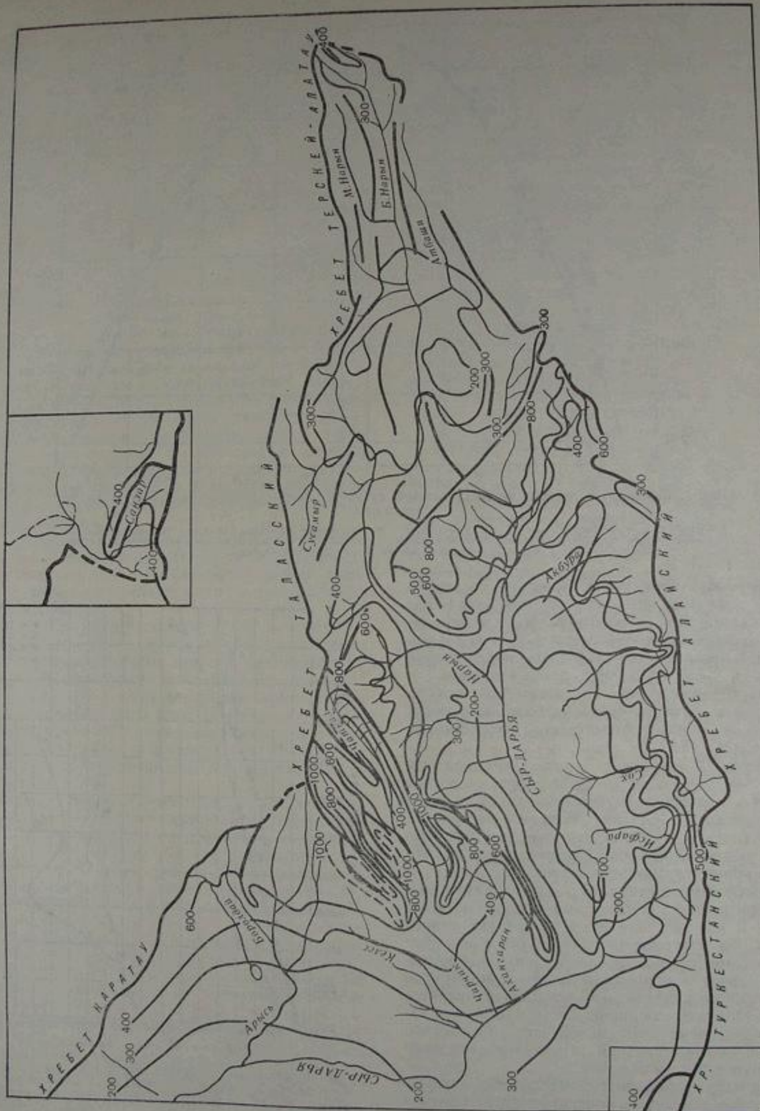
Рис. 7. Схематическая карта годовых сумм осадков в горной части бассейна Сыр-Дарьи.
