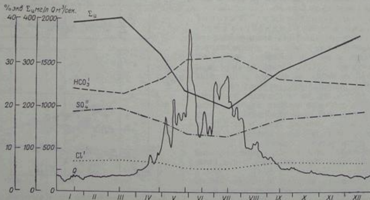
Рис. 158. Внутригодовое изменение минерализации и содержания главных анионов в воде р. Нарына у кишла. Учкурган за 1956 г.
