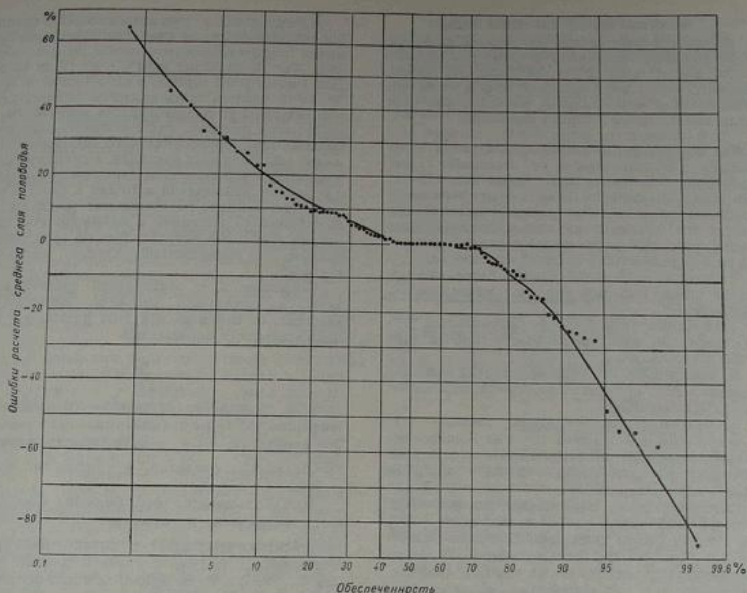
Рис. 84. Обеспеченность относительных ошибок расчета среднего слоя половодья.
