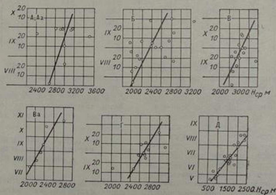
Рис. 98. Зависимость средней даты начала межеи от средней высоты водосборов ( H_{cp} ).
