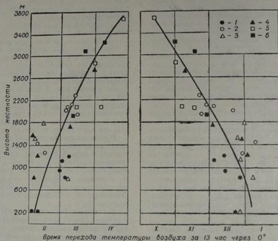
Рис. 9. Зависимость времени перехода температуры воздуха в 13 час. через 0° от высоты местности.
