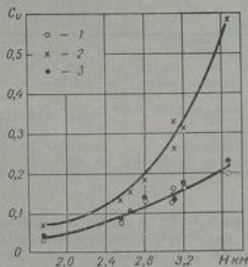
Рис. 56. Изменение коэффициентов вариации сумм положительных температур воздуха ( C_v ) с высотой местности ( H ) в экспериментальном бассейне р. Чон-Кызылсу.
