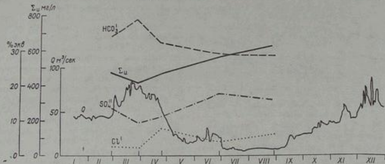
Рис. 171. Внутригодовое изменение минерализации воды ( \Sigma_{и} мг/л) и содержания главных анионов в воде р. Арысь у ж.-д. ст. Арысь за 1957 г.
