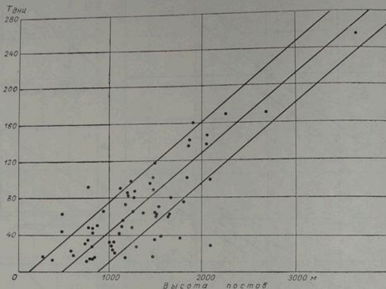
Рис. 121. Зависимость продолжительности ледовых явлений ( T ) от высоты постов.
