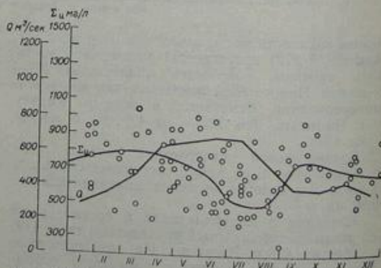
Рис. 176. Внутригодовое изменение минерализации ( \Sigma_{и} ) и расходов воды ( Q ) в р. Сыр-Дарье у г. Казалинска.
