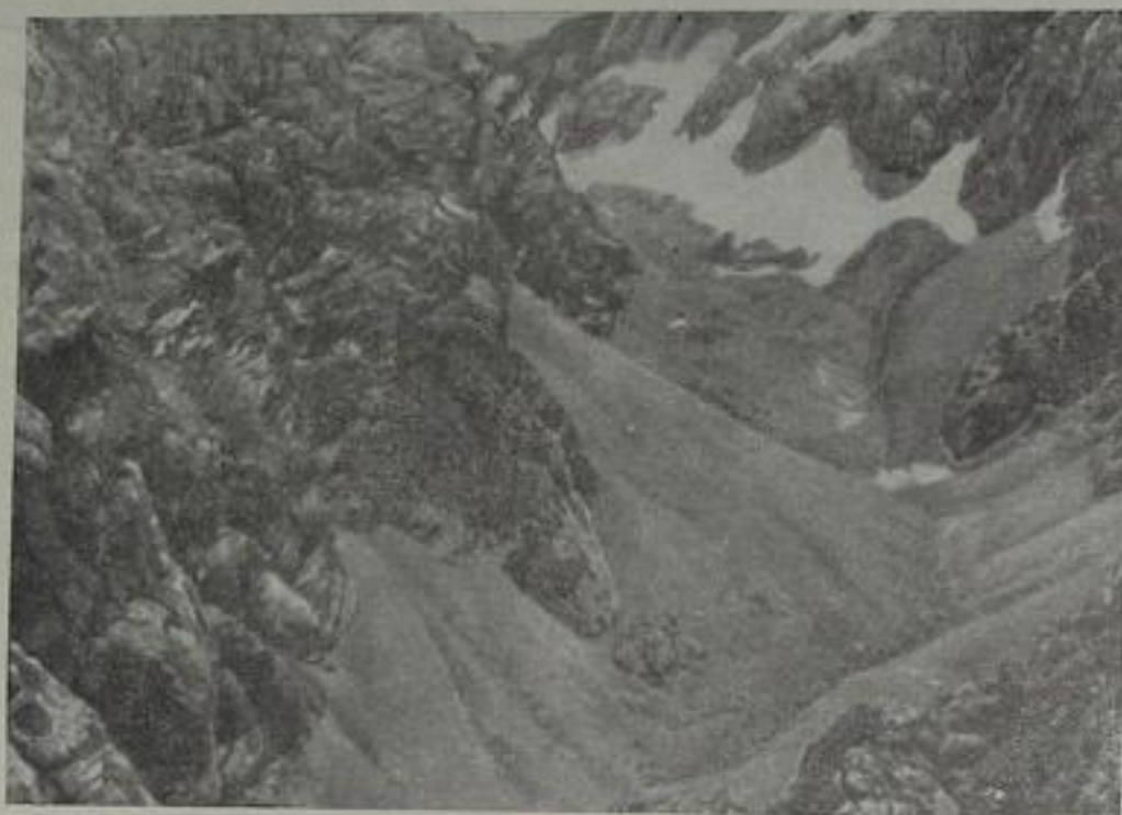
Рис. 12. Русло левого притока р. Мустыр в бассейне р. Майлису, засыпанное моренами и щебнистыми осыпями со склонов.
