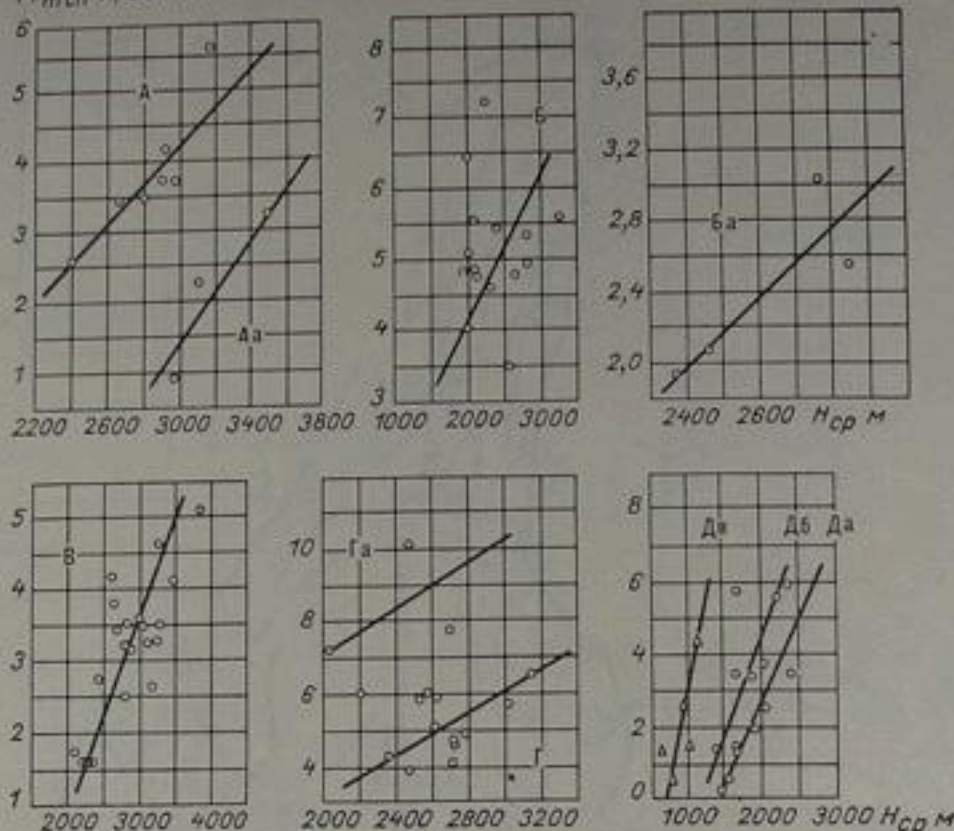
Рис. 107. Зависимость месячного модуля минимального стока M_{min} от средней высоты водосбора ( H_{cp} ).
