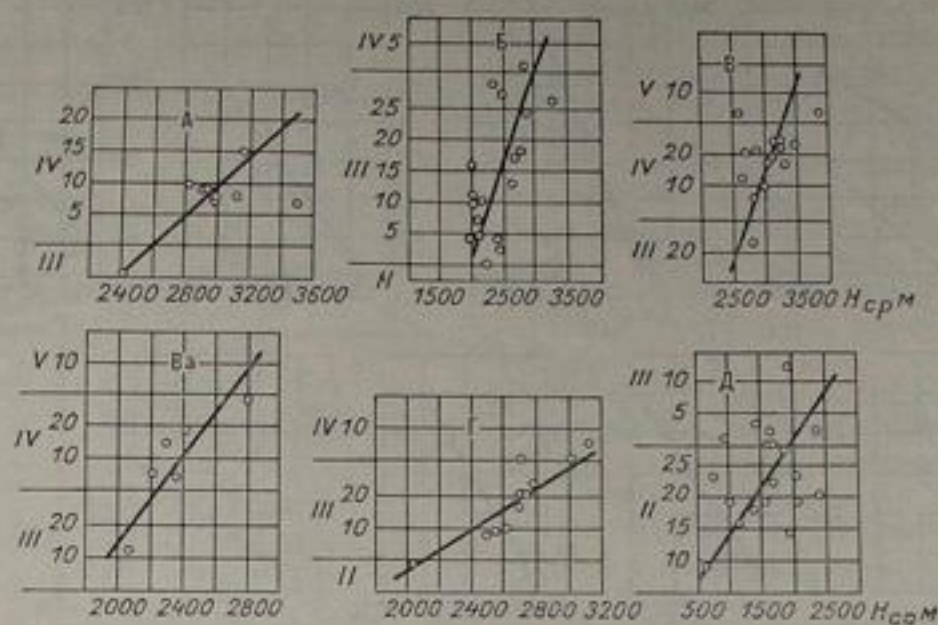
Рис. 99. Зависимость средней даты окончания межени от средней высоты водосборов ( H_{ср} ).
