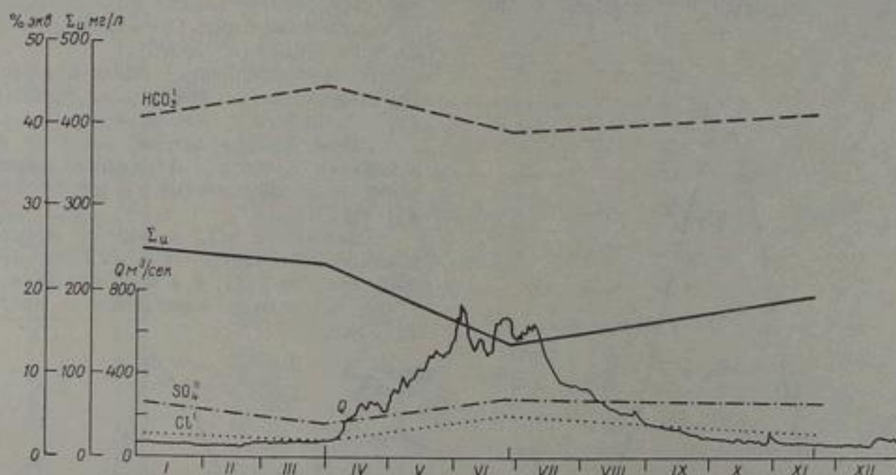
Рис. 166. Внутригодовое изменение минерализации ( \Sigma_{и} ) и содержания главных анионов в воде р. Чирчик у с. Ходжикент за 1943 г.
