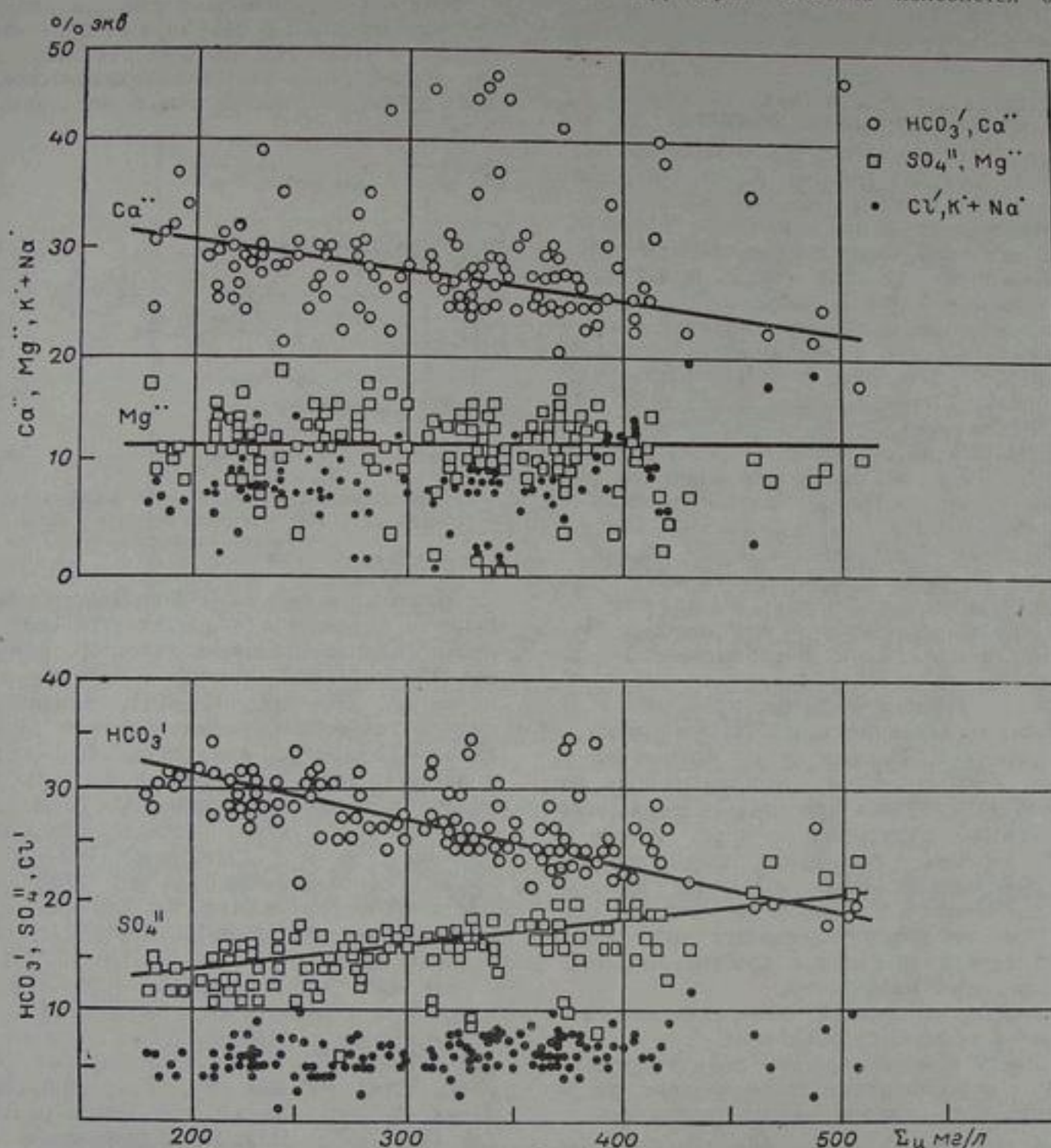
Рис. 155. Характер связи между величиной минерализации воды ( \Sigma_{\text{с}} мг/л) и содержанием главных анионов и катионов (% экв) по данным за 1938—1943, 1950—1962 гг. для р. Нарына у поста кишла. Уч-курган.
