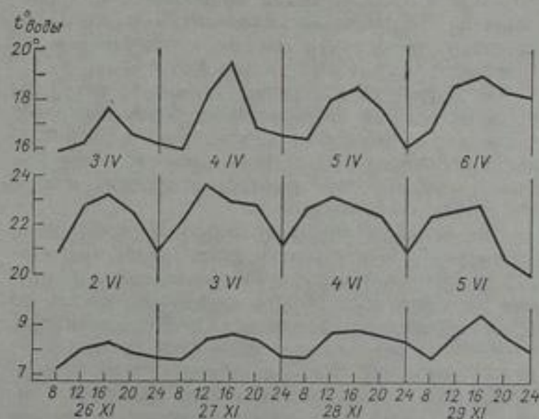
Рис. 113. Суточный ход температуры воды в р. Сыр-Дарье у г. Бекабад в 1947 г.
