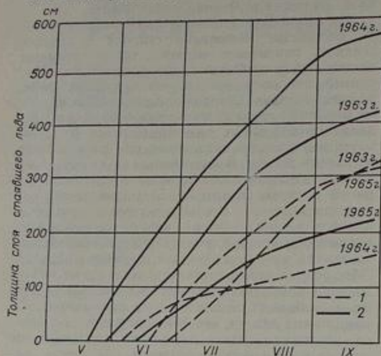
Рис. 149. Интегральные кривые стаивания поверхности ледников. 1 — ледник Давыдова, 2 — ледник Кенгтур.
