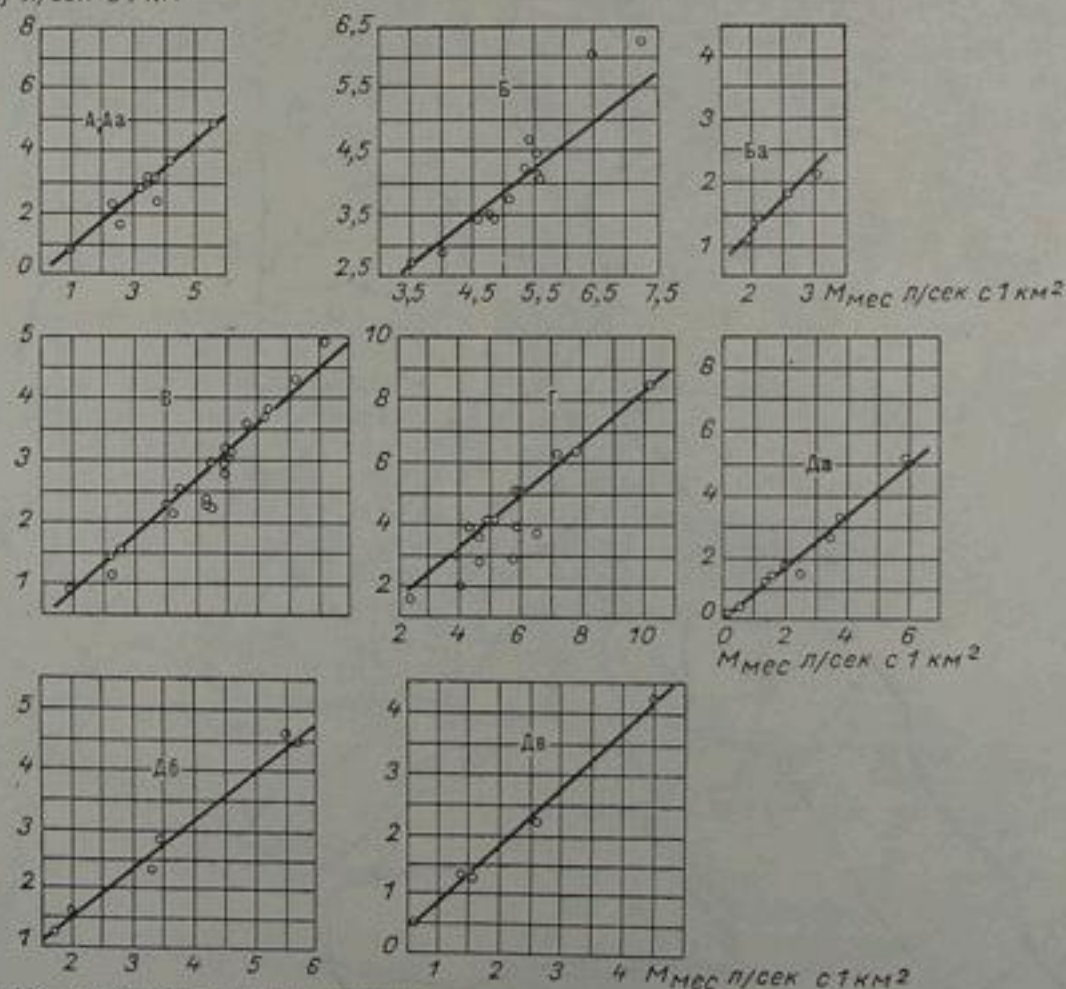
Рис. 108. Зависимость модуля суточного минимального стока ( M_{сут} ) от модуля месячного минимального стока ( M_{мес} ).
