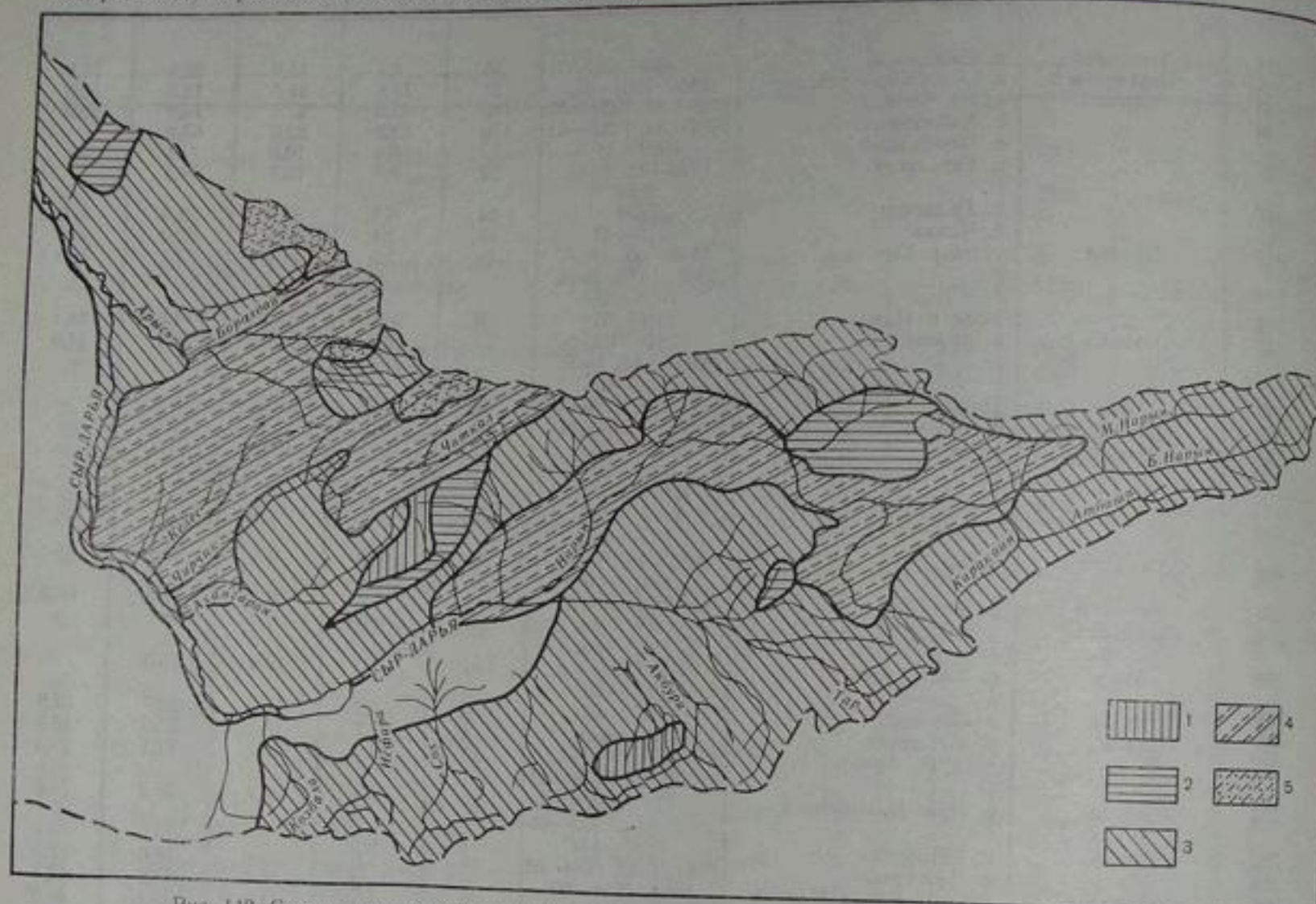
Рис. 142. Схематическая карта крупности взвешенных наносов в реках бассейна Сыр-Дарьи. Содержание фракции <0,05 мм в % от общего количества наносов: 1 — <25 , 2 — 25—50, 3 — 50—75, 4 — 75—90, 5 — >90 .
