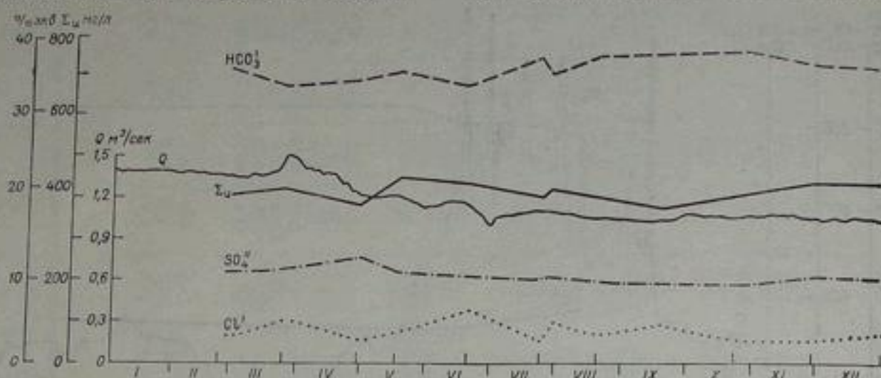
Рис. 173. Внутригодовое изменение минерализации ( \Sigma_{и} ) и содержания главных анионов в воде р. Карасу (Кочкарата) у г. Чимкента за 1957 г.
