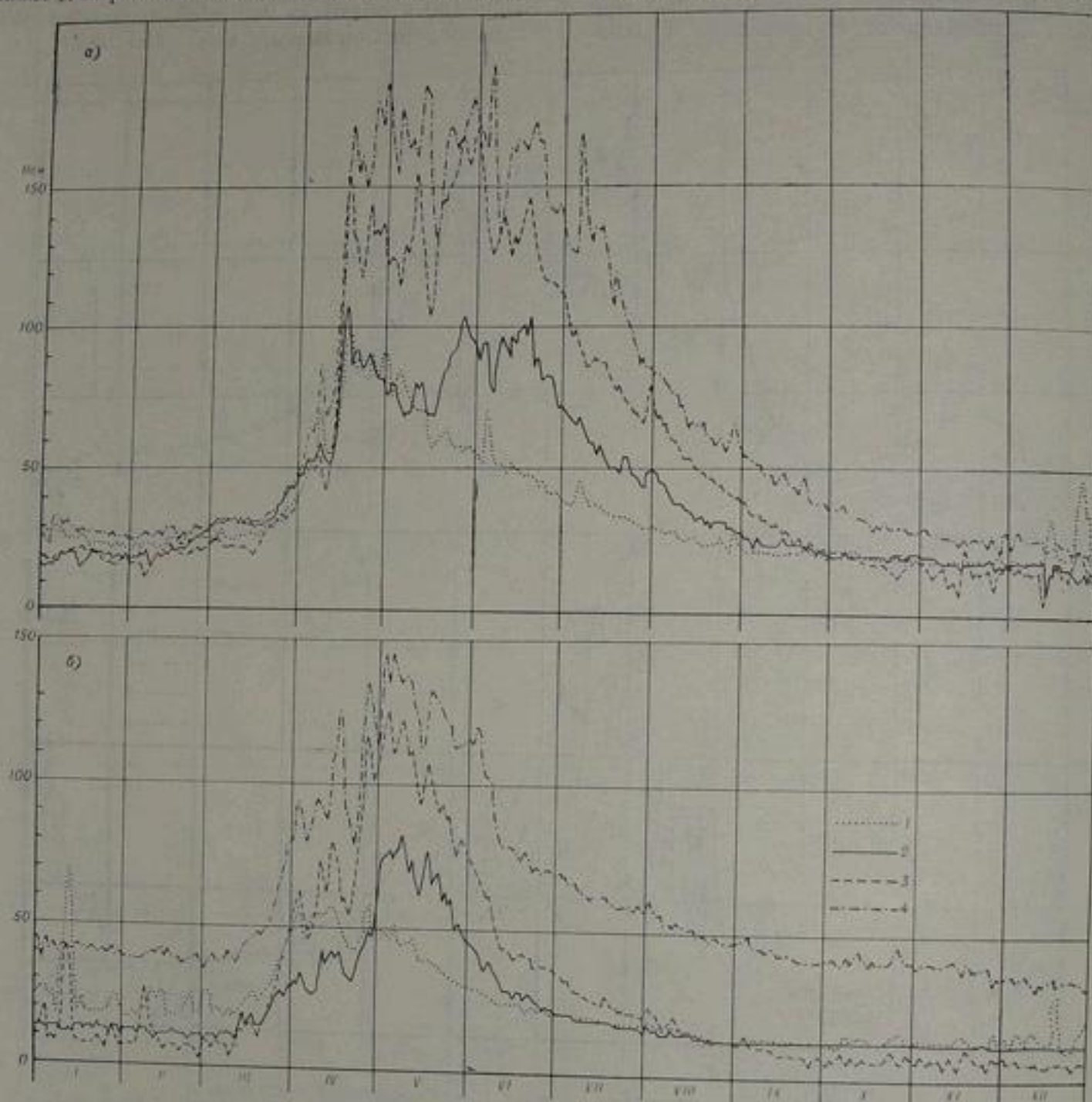
Рис. 25. Годовой ход уровня на реках снегового питания. а — многоводный 1952 г., б — маловодный 1961 г.; 1 — р. Донгузтау — кишл. Донгуз-Тау, 2 — р. Чадак — устье р. Джулайсай, 3 — р. Ахангаран — устье р. Якаарча, 4 — р. Яссы — с. Саданалик.
