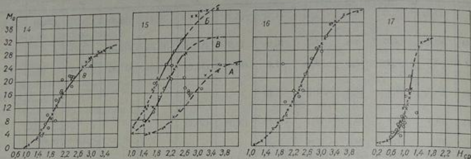
Рис. 50. Районные зависимости модуля стока M_0 от средней высоты водосбора по рекам бассейна Ахангаран, Чирчик, Арысь и рекам юго-западных склонов хр. Каратау. 14—17 — номера районов.
