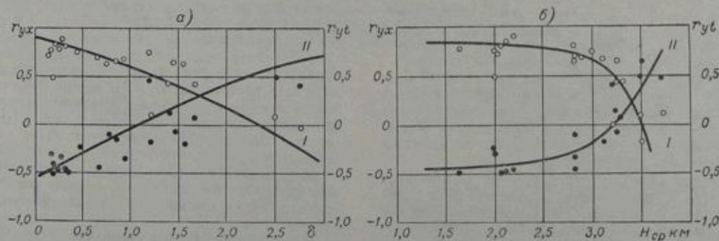
Рис. 58. Изменение тесноты связи годового стока с метеорологическими факторами в зависимости от условного показателя типа питания реки \delta (а) и от средневзвешенной высоты H_{cp} (б).
