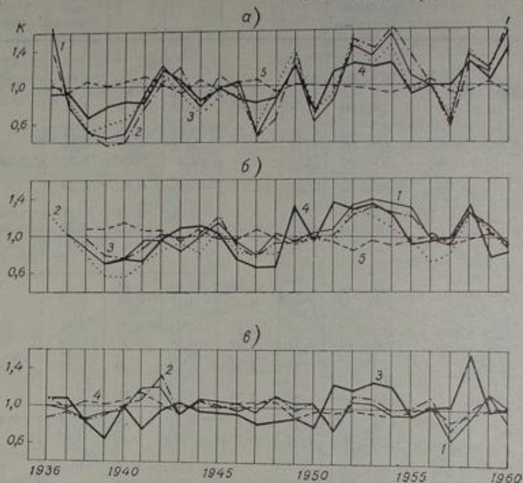
Рис. 59. Хронологические графики изменения модульных коэффициентов годового стока рек разного типа питания ( K ), годовых сумм осадков и положительных температур воздуха.
