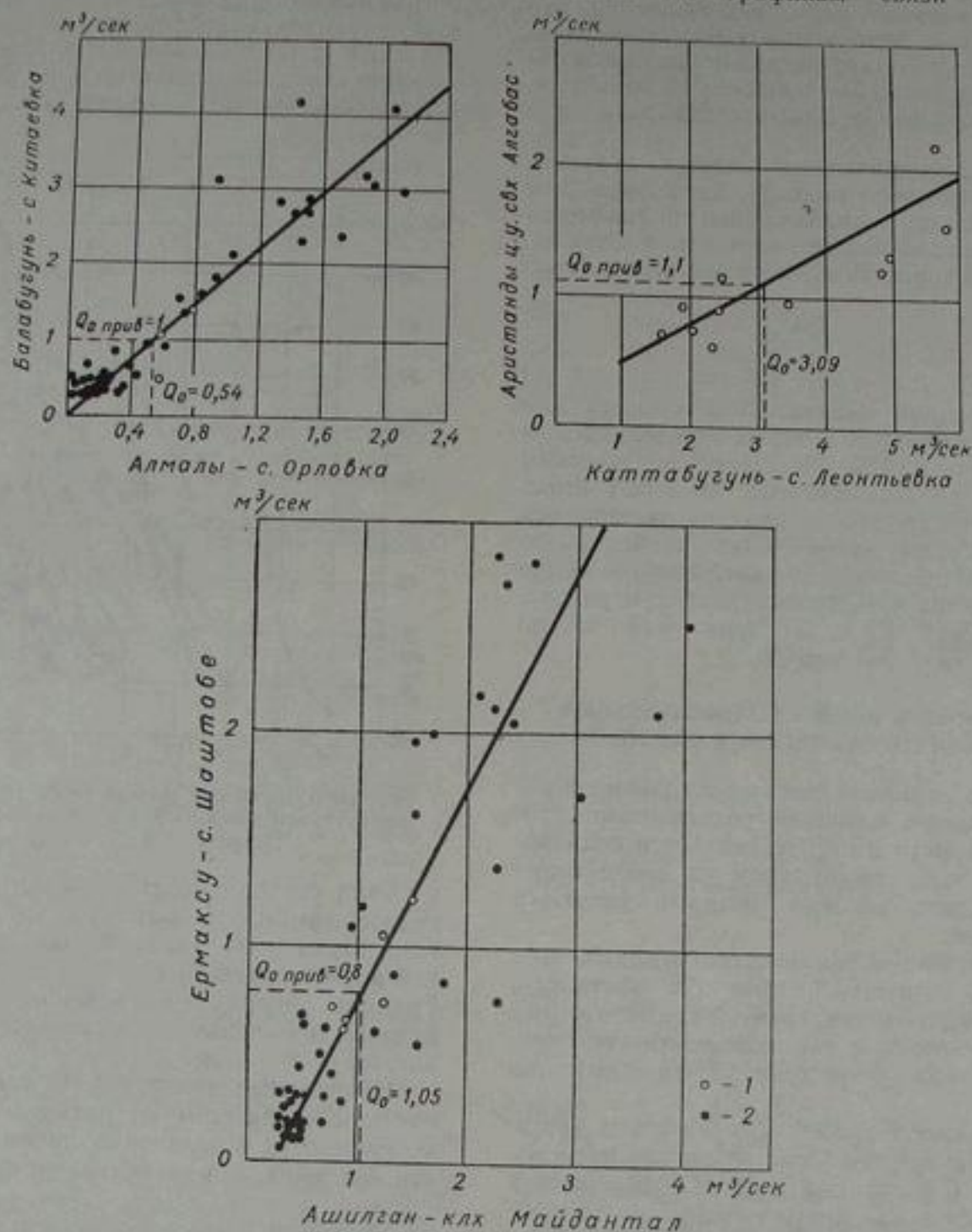
Рис. 41. Графики связи среднегодовых (1) и среднемесячных (2) расходов воды по рекам хр. Каратау.
