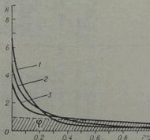
Рис. 74. Средние кривые продолжительности суточных расходов воды рек различных групп.
