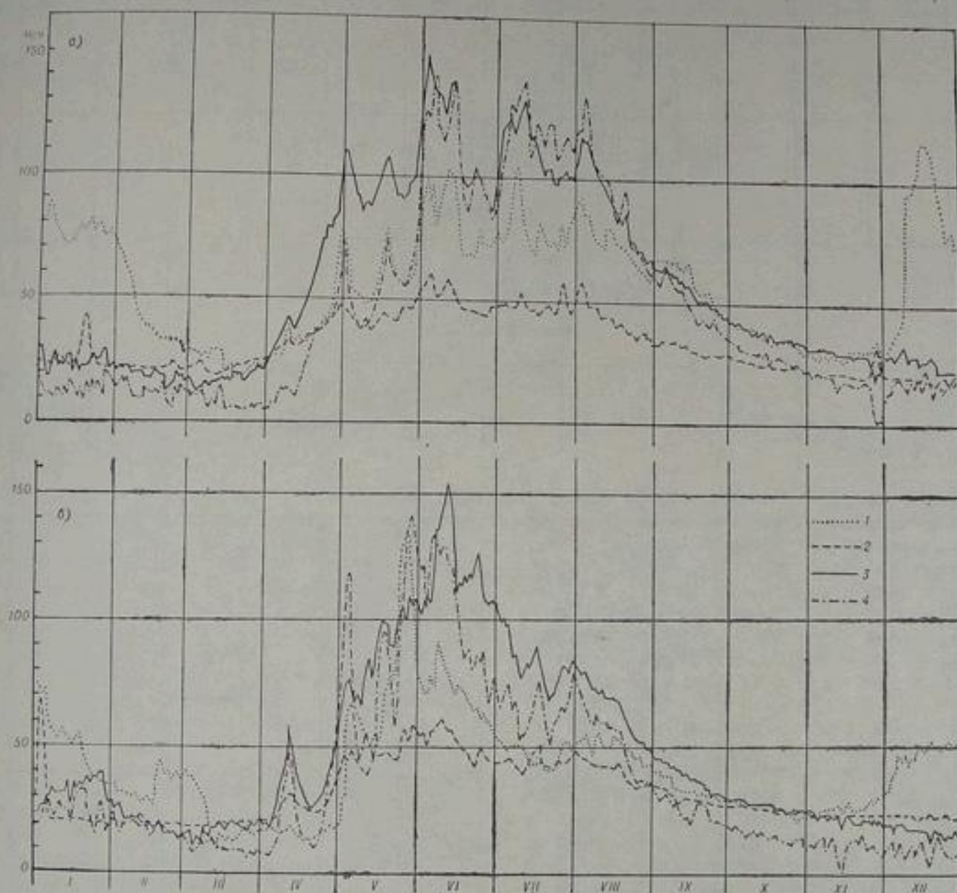
Рис. 24. Годовой ход уровня на реках снегово-ледникового питания.
