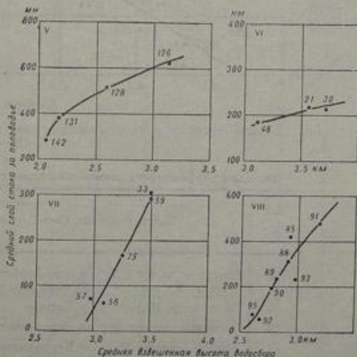
Рис. 82. Зависимость среднего многолетнего слоя стока за половодье от средней высоты водосборов для рек V—VIII районов.
