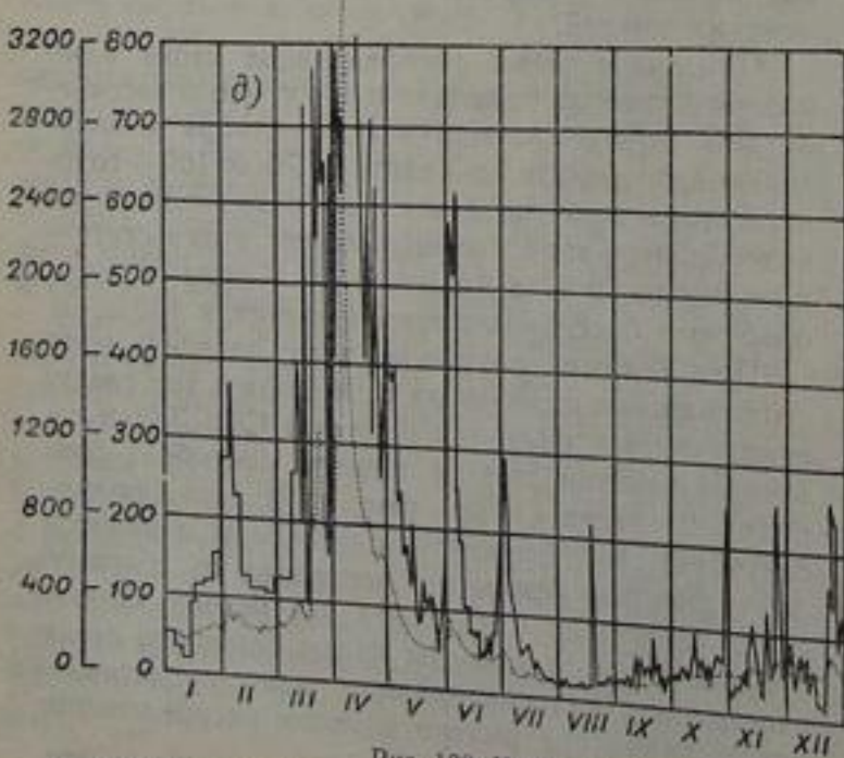
Рис. 138. Хронологические графики хода мутности и расходов воды за 1959 г. а — Кельджерты — х. Акталя, б — Ангбаша — устье р. Ичкекаманды, в — Аралсай — устье р. Косчан, г — Сох — кишла. Сарыканда, д — Арысь — ж.-д. ст. Арысь, е — Каттабугунь — с. Леонтьевна; 1 — расходы воды, 2 — мутность воды.
