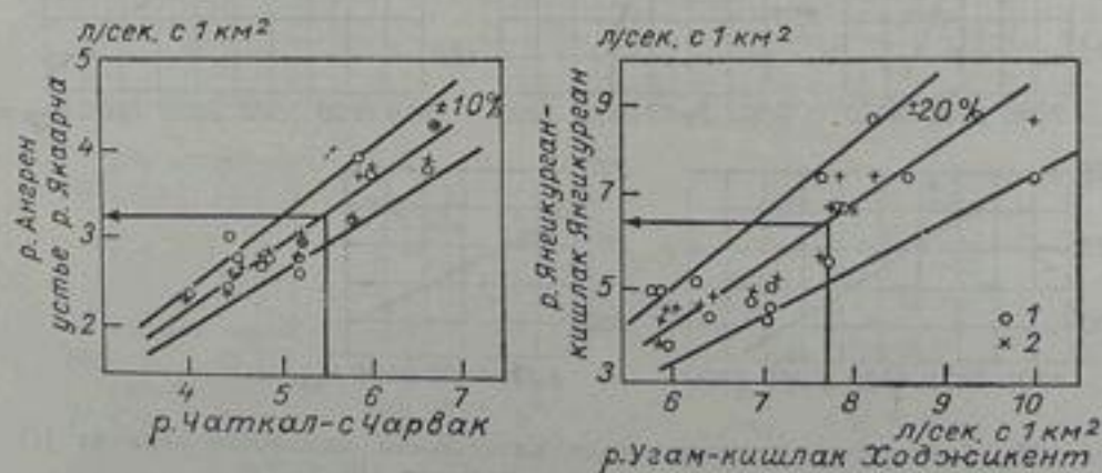
Рис. 102. Графики связи месячных минимальных модулей стока по рекам-аналогам.
