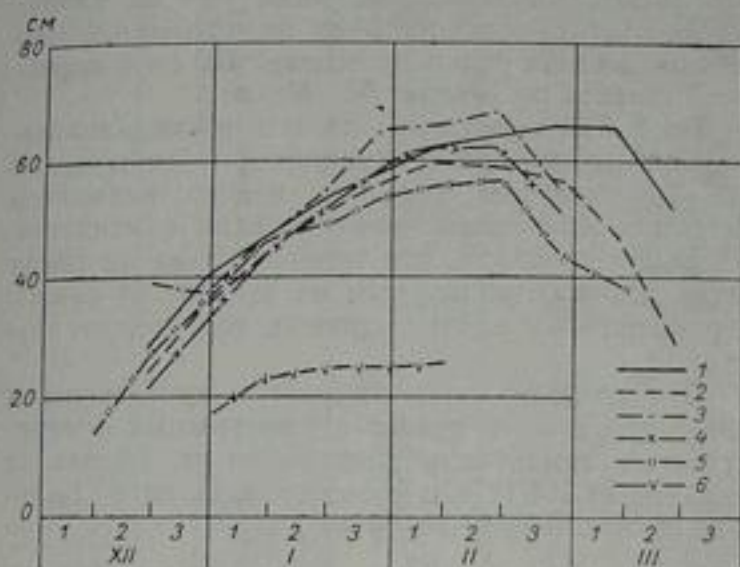
Рис. 125. Средняя многолетняя толщина льда по декадам в разных створах р. Сыр-Дарья.
