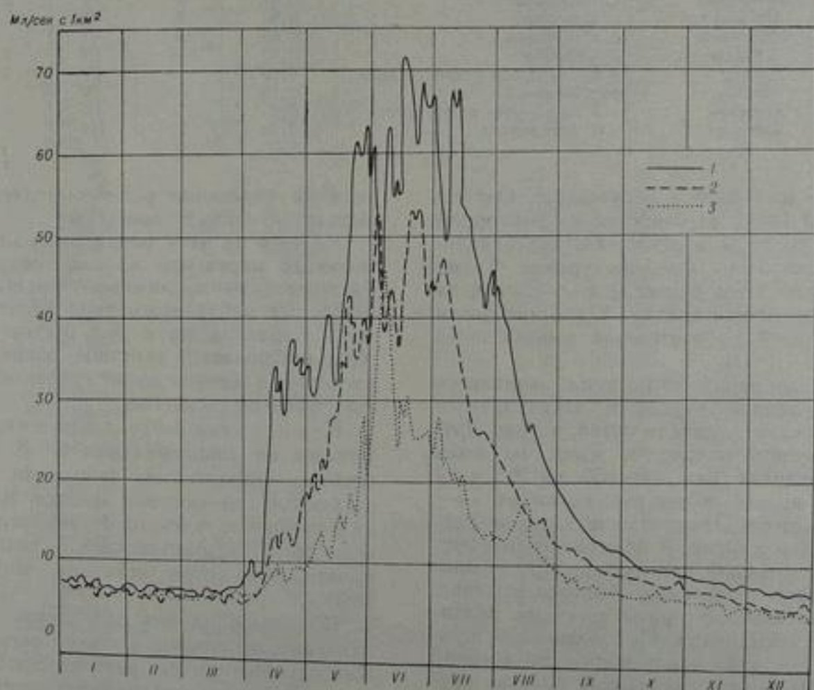
Рис. 16. Гидрографы стока по р. Чаткал — устье р. Терс за характерные по водоносности годы. 1 — 1962 г., 2 — 1943 г., 3 — 1967 г.
