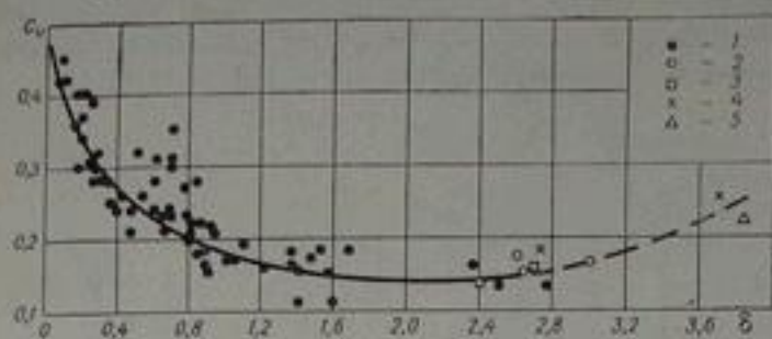
Рис. 57. Зависимость изменчивости годового стока ( C_v ) от типа питания реки ( \delta ).
