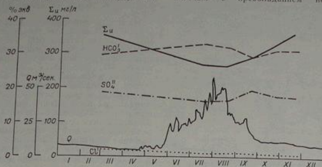
Рис. 161. Внутригодовое изменение минерализации и содержания главных анионов в воде р. Исфара у г. Исфара за 1954 г.
