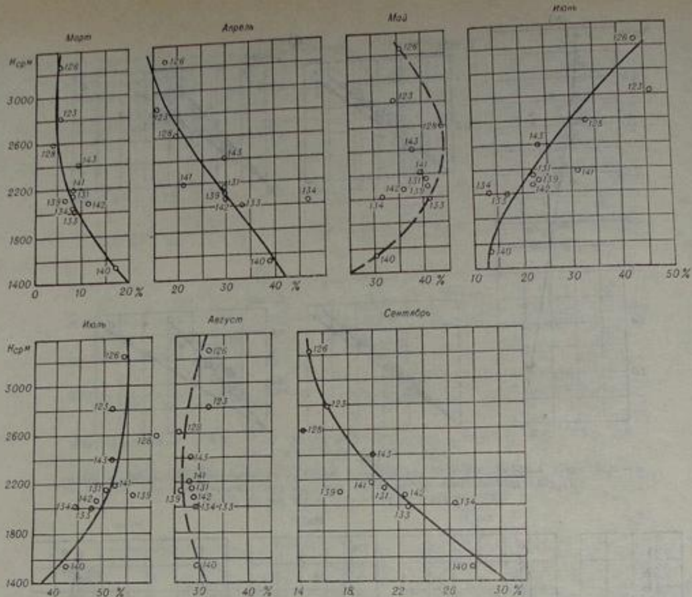
Рис. 69. Зависимость месячного стока весеннего и летнего сезонов (в % от сезонного) от средневзвешенной высоты водосбора H_{cp} для рек II района.
