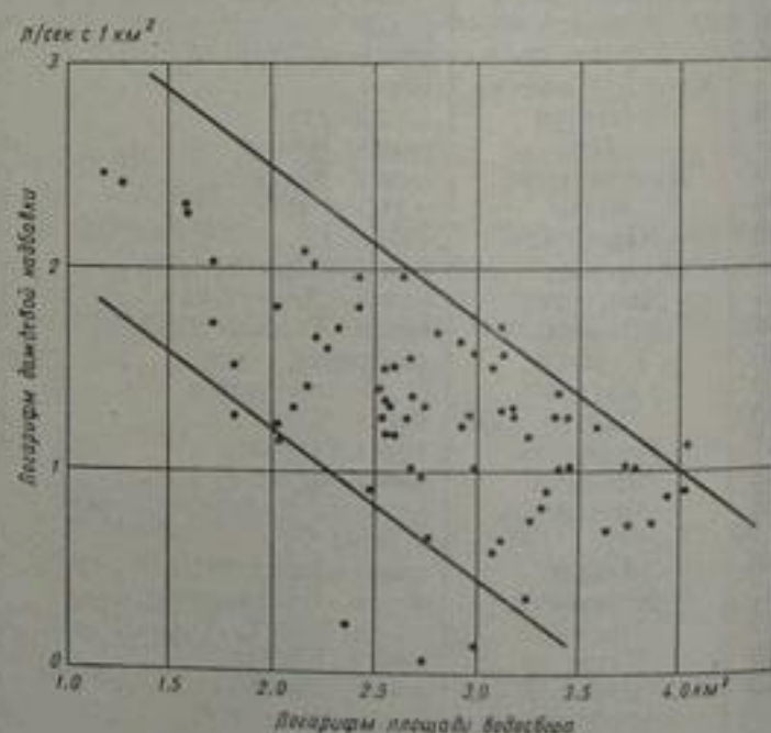
Рис. 87. Зависимость величины дождевой надбавки к максимальным расходам талых вод от площади водосбора.
