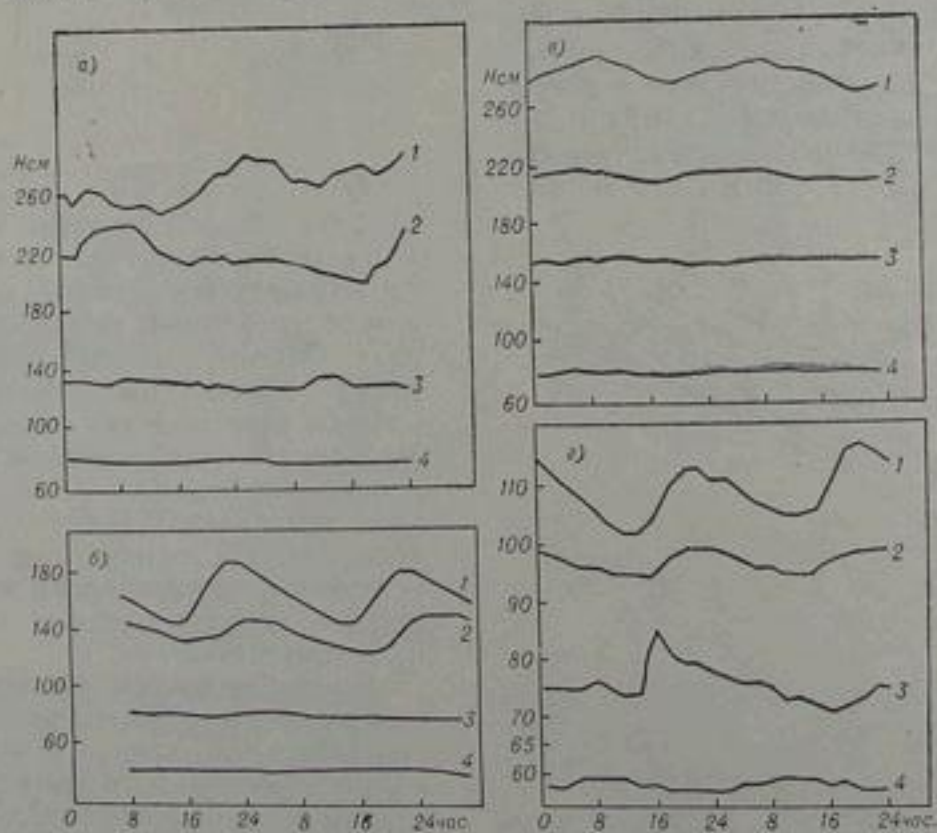
Рис. 32. Суточный ход уровня воды на реках бассейна Сыр-Дарьи в характерные фазы их режима.
