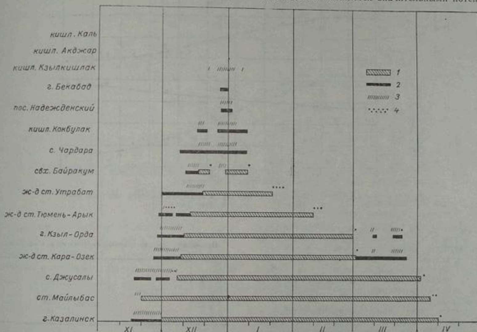
Рис. 122. Совмещенный график ледовых явлений по постам р. Сыр-Дарьи за зиму 1959-60 г.
