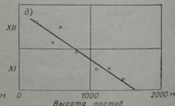
Рис. 119. Зависимость средних дат начала ледовых явлений от высоты постов.
