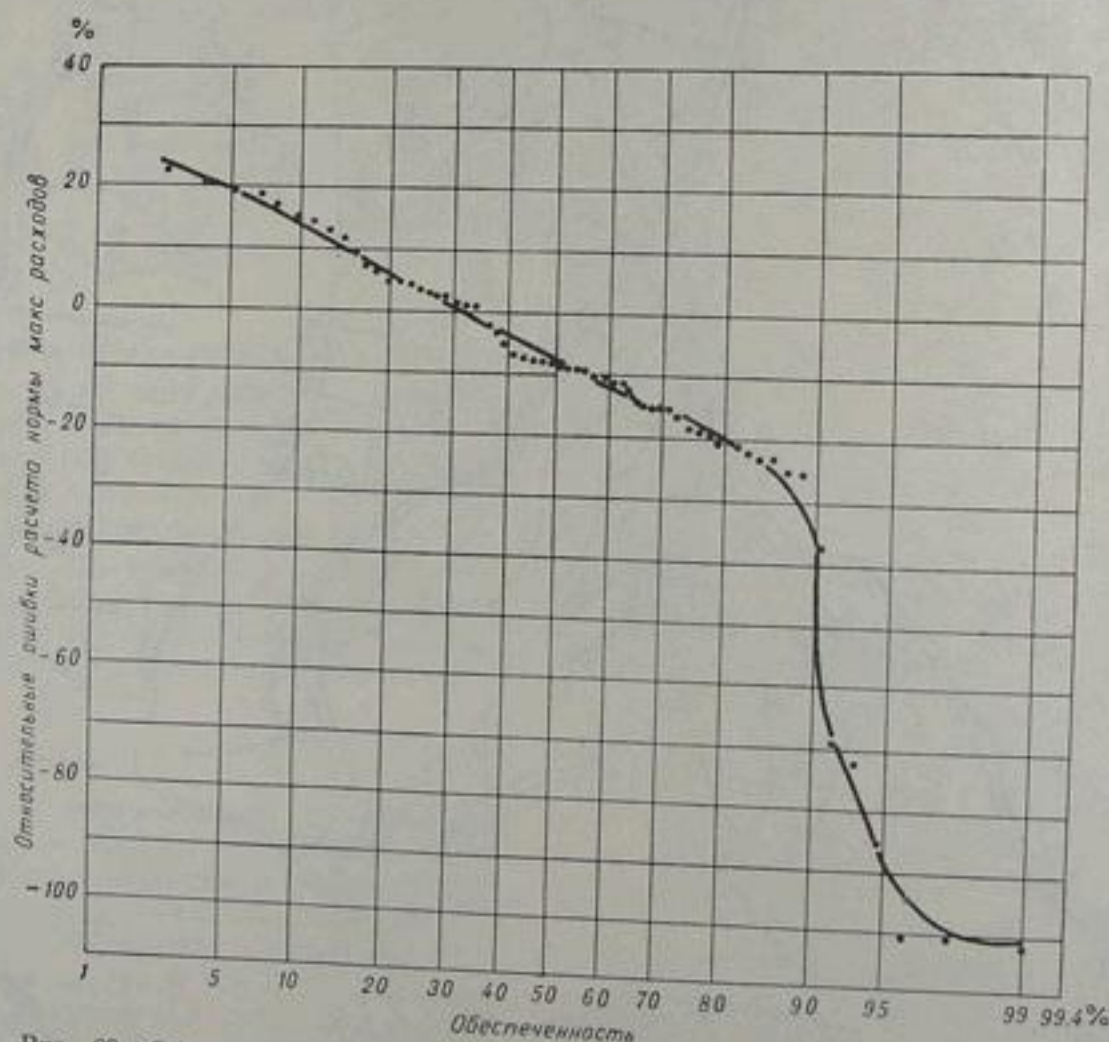
Рис. 89. Обеспеченность относительных ошибок расчета нормы максимального модуля стока.
