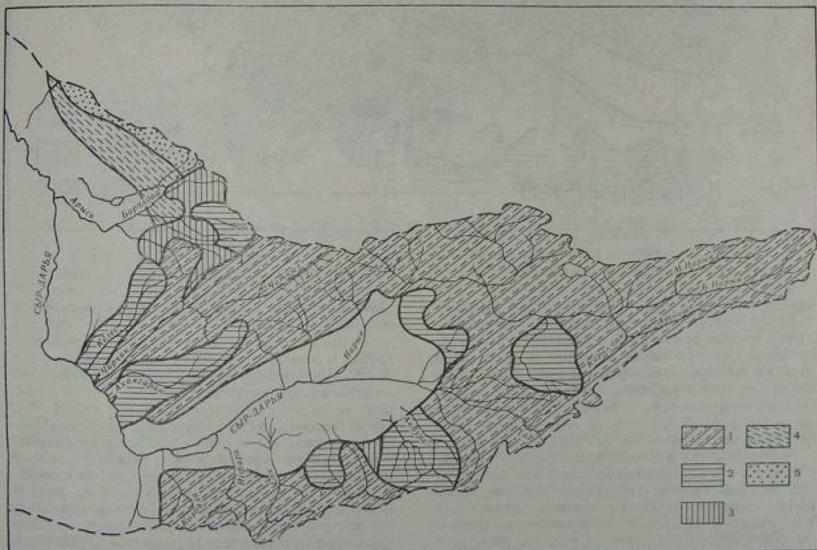
Рис. 139. Схематическая карта распределения стока наносов за октябрь — февраль (в % от годового). 1 — 0—2%, 2 — 3—5%, 3 — 6—10%, 4 — 11—20%, 5 — 21—30%.
