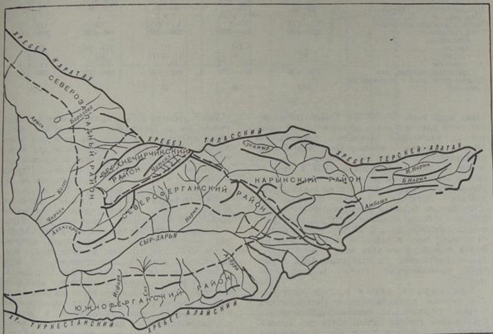
Рис. 21. Схема природного районирования бассейна р. Сыр-Дарья.
