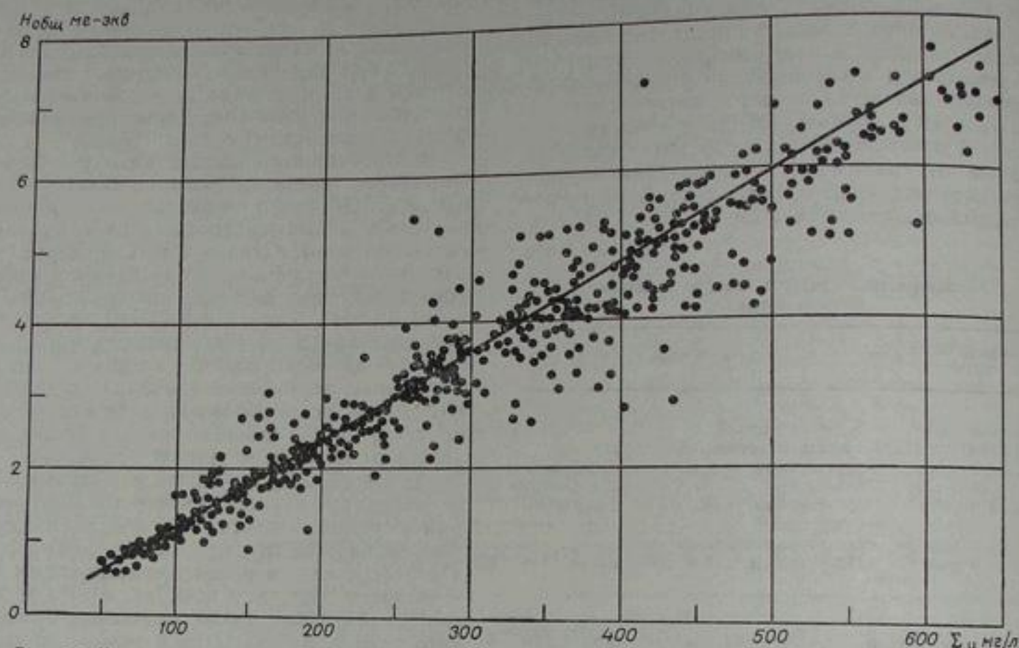
Рис. 177. Характер связи величин общей жесткости ( H ) и минерализации воды ( \Sigma_{и} ) в реках, за исключением р. Сыр-Дарьи, по многолетним данным.
