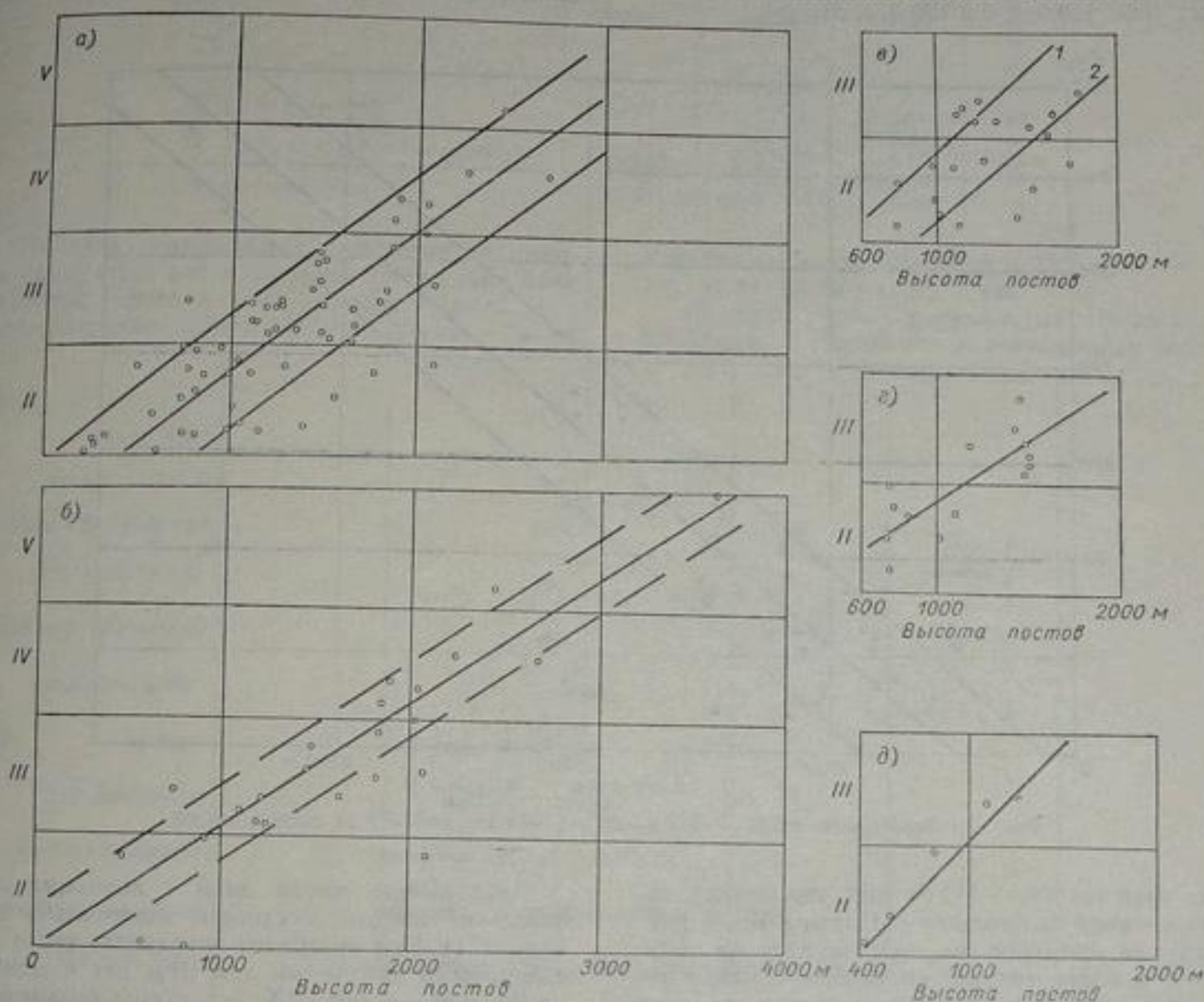
Рис. 120. Зависимость средних дат конца ледовых явлений от высоты постов:
