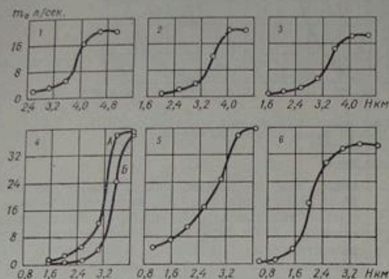
Рис. 44. Районные зависимости зональных модулей нормы годового стока воды от высоты водосборов m_0 = f(H) для рек бассейна Нарына. 1-6 — номера районов.
