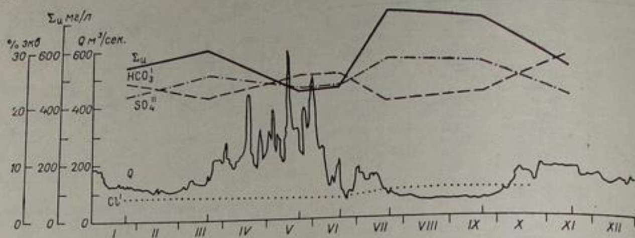
Рис. 159. Внутригодовое изменение минерализации и состава анионов воды р. Карадарьи у кишл. Учтепе, 1956 г.
