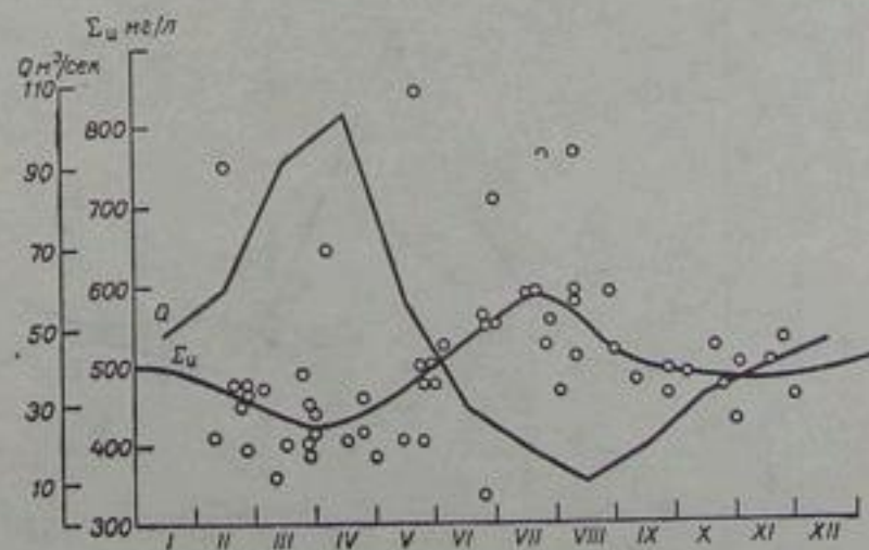
Рис. 172. Внутригодовое изменение минерализации ( \Sigma_{и} ) и расходов воды ( Q ) в р. Арысь у ж.-д. ст. Арысь.
