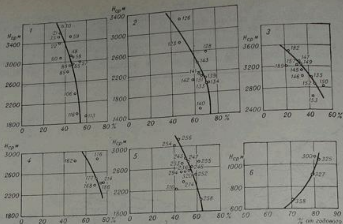
Рис. 65. Зависимость весеннего стока рек бассейна Сыр-Дарьи (в % от годового) от средневзвешенной высоты водосборов H_{cp} .
