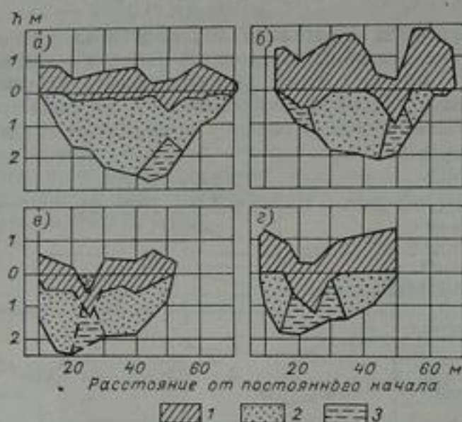
Рис. 127. Поперечные профили по гидропостам рек Большого и Малого Нарына в зимнее время. а — р. Большой Нарын 22/XII 1956 г., б — то же 9/I 1957 г., в — р. Малый Нарын 23/XII 1956 г., г — то же 9/I 1957 г.; 1 — лед, 2 — шуга, 3 — вода.
