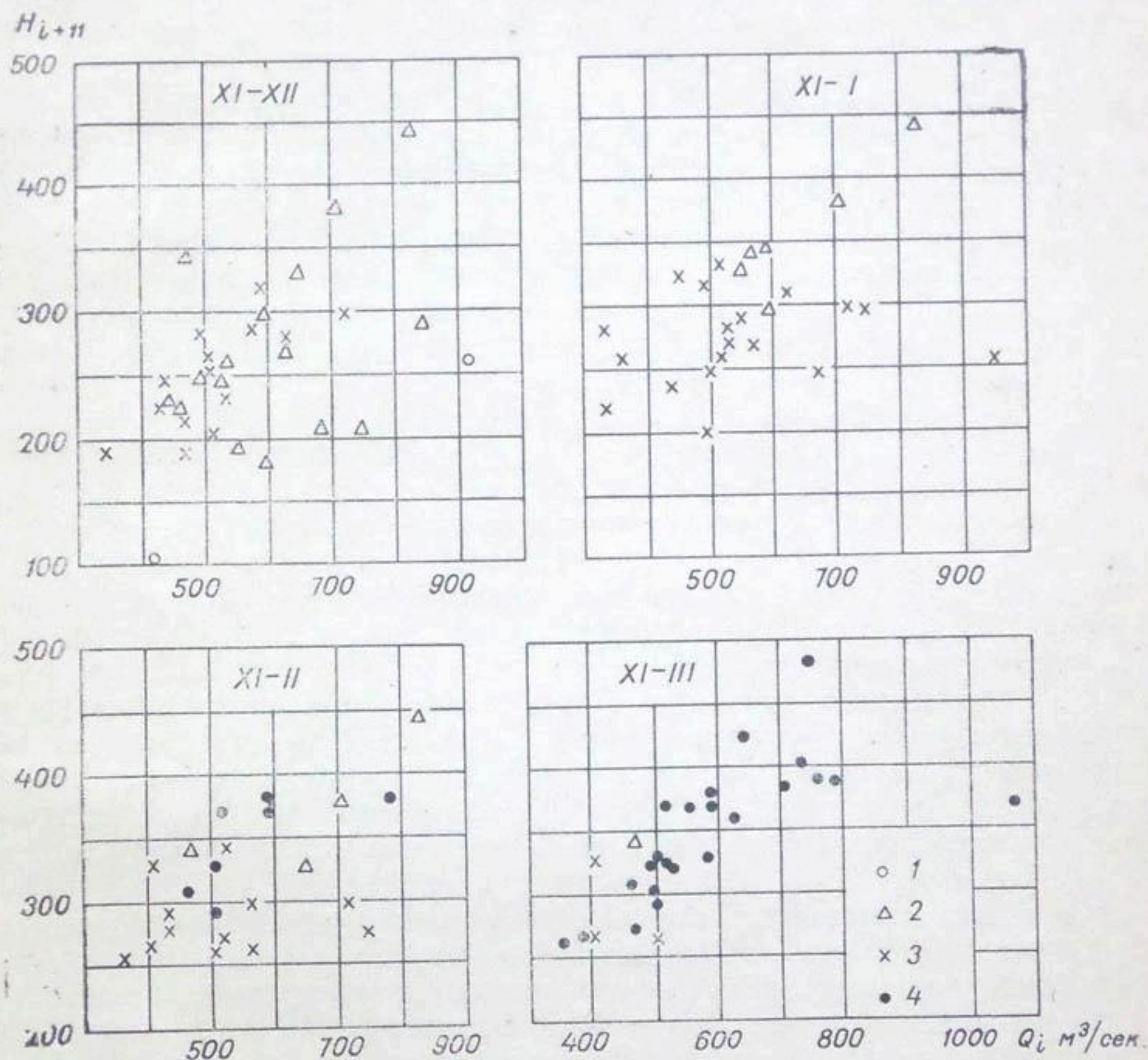
Рис. 6. Зависимость наибольшего (по периодам) уровня в Кзыл-Орде (город) H_{i+n} от соответственного среднего декадного расхода воды в Кок-Булаке (Чардаре) Q_i .
