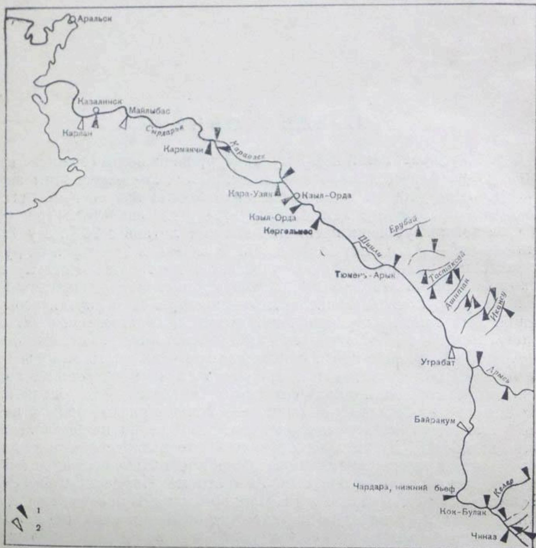
Рис. 1. Схема расположения постов на р. Сырдарье. 1 — посты, учитывающие сток воды, 2 — посты уровенные.
