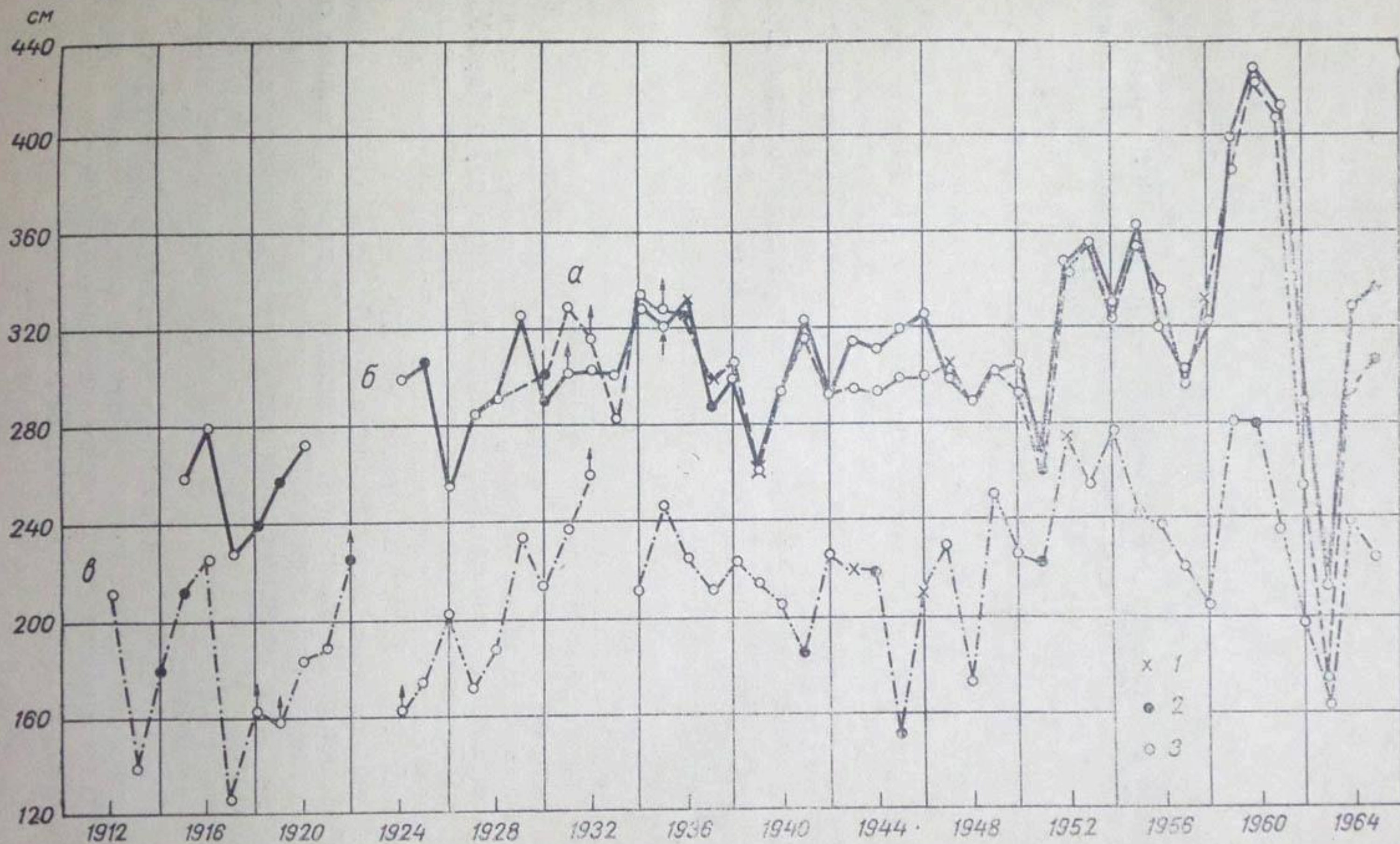
Рис. 2. Высшие зимние уровни на постах Кармакчи, река (а), Кармакчи, проток (б) и Казалинск (в). ; — замерзание, 2 — ледостав, 3 — вскрытие; стрелка — высший уровень не был отмечен.
