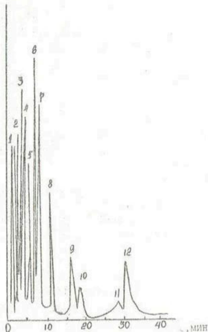
рис. 1. Хроматограмма элюата первой градиентной ступени. P - сигнал детектора, мм; t - время удерживания, мин; 1-4-ГХБД, ПХНБ; α β γ - ГХЦГ, ДДЕ, трефлан, тиодан-1, ДЛТ; 5 - изофен, сатурн; 6 - дактал; 7 - иллоксан; 8 - карбофос, кельтан, мета- фос; 9 - фозалон; 10 - рамрод; 11 - дихлофос; 12 - фталофос.
