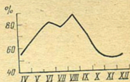
Рис. 2. Внутригодовой ход потребления азота в Восточно-Арнасайских озерах
