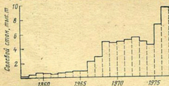
Рис. 3. Ежегодный привнос солей с коллекторно-дренажными водами в Арнасайские озера
