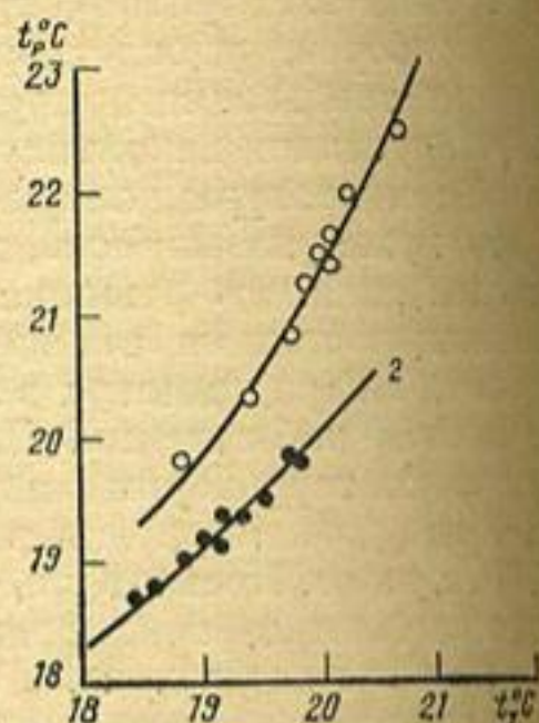
Рис. 3. Связь температур воды измеренной ртутным термометром ( t_w ) и ИК радиометром ( t_p ):
