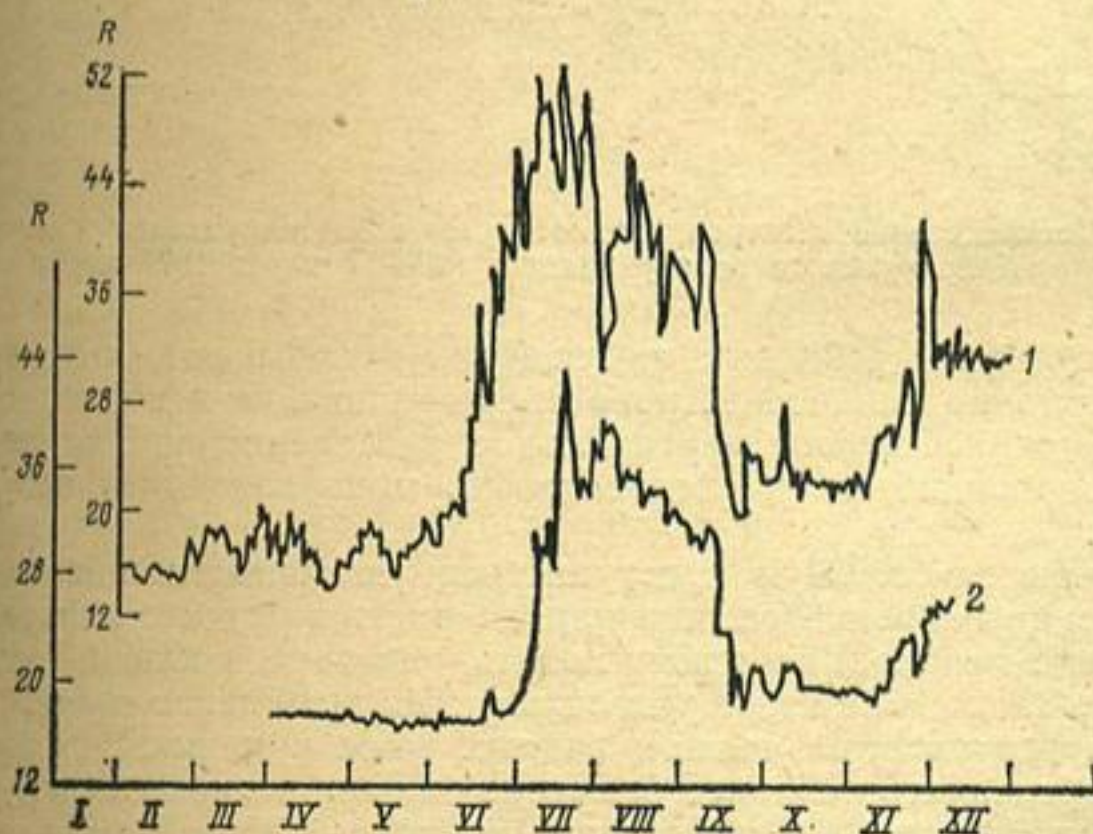
Рис. 1. Ежедневное сопротивление воды на постах Акдзар (1) и Кайракум (2) за 1977 г.
