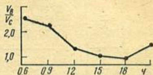
Рис. 2. Суточный ход соотношений скорости ветра над водоемом и сушей
