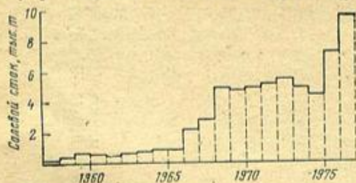
Рис. 3. Ежегодный привнос солей с коллекторно-дренажными водами в Арнасайские озера
