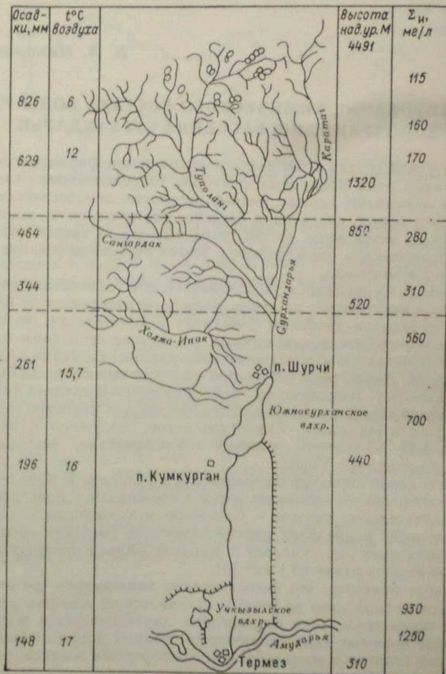
Рис. 1. Изменение минерализации воды р. Сурхандарья по длине реки.
