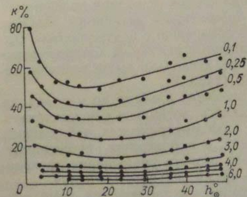
Рис. 2. Зависимость альбедо и коэффициента пропускания от высоты Солнца.
