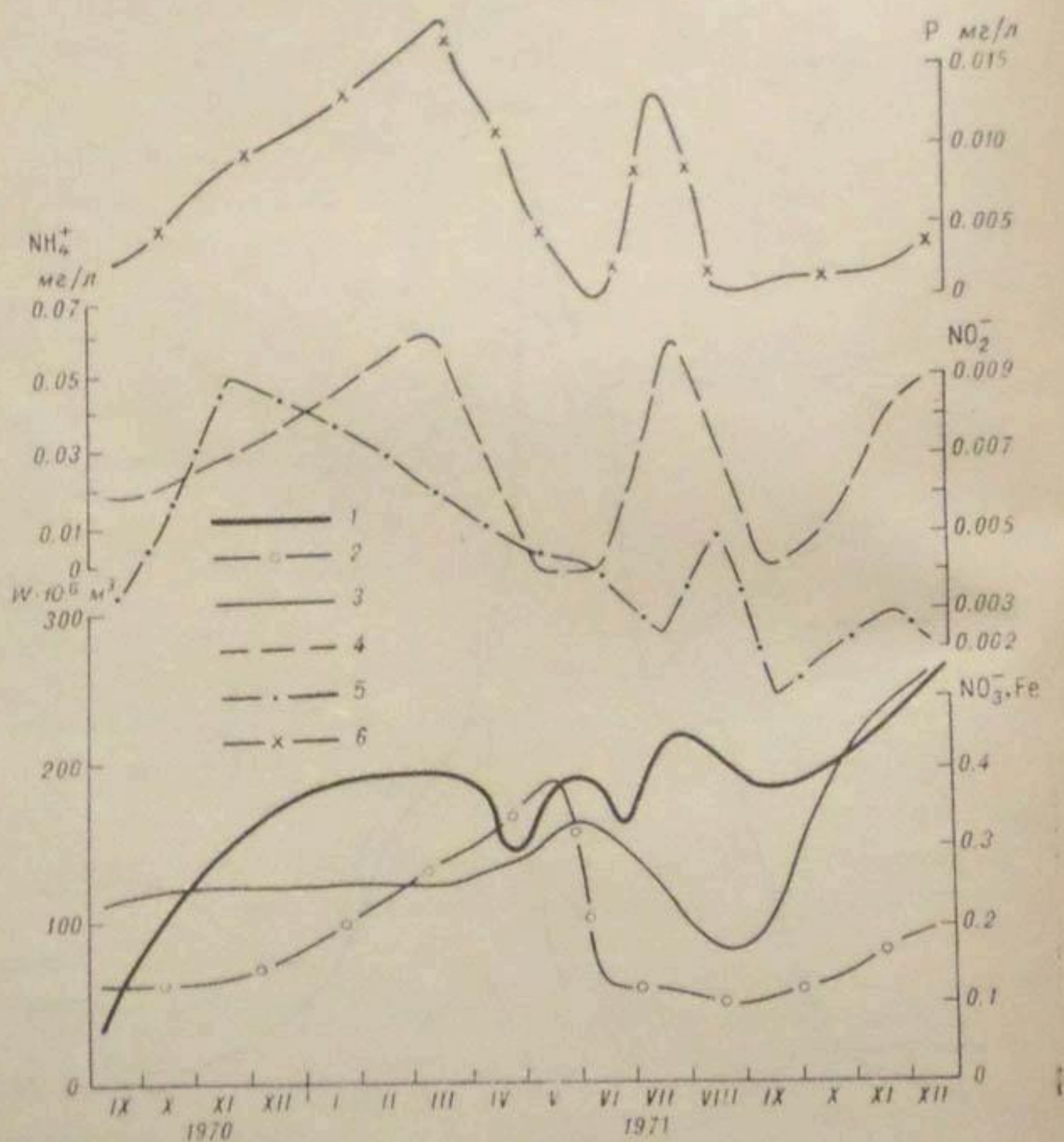
Рис. 3. Динамика биогенных элементов в воде приплотинного участка Чарвакского водохранилища (поверхностный слой). 1 — расходы воды, 2 — Fe, 3 — N_{NO_3^-} , 4 — N_{NH_4^+} , 5 — N_{NO_2^-} , 6 — P.
