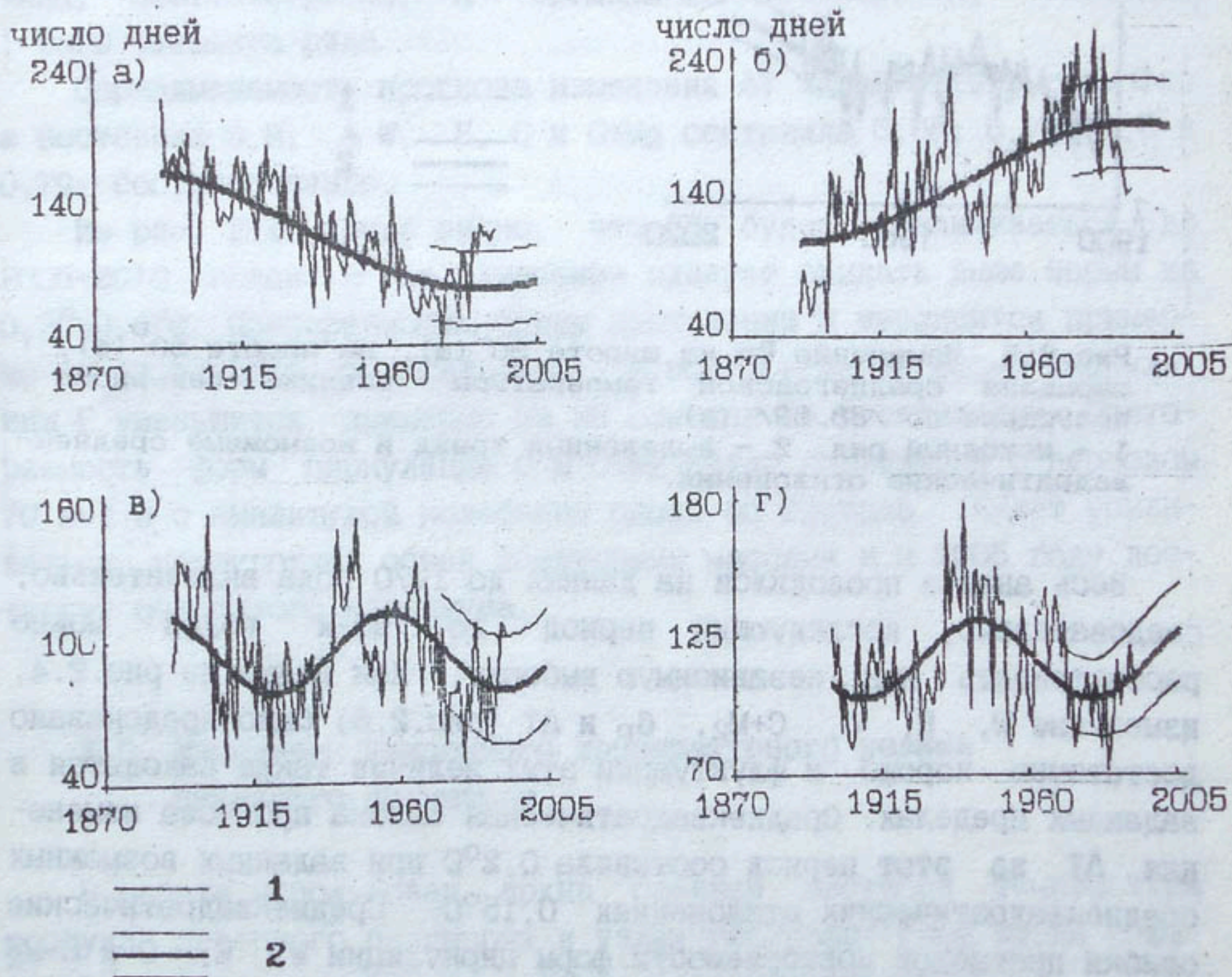
Рис.2.4. Изменение повторяемости форм циркуляции W (а), E (б), S (в), S+M_2 (г).
