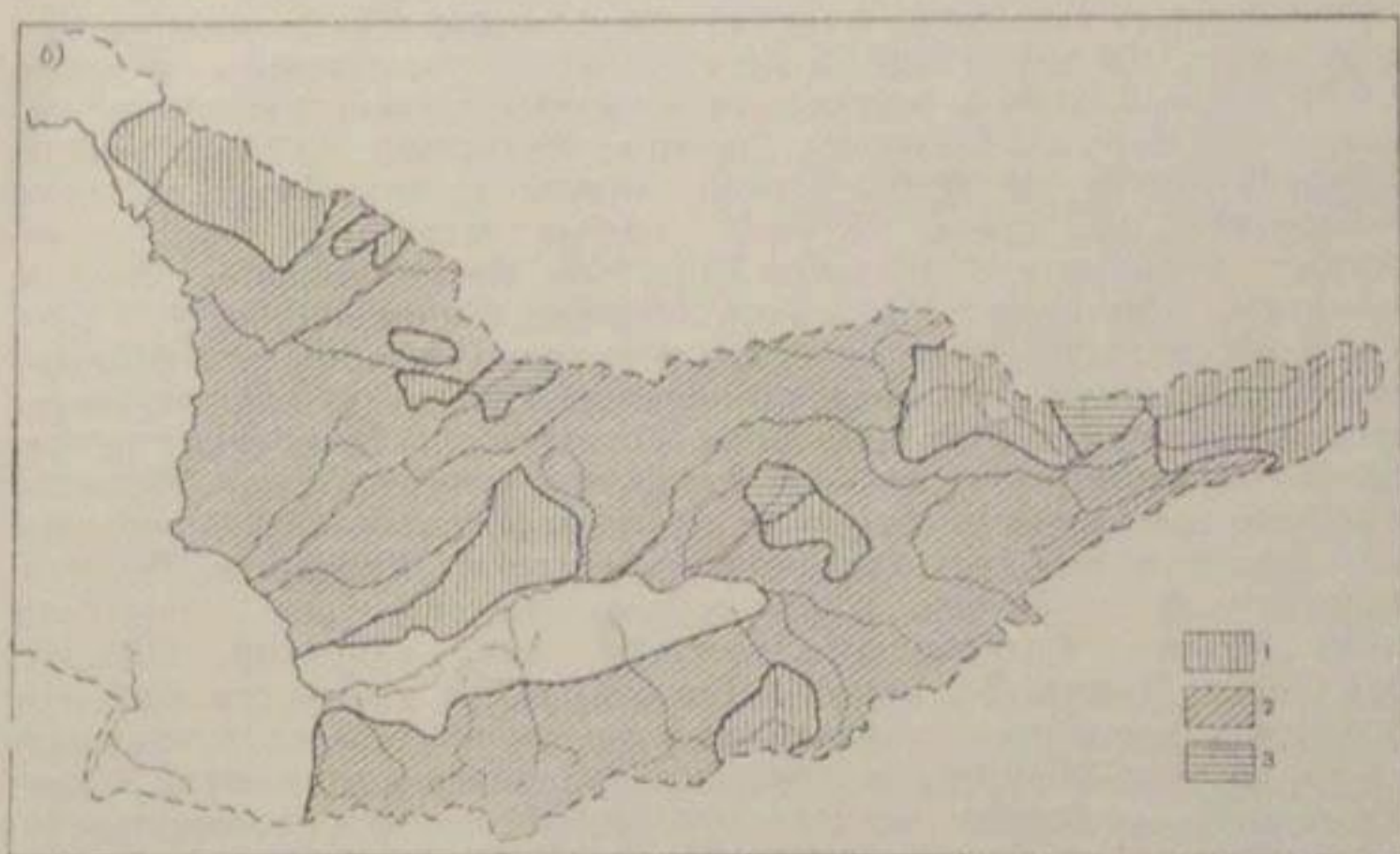
Рис. 29. Схематические карты крупности взвешенных иллов в реках бассейна Сыр-Дарья
