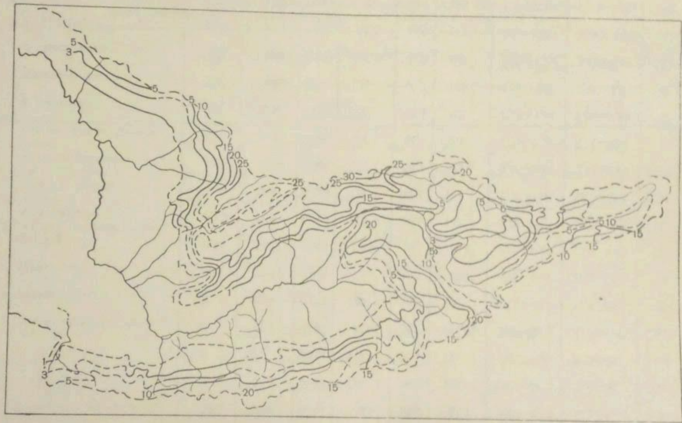
Рис. 17. Схематическая карта модулей стока воды рек бассейна Сыр-Дарьи (л/сек. с км²).
