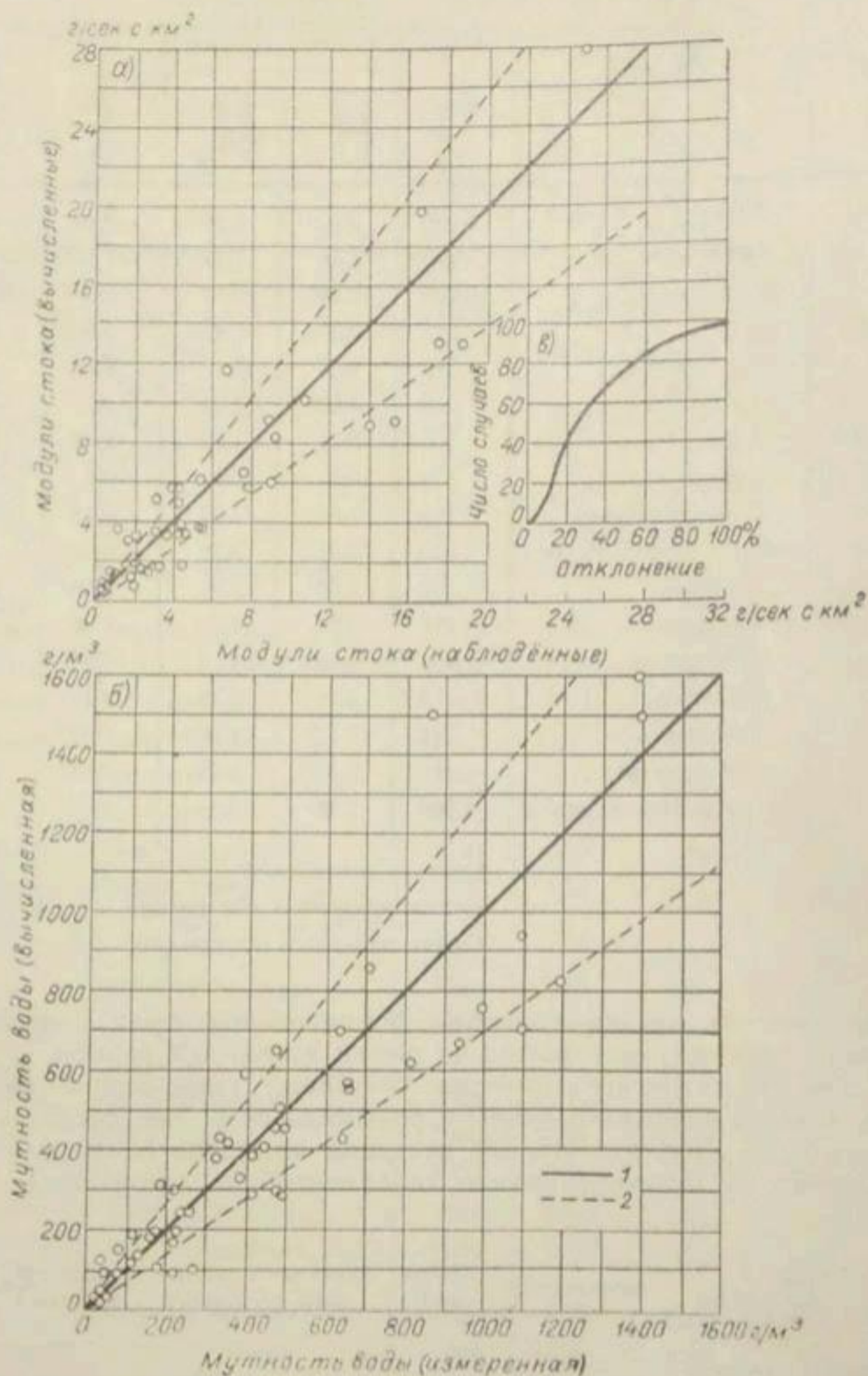
Рис. 16. Связь вычисленных и наблюдаемых модулей стока взвешенных наносов ( а ), вычисленных и наблюдаемых мутностей ( б ) и интегральная кривая распределения отклонений вычисленных модулей стока взвешенных наносов от наблюдаемых ( в ).
