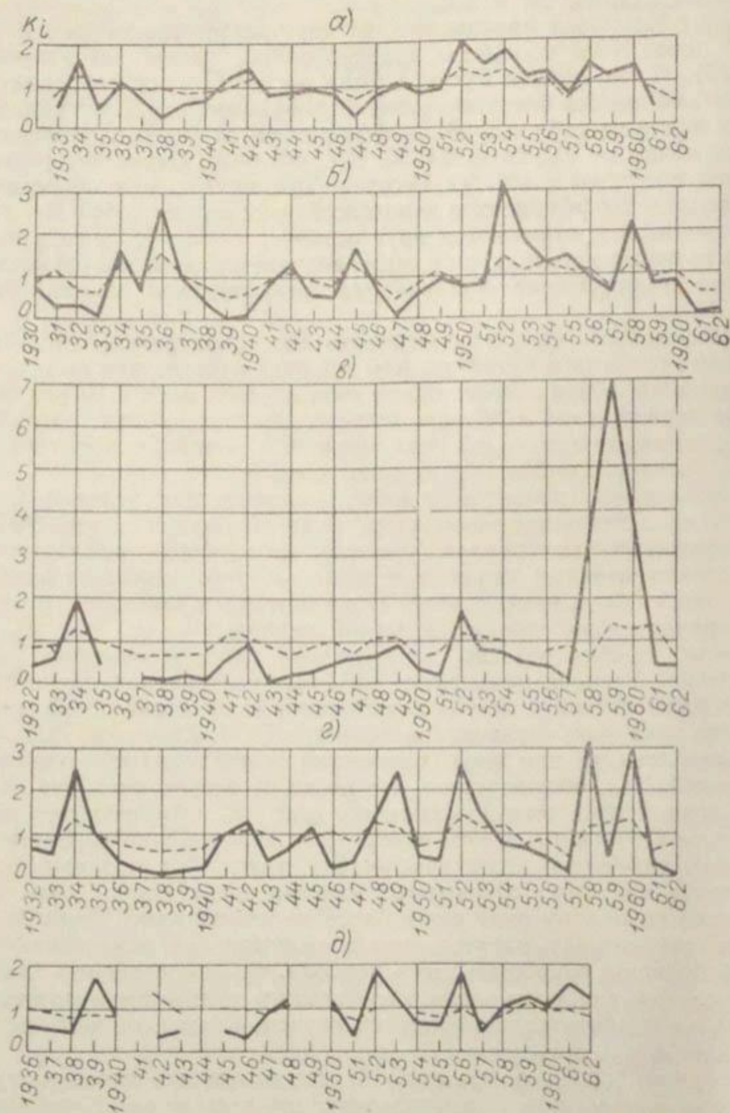
Рис. 18. Колебание модульных коэффициентов средних годовых а — р. Нарын — кишл. Учкурган, б — р. Карадарья — кишл. Кампырран в — р. Сох — кишл. Сарыканда, г — р. Ойганг — устье, ж — р. Пскем — 1 — модульные коэффициенты расходов взвешенных паводков, 2 — модуль
