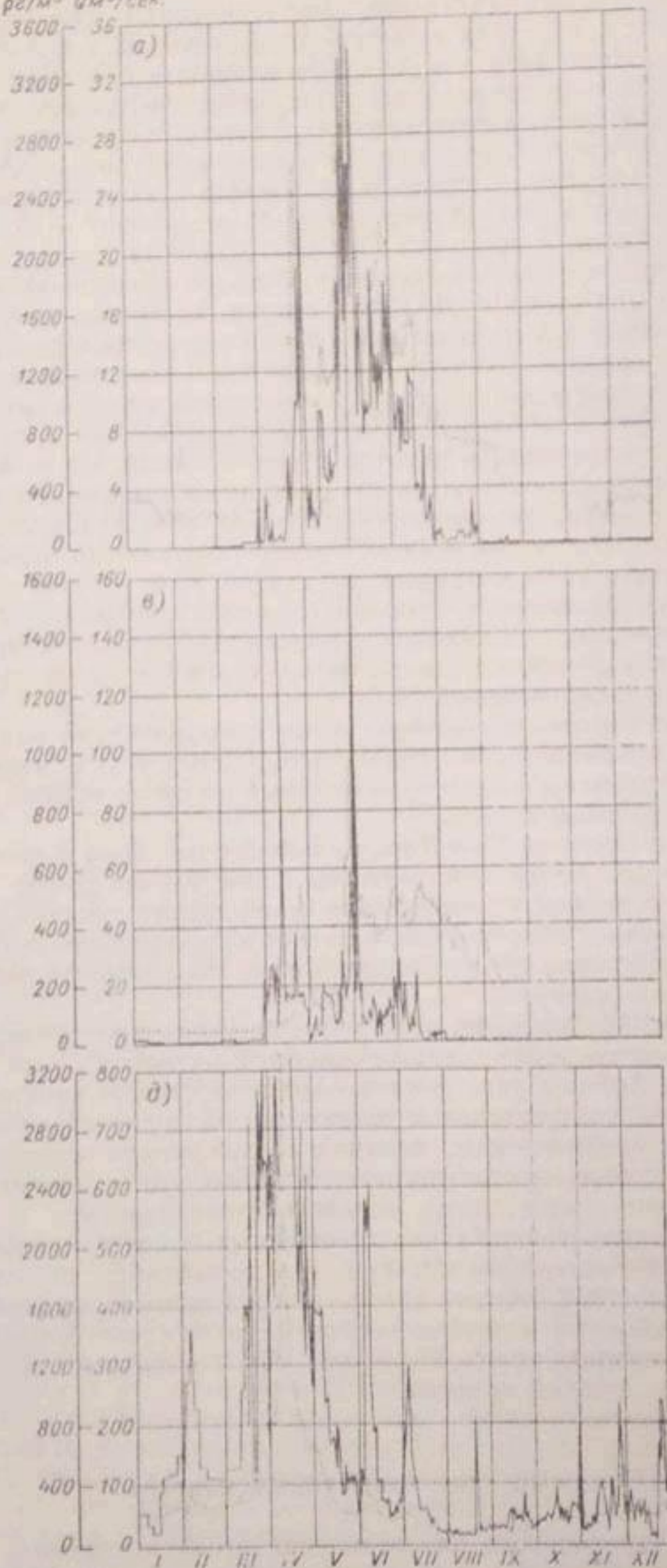
Рис. 25. Ежедневные расходы воды ( I ) и величины мутности
