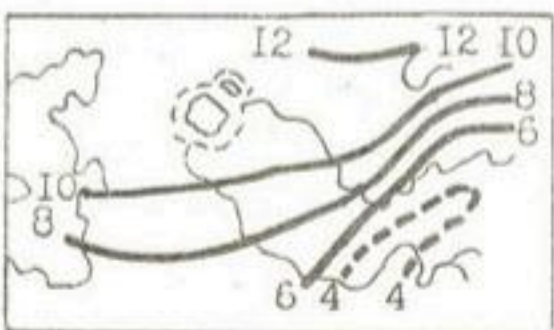
октябрь 700 гПа
