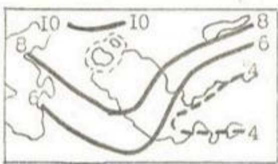
июль 700 гПа
