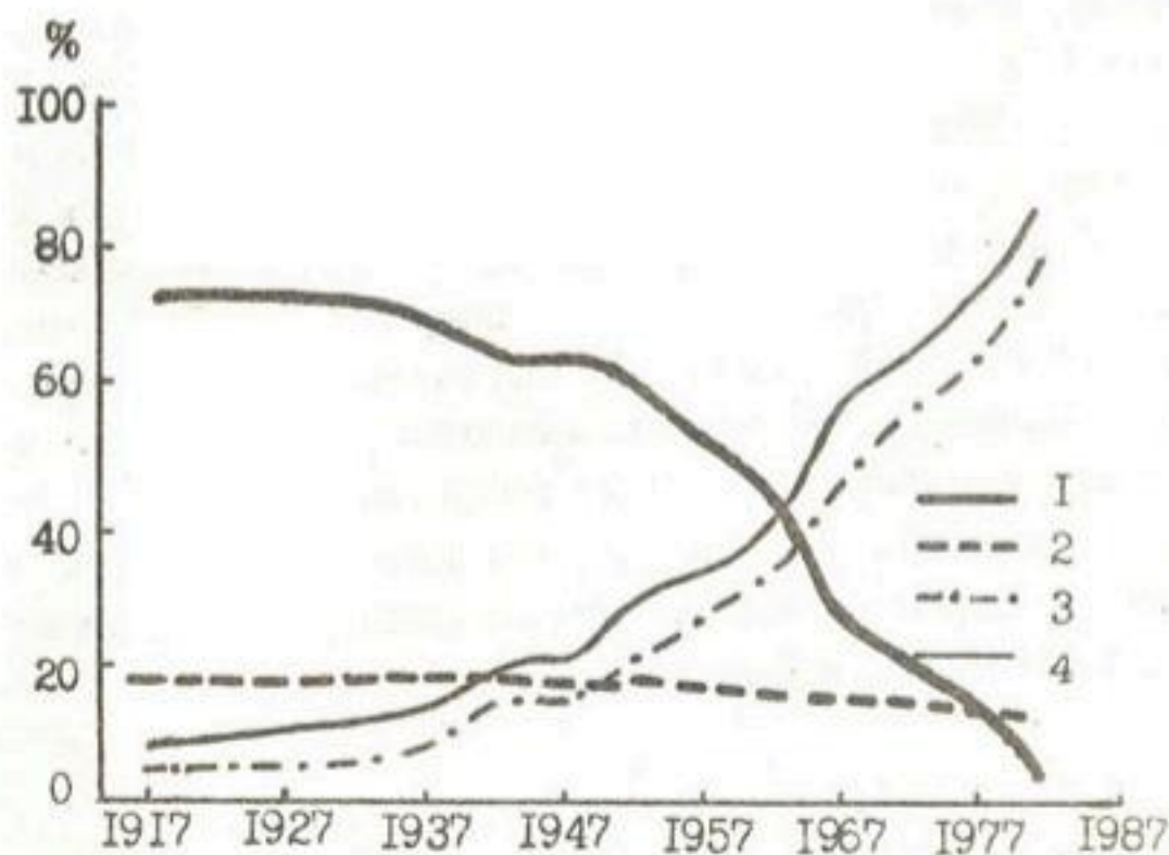
Рис. 8.2. Изменения структуры теплового баланса в Голодной степи. 1- \bar{LE}/\bar{R} , 2- F_{ор}/F_{общ} , 3- \bar{B}/\bar{R} , 4- \bar{P}/\bar{R} .
