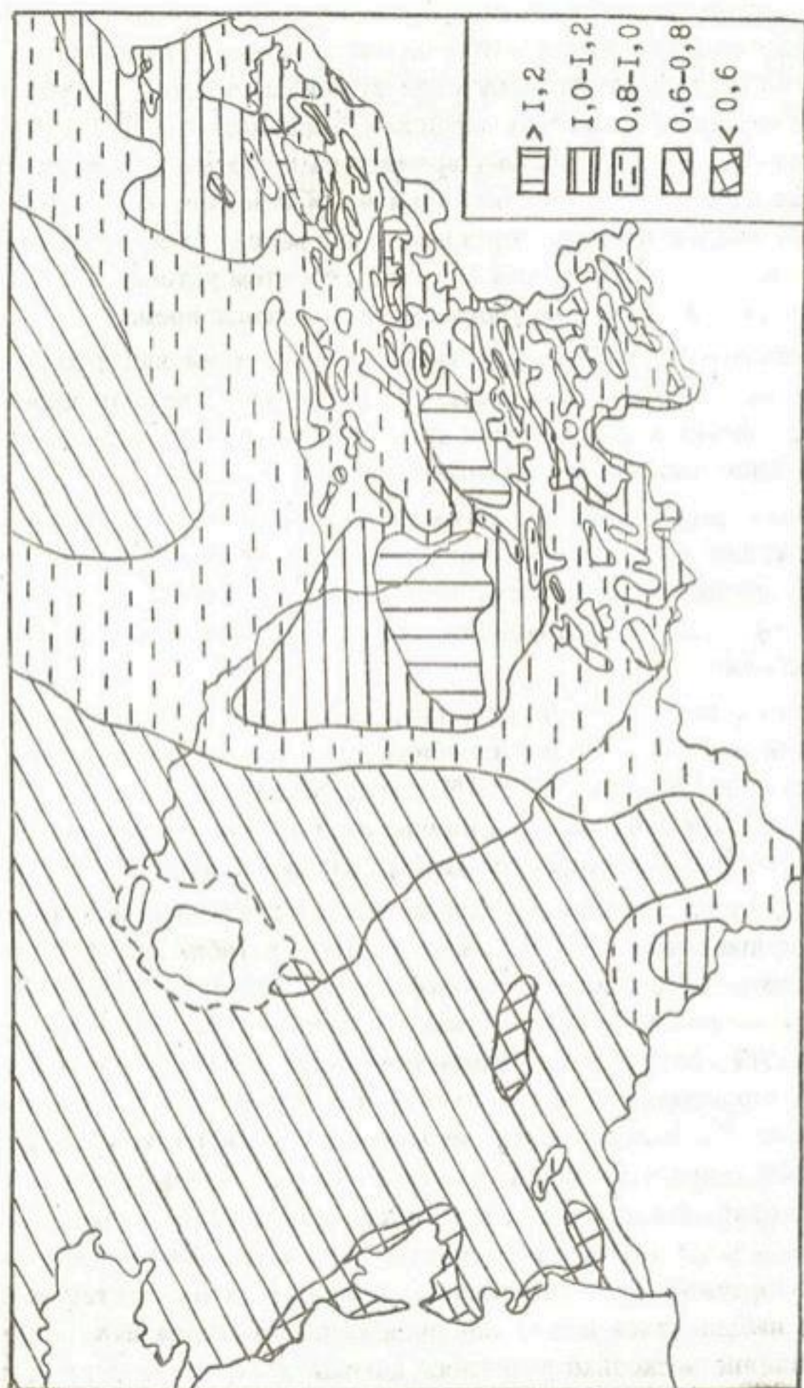
Рис. 7.2. Карта - схема распределения коэффициента вариации С у скорости ветра.
