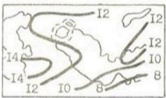
июль 500 гПа
