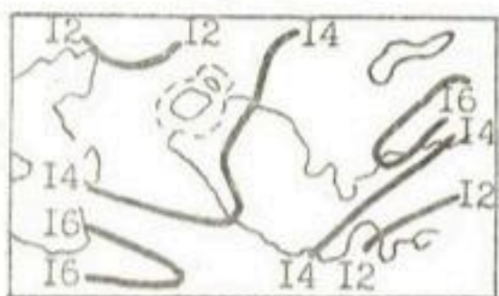
апрель 500 гПа
