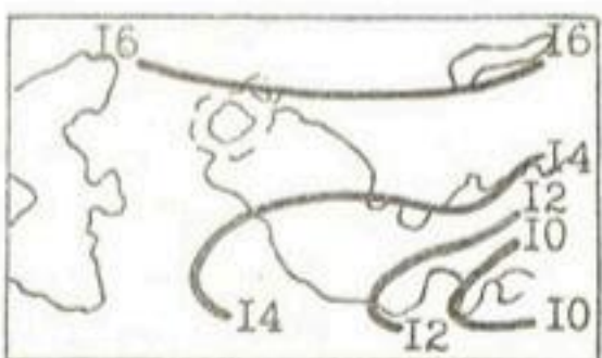
октябрь 500 гПа
