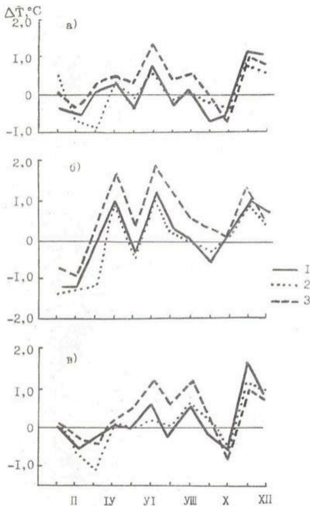
Рис. 3.3. Годовой ход разности средних месячных температур воздуха (1), минимальных (2) и максимальных (3) между периодами: а) (1961-1990) - (1931-1960), б) (1971-1980) - (1931-1960), в) (1981-1990) - (1931-1960) гг. на станции Анзобский перевал.
