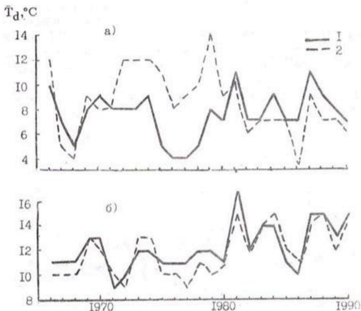
Рис. 6.5. Многолетний ход температуры точки росы в Тамбове (а), Термезе (б) в июле в разное время суток. 1 - 03ч, 2 - 12ч.
