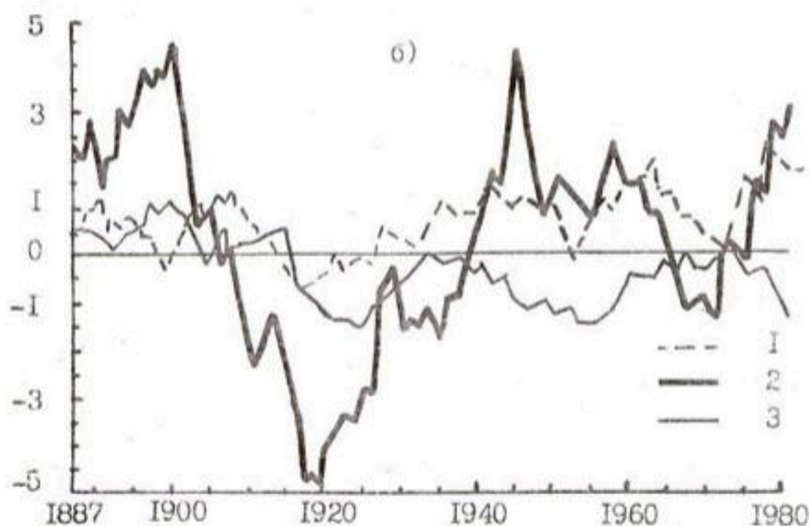
Рис. 6.7. Десятилетние скользящие средние отклонения от нормы повторяемости ( \Delta\P , %) сочетаний различных градаций температуры воздуха \leq 22,0^\circ (1), 22,1-27,9^\circ (2), \geq 28,0^\circ\text{C} (3) с относительной влажностью 41-60% в Ташкенте. а) июль, б) август.
