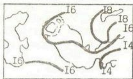
январь 500 гПа
