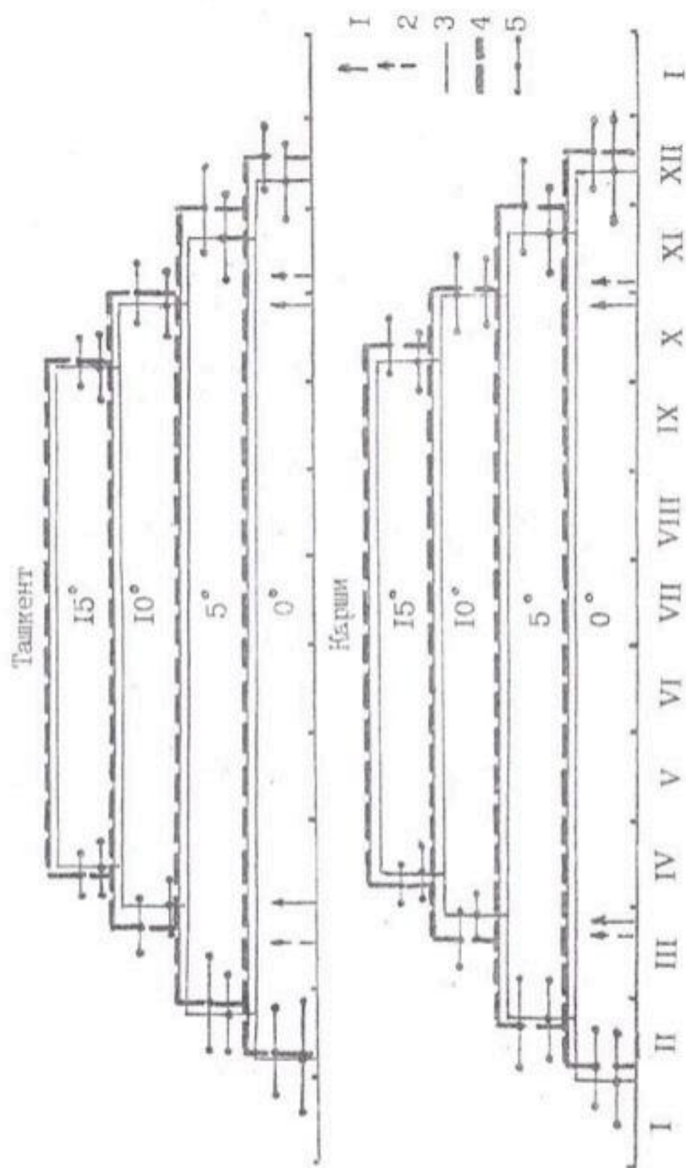
Рис. 4.12. Диаграмма изменения крайних дат заморозков (1, 2) и дат перехода средних суточных температур воздуха (3, 4) через различные пределы на станциях Ташкент и Карши. 1, 3- период 1936-1960 годов; 2, 4- период 1961-1985 годов; 5- \sigma .
