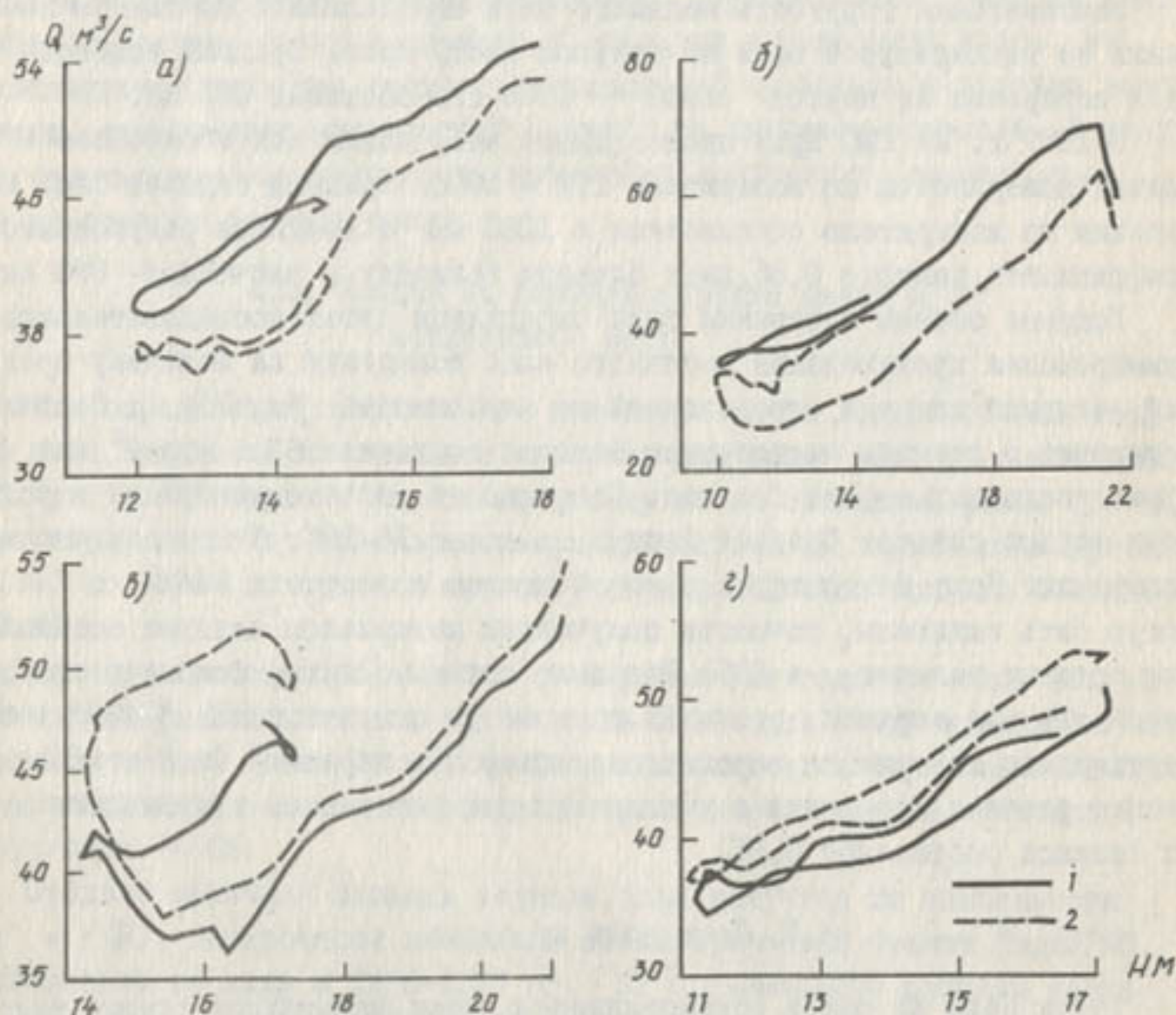
Рис. 4.1. Зависимость расходов воды р. Бартанг (п. Барчишев) от уровня воды в Сарезском озере в 1972 (а), 1973 (б), 1974 (в), 1975 (г) гг.:
