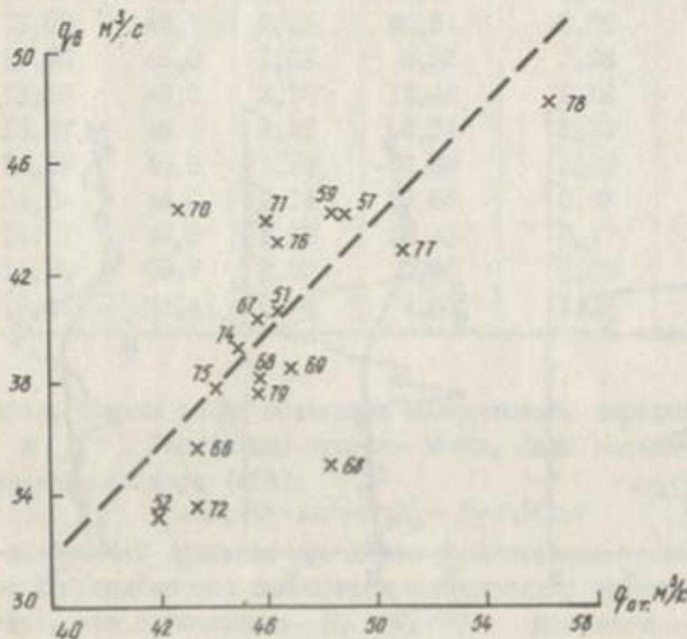
Рис. 4.3. Связь среднегодовых расходов воды р. Бартанг - п. Барчидев ( q_{\text{б}} ) и среднегодового оттока из озера ( q_{\text{от}} ), вычисленного по уравнению (4.10)
