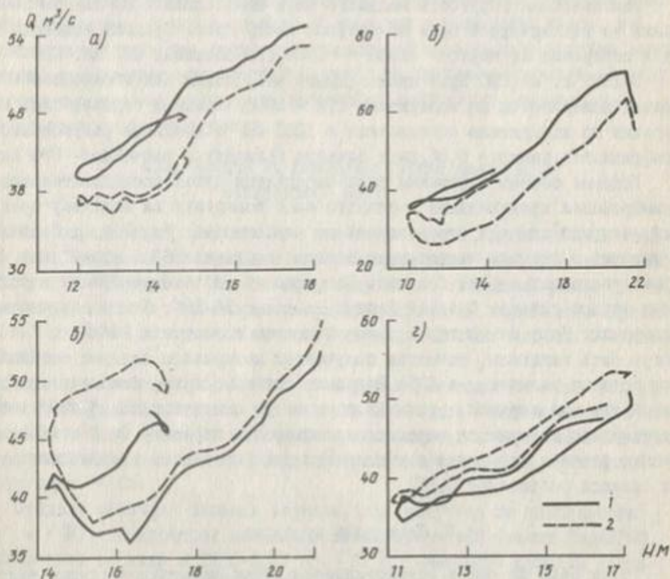
Рис. 4.1. Зависимость расходов воды р. Бартаг (п. Барчидава) от уровня воды в Сарезском озере в 1972 (а), 1973 (б), 1974 (в), 1975 (г) гг.: 1 — без поправки на боковую приточность, 2 — с поправкой
