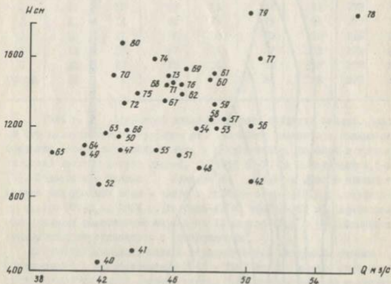
Рис. I.4. Зависимость расходов воды (п.Барчицев) от уровня озера (цифры у точек – годы).
