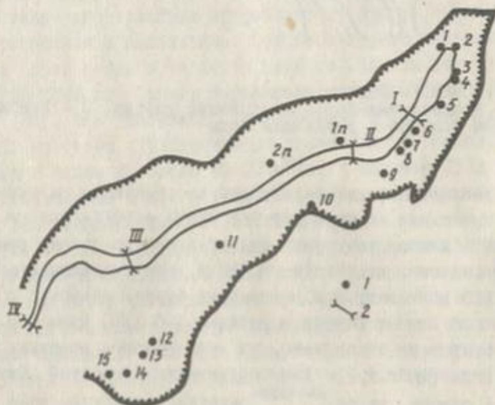
Рис. 1.2. Схема каньона на теле завала: 1 - родники, 2 - створы
