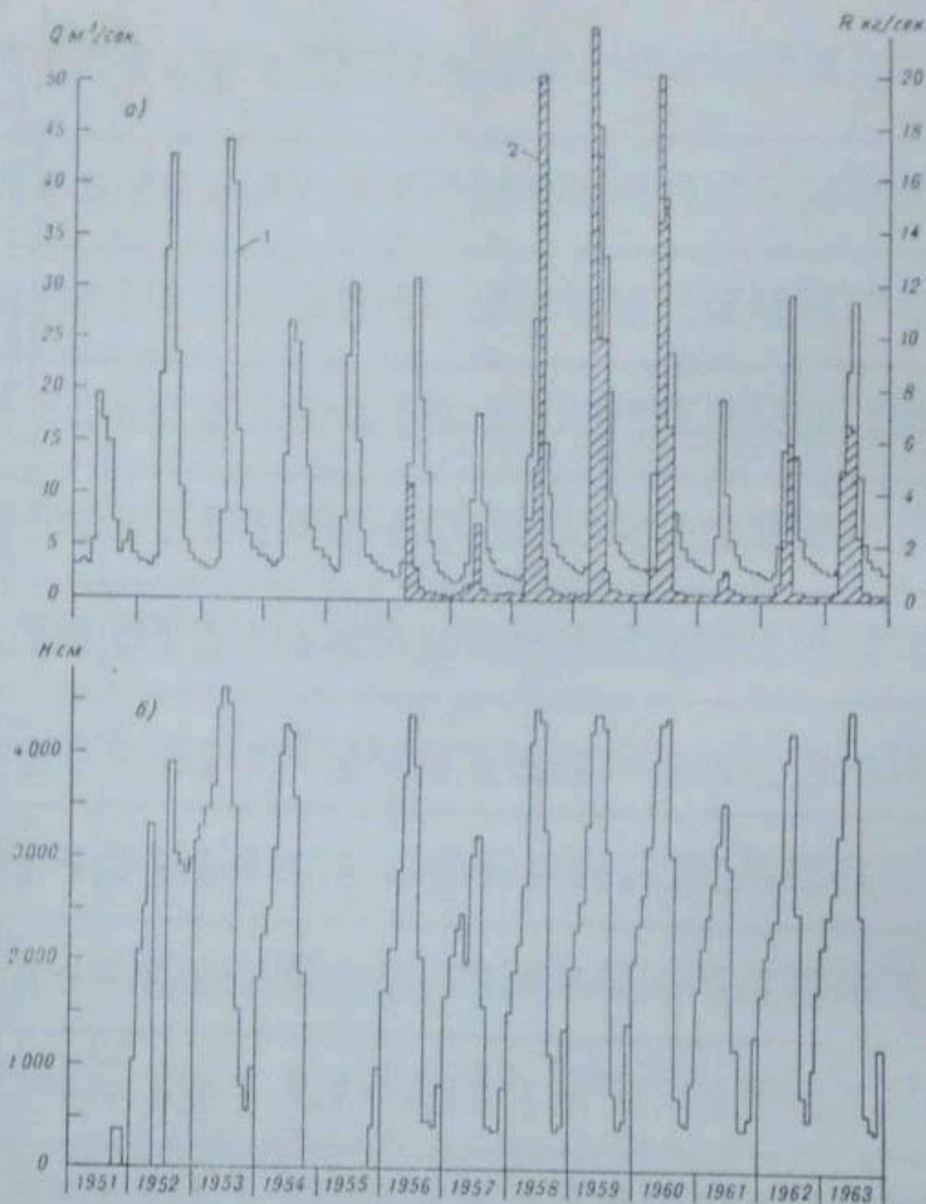
Рис. 1. а — хронологический график среднемесячных расходов воды (1), взвешенных наносов (2) р. Кассансай при впадении в Урта-токайское водохранилище; б — хронологический график среднемесячных уровней водохранилища.
