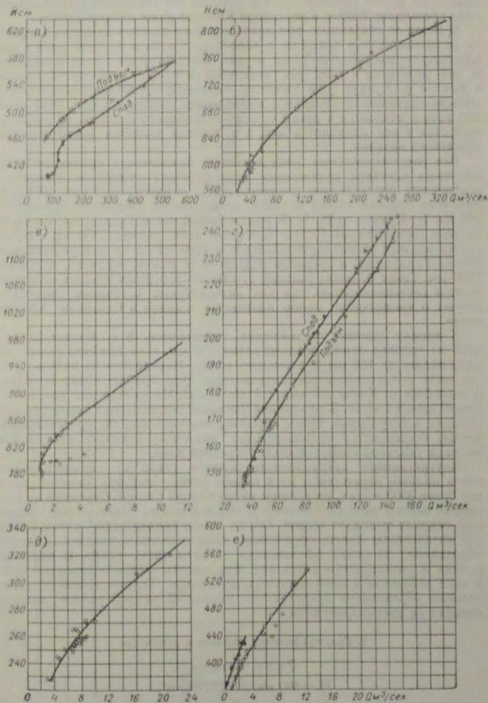
Рис. 2. Кривые Q \rightarrow I(H) рек Северного Афганистана за 1964—1965 гг.
