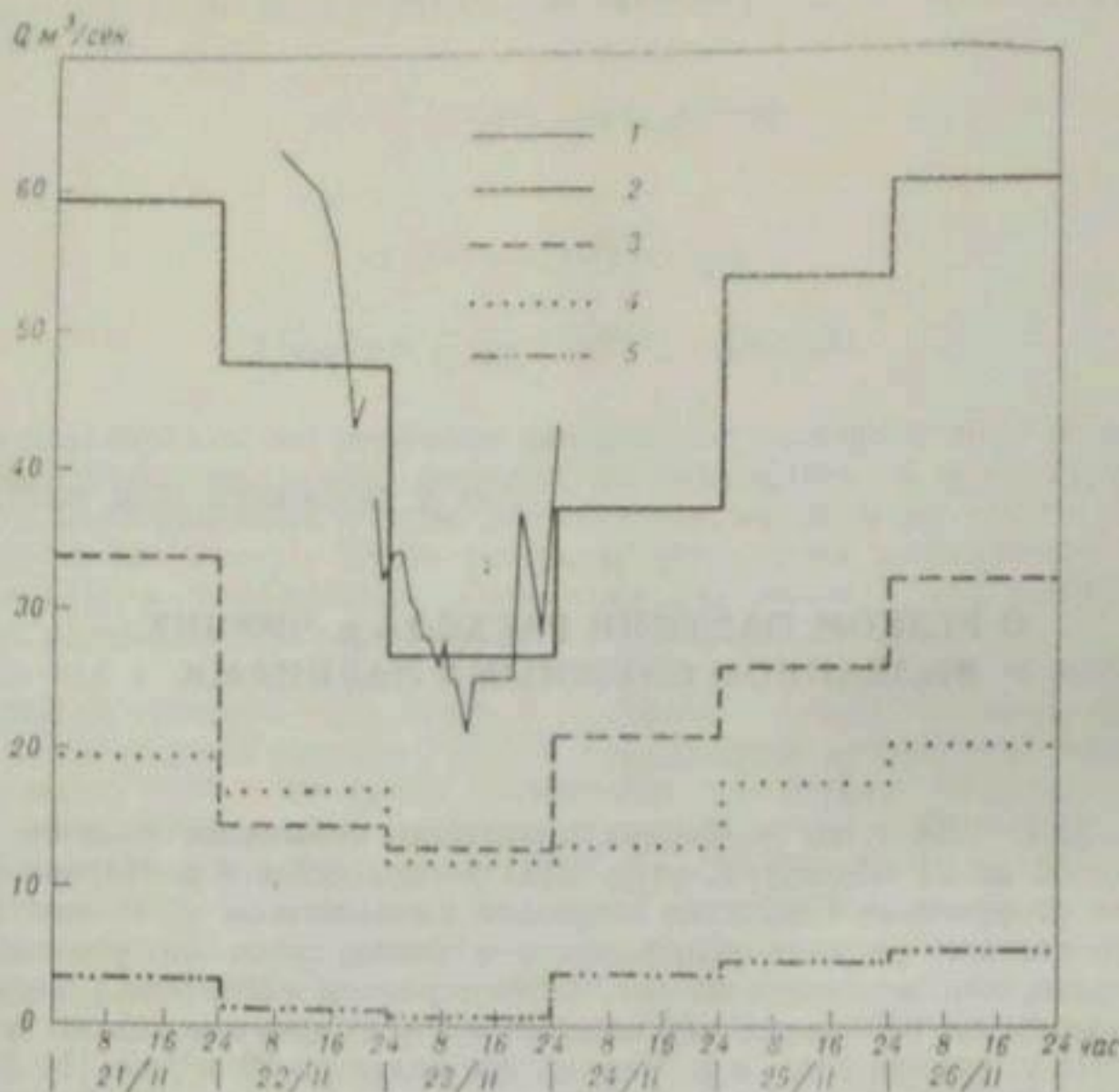
Рис. 1. Ежедневные и часовые расходы воды в реках Чирчик на головном сооружении ГЭС (1) и посту Ходжикент (2), Чаткал (3), Пскем (4) и Ойганг (5) 21—26/II 1956 г.
