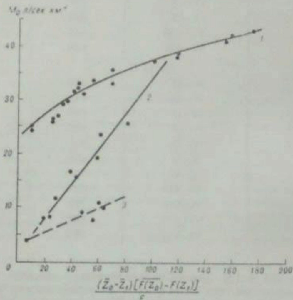
Рис. 2. Зависимость модуля стока от интегрального параметра водоподдачи j .
