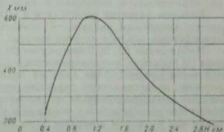
Рис. 1. Распределение годовых сумм жидких осадков на хр. Коржантау в зависимости от высоты (по З. А. Листровой).
