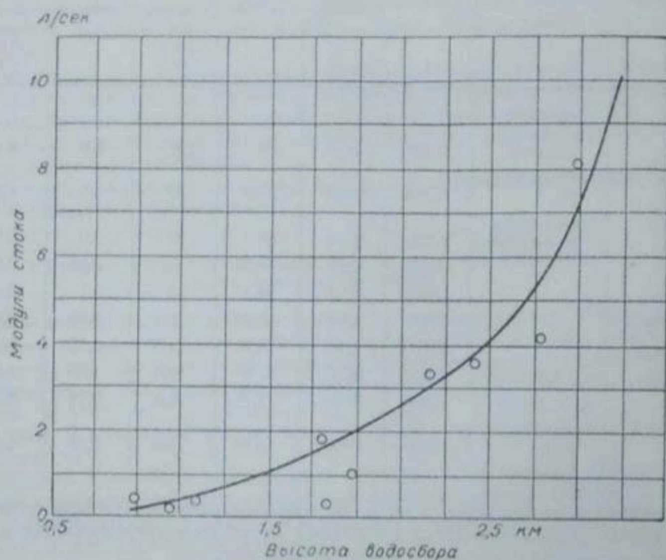
Рис. 5. Зависимость модулей стока рек Северного Афганистана от средних взвешенных высот водосборов.
