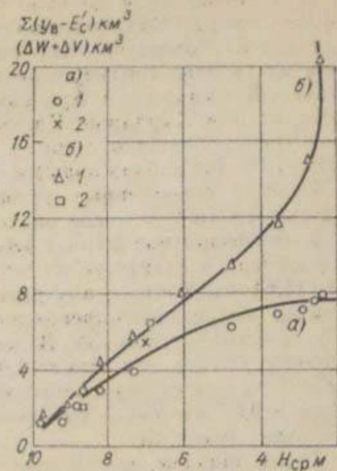
Рис. 4. Зависимость емкости почво-грунтов от уровня залегания грунтовых вод (а) и положения УГВ от разности водозабора и испарения (б). 1 — значения для новой зоны орошения, 2 — значения для старой зоны орошения.
