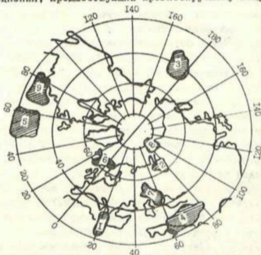
Области значимых значений коэффициентов корреляции (заштрихованы) между стоком р.Зеравшан и приземным давлением (1 – 3, 5 – 7) и температурой (4, 8, 9)
