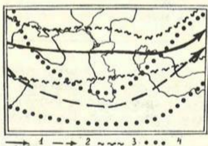
Рис. I. Среднее положение оси ПВФЗ (изогипсы 552 гПа) в марте 1969 г. (I) и 1983 г. (2) и границы его изменения внутри месяца (3, 4 - соответственно)
