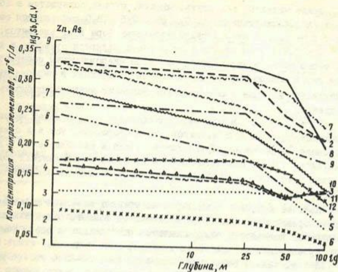
Рис. 1. Распределение микроэлементного состава прибрежных зон оз. Иссык-Куль:
