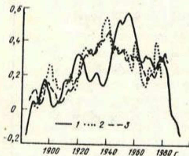
Рис.4. График осредненных по пятилеткам климатических изменений средней температуры поверхности Земли, рассчитанных по предложенной модели (1), Е.П.Борисенковым и В.Н.Приемовым (2) и полученные К.Я.Вяниковым, Г.В.Грузой и др. (3)
