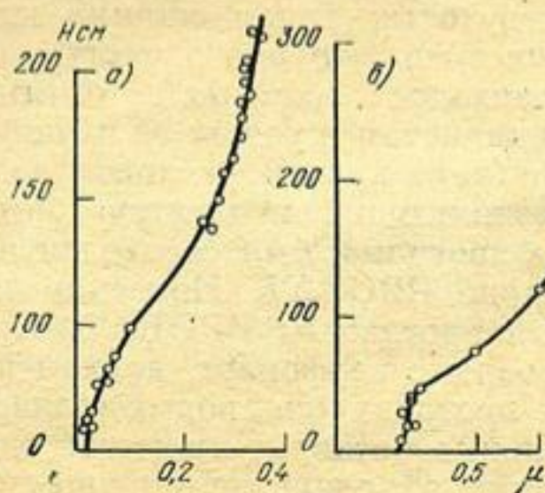
Зависимость параметра \mu от уровня воды для пунктов р. Сясь — д. Яхново (а) и р. Шалица — д. Никитинская (б) за 1959 г.
