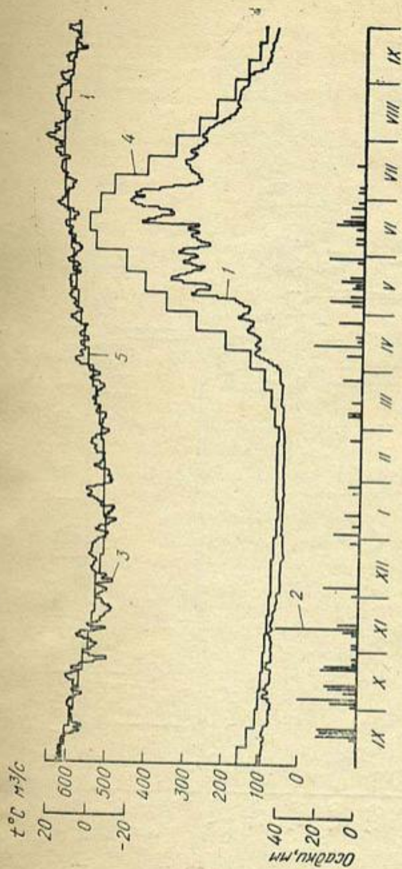
Рис. 1. Совмещенный график среднесуточных расходов притока воды в Чарвакское водохранилище (1), суточных сумм осадков по ГМС Пскем (2), температуры воздуха по ГМС Ангрен (3) за IX 1982—1983 гг., многолетних средних декадных расходов притока воды (4) и многолетних средних декадных температур воздуха (5)
