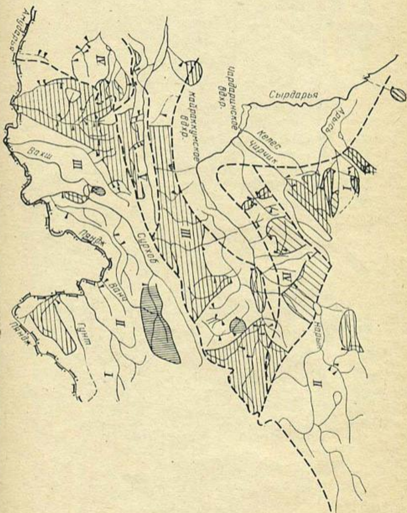
Рис. 3. Районирование территории Средней Азии (бассейны малых рек) по среднегодовому количеству осадков ( O_2 ):
