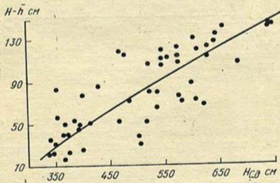
Рис. 3. Зависимость средних отметок дна р. Келес (пост Устье) от уровня воды в р. Сырдарья ( H_{c.a} )
