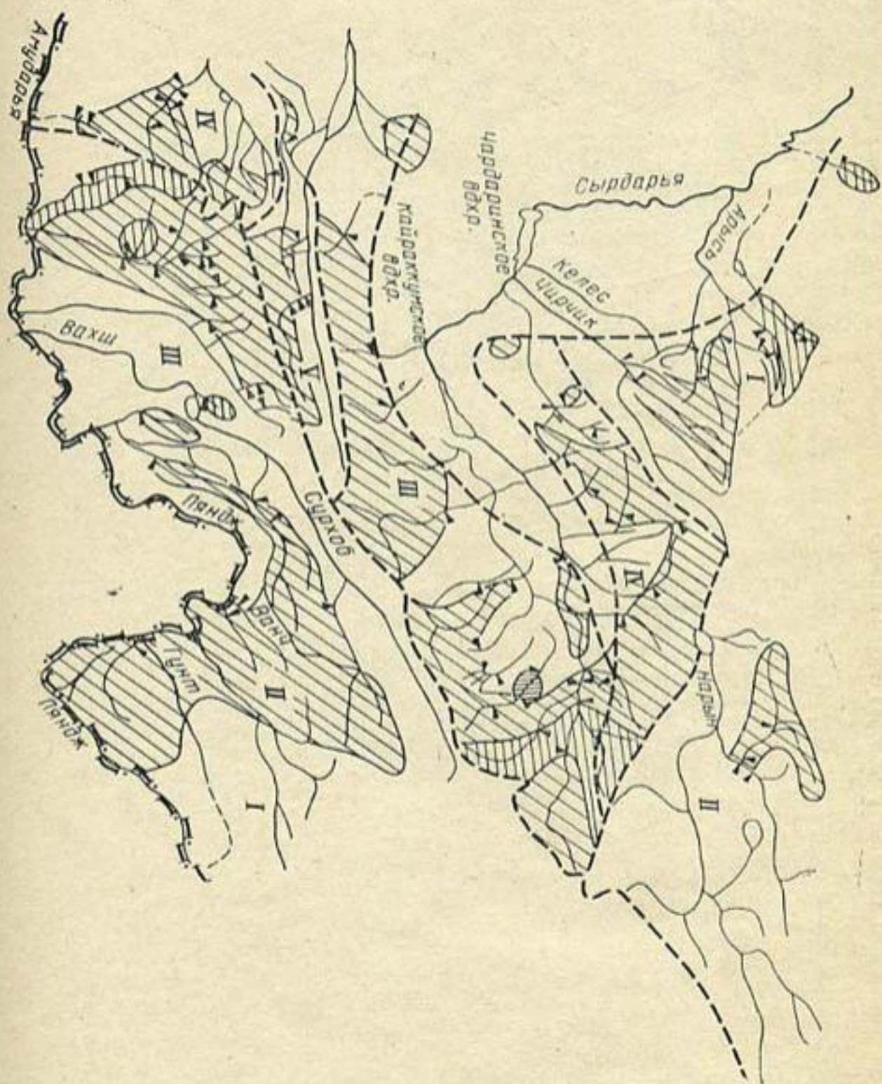
Рис. 5. Районирование территории Средней Азии (бассейны малых рек) по среднегодовому показателю — биохимической окисляемости:
