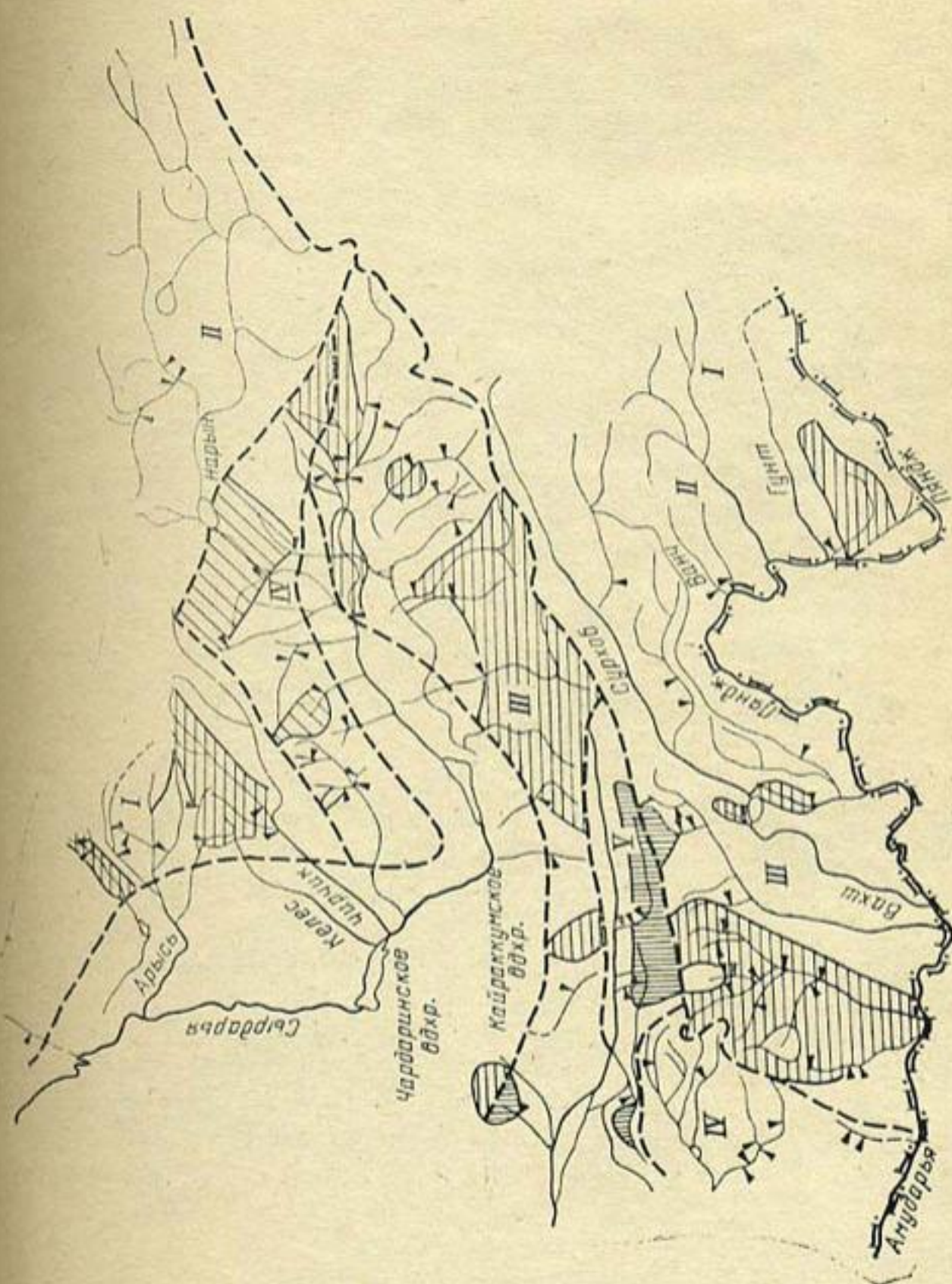
Рис. 4. Районирование территории Средней Азии (бассейны малых рек) по среднегодовому показателю БПК 5 :
