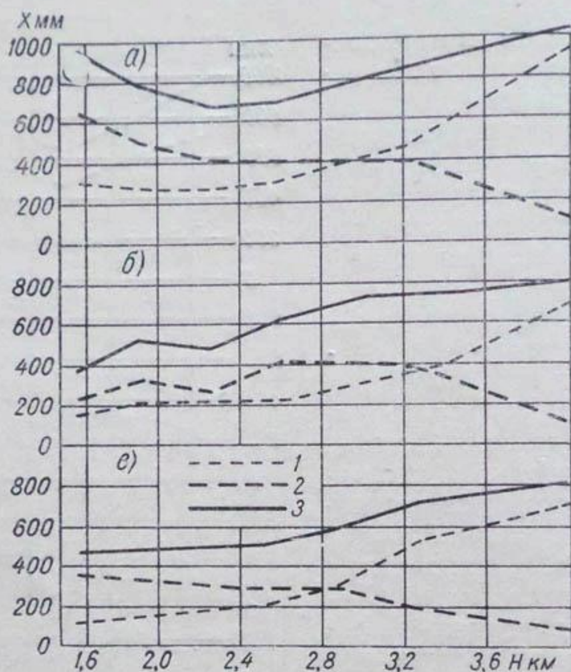
Рис. 24. Распределение зимних (1), летних (2) и суммарных годовых (3) осадков по высотному простиранью бассейна за 1957-58 (а), 1958-59 (б), 1959-60 (в) гг. в рамках естественных осадковых циклов.
