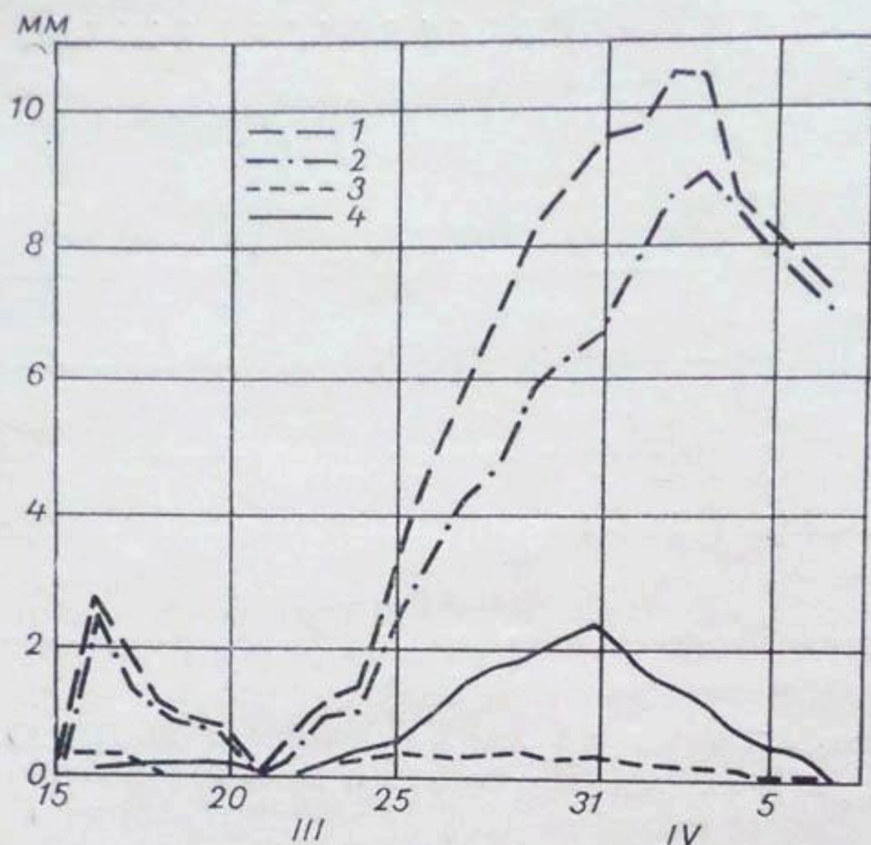
Рис. 28. Изменение составляющих водного баланса в период снеготаяния на стоковой площадке (бассейн р. Чонкызылсу) 1961 г.
