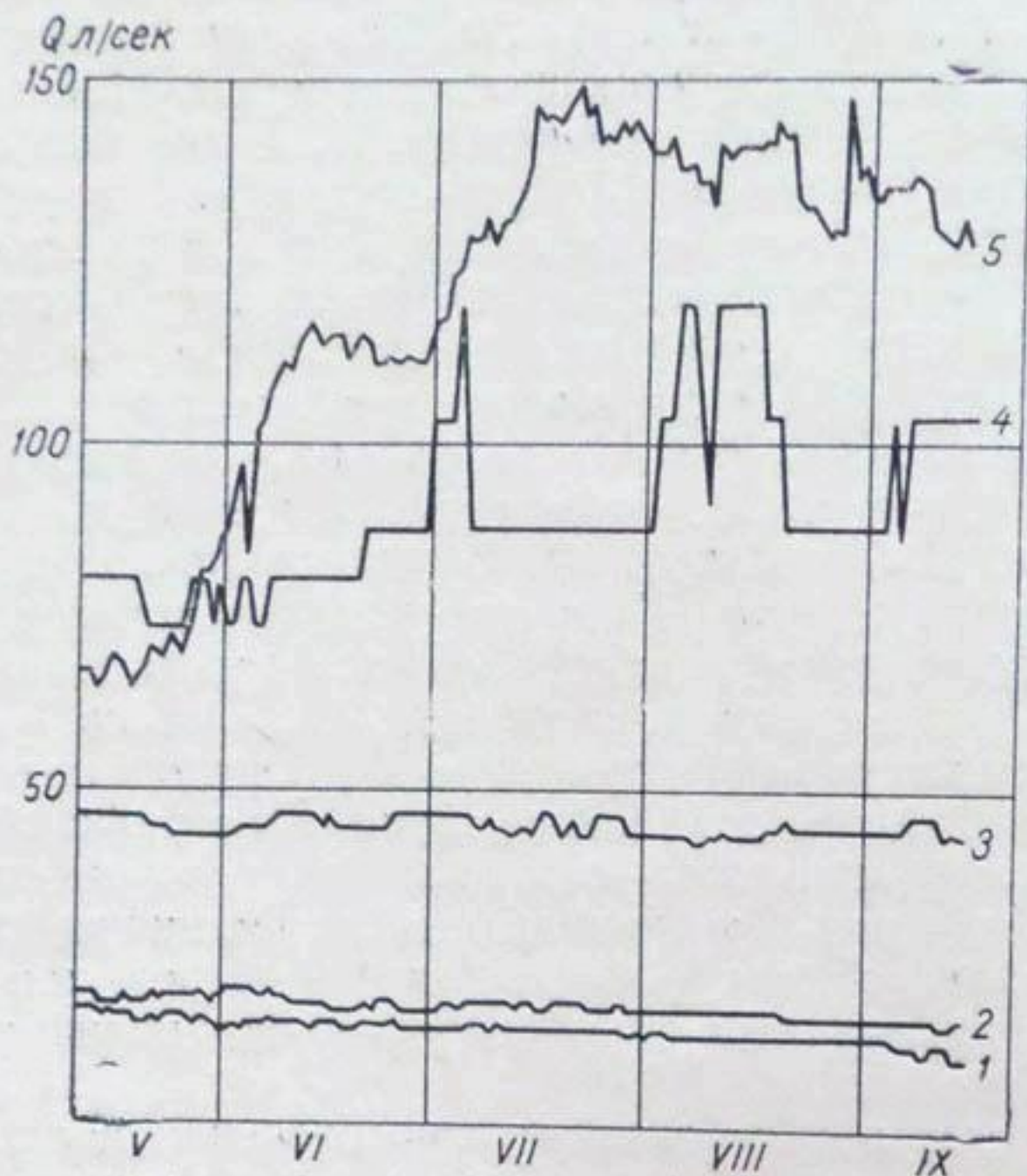
Рис. 17. Гидрографы некоторых источников подземного питания в Алаарчинском бассейне, 1959 г.
