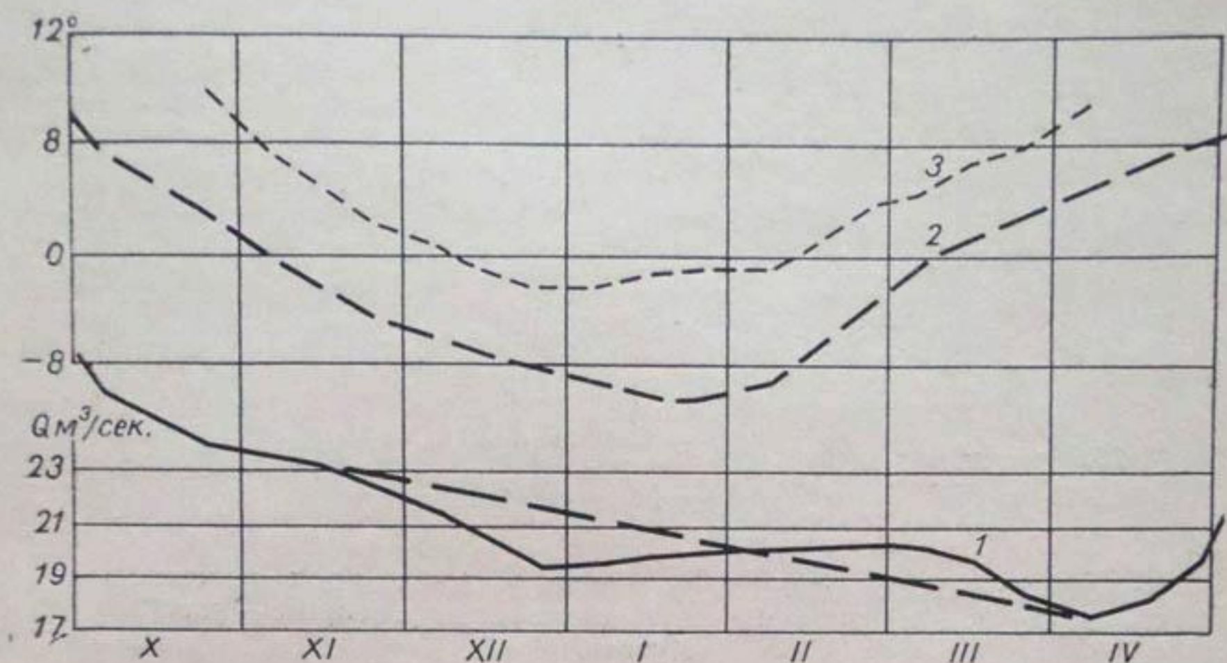
Рис. 45. Многолетний ход температуры воздуха по средним суточным (2) и 13-часовым (3) данным и расходов воды р. Чу (1) по метеостанции и гидрологическому посту Кочкорка.
