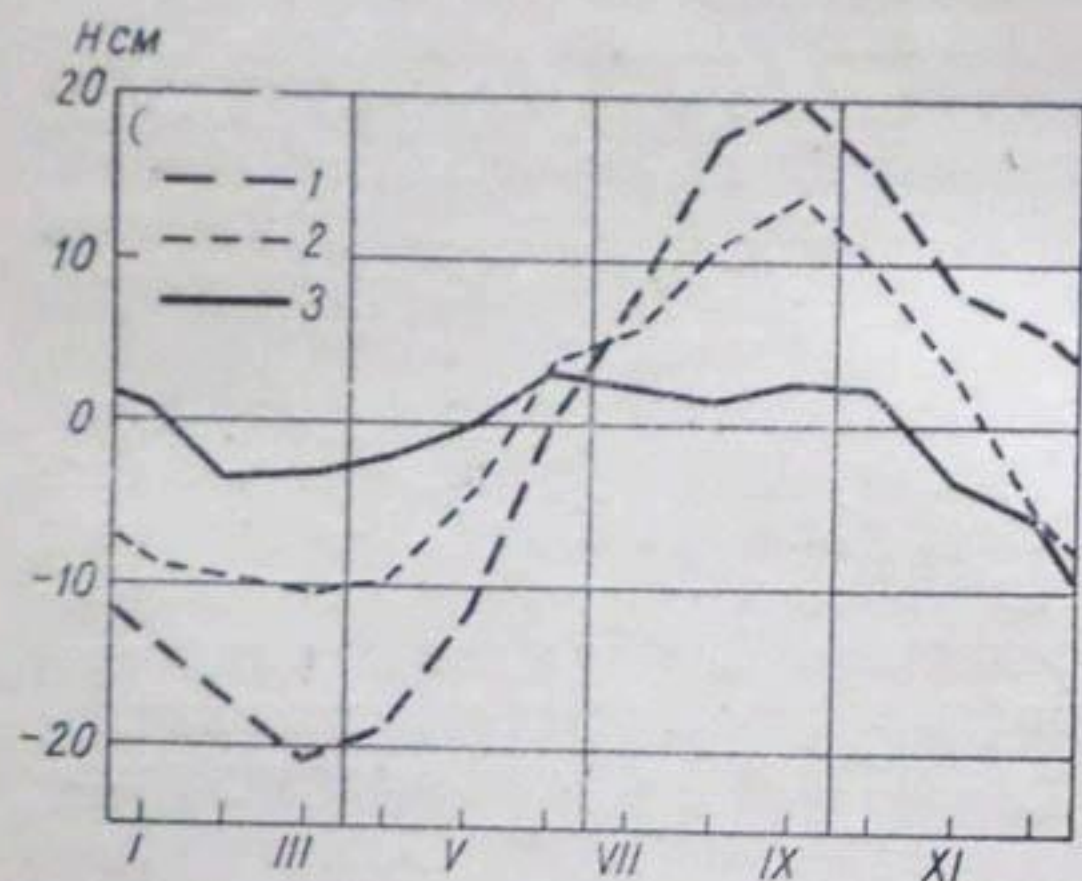
Рис. 5. Сезонные колебания уровня воды оз. Иссык-Куль.
