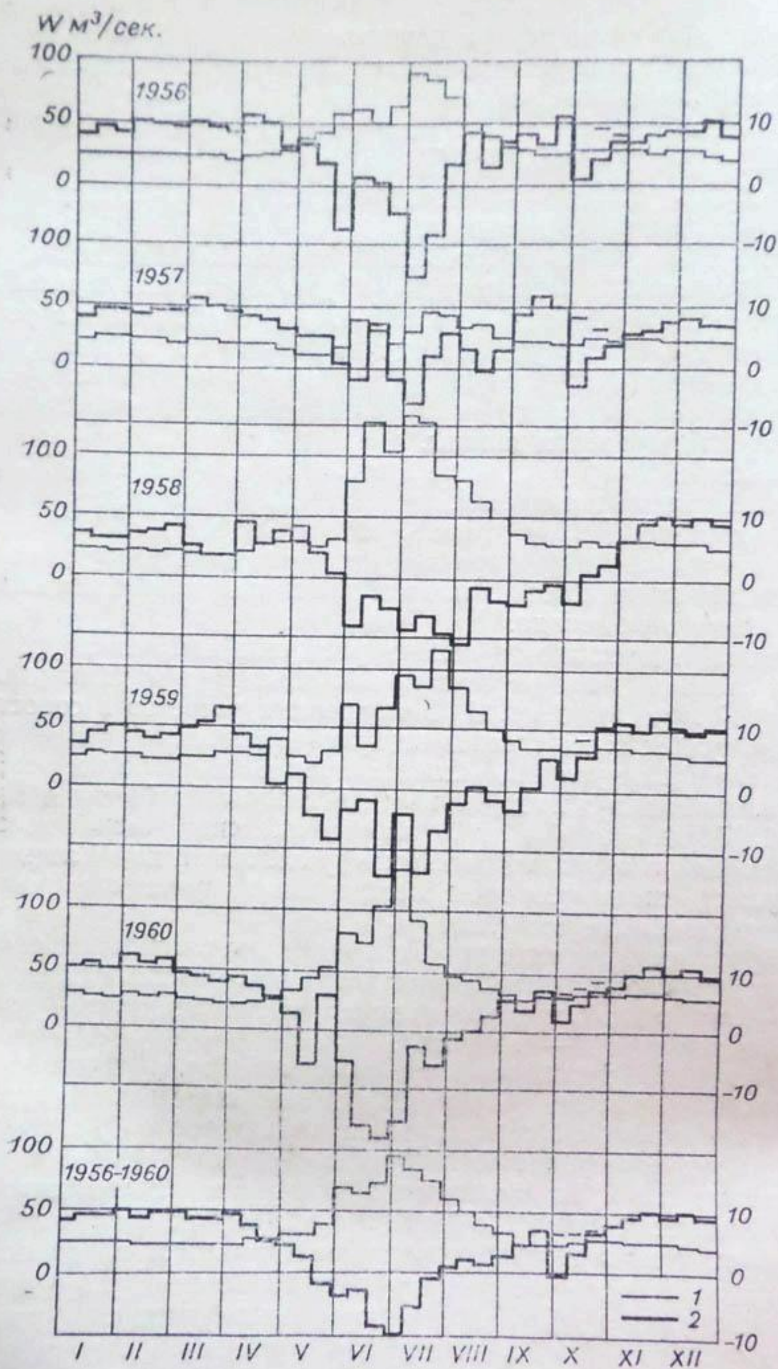
Рис. 33. Календарный ход руслового стока (пост Кировское) (1) и его изменения в долине (2).
