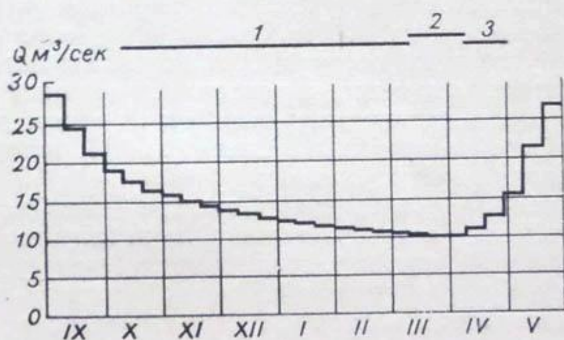
Рис. 43. Расходы меженного периода, р. Исфайрам — пост Уч-Коргон (1936—1960 гг.).
