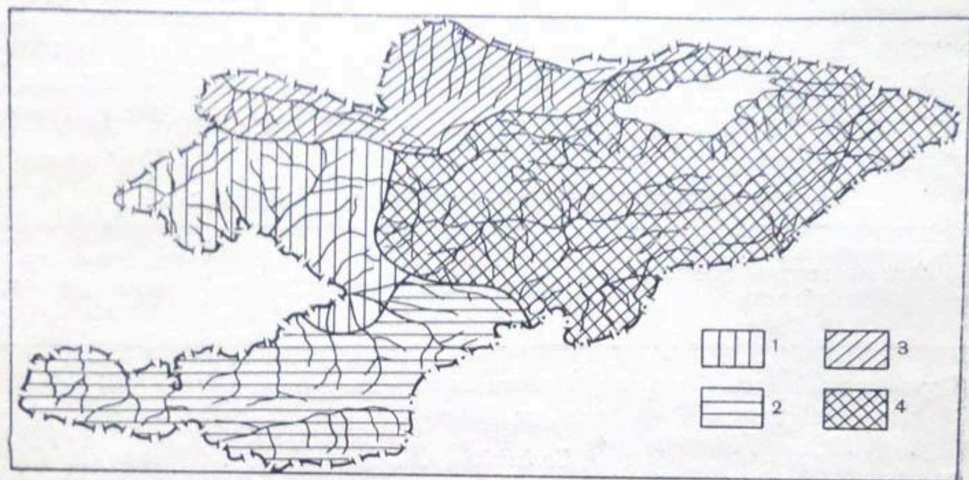
Рис. 3. Доля осадков теплого периода (апрель — октябрь) в годовой сумме осадков.
