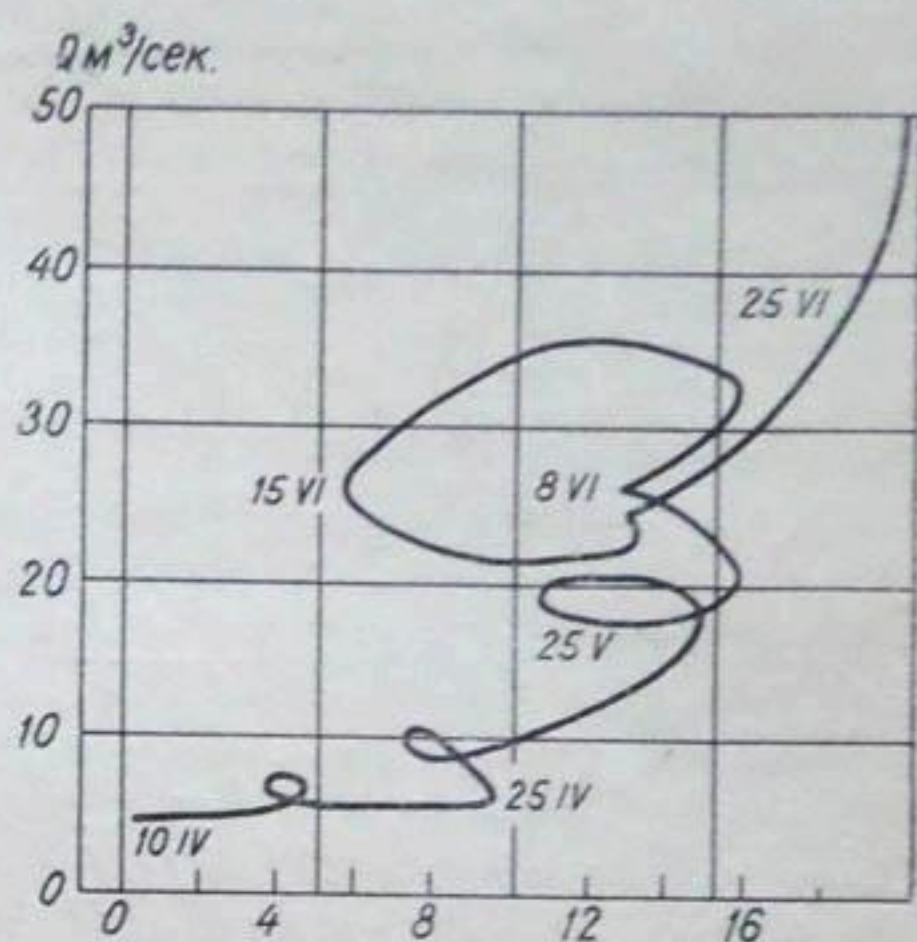
Рис. 15. Зависимость расходов р. Исфара (Таш-Курган) за апрель — июнь 1941 г. от тринадцатичасовой температуры воздуха по ст. Сары-Таш для скользящих пентад.
