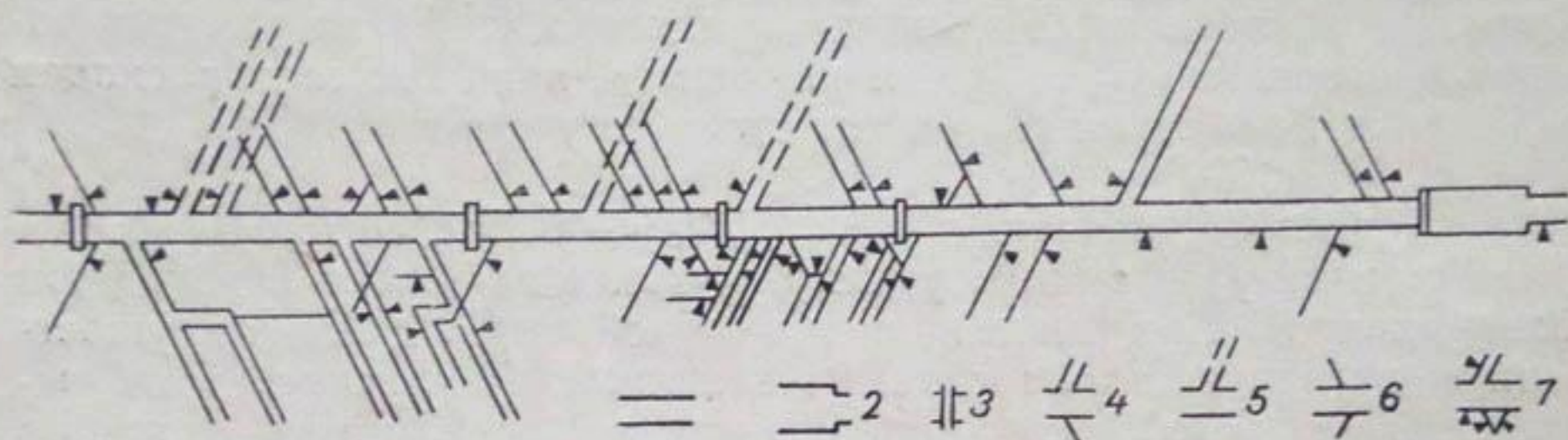
Рис. 30. Линейная балансовая схема р. Чу.
