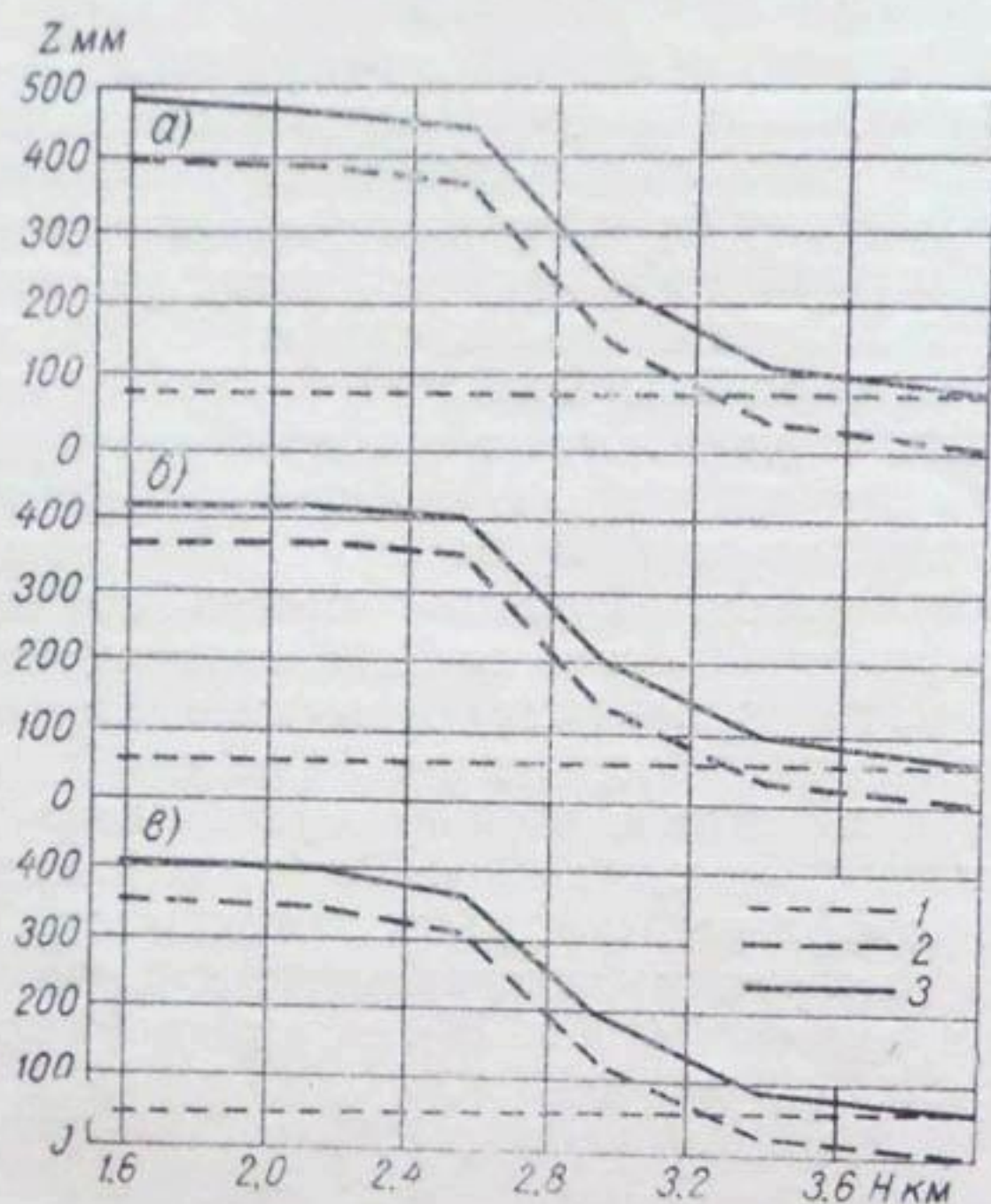
Рис. 25. Распределение зимнего (1), суммарного летнего (2) и общего годового (3) испарения по высотным зонам бассейна за 1957-58 (а), 1958-59 (б) и 1959-60 (в) гг. в рамках естественных осадково-испарительных циклов.
