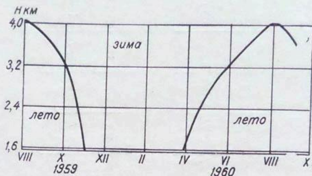
Рис. 21. Границы осадкового года и полугодий в бассейне (1959-60 г.).
