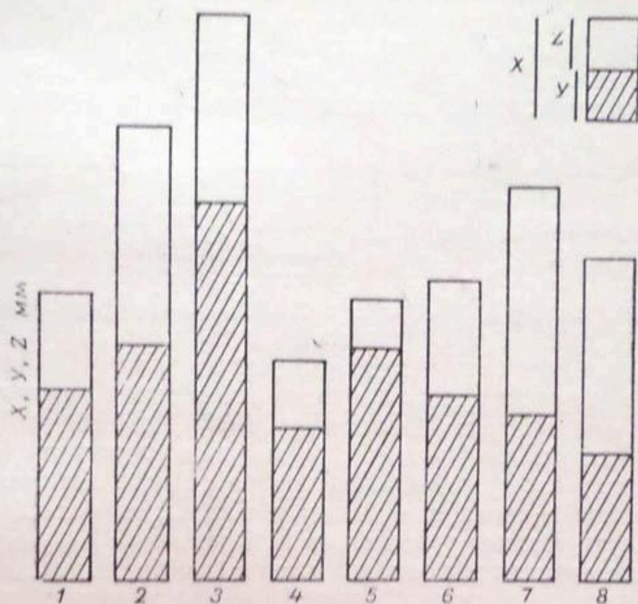
Рис. 40. Составляющие водного баланса гидрографических бассейнов (осадки X , сток Y и испарение Z ).
