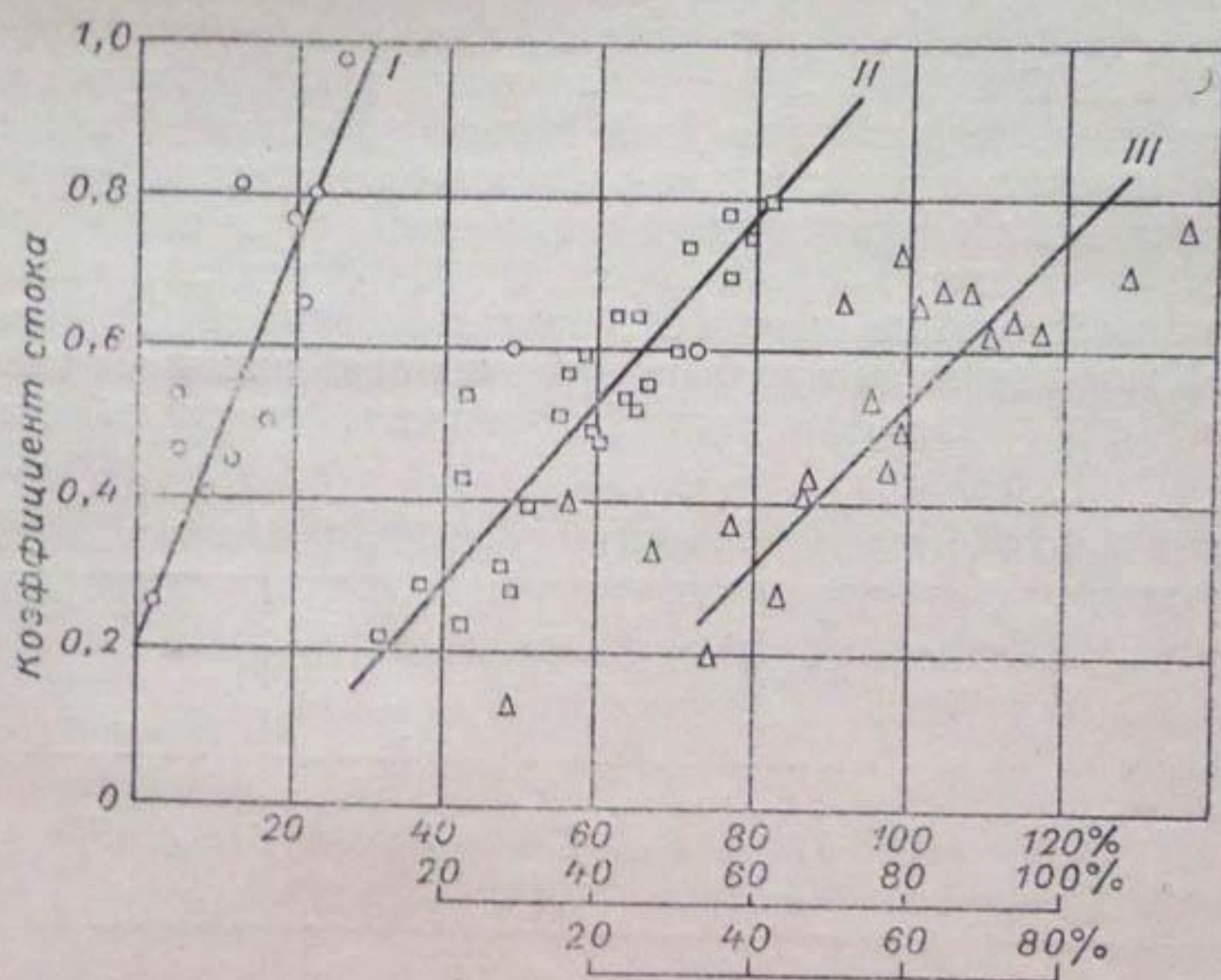
Рис. 39. Зависимость коэффициента стока от площади бассейна, занятой лесами, кустарниками, обнажениями скал, осыпями и ледниками в процентах от всей площади водосбора (по И. А. Ильину).
