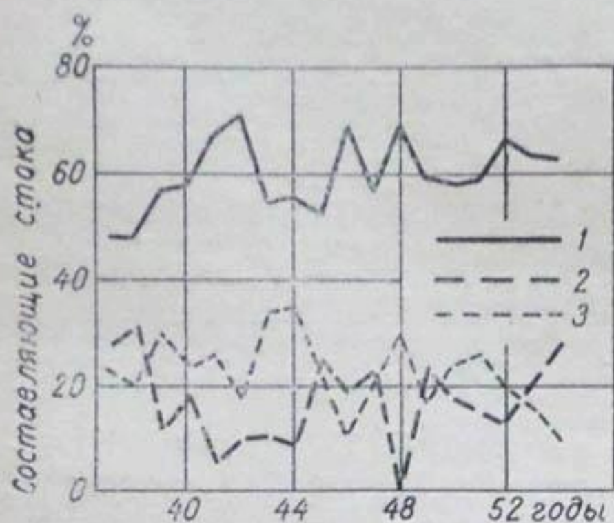
Рис. 12. Доля талых снеговых вод (1), талых вод зоны ледников и вечного снега (2) и жидких осадков (3) в годовом стоке р. Сокулук в процентах от общего стока.
