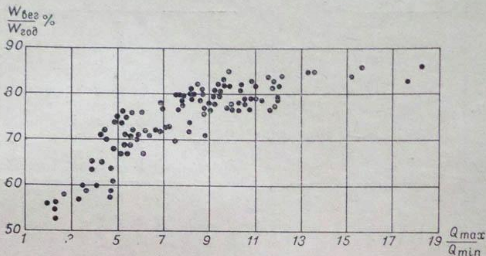
Рис. 49. Зависимость распределения стока между паводковым и меженным периодами от степени устойчивой грунтовой зарегулированности стока.
