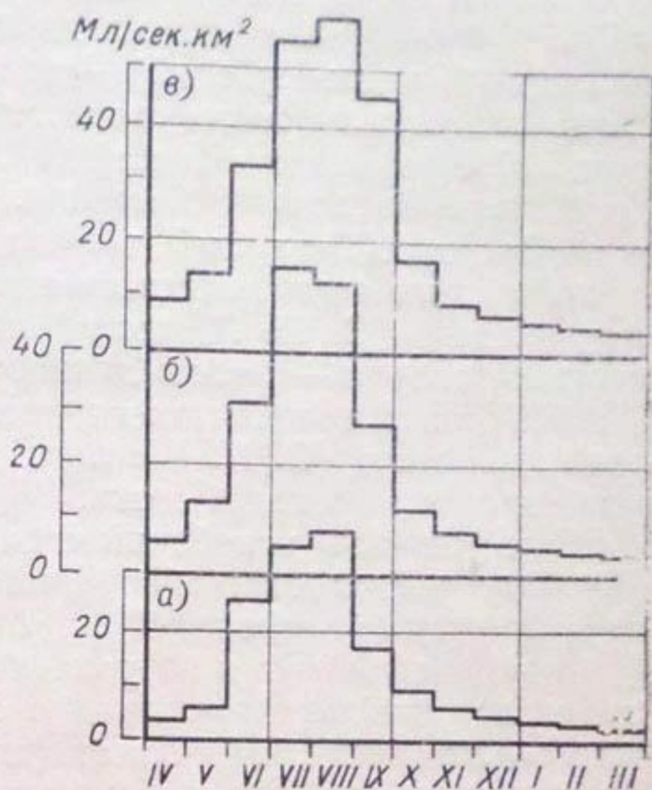
Рис. 61. Гидрографы стока р. Сох (кишл. Сары-Канда) за маловодный (а; 1957-58 г.), средний (б; 1911, 1913—1915, 1926—1950 гг.) и многоводный (в; 1959-60 г.) годы (в модулях стока).
