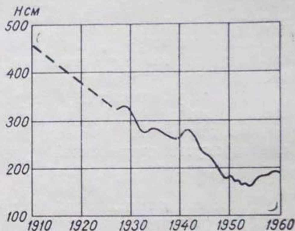
Рис. 6. Многолетние колебания уровня воды оз. Иссык-Куль.
