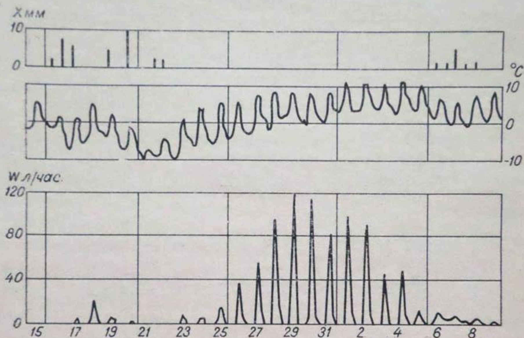
Рис. 27. Сток и метеорологические элементы на площадке на склоне восточной ориентации (бассейн р. Чонкызылсу).
