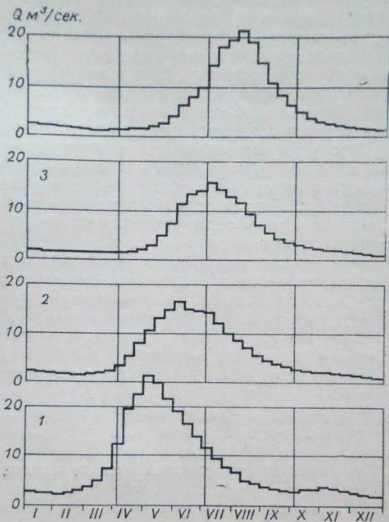
Рис. 41. Гидрографы средних многолетних расходов воды (1936—1960 гг.) рек снегово-дождевого (1—Майлису), снегового (2—Падшаата), снегово-ледникового (3—Карабалты) и ледникового (4—Джуука) питания.
