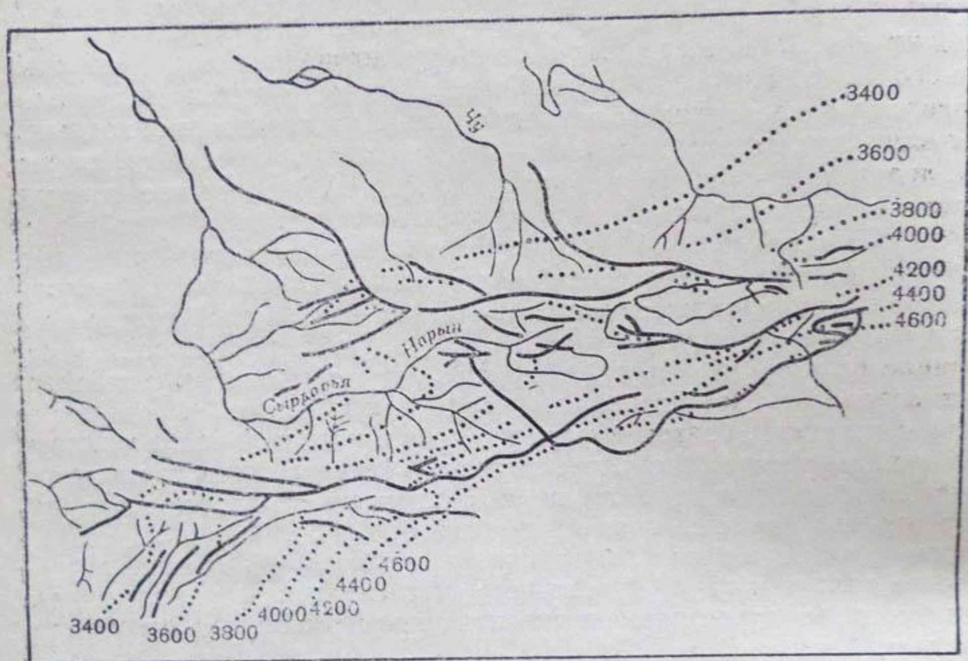
Рис. 4. Высотное положение снеговой линии.
