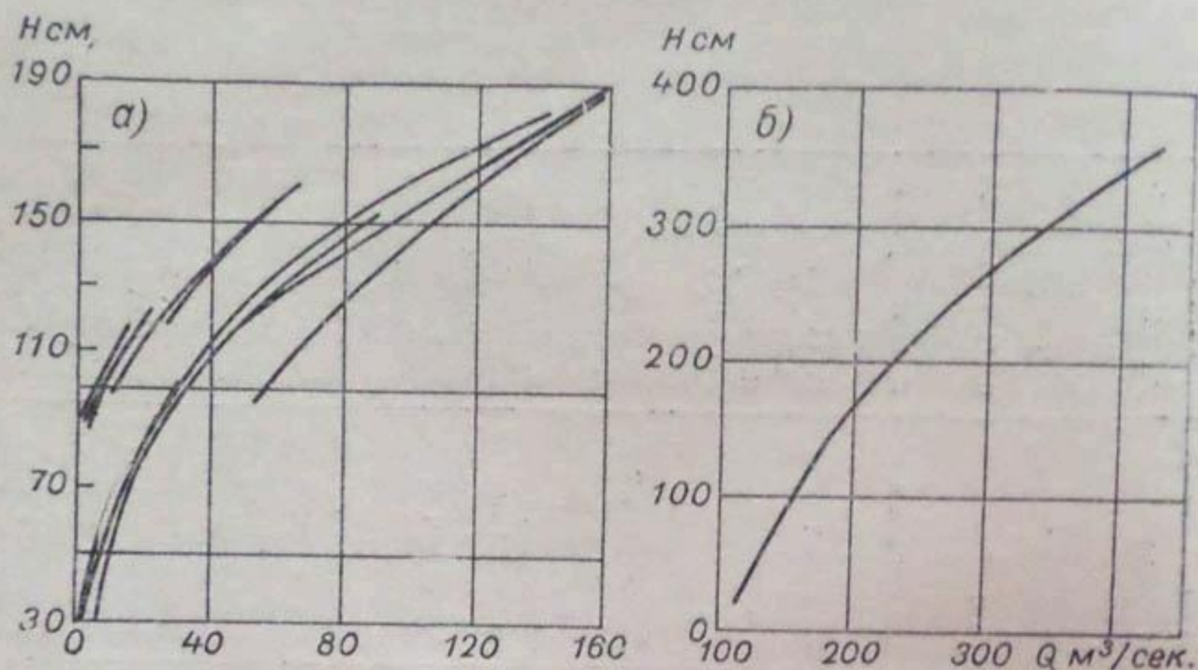
Рис. 47. Кривые связи уровней с расходами воды (1963—1964 гг.) как показатели степени устойчивости русел.
