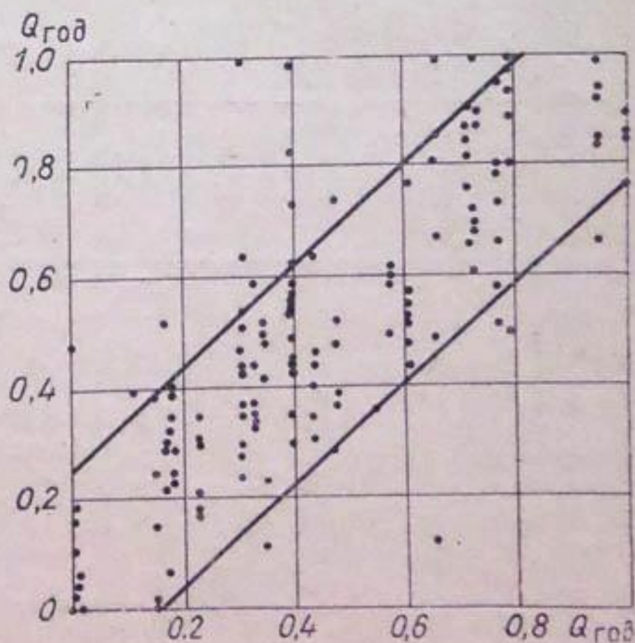
Рис. 57. График синхронности колебаний годового стока рек Южно-Ферганского гидрологического района.
