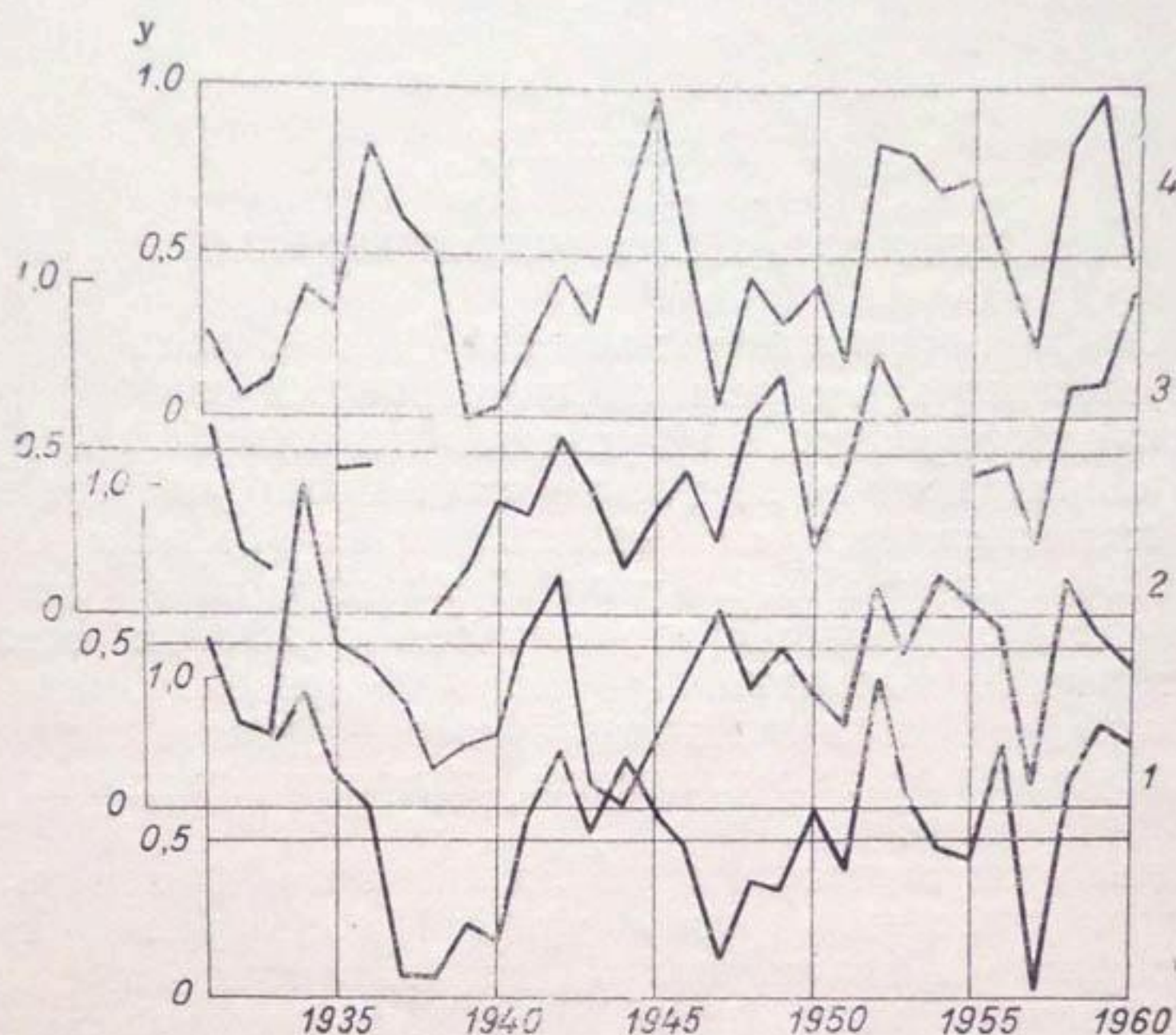
Рис. 55. Хронологический ход годового стока ряда рек. 1 — р. Нарын — г. Нарын, 2 — р. Талас — пост Чат-Базар, 3 — р. Тентяксай, 4 — р. Исфайрам. Сток выражен в относительных единицах.
