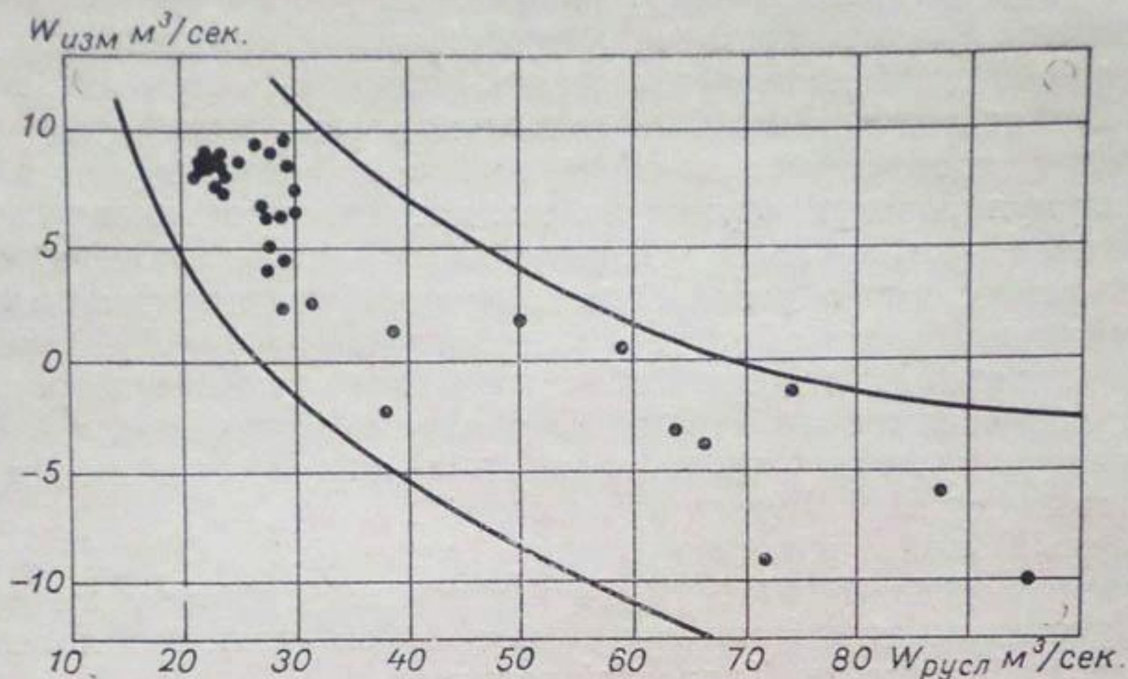
Рис. 35. Зависимость изменения руслового стока в долине от общих размеров руслового стока (пост Кировское) по средним декадным данным за 5 лет (1956—1960 гг.).
