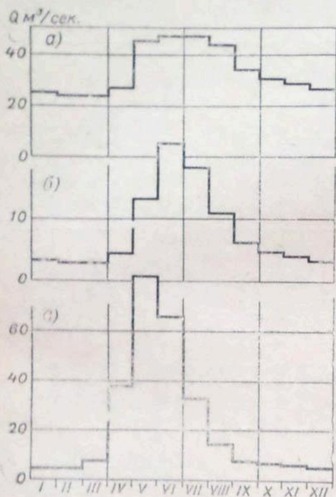
Рис. 48. Гидрографы среднего многолетнего стока рек различных степеней устойчивой зарегулированности: очень сильной (а) — р. Атбаши — п. Джангистал, средней (б) — р. Кекемерен — ниже устья Джумгол и очень слабой (в) — р. Яссы — п. Саламалик.
