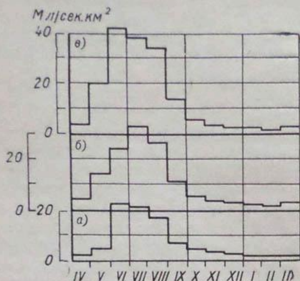
Рис. 58. Гидрографы стока р. Малого Нарына (устье) за маловодный (а; 1957-58 г.), средний (б; 1939 — 1960 гг.) и многоводный (в; 1942-43 г.) годы (в модулях стока).
