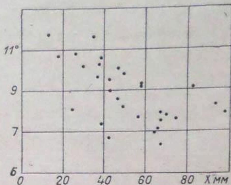
Рис. 53. Характер зависимости между летней температурой воздуха и осадками, август, метеостанция Тянь-Шань.
