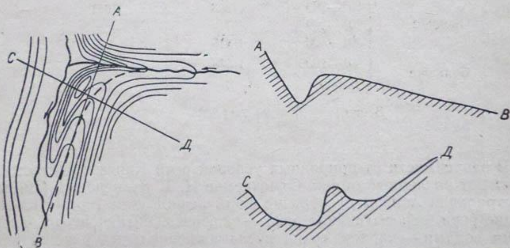
Рис. 7. Схема спрямления нижних течений притоков, параллельных основной реке, с образованием брошенных висячих долин.
