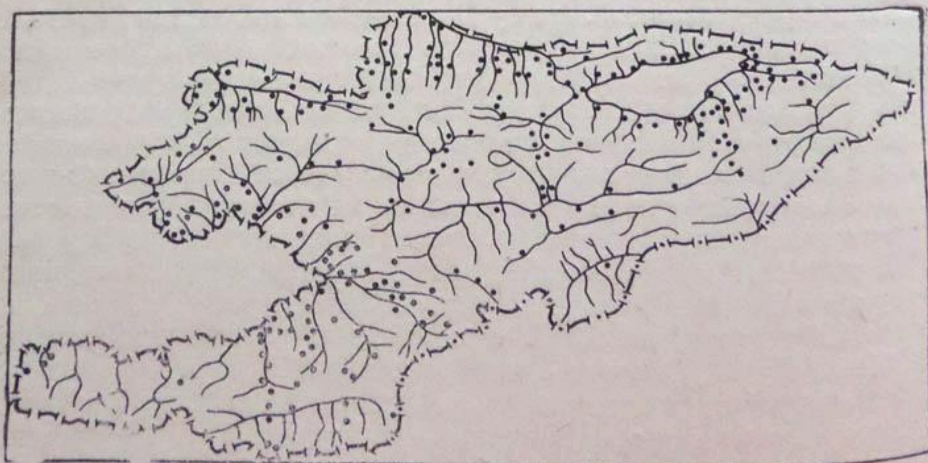
Рис. 10. Размещение метеорологической наблюдательной сети.
