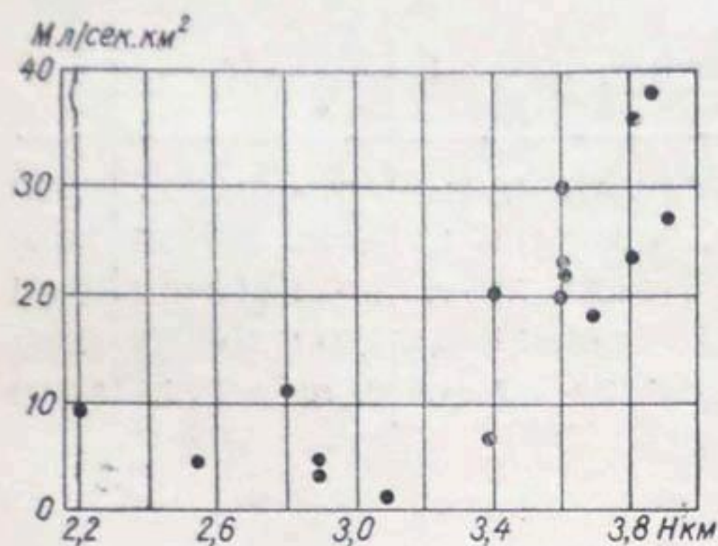
Рис. 20. Зависимость модулей стока за 1959-60 стоковый год от средневзвешенных высот бассейнов.
