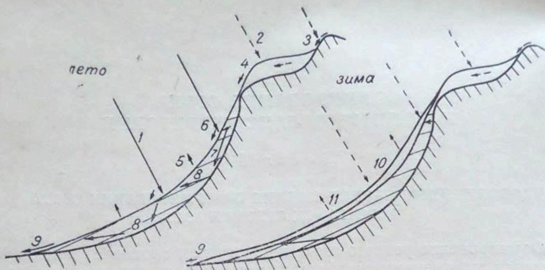
Рис. 11. Схема водного баланса горного бассейна в летний и зимний периоды.
