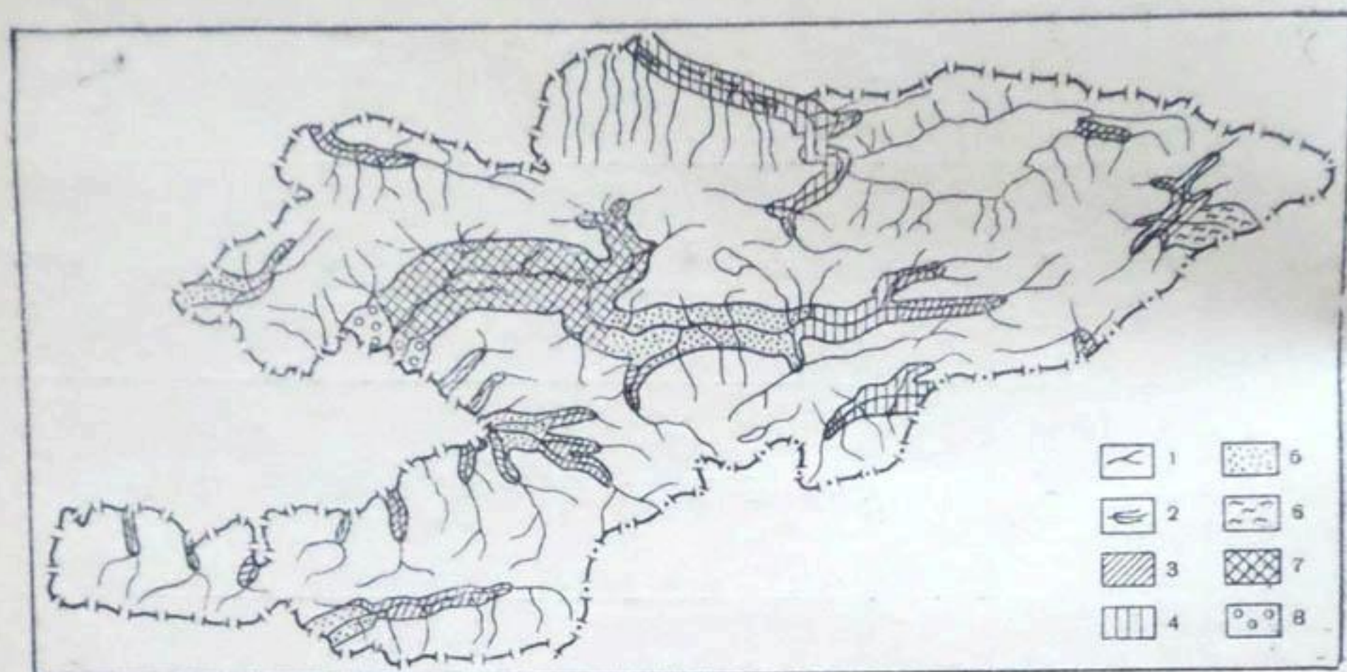
Рис. 37. Водоносность рек Киргизии. Средние расходы в м³/сек.: 1 — 10, 2 — 10—20, 3 — 20—50, 4 — 50—100, 5 — 100—200, 6 — 200—300, 7 — 300—400, 8 — 400.
