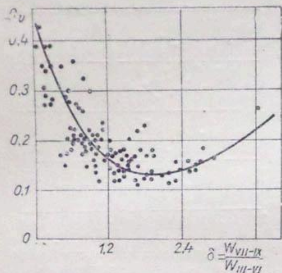
Рис. 54. Зависимость степени изменчивости годового стока рек ( C_v ) от типа питания ( \delta ).
