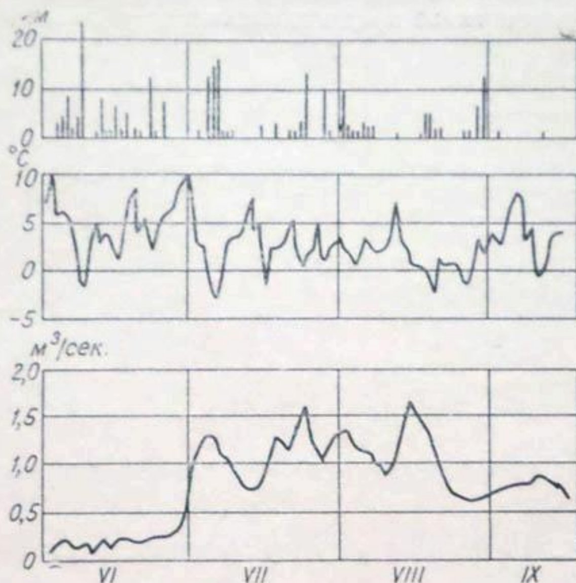
Рис. 18. Атмосферные осадки, температура воздуха в зонах таяния и расходы воды р. Адыгине (ниже устья р. Тезтор).
