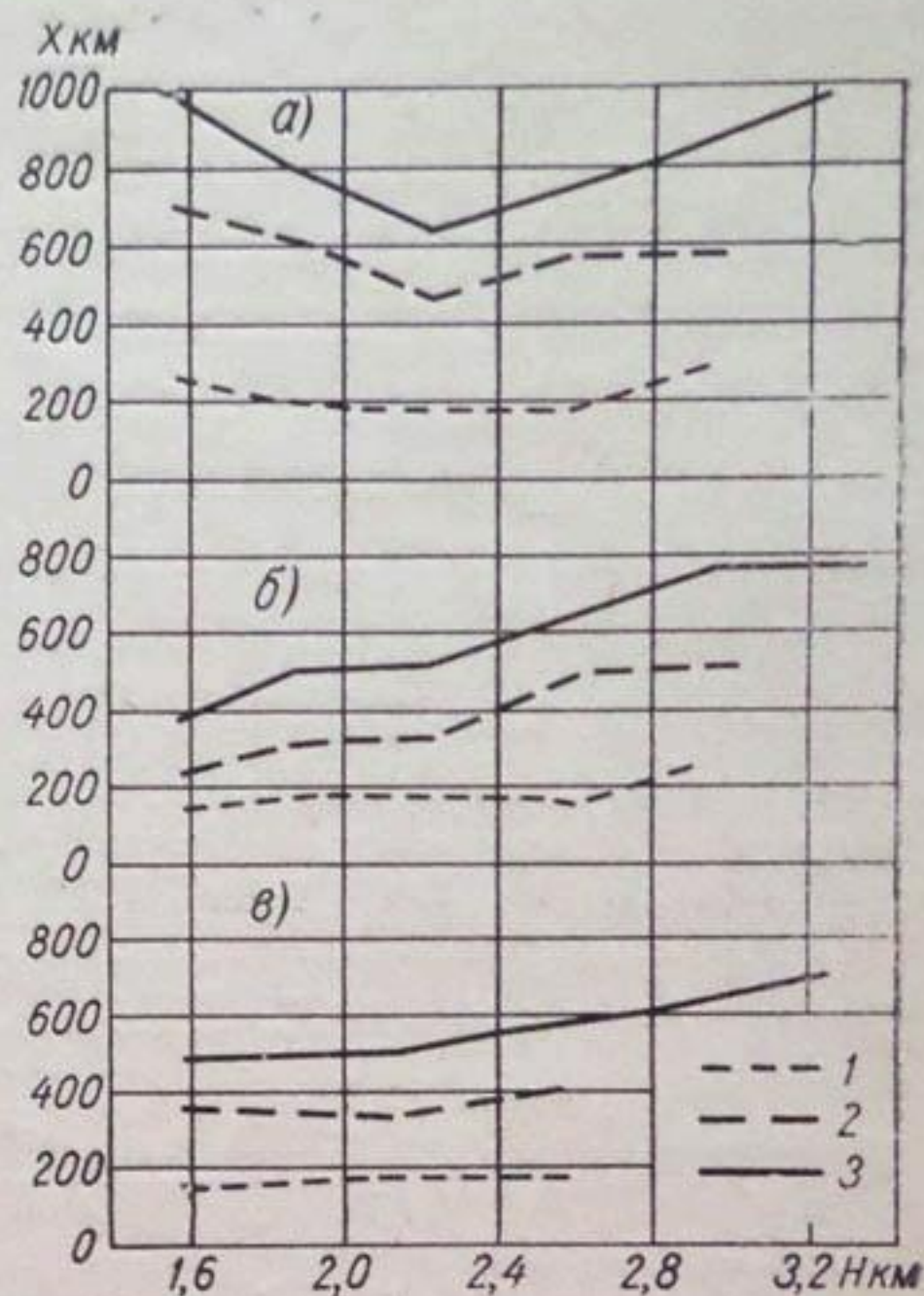
Рис. 23. Распределение зимних (1), летних (2) и суммарных годовых (3) осадков по высотным зонам бассейна за 1957-58 (а), 1958-59 (б) и 1959-60 (в) гг. в стандартных календарных рамках зимнего (октябрь — март) и летнего (апрель — сентябрь) полугодий и соответствующего им года (октябрь — сентябрь).
