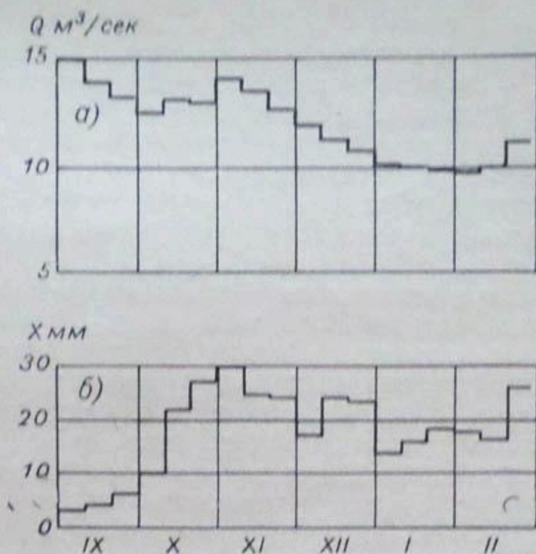
Рис. 44. Осенний паводок (а) и осенние осадки (б), р. Тентяксай — пост Чарвак.
