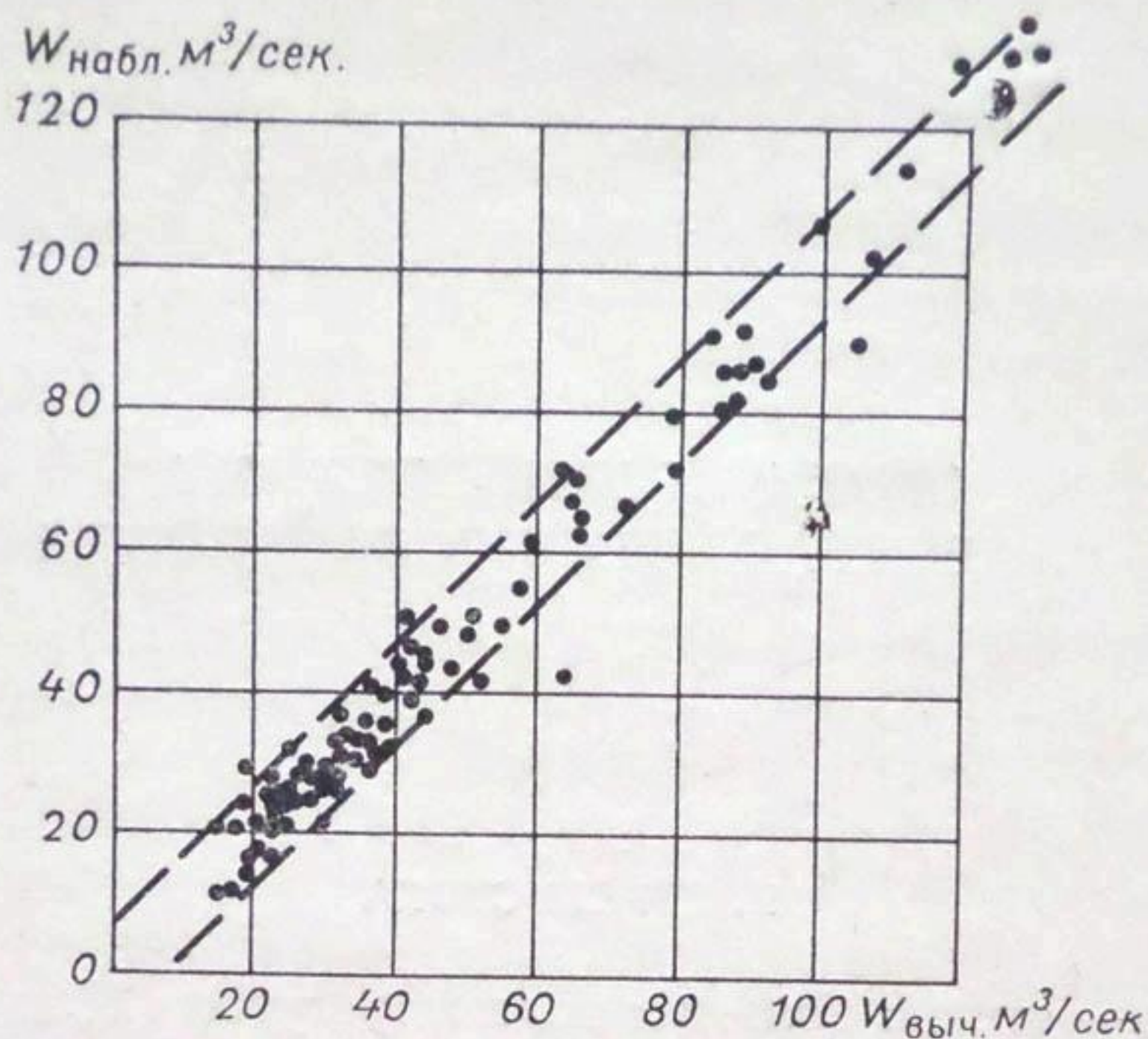
Рис. 36. Зависимость наблюдаемых и вычисленных по уравнению водного баланса значений декадного стока по посту Кировское за паводковый период 1956—1960 гг.
