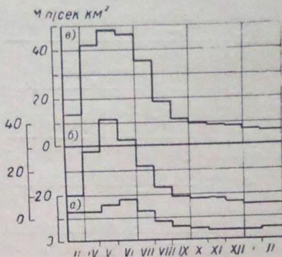
Рис. 59. Гидрографы стока р. Карасу правая (устье) за маловодный (а; 1957-58 г.), средний (б; 1937—1943, 1947—1960 гг.) и многоводный (в; 1958-59 г.) годы (в модулях стока).
