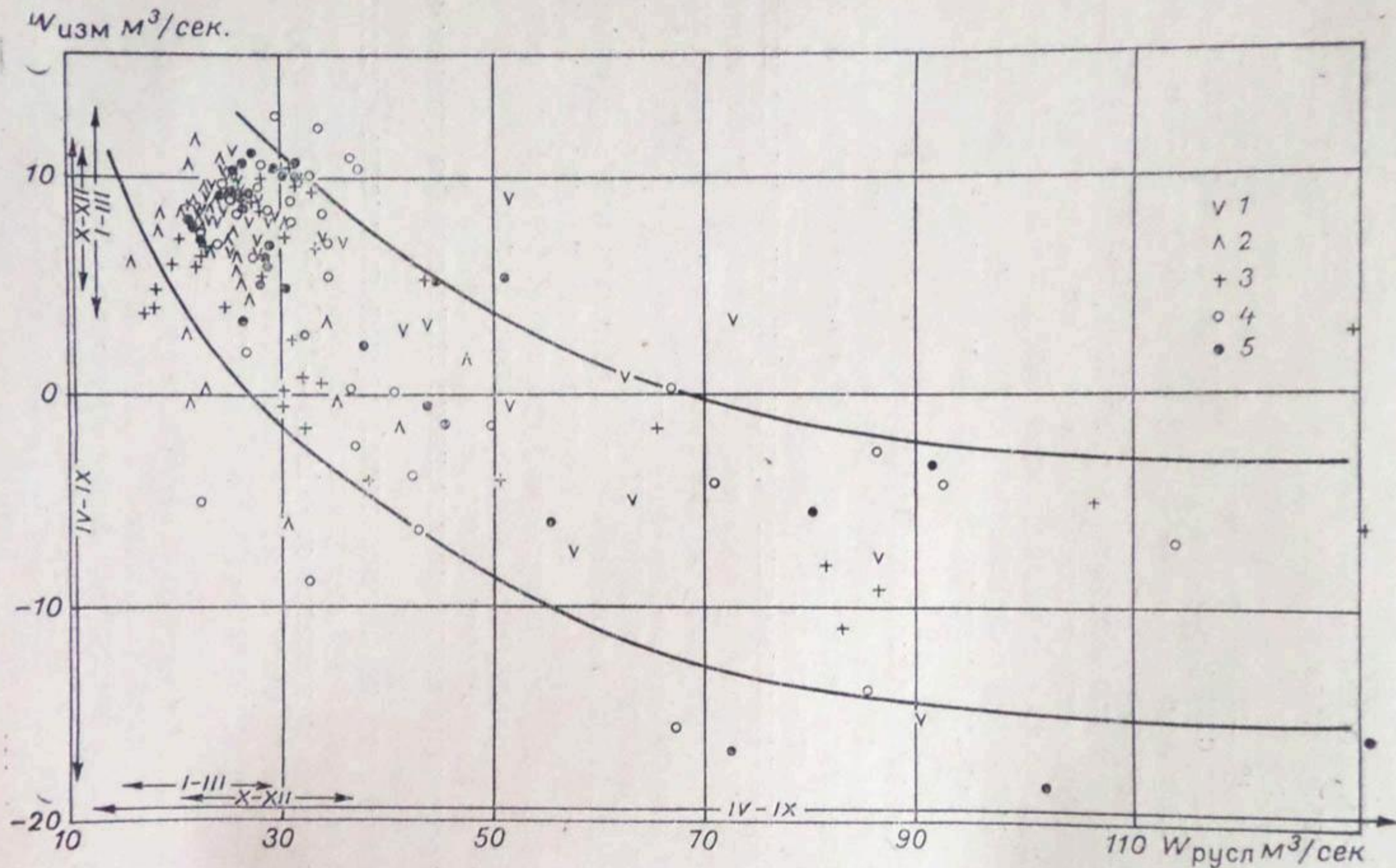
Рис. 34. Зависимость изменения декадного стока в долине от общих размеров руслового стока (пост Кировское).
