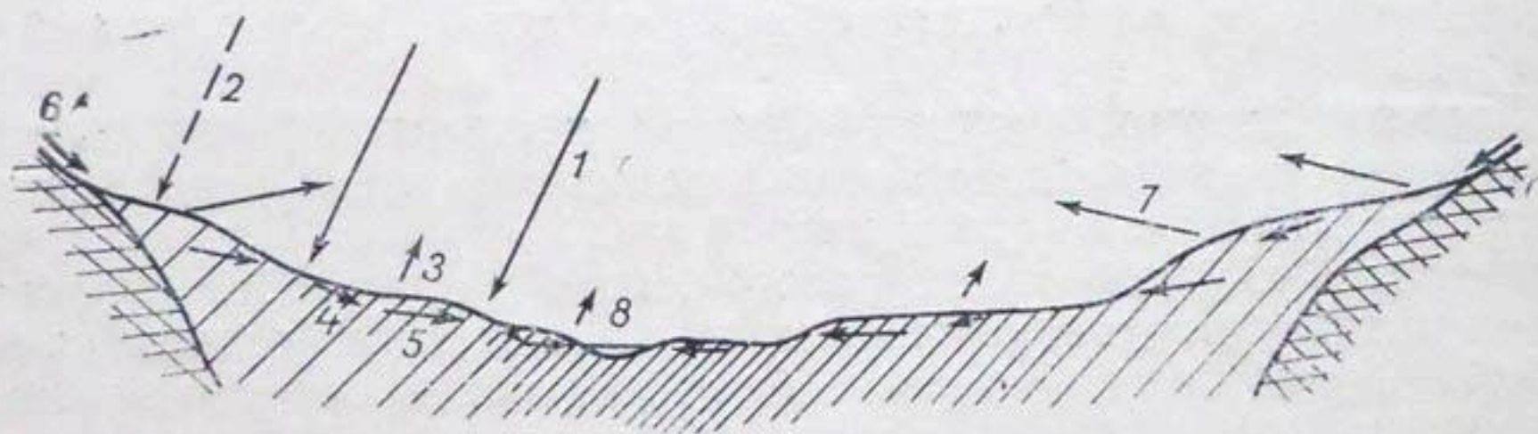
Рис. 29. Схема водного баланса межгорных долин.
