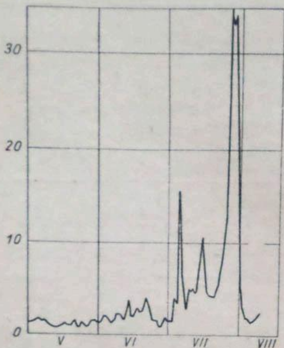
Рис. 50. Гидрограф стока половодья на реке со слабой сезонной зарегулированностью, р. Тосор — пост устье р. Кодол (Иссык-Кульский бассейн), 1965 г. В августе очередным большим паводком пост был разрушен, поэтому наблюдения были прерваны.
