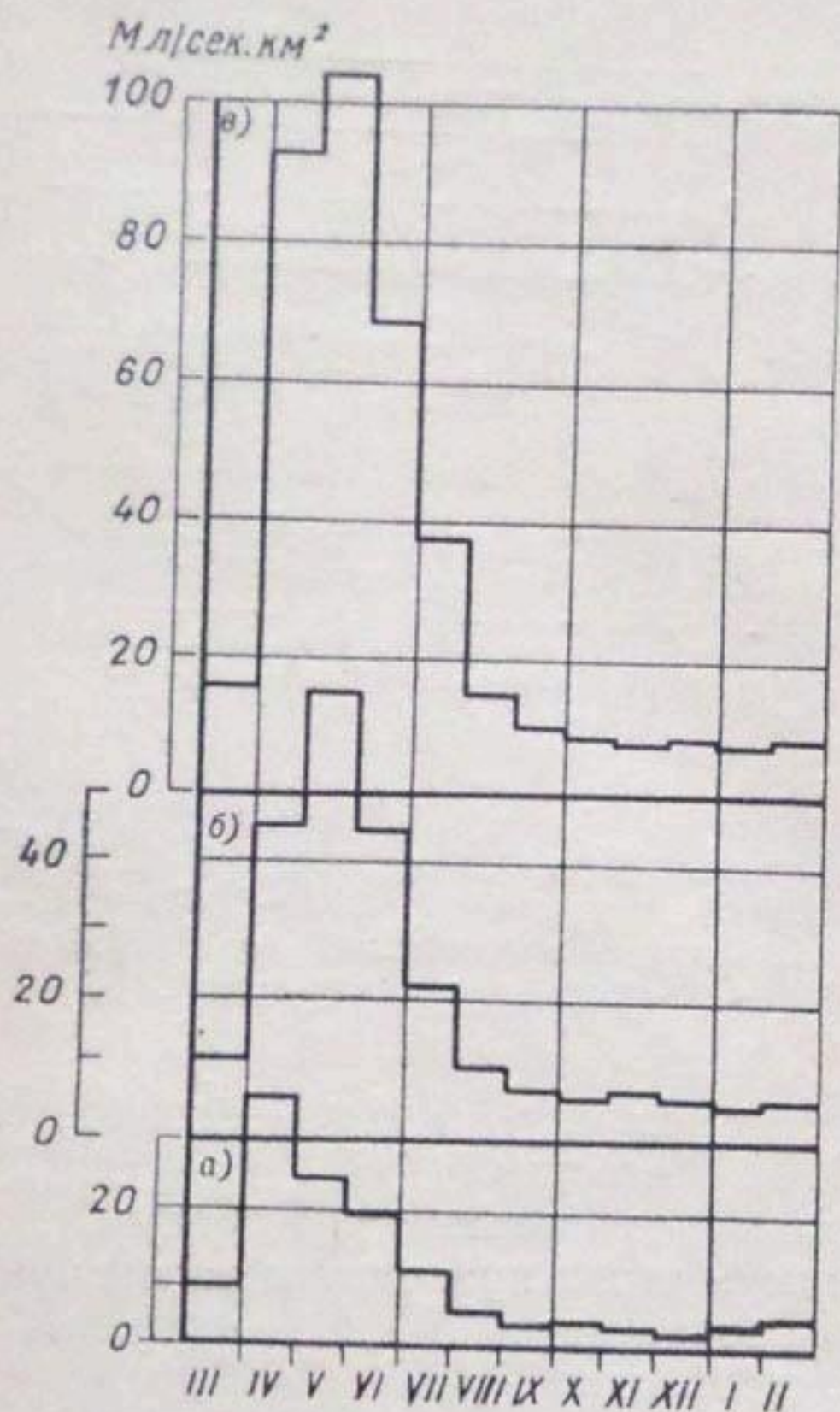
Рис. 60. Гидрографы стока р. Кугарт (с. Михайловка) за маловодный (а; 1938-39 г.), средний (б; 1925—1960 гг.) и многоводный (в; 1952-53 г.) годы (в модулях стока).
