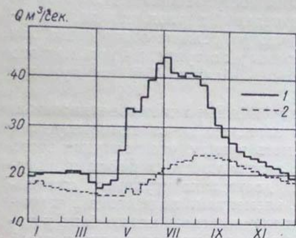
Рис. 14. Многолетние гидрографы общего (1) и подземного (2) стока р. Чу (пост Кочкорка).
