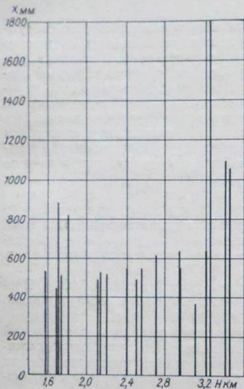
Рис. 22. Годовые осадки в бассейне по данным осадкомеров за 1959-60 г. в стандартных календарных рамках осадкового года (октябрь — сентябрь).
