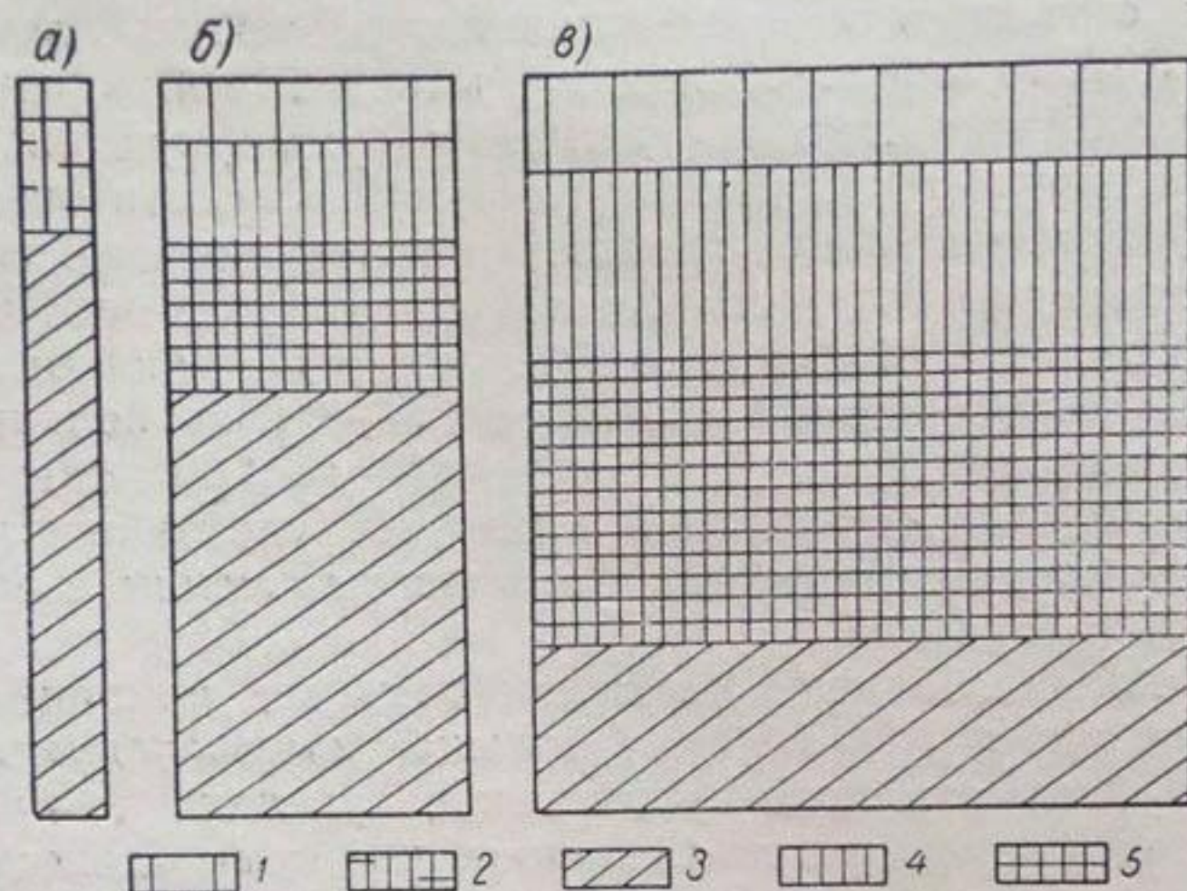
Рис. 26. Состав водного баланса стока Алаарчинского бассейна за пентадный (а), сезонный (б) и годичный (в) расчетные периоды.
