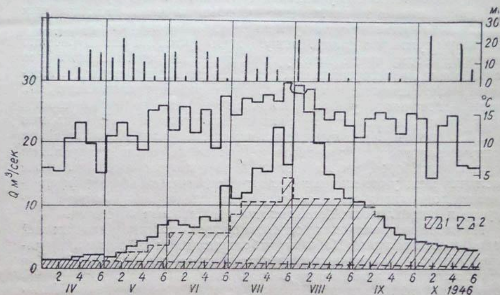
Рис. 13. Гидрограф стока р. Шамси (пост Лесной Кordon) с выделением устойчивой грунтовой (1) и сезонной грунтовой (2) составляющих стока. Температура воздуха и осадки взяты по метеостанции Байтык.
