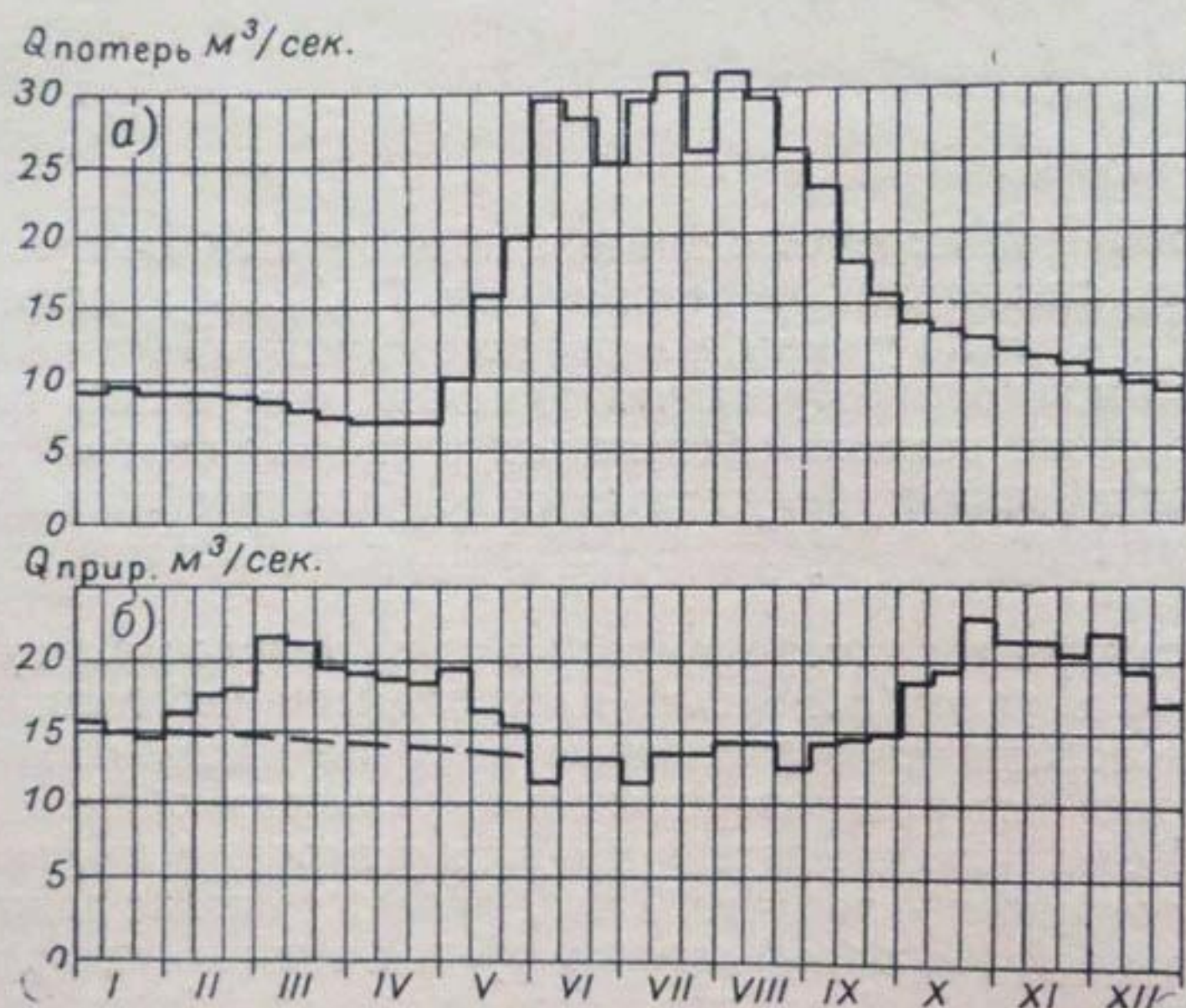
Рис. 32. Средние многолетние гидрографы потерь русловых вод на участке п. Бурулдайский мост — г. Токмак (а) и приращения руслового стока на участке г. Токмак — п. Милянфан (б).
