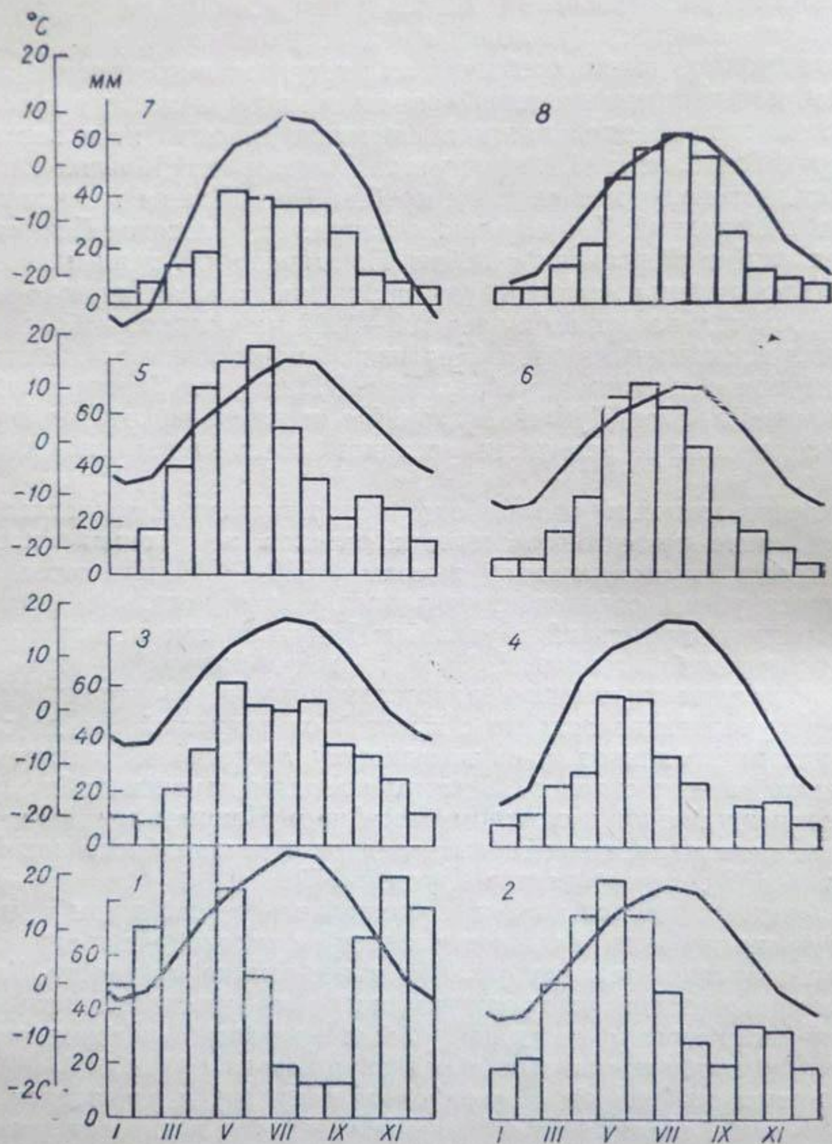
Рис. 2. Внутригодовое распределение атмосферных осадков и ход температуры воздуха по некоторым станциям в многолетнем разрезе (осадки взяты за 1936—1960 гг., по ст. Акташ — за 1951—1960 гг., температура приведена к периоду 1881—1960 гг.).
