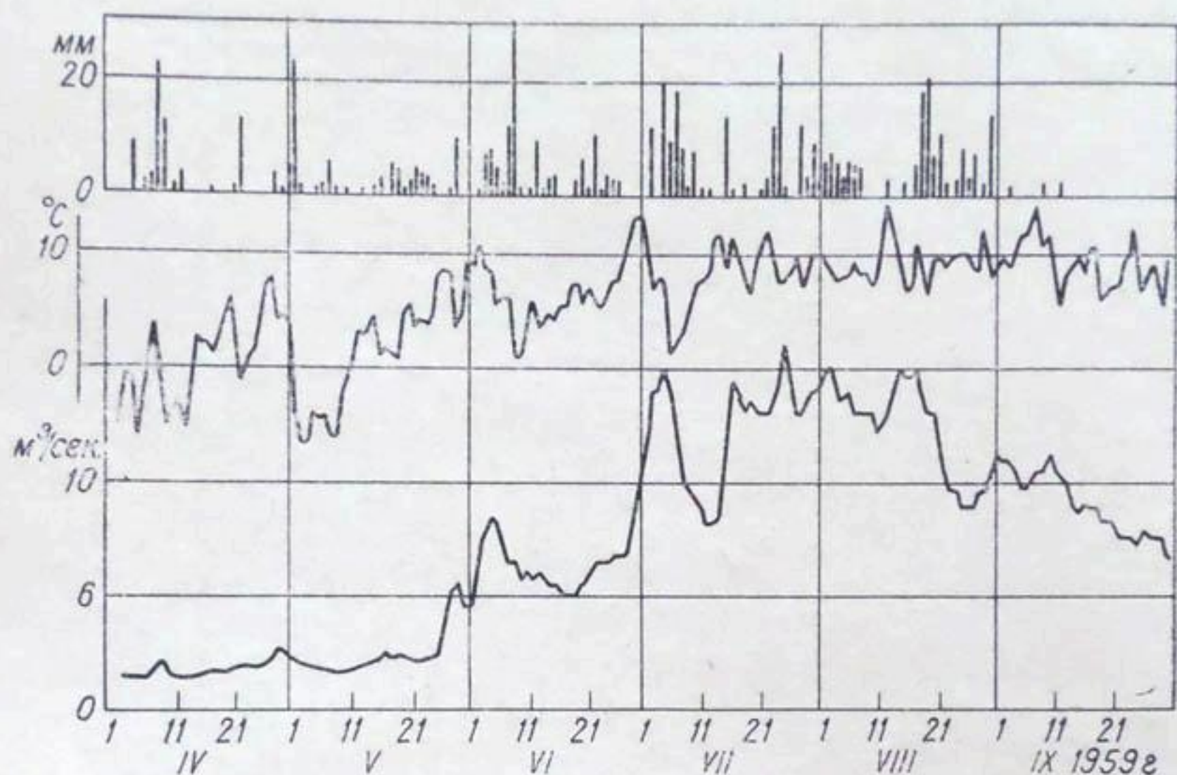
Рис. 19. Ход осадков, температуры воздуха (метеостанция Алаарча) и стока р. Алаарчи (устье р. Кашкасу).
