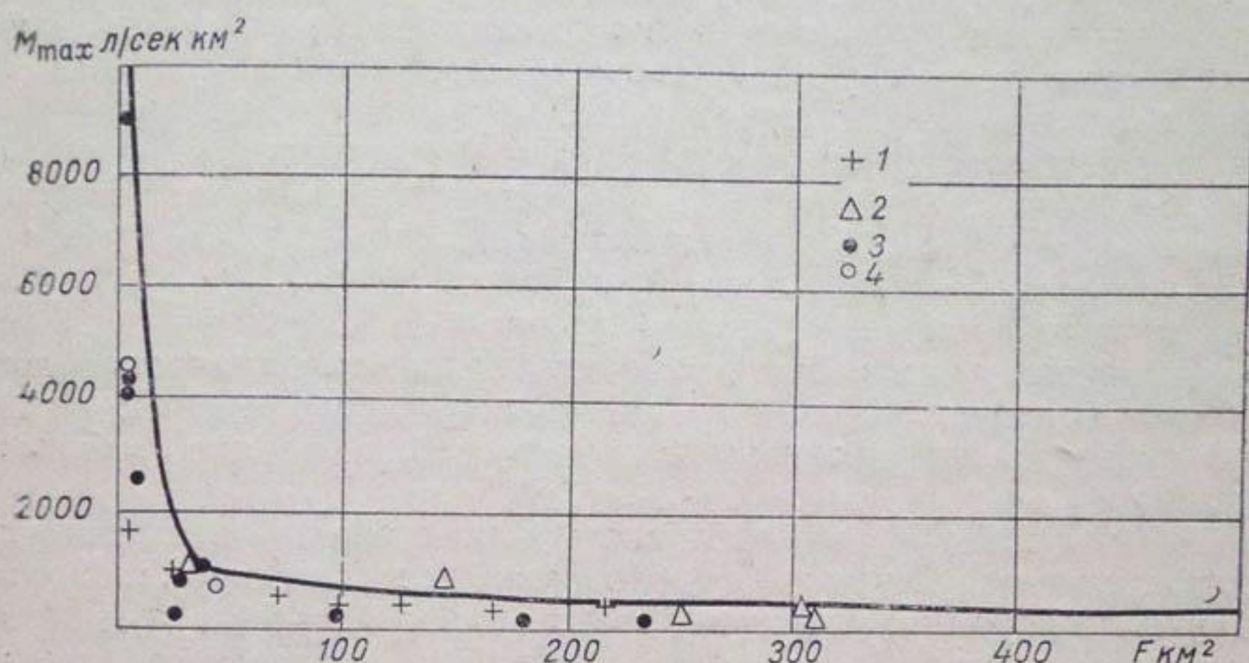
Рис. 52. Зависимость (верхняя огибающая) модулей максимального стока (3—5%-ной обеспеченности) для рек и саев Киргизии от площадей водосборов.
