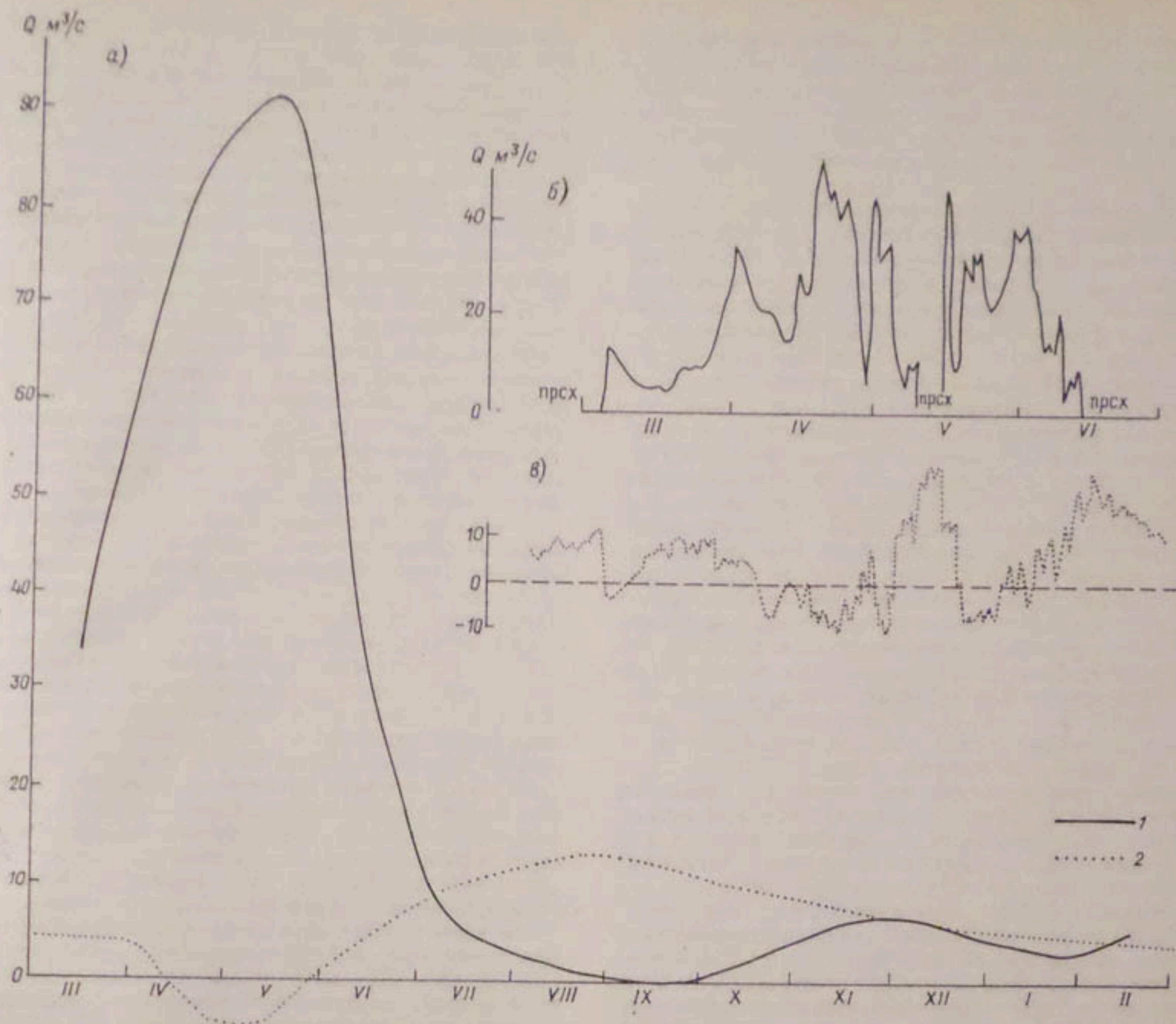
Рис. 4.5. Гидрограф стока р. Ахангаран и результирующей дополнительного притока в Туябугузское водохранилище. а — средние многолетние значения, б — паводковый период 1975 г., г — невязка суточных балансов, 1975 г. 1 — приток из р. Ахангаран, 2 — подземный приток.
