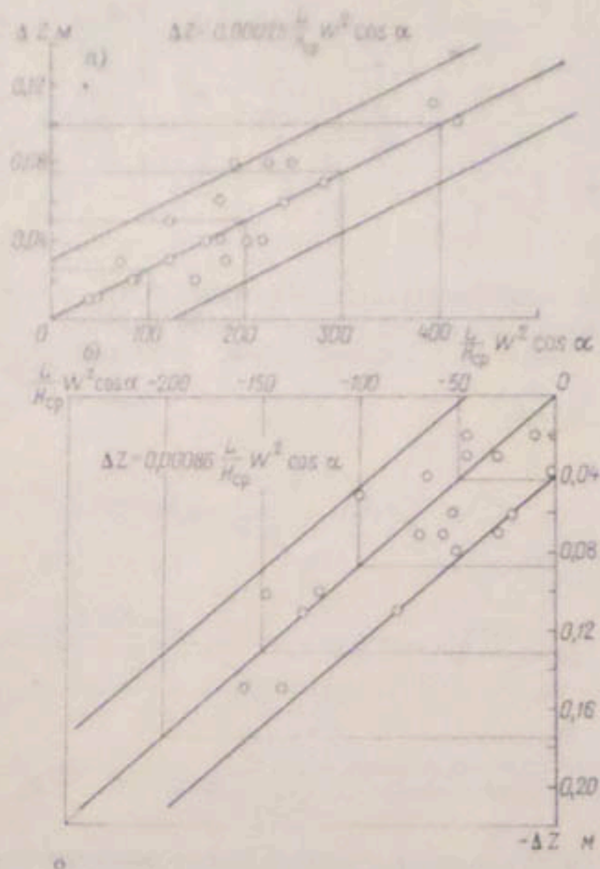
Рис. 3.4. Зависимость значений стога — нагона от скорости ветра и морфологических параметров чаши Кайракумского водохранилища. а — нагон, б — стог.
