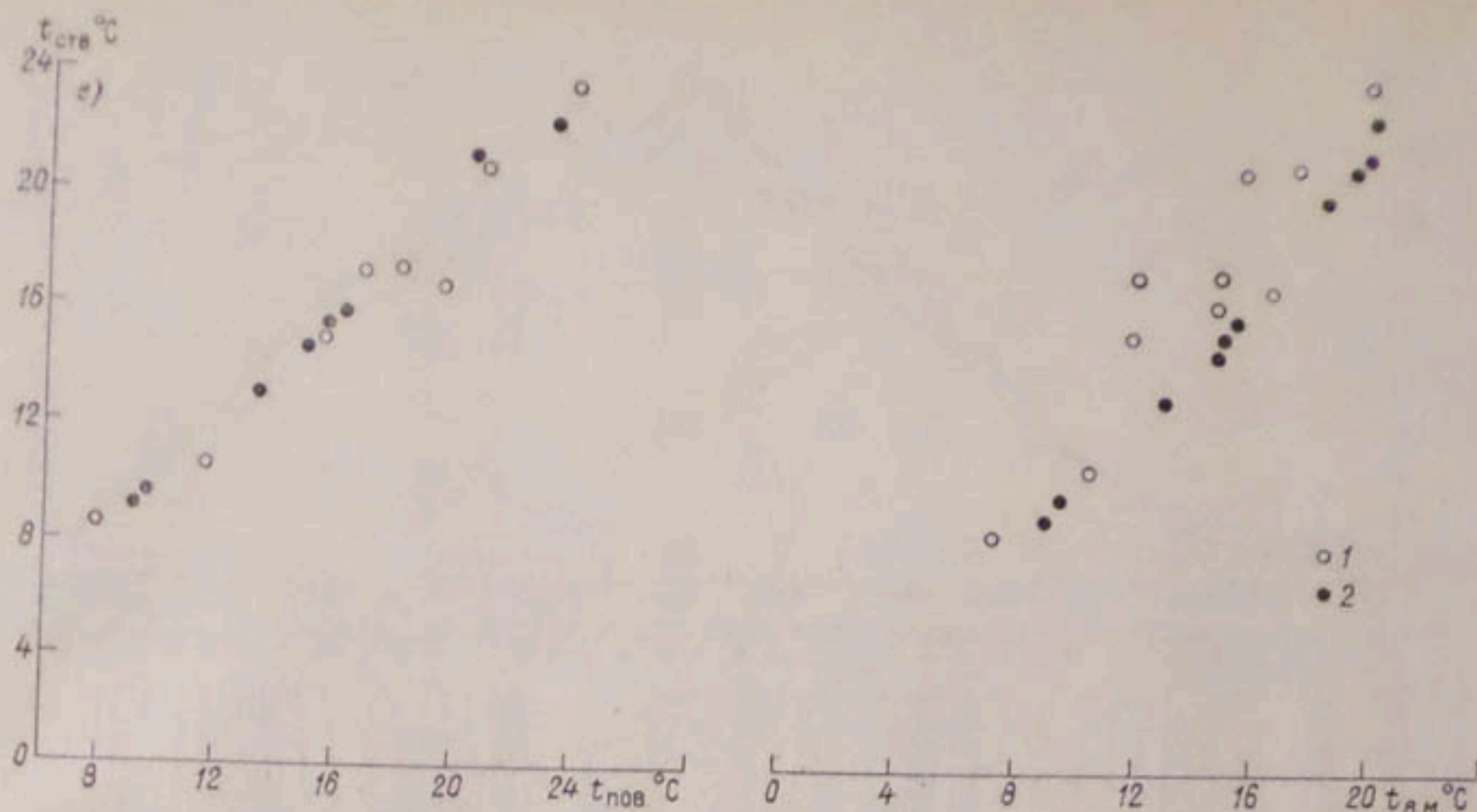
массы (2) ( t_{г, в} ) от температуры воды на гидрометрическом створе ( t_{ств} ). а — Кайраккумское, б — Гумбузекское, в — Уртатокайское.
