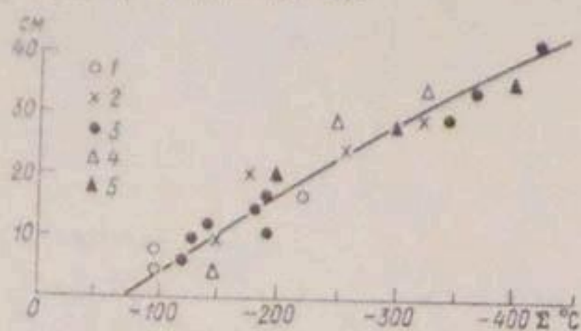
Рис. 6.7. Зависимости толщины льда (см) от сумм отрицательных температур воздуха для водохранилищ Средней Азии.
