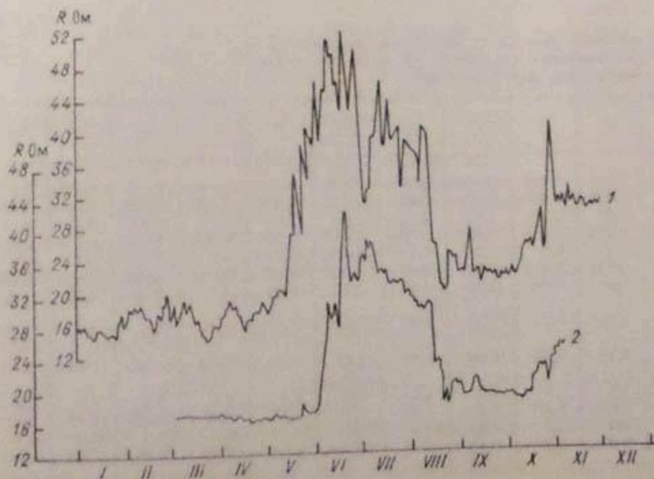
Рис. 10.10. Ежедневное сопротивление воды ( R ) на постах р. Сырдарья у кишла. Акджар (1) и Кайраккумского водохранилища у г. Кайраккум (2).
