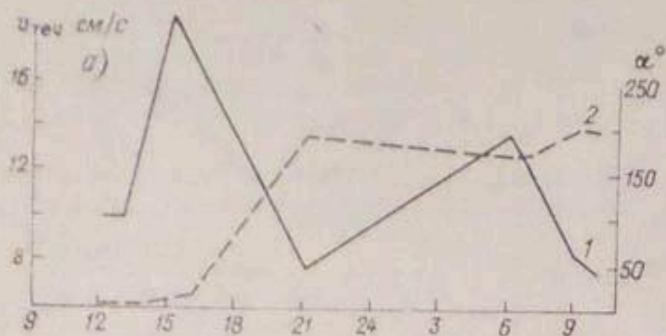
Рис. 8.9. Суточный ход направлений скоростей ветровых течений в поверхностном слое (20 см) воды Чарвакского водохранилища и ветра 5—6/VIII 1977 г.
