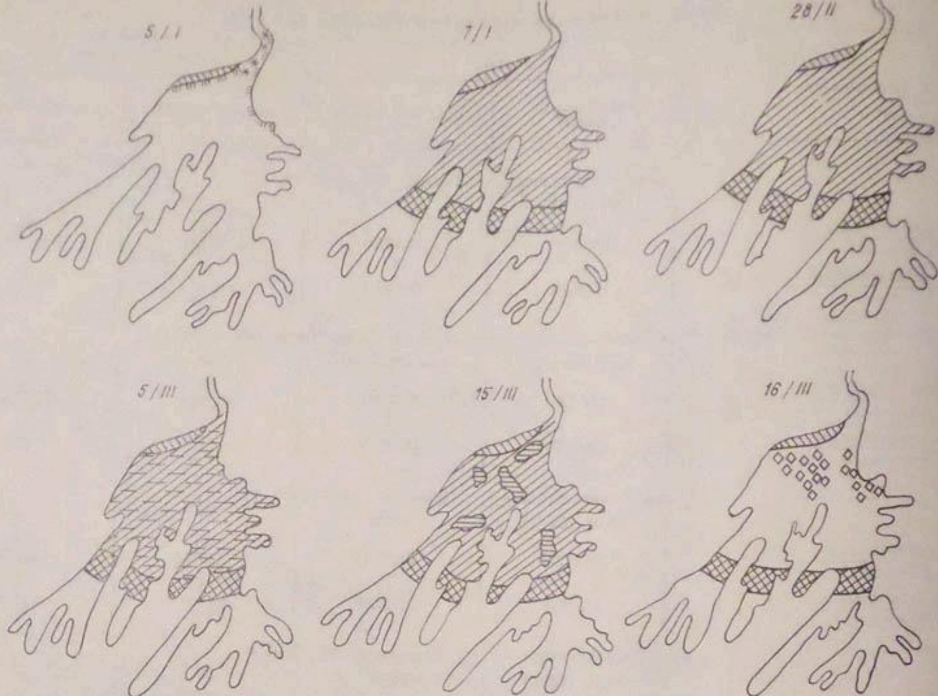
Рис. 6.2. Картограммы ледовых явлений Каттакуртанского водохранилища. Усл. обозначения см. на рис. 6.1.
