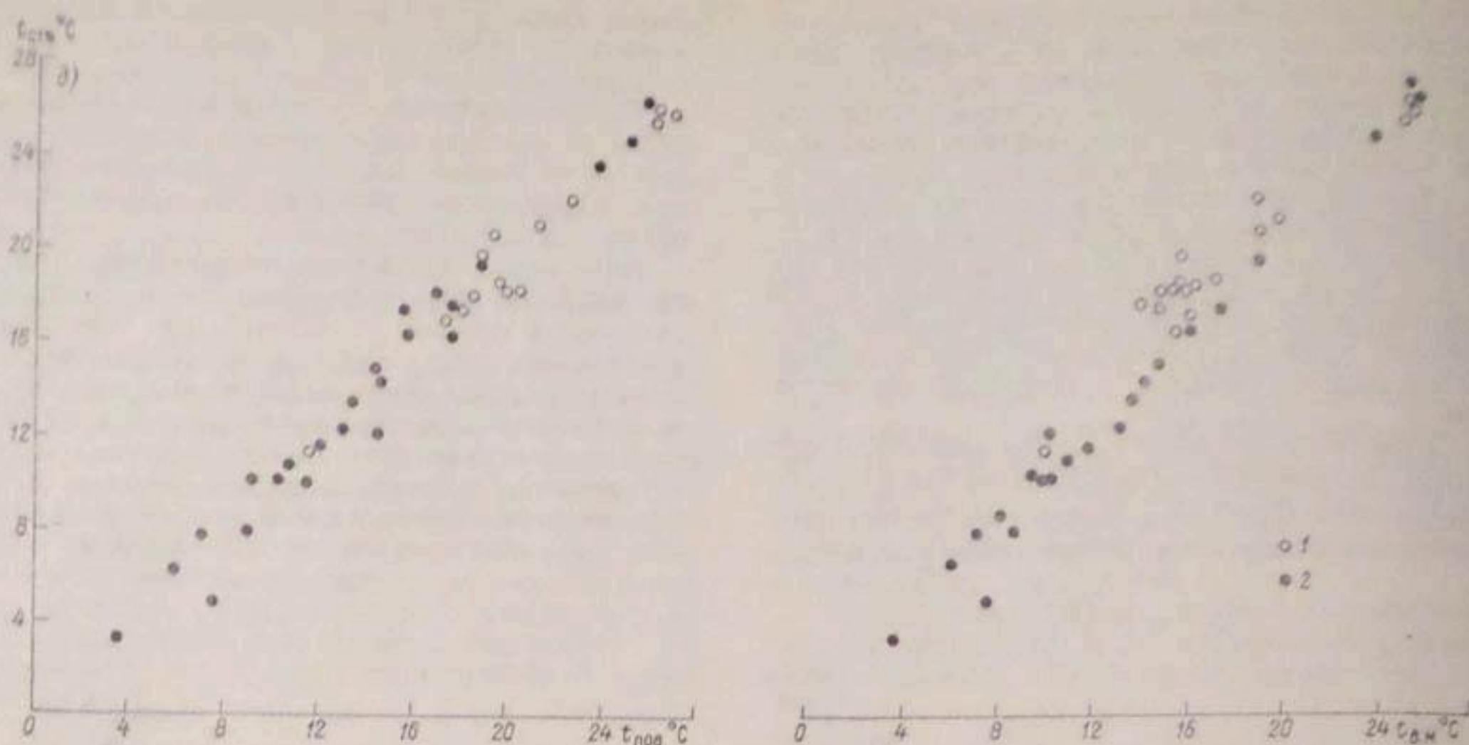
Рис. 5.7. Зависимости температуры поверхности воды (1) ( t_{\text{поверх}} ) и водной (2) ( t_{\text{глубина}} ) в водохранилищах: а — Чимкурганское, б — Каттакурганское, в — Куюмазарское.
