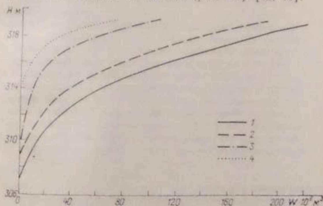
Рис. 9.1. Изменение объема чаши Фархадского водохранилища. 1 — 1948 г., 2 — 1950 г., 3 — 1953 г., 4 — 1955 г.
