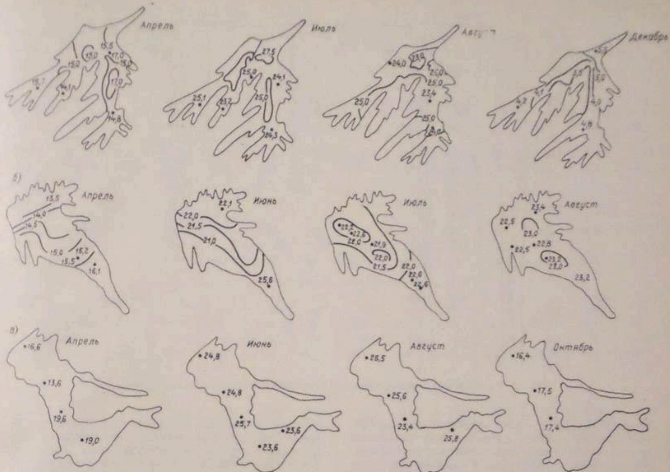
Рис. 5.3. Изменение температуры воды (°C) по сезонам года на поверхности водохранилищ. Водохранилище: а — Каттакурганское, б — Уртатокайское, в — Туymbугузское.
