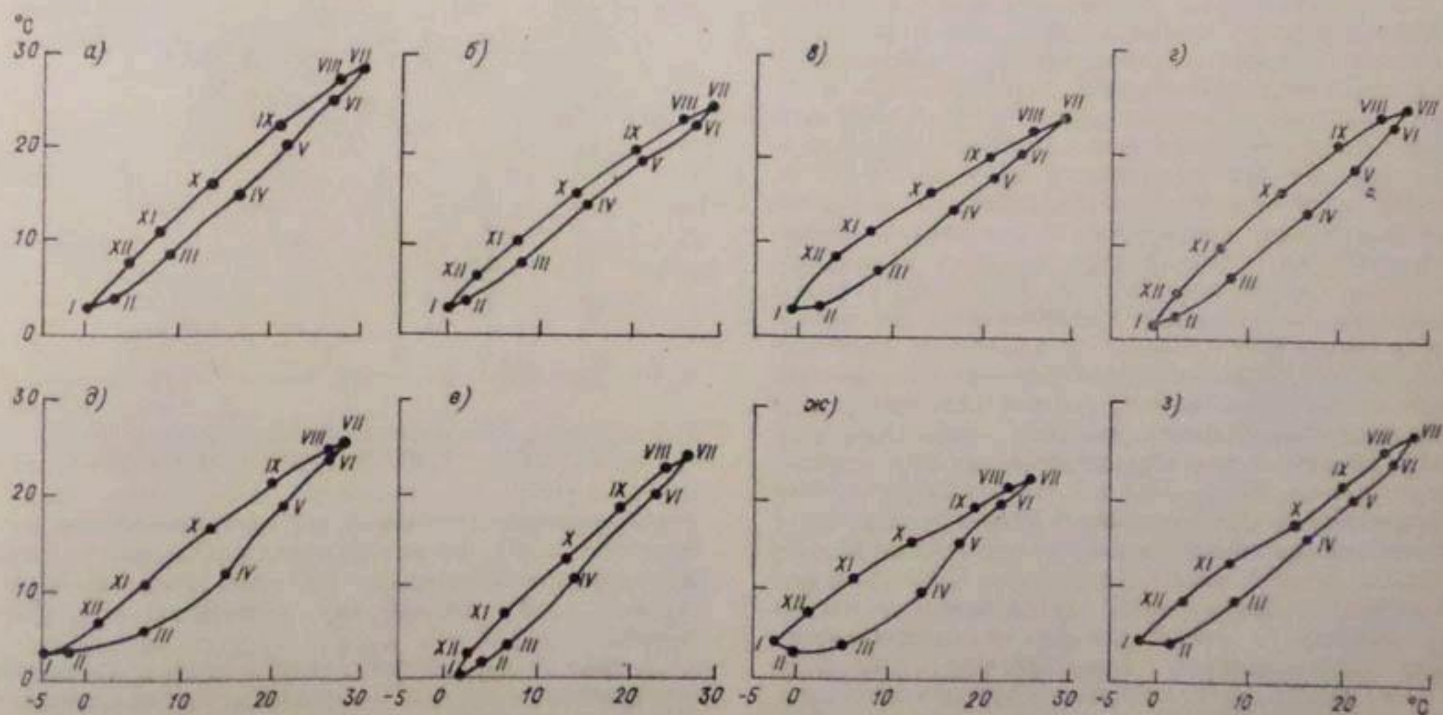
Рис. 5.4. Зависимости температуры поверхности воды (вертикальная шкала) от температуры воздуха (горизонтальная шкала). Водохранилище: а — Каттакурганское, б — Каттакурганское, в — Куюмзаарское, г — Кайраккумское, д — Чардаринское, е — Уртатокайское, ж — Чарвакское, з — Туymbугузское.
