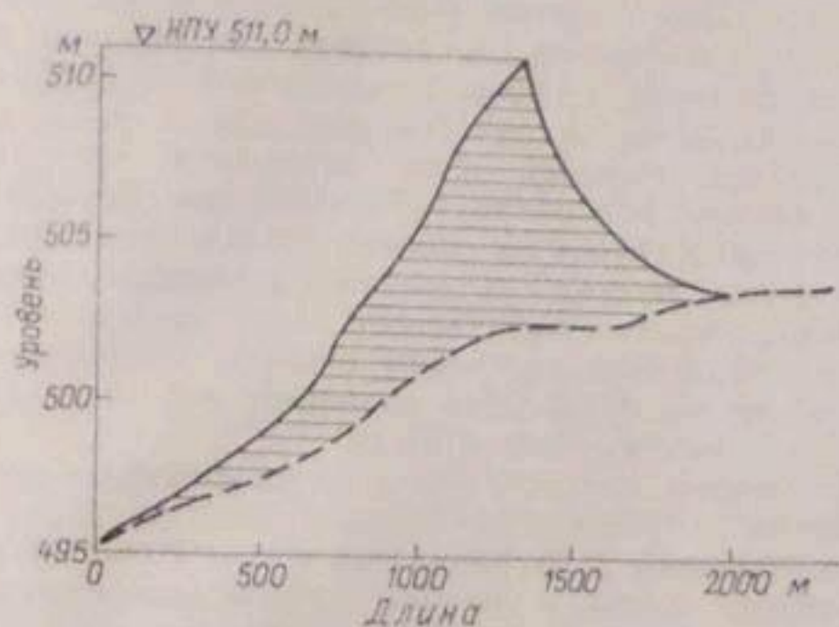
Рис. 4.3. Контур подземной регулирующей емкости Каттакурганского водохранилища. Штриховая линия — подошва.
