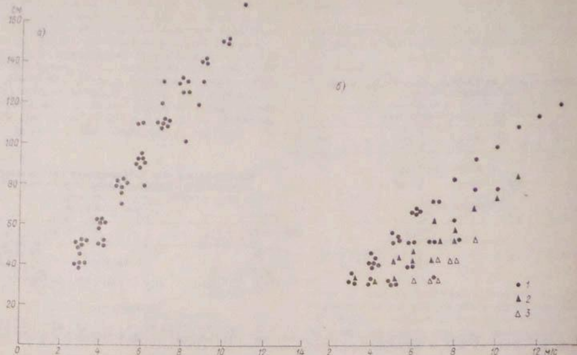
Рис. 7.2. Зависимость высоты волн (см) от скорости ветра (м/с) для Кайраккумского водохранилища. Волномерный пункт: а—г. Кайраккум, б—кишл. Джидалык. Ветер: 1—восточный, 2—северо-восточный, 3—юго-западный.
