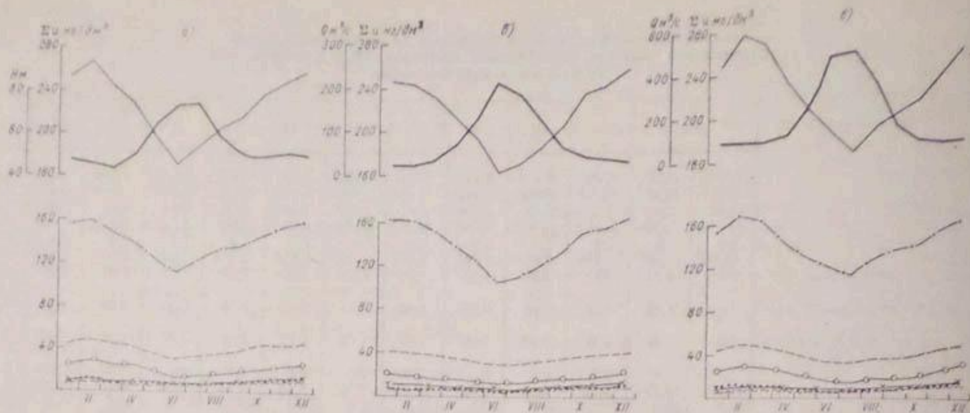
Рис. 10.12. Средневзвешенное содержание ионов и минерализация воды Чарвакского водохранилища (а), р. Пскем у кишла. Муалала (б) и р. Чирчик у г. Газалкент (в). Усл. обозначения см. на рис. 10.3.
