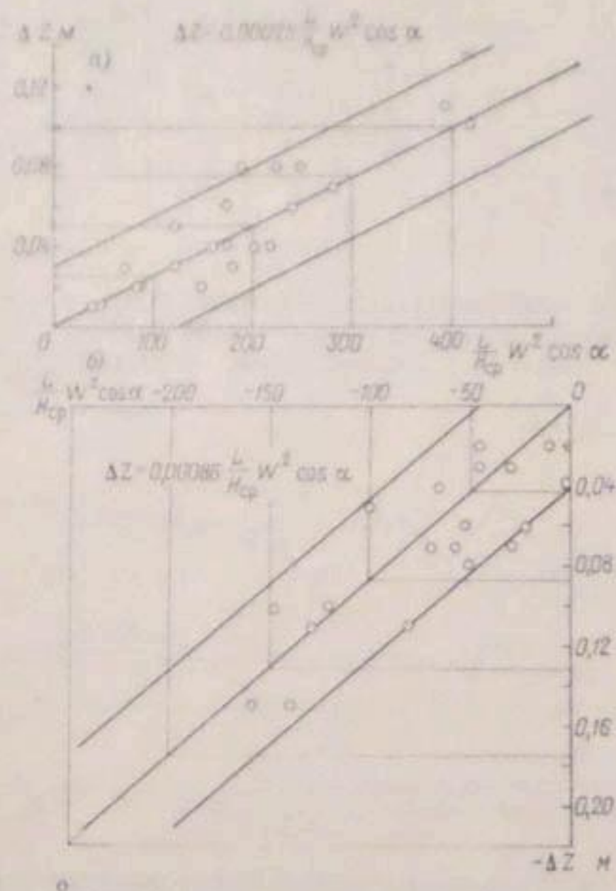
Рис. 3.4. Зависимость значений стога — нагона от скорости ветра и морфологических параметров чаши Кайраккумского водохранилища. а — нагон, б — стоп.
