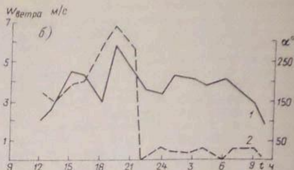
Рис. 8.9. Суточный ход направлений скоростей ветровых течений в поверхностном слое (20 см) воды Чарвакского водохранилища и ветра 5—6/VIII 1977 г.
