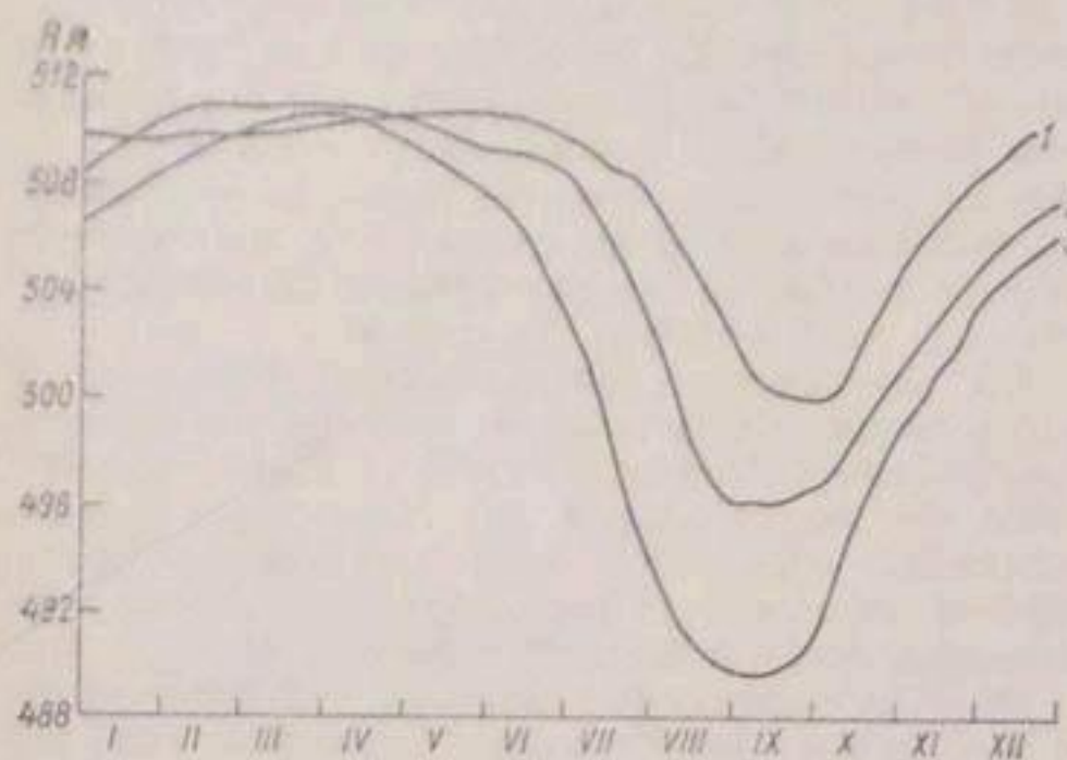
Рис. 3.9. Ход уровня Каттакурганского водохранилища за характерные годы.
