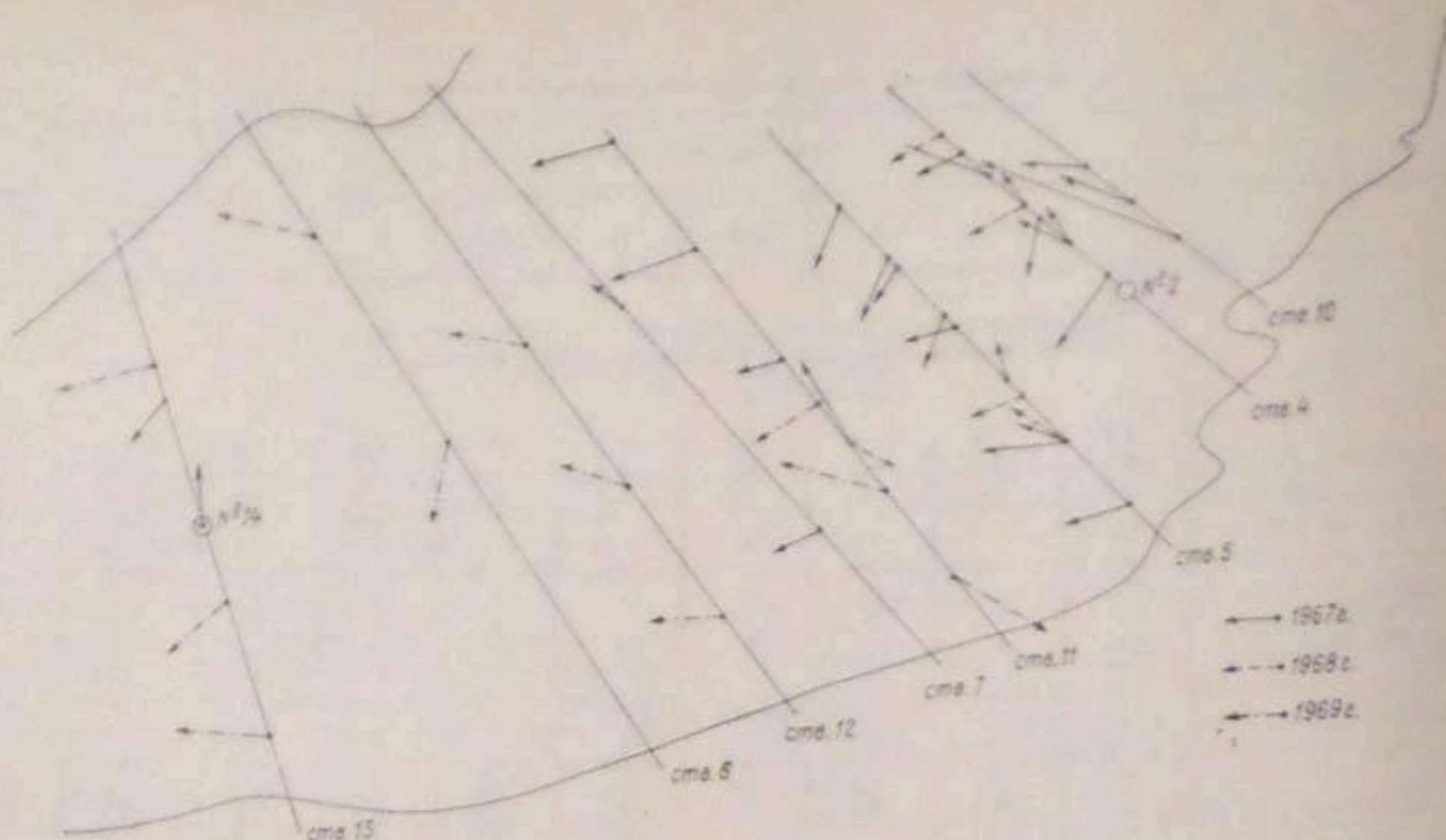
Рис. 8.1. Распределение скорости и направления течения в зимний период на 0.2 глубины Кайракумского водохранилища в зоне его активного заполнения.
