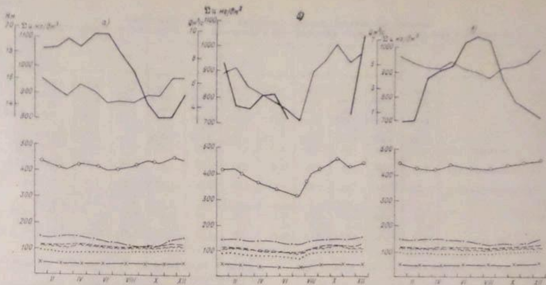
Рис. 10.4. Среднемесячное содержание ионов и минерализация воды Учкызылского водохранилища (а), канала Занг (б) и нижнего бьефа водохранилища (в). Усл. обозначения см. на рис. 10.3.
