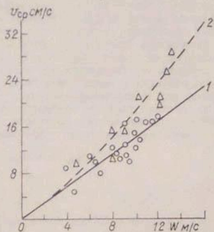
Рис. 8.5. Зависимость средней скорости вдольберегового потока ( v_{ср} ) от скорости ветра ( W ).
