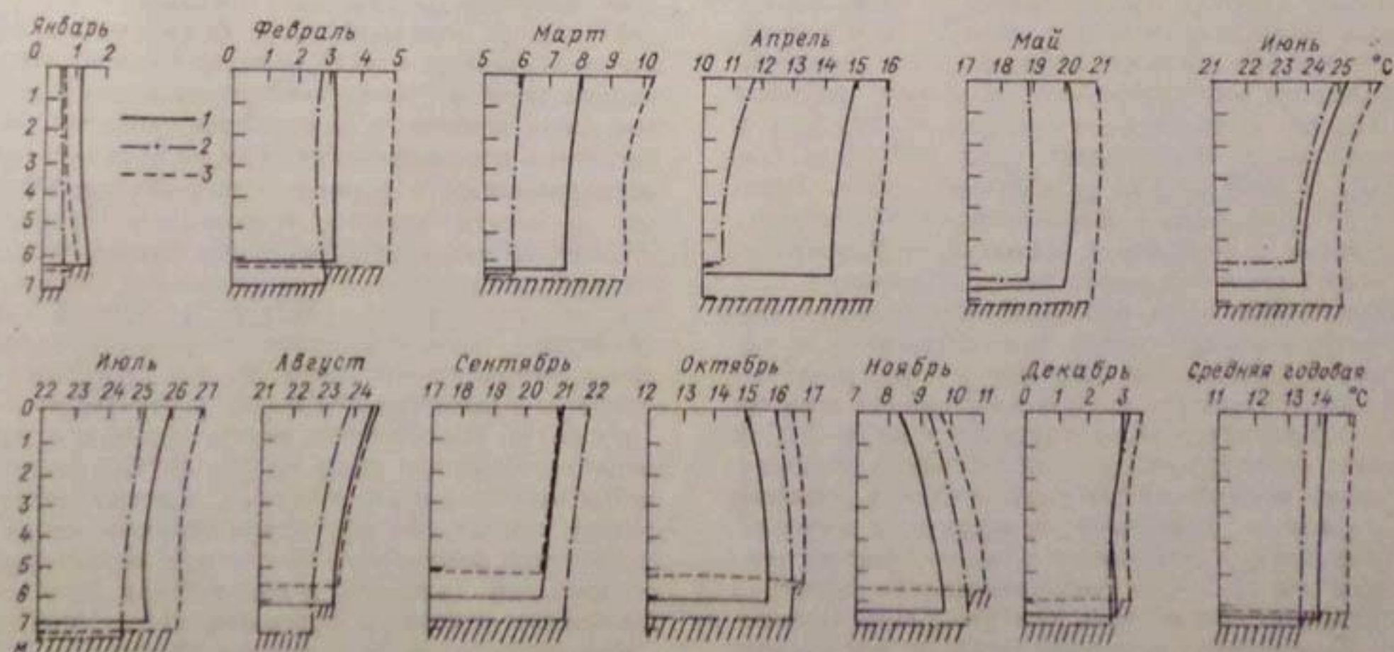
Рис. 5.9. Средние месячные эюры распределения температуры воды ( ^\circ\text{C} ) по глубине Кайраккумского водохранилища в средний и экстремальные годы.
