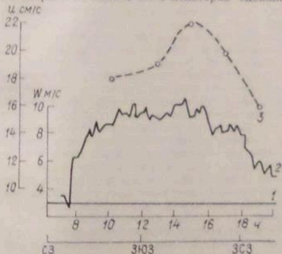
Рис. 8.3. Совмещенный график развития ветра и течения.
