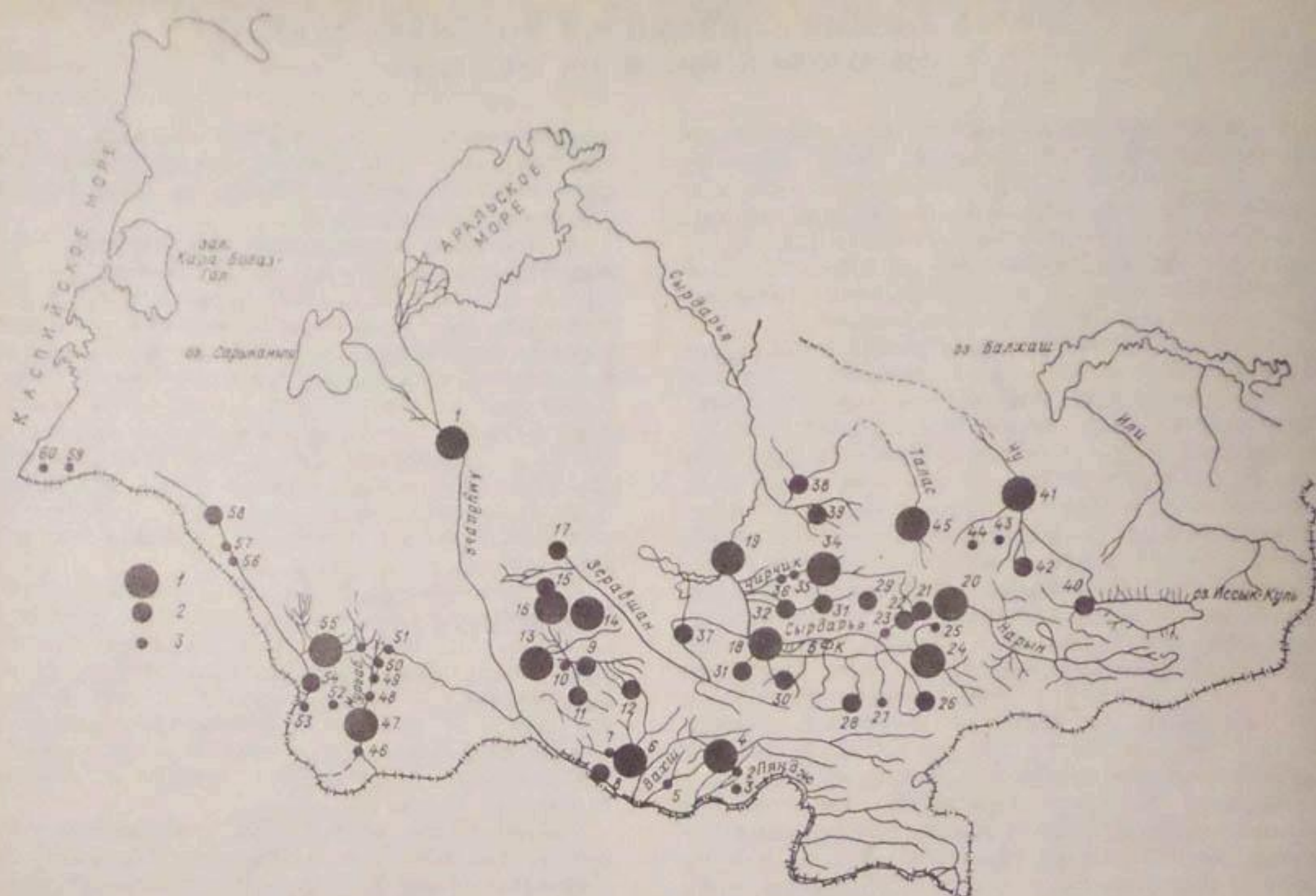
Рис. 1.1. Схема расположения водохранилищ Средней Азии.
