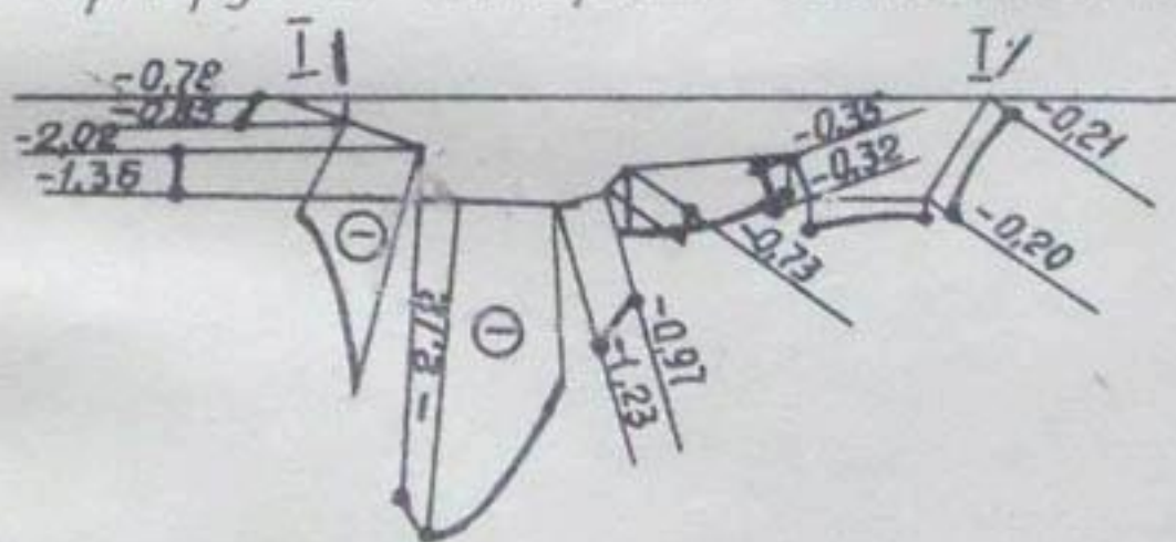
Рис. 3. Расчетные эпюры напряжений \sigma_y , кг/см и \sigma_y^{(A=1)} , т/см 2 в натуре по контактным сечениям плотина-основание: А- напряженное состояние под бычком в сечении I-I; Б- напряженное состояние под водосливом в сечении II-II; "а-в" - зона трещины по контакту.
