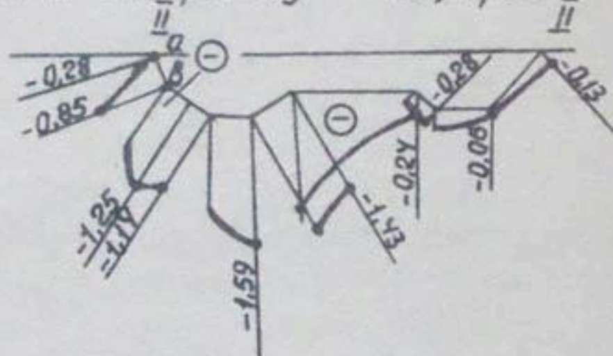
Рис. 3. Расчетные эпюры напряжений \sigma_y , кг/см и \sigma_y^{(A=1)} , т/см 2 в натуре по контактным сечениям плотина-основание: А- напряженное состояние под бычком в сечении I-I; Б- напряженное состояние под водосливом в сечении II-II; "а-в" - зона трещины по контакту.
