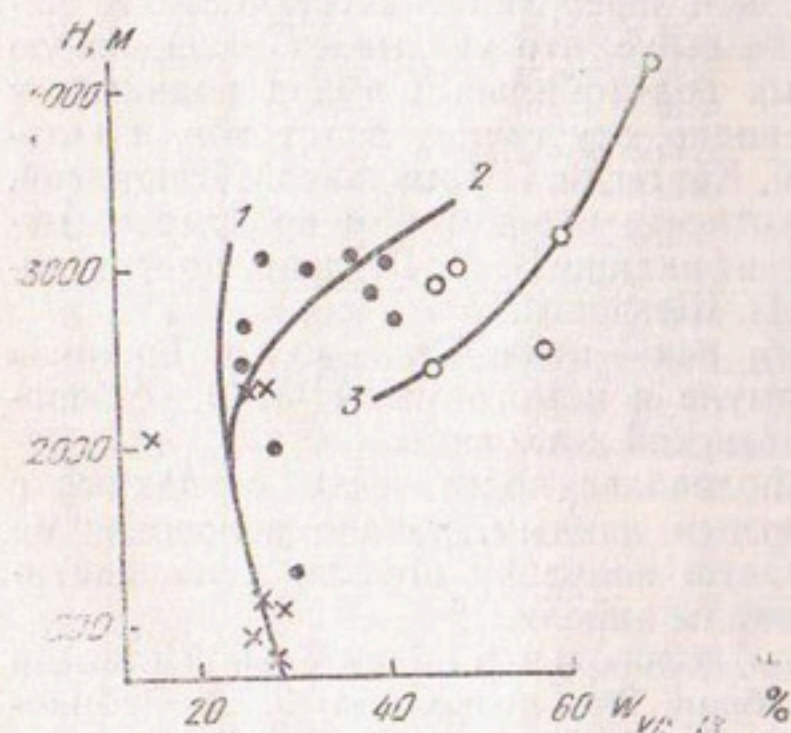
Рис. 26. Зависимость стока за июль — сентябрь от средневзвешенной высоты:
