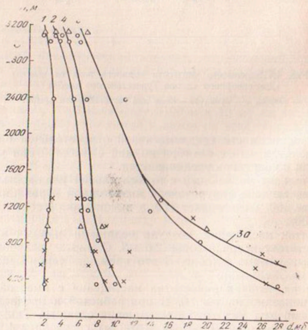
Рис. 7. Зависимость недостатка насыщения воздуха водяными парами от высоты за календарные сезоны: 1 — зима; 2 — весна; 3 — лето; 4 — лето для западной части хребта; 4 — осень.
