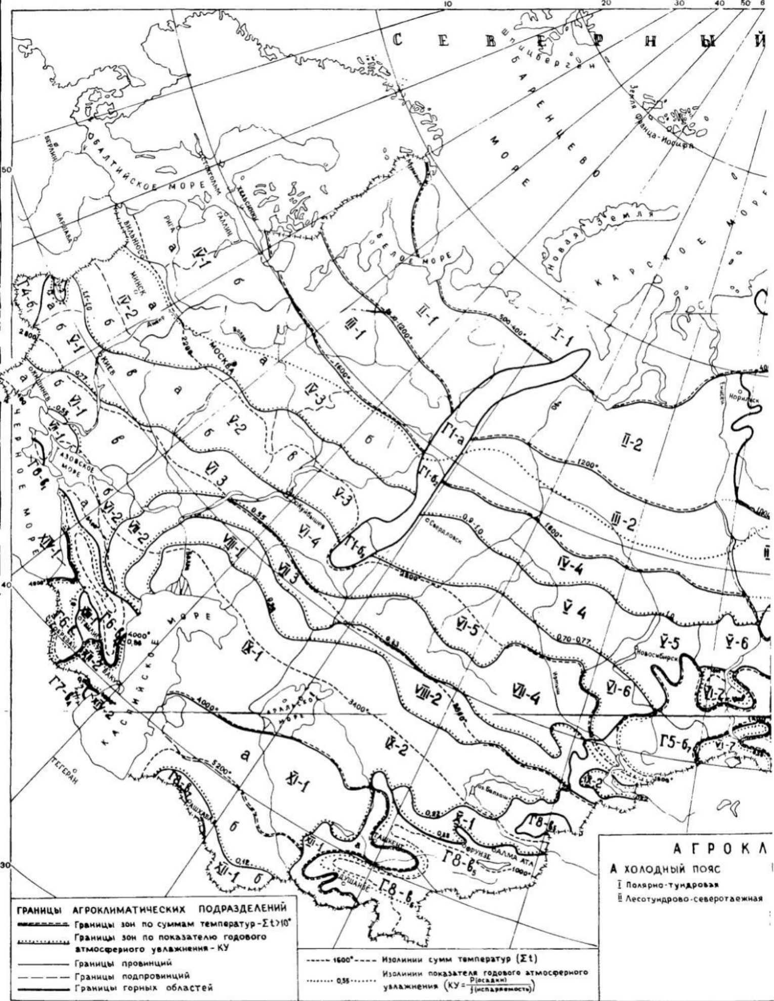
Рис. 33. Агроклиматическое ра
