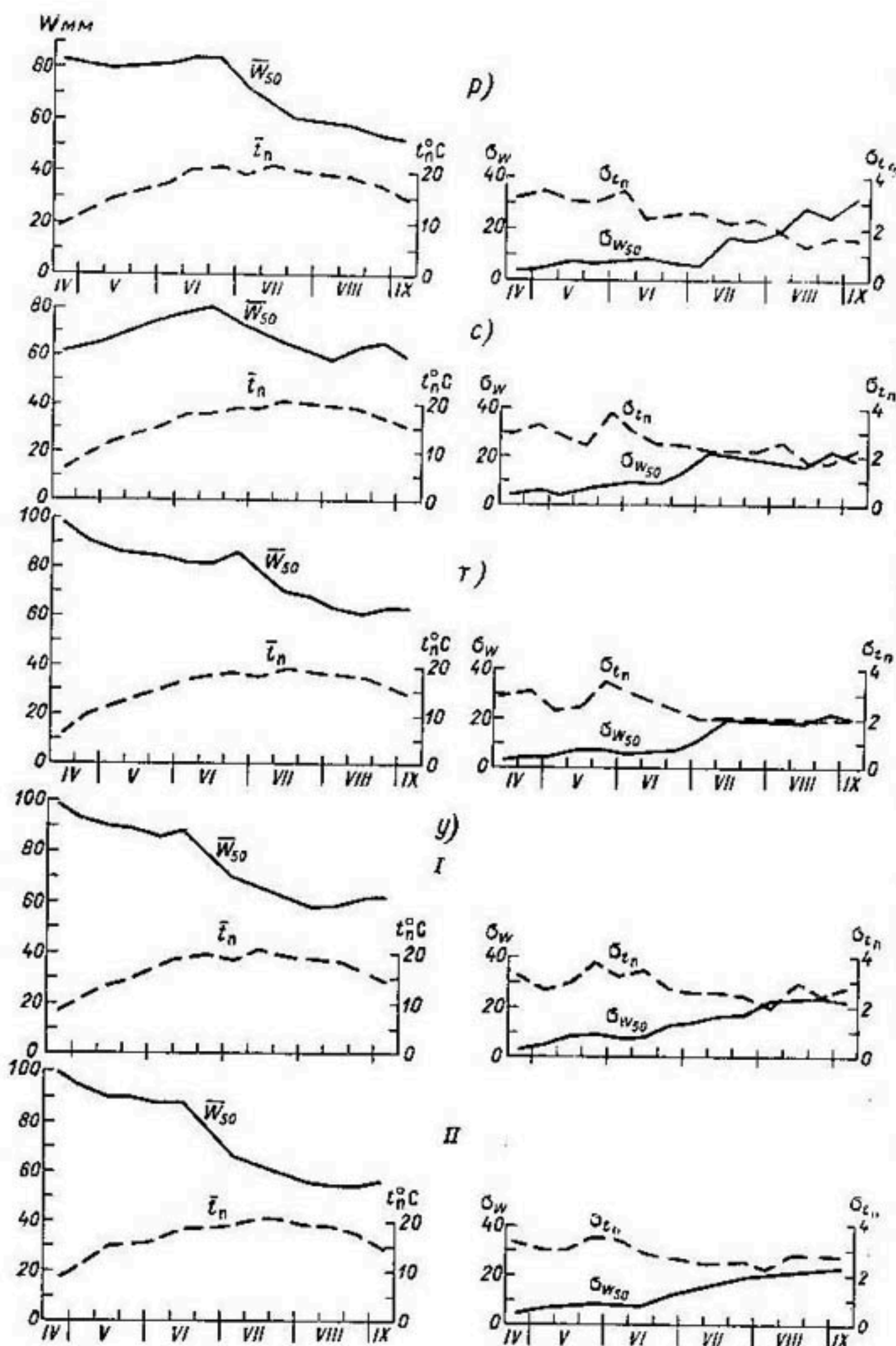
Рис. 20 p—ч. Изменение средних влагозапасов \bar{W} , температур \bar{t}_n и \sigma — Порецкое, n=20 ; c — Марыина Горка, n=20 ; r — Рославль, n=21 ; y — Волово; ч — Камешная
