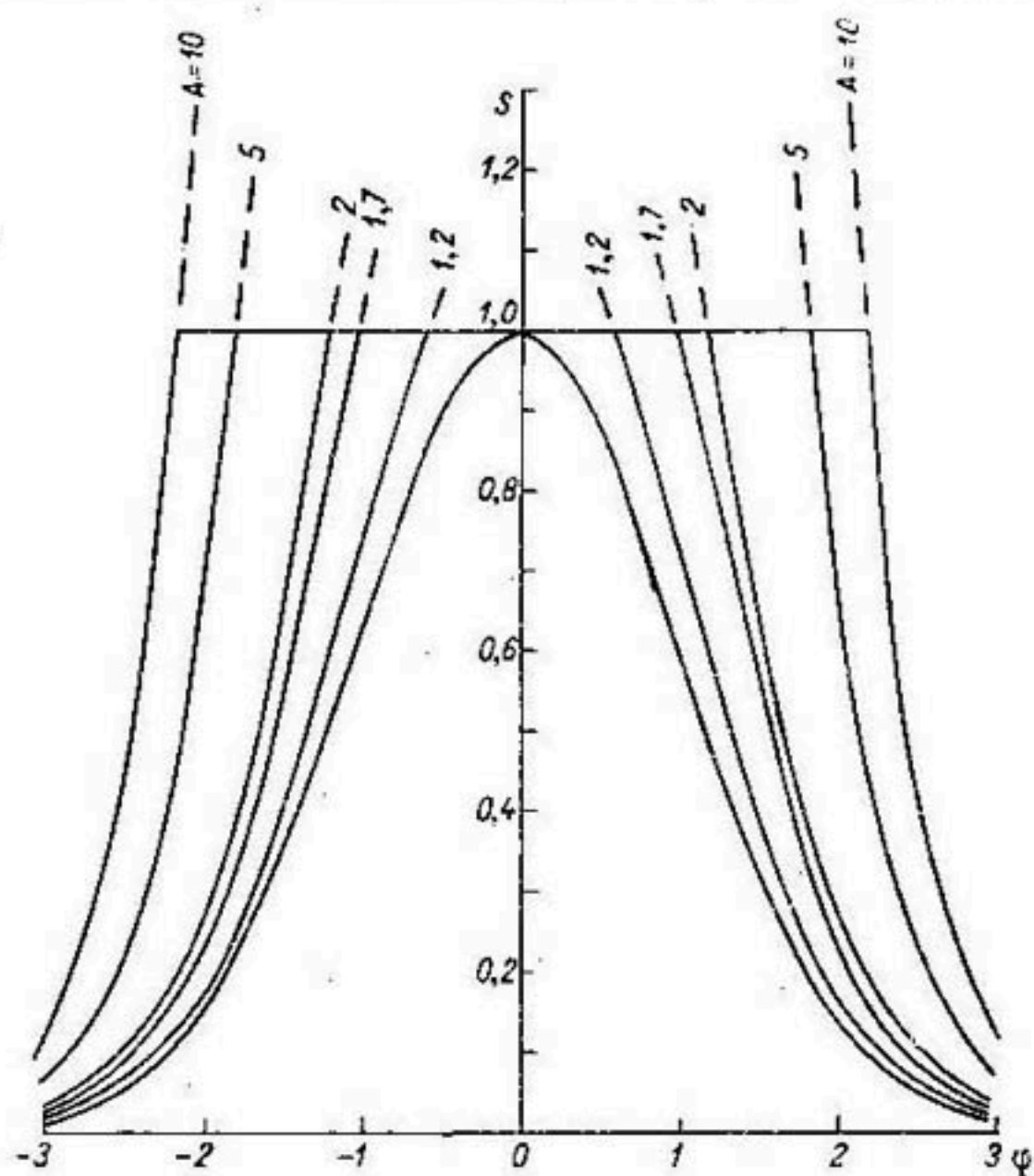
Рис. 10. Зависимости S = A_1 \exp(-\varphi^2/2) при разных значениях A_1 .
