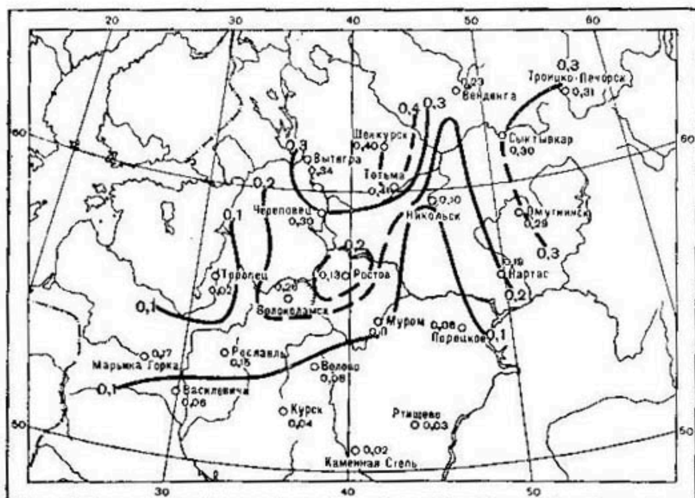
Рис. 21. Вероятность оптимальных гидротермических условий P_{\text{ср. опт.}}
