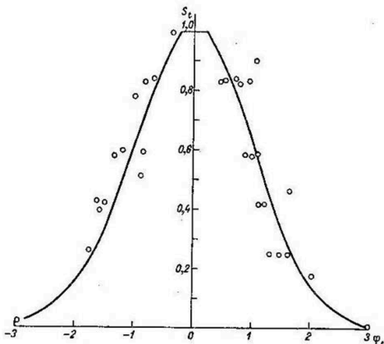
Рис. 8. Зависимость урожая картофеля от температуры.
