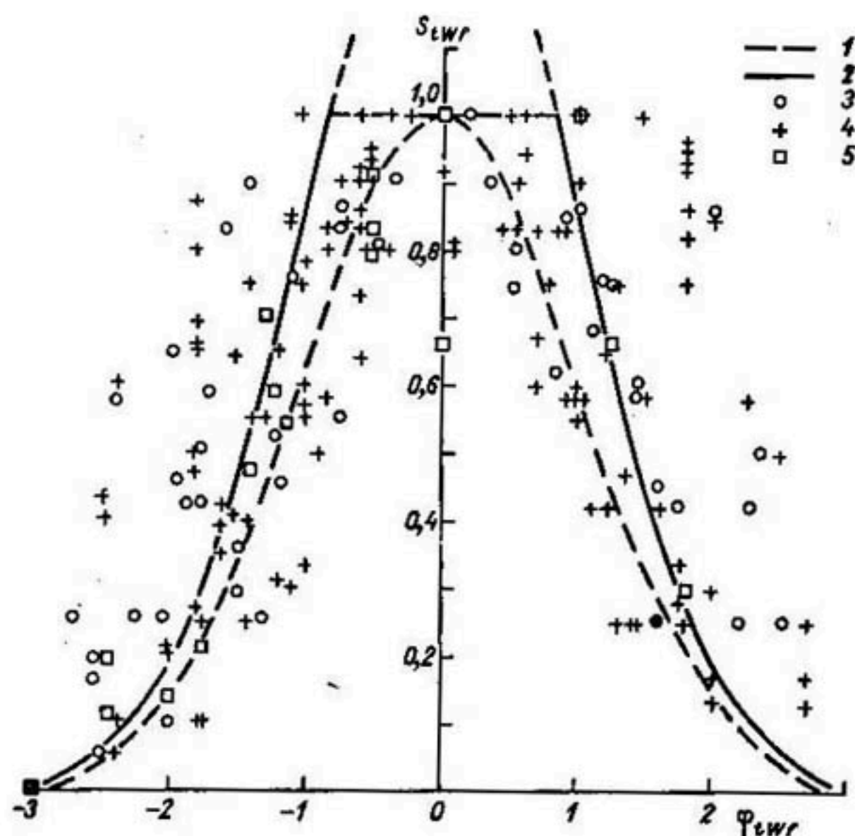
Рис. 5. Зависимость жизнедеятельности растений S от факторов внешней среды (водного \varphi_w , теплового \varphi_t и фактора питания \varphi_f ). 1 — S = 1,0 \exp(-\varphi^2/2) , 2 — S_{twf} = 1,38 \exp(-\varphi^2/2) , 3 — вода, 4 — температура, 5 — питание.
