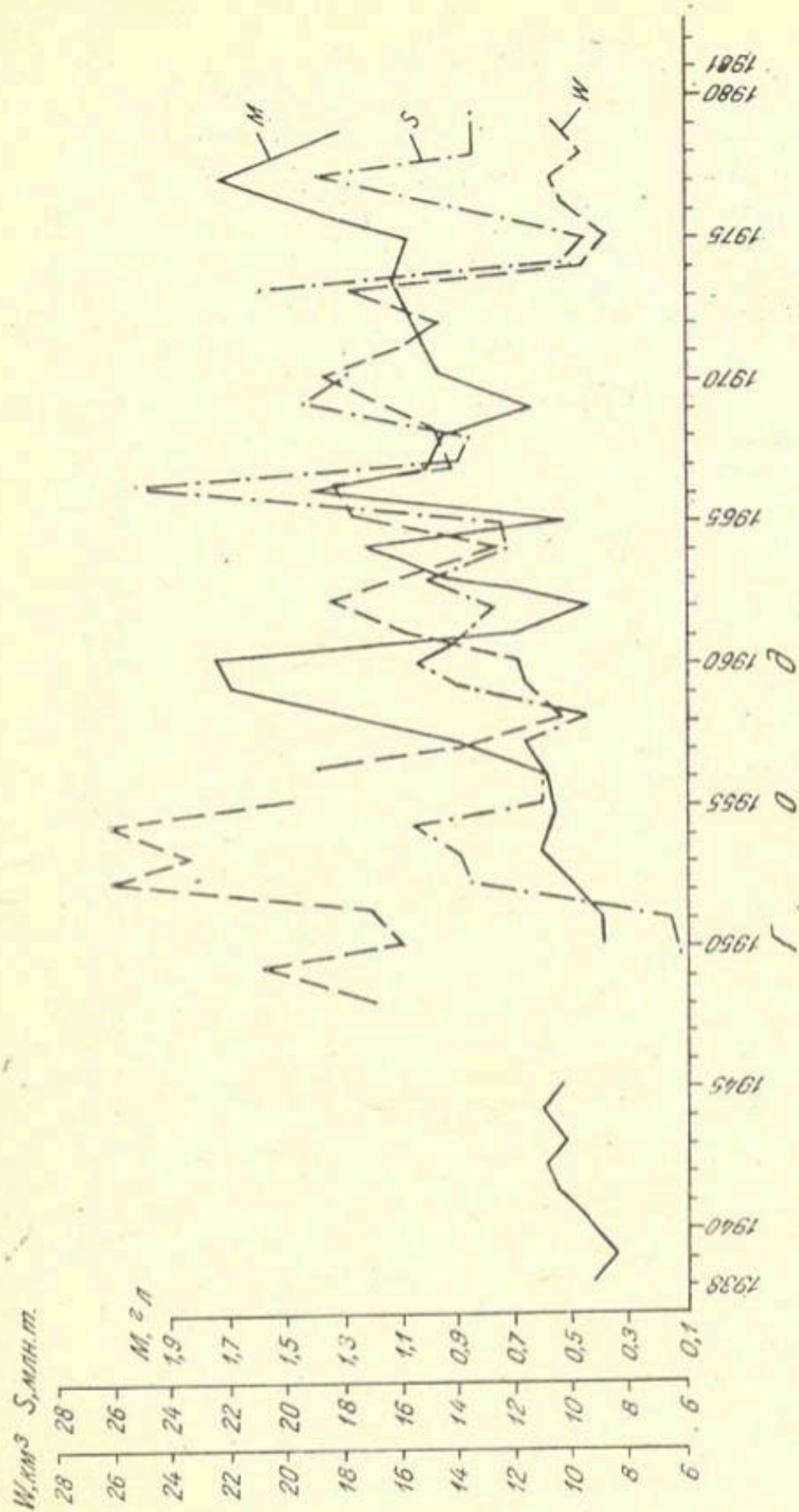
Рис. 42. Многолетние изменения минерализации (М, г/л), водного (W, \text{km}^3 ) и солевого (S, млн т) стоков в р. Сырдарье у створа Кзыл-Кышлак.
