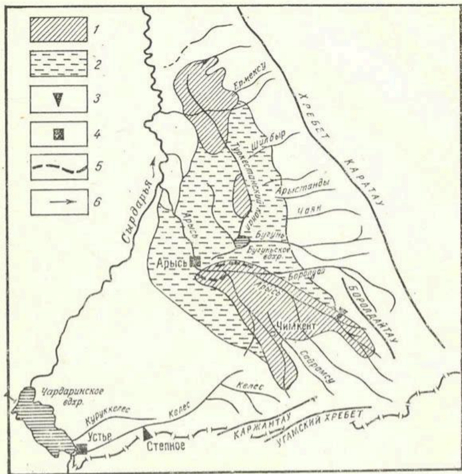
Рис. 19. Араль-Туркестанский оазис:
