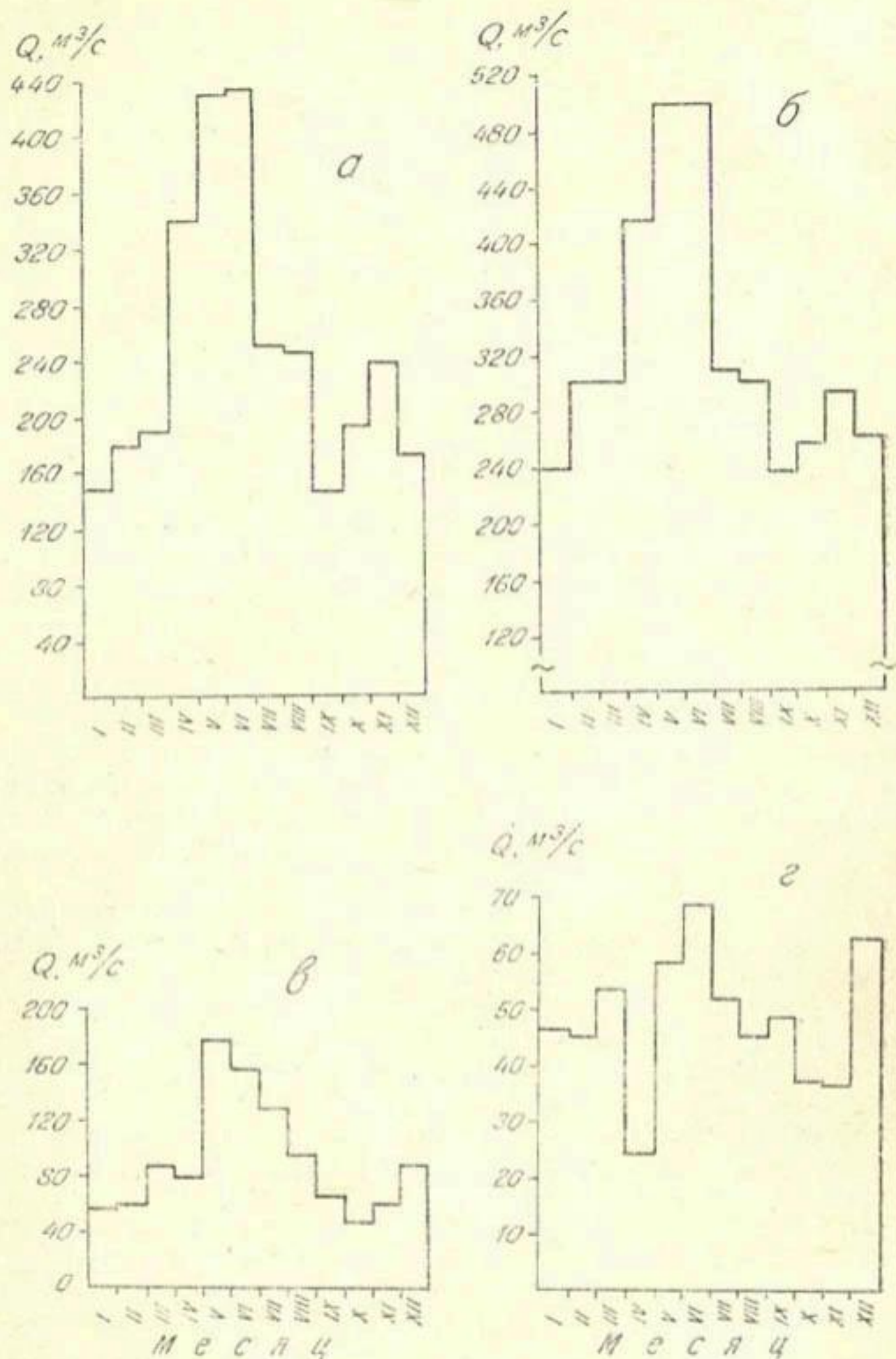
Рис. 1. Внутригодовое распределение стока р. Сырдарьи на створах: а) Каль; б) Акджар; в) Кзыл-Сурда; г) Казалинск.
