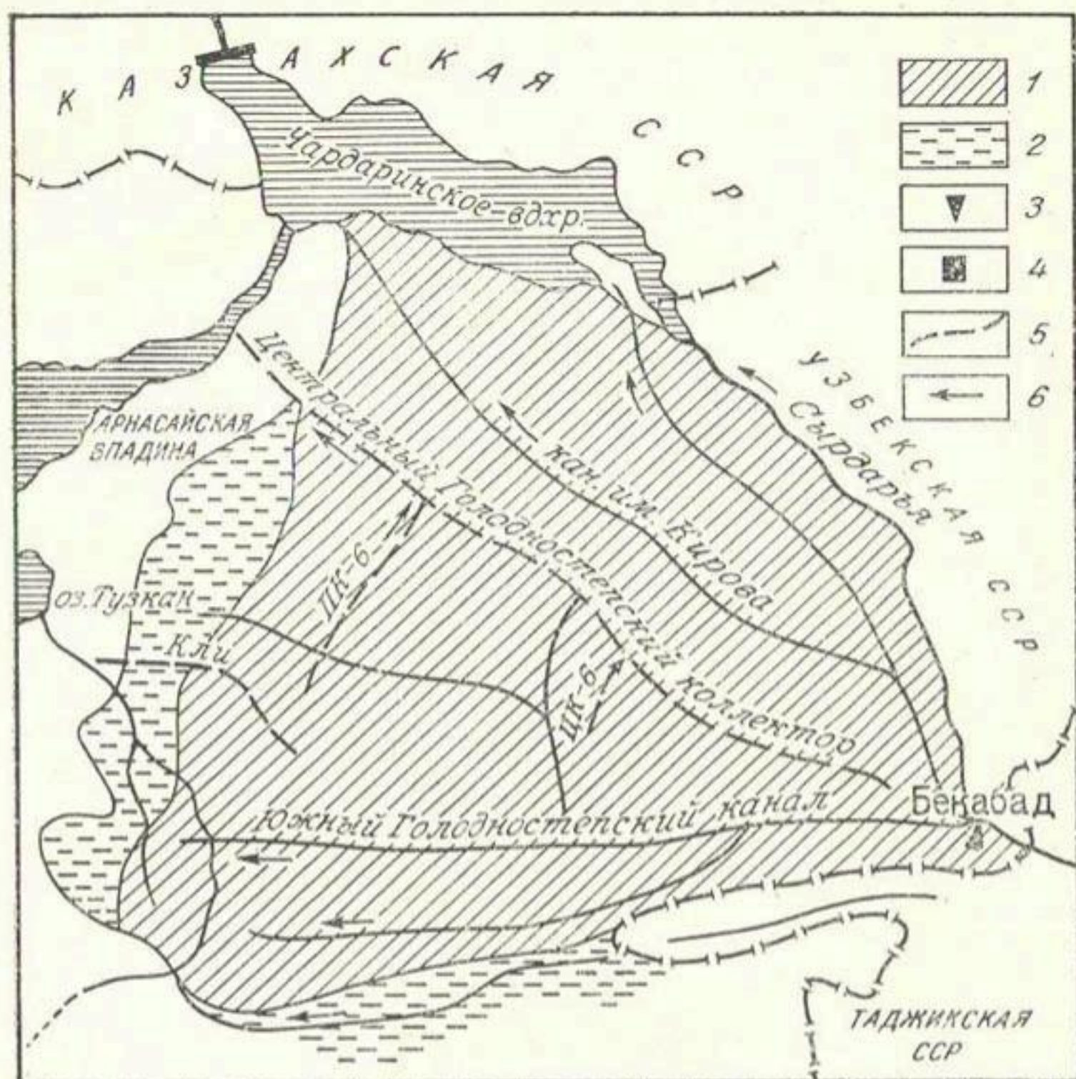
Рис. 16. Голодная степь:
