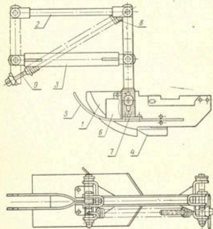
Рис. 9. Сошник сеялки СТВХ-4:
