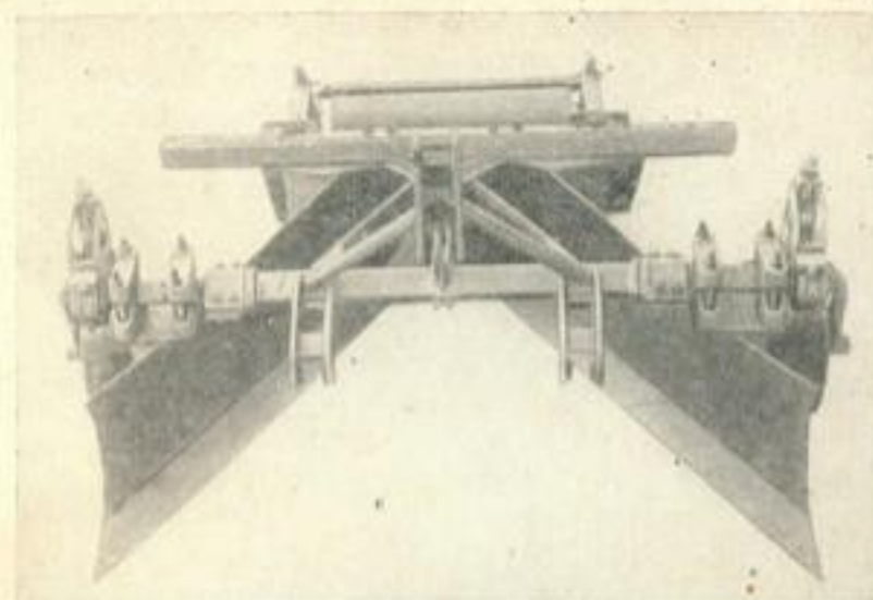
Рис. 33. Канавокопатель-заравниватель универсальный (КЗУ-0,3Б) в варианте валикоделателя (вид спереди).
