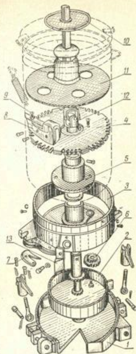
Рис. 10. Высевяющий аппарат сеялки СТВХ-4:
