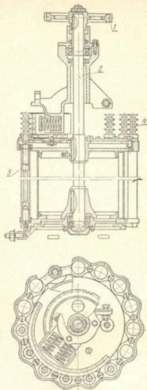
Рис. 22 Шпindelный барабан хлопкоуборочной машины ХВС-1,2: 1 — приводная шестерня; 2 — вал барабана; 3 — шпindel; 4 — приводные ролики шпинделя.
