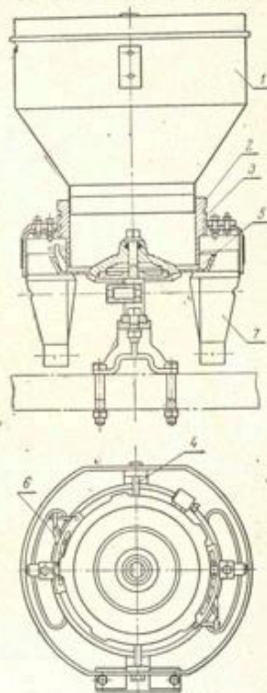
Рис. 16. Культиватор-удобритель НКУ-4-6А:
