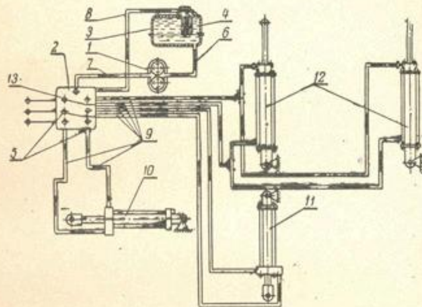
Рис. 27. Гидросистема:
