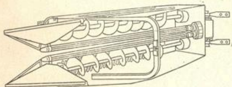
Рис. 30. Рабочий орган машины SKO-4.
