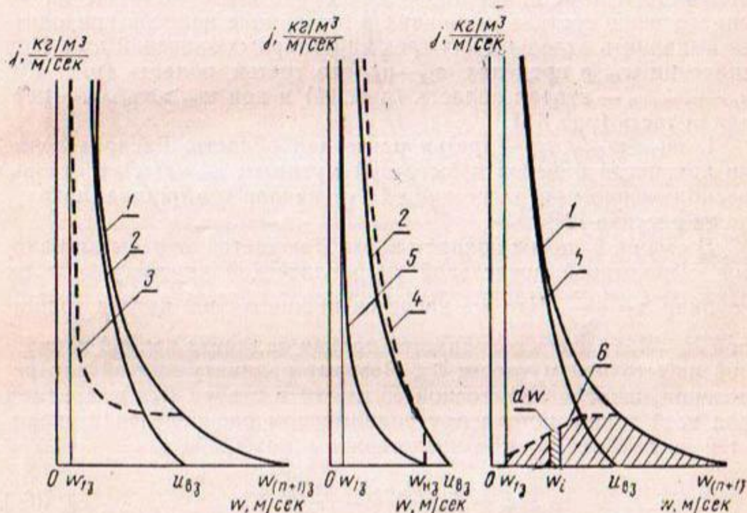
Рис. 13. Кривые распределения по крупности наносов при \omega_{тз} < \omega_{нз} < u_{вз} :
