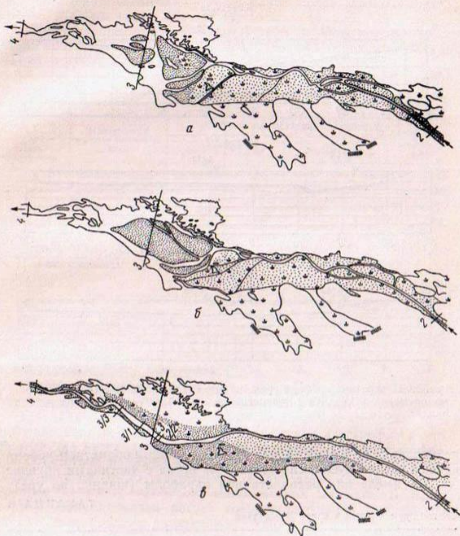
Рис. 49. Динамика заиления озера Двадцатка: а — июнь 1958 г.; б — октябрь 1958 г.; в — июнь 1961 г.
