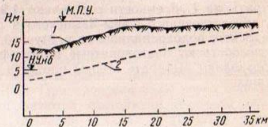
Рис. 47. Продольный профиль Таш-Кепринского водохранилища:
