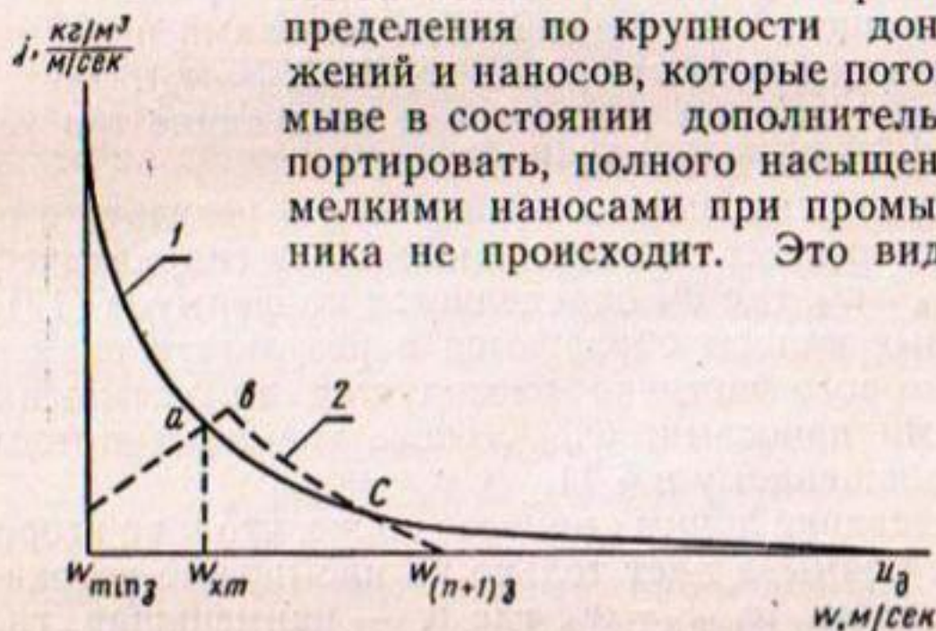
Рис. 20. Кривые распределения по крупности наносов:
