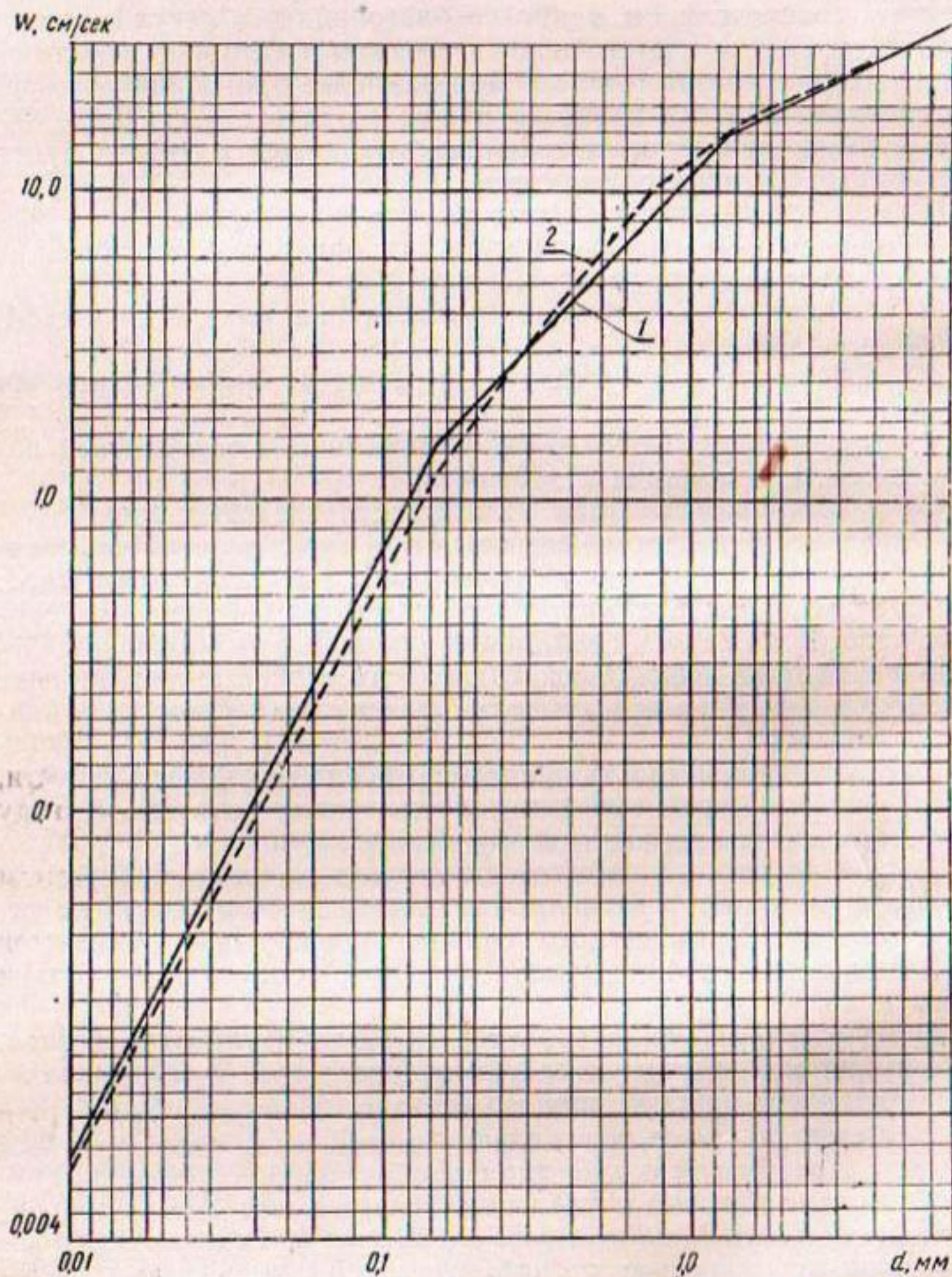
Рис. 11. Кривые зависимости w=f(d) при температуре воды 20^{\circ}\text{C} : 1 — по шкале В. Н. Гончарова; 2 — по шкале А. А. Саркисян.
