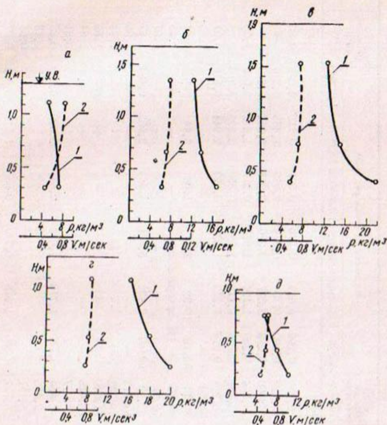
Рис. 33. Распределение по глубине взвешенных наносов и скорость течения воды \rho . Теджен в створе Ауль-Ата, по данным измерений:
