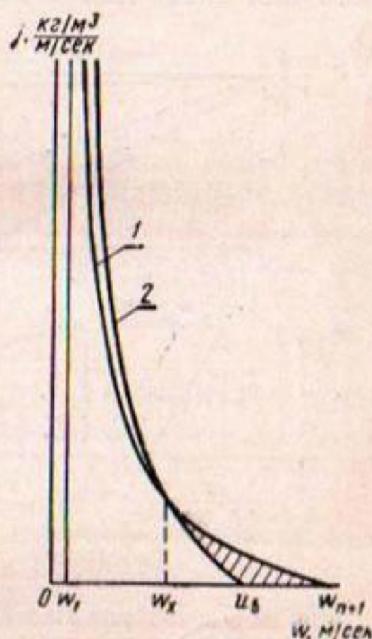
Рис. 3. Кривые зависимости j_0 и j_T от w :
