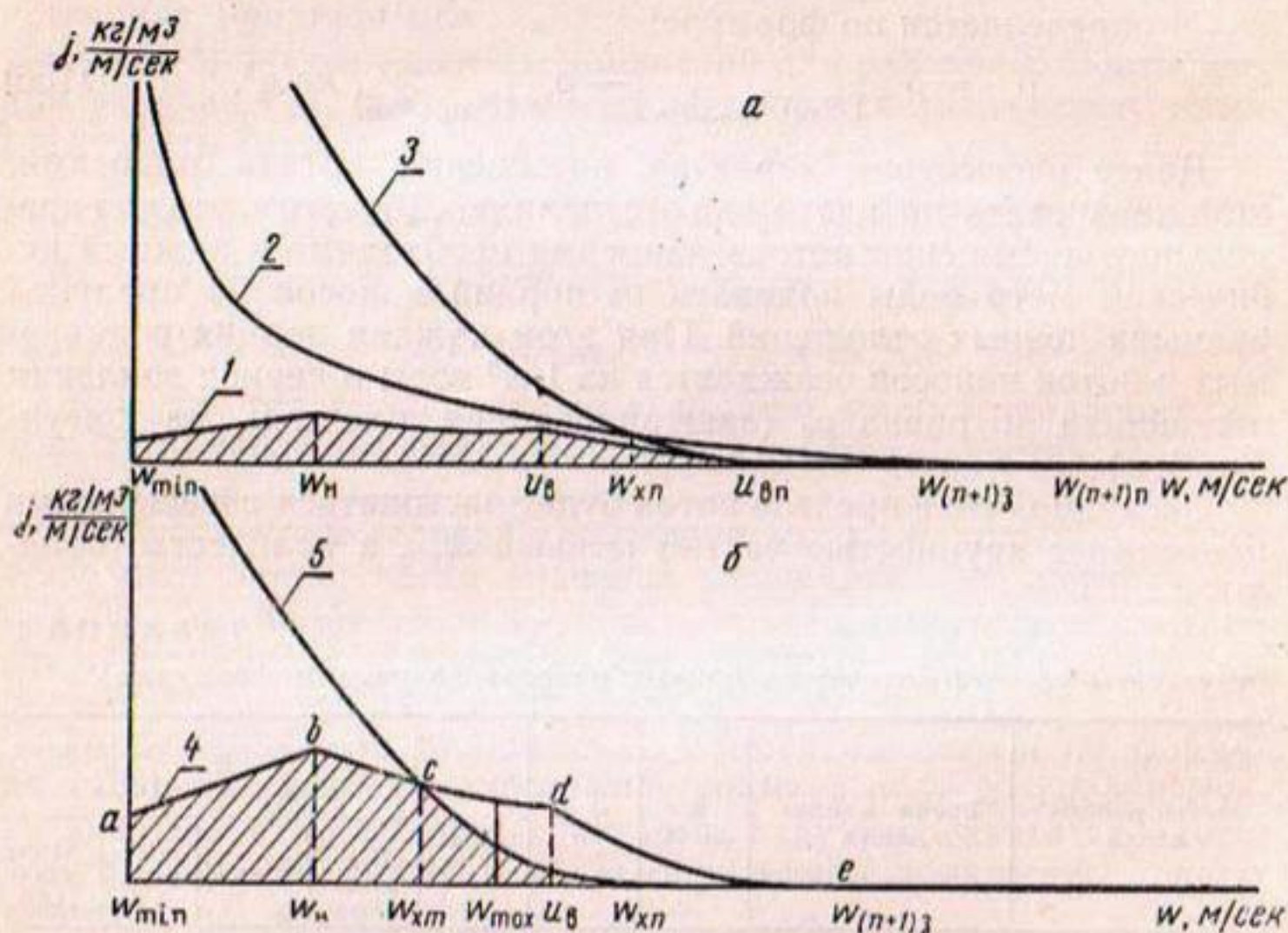
Рис. 21. Кривые распределения наносов при u_{\text{нп}} < w_{(n+1)з} < w_{(n+1)н} :
