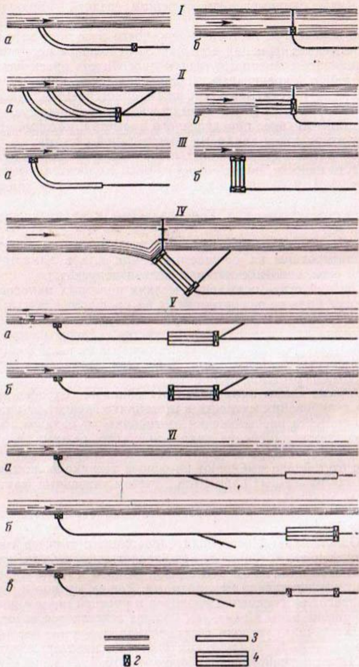
Рис. 10. Схемы расположения отстойников:
