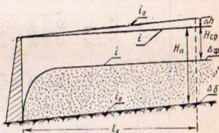
Рис. 41. Схематический продольный разрез заиленного водохранилища.
