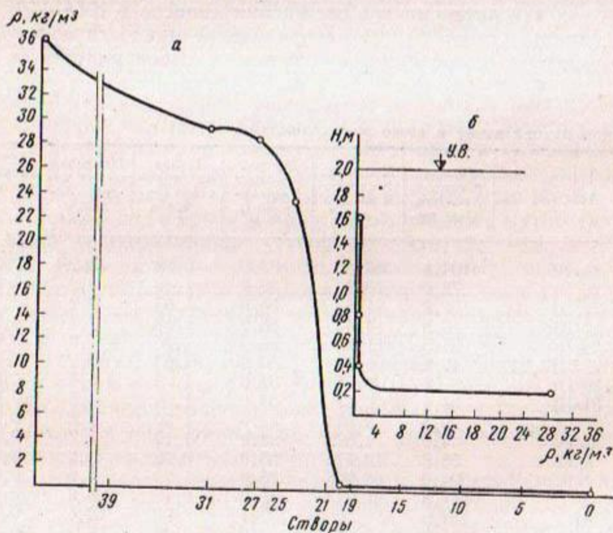
Рис. 29. Изменение мутности на участке Ауль-Ата — Тедженстрой и распределение мутности по глубине потока за 15/V 1962 г.:
