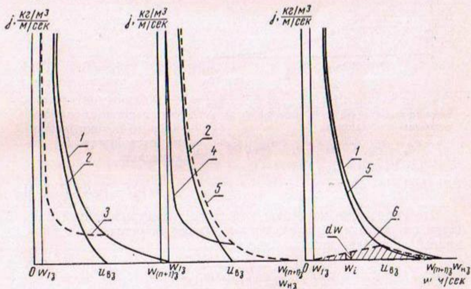
Рис. 15. Кривые распределения по крупности наносов при w_{(n+1)3} < w_{n3} :
