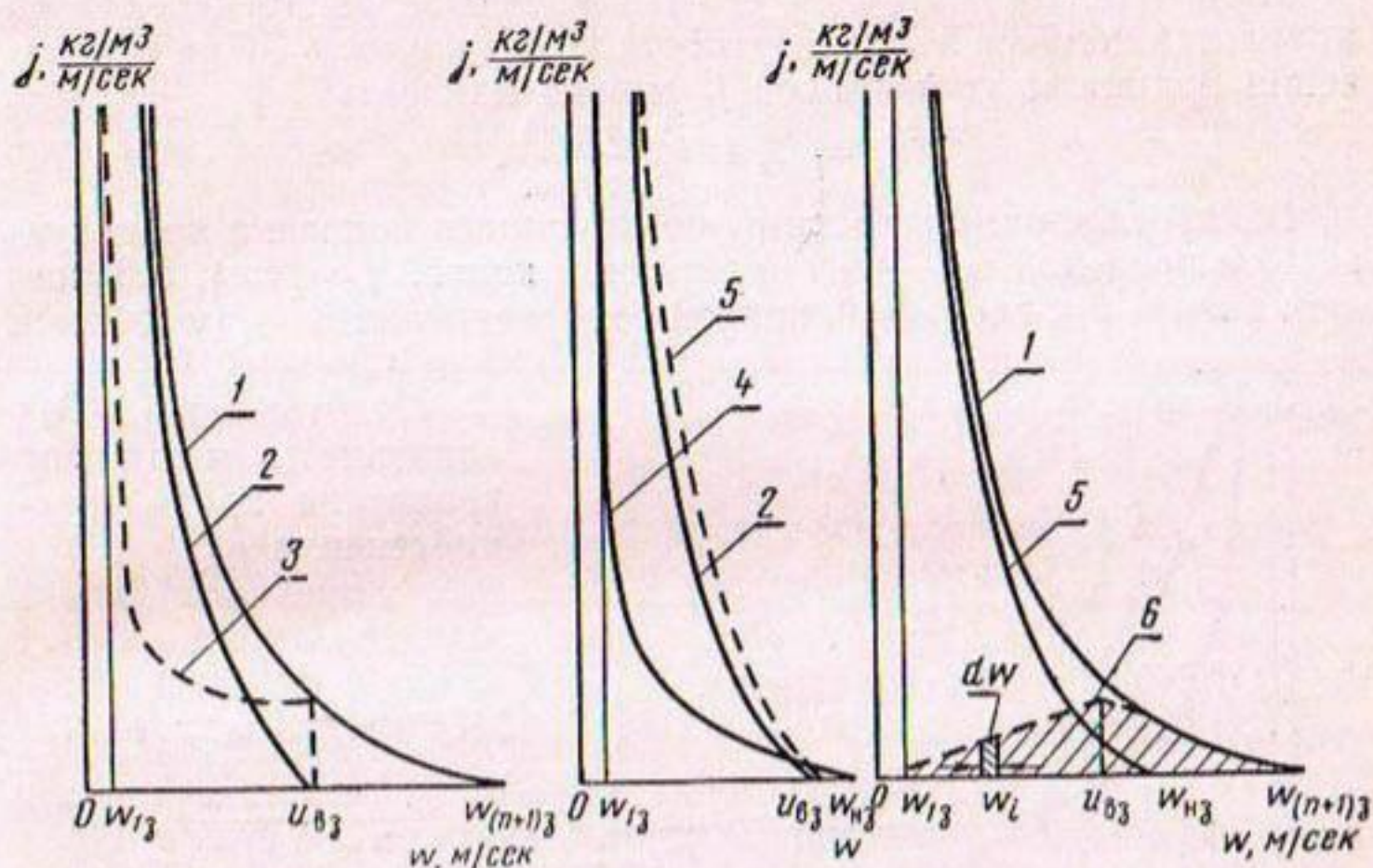
Рис. 14. Кривые распределения по крупности наносов при u_{03} < w_{n3} < w_{(n+1)3} :
