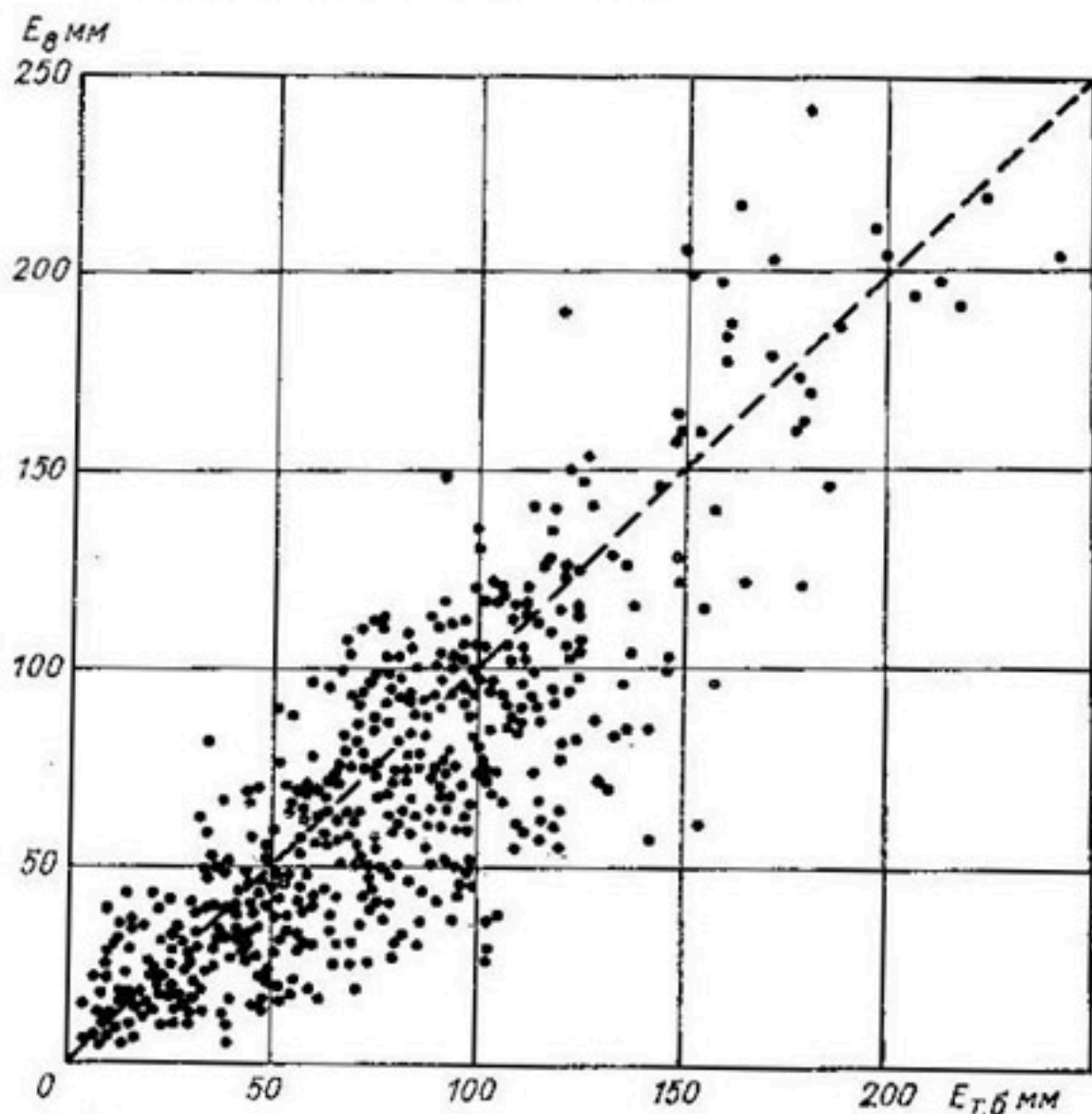
Рис. 46. Связь рассчитанных величин суммарного испарения E_{с} с измеренными E_{т, с} .
