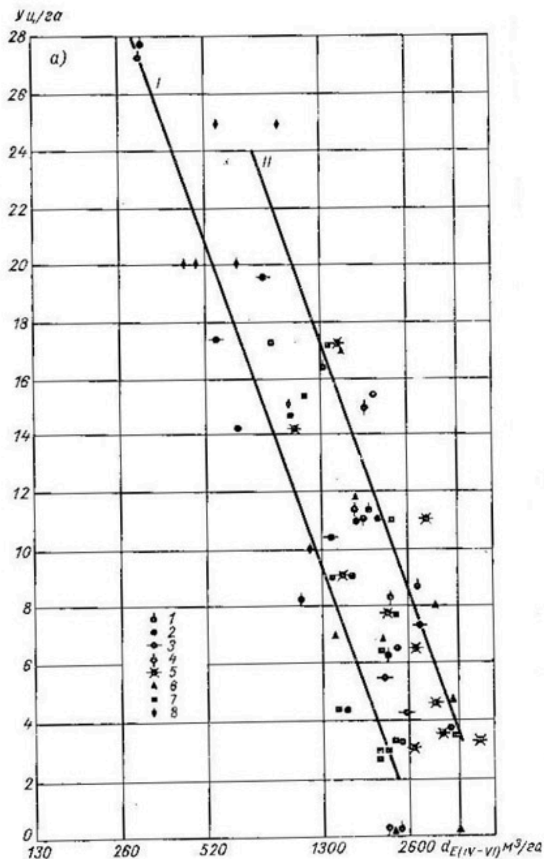
Рис. 99. Территориально общие зависимости урожая озимой (а) потребления d_E для отдельных физико-географических и ме I — север Ростовской области, юг Воронежской и Волгоградской обла- пинск, 4 — Золотое, 5 — Новоузенск, 6 — Арчеда, 7 — Орлов Гай, 8 — 2 — Пенза, 3 — Кузнецк, 5 — Апенково, 6 — Мелексс, 7 — Безво- ное Поселение, 9 — Большая Глуши
