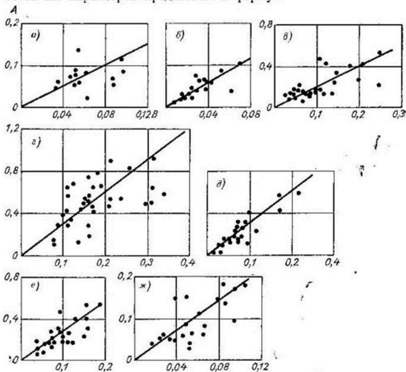
Рис. 40. Зависимости отношения A = \frac{E}{2W_{\text{н.з.}} + X + M - Y_{\text{п.з.}} - E - K - I} от величины B = \frac{E_0}{2\gamma} для определения параметра \beta , построенные по данным наблюдений ДГМО, Нижнедевицкой, Придеснянской и Кустапайской стокowych станций, агрометстанций «Гигант», Елшанки для колосовых сельскохозяйственных культур.
