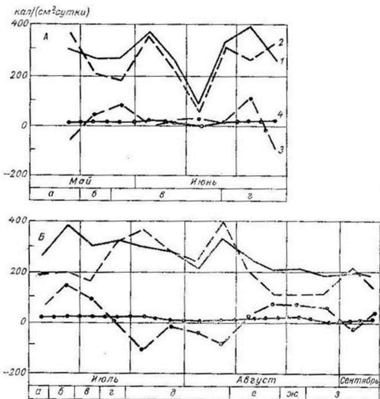
Рис. 29. Графики хода среднепятнадных величин составляющих теплового баланса на полях, занятых озимой пшеницей (А) и кукурузой (Б). Свх «Изобильненский», Ставропольского края, 1966 г.
