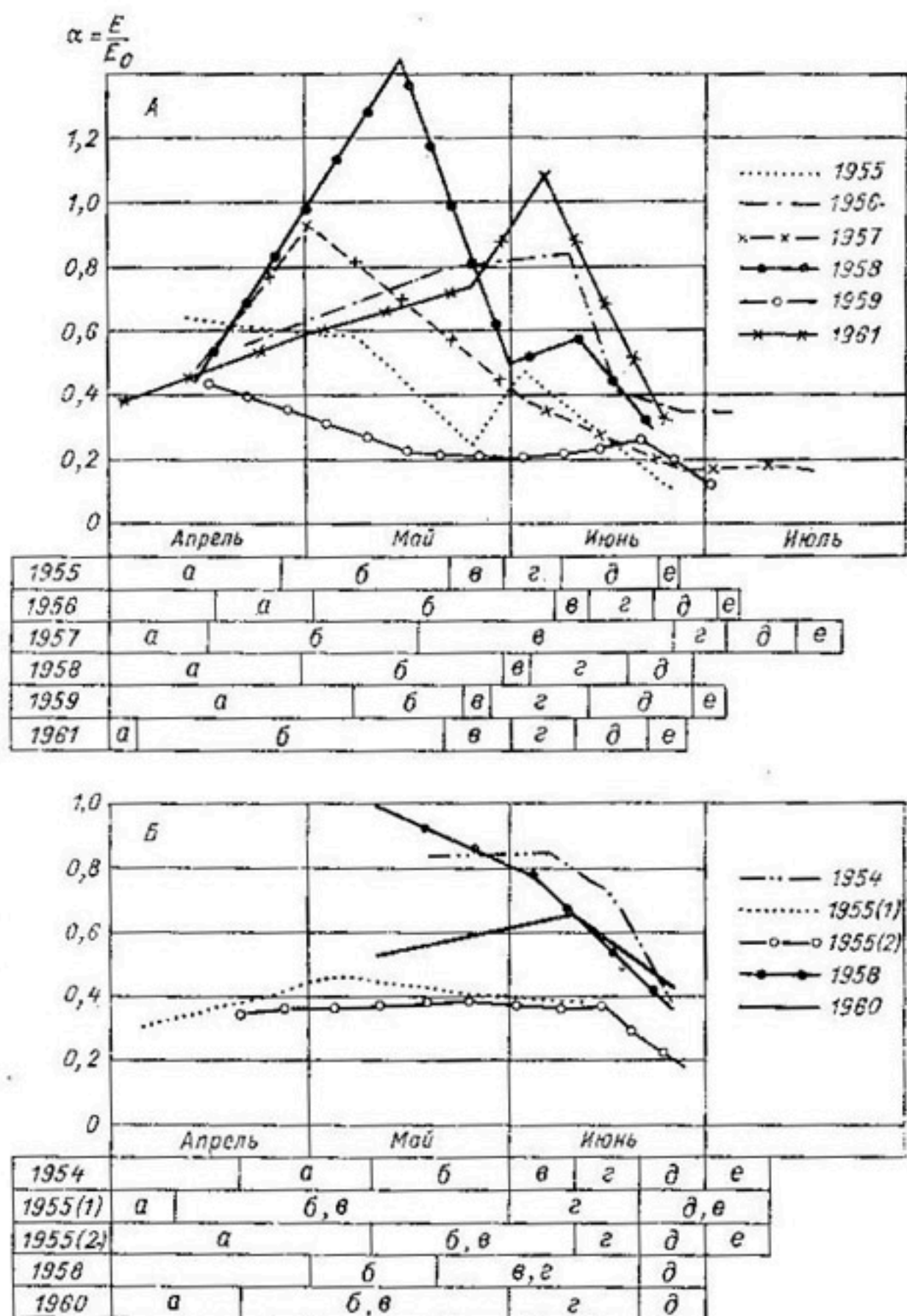
Рис. 38. Графики изменения во времени параметра \alpha в различные А — ДГМО (озимая пшеница); Б — агрометстанция «Гигант» (озимая пшеница); ская стоковая станция (озимая пшеница); 1958, 1961 гг.; Г — подбалансовый пункт (яровая пшеница); 1962 (2), 1963 гг. Фазы развития растений: а — возобновление неге колосение (или вымывание метелки для риса); в — колосение (или вымывание спелость — носками спелость; е —
