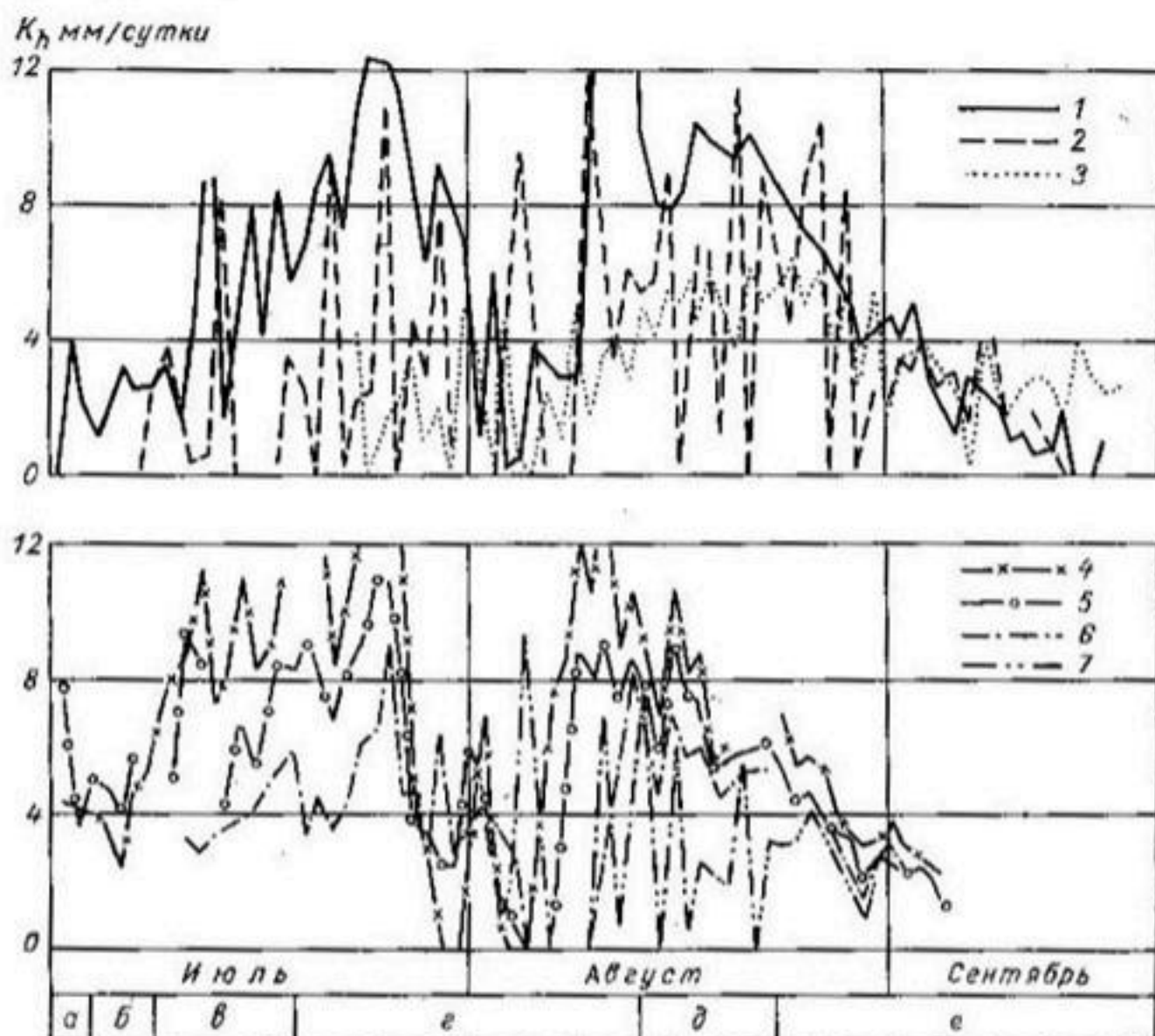
Рис. 53. График хода интенсивности расхода грунтовых вод в зону аэрации при различных глубинах их залегания. Кукуруза, свх «Изобильненский», Ставропольского края, 1966 г.
