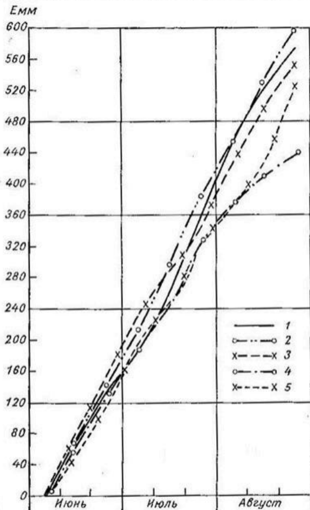
Рис. 26. Интегральные кривые суммарного испарения с риса. 1 — 1958 г., 2 — 1959 г., 3 — 1961 г., 4 — 1964 г., 5 — 1965 г.
