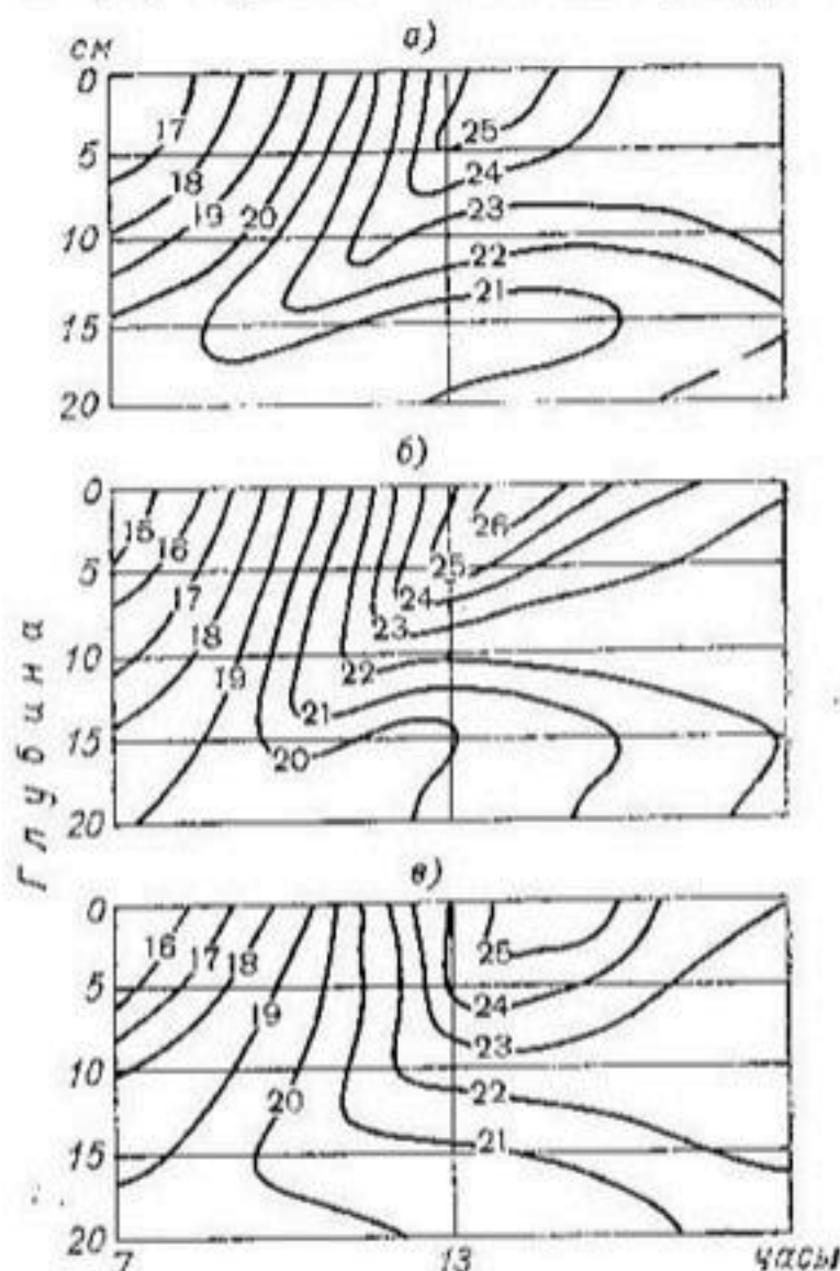
Рис. 13. Термоизоплеты суточного хода температуры почвы в поле, засеянном гречихой, и в монолитах лизиметров. Заволжская опытно-мелиоративная станция, 1966 г.
