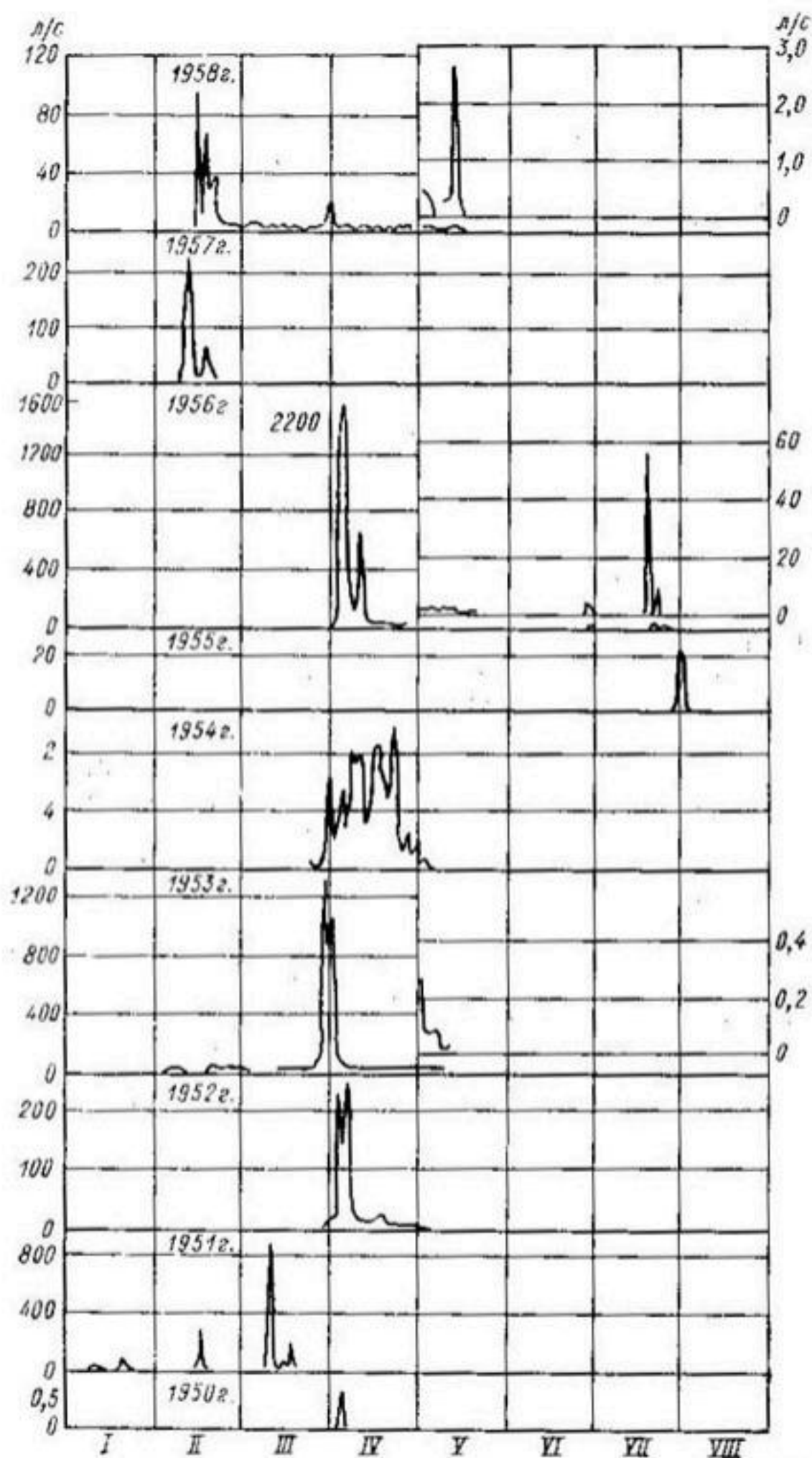
Рис. 58. Гидрографы стока балки Бузиповки у гидроствора № 1. (С сентября по декабрь 1950—1958 гг. сток фактически отсутствовал.)
