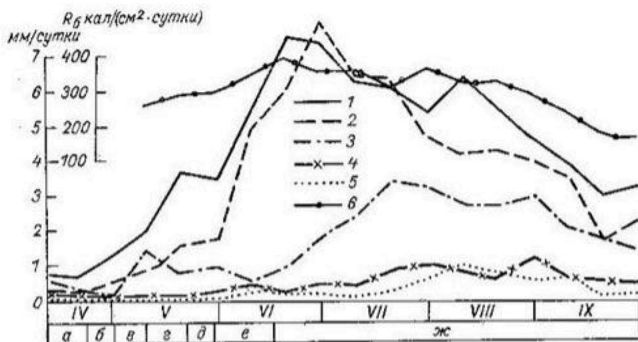
Рис. 52. Хронологический график величины расхода влаги в зону аэрации на поле с сахарной свеклой и радиационного баланса (осредненные за четыре года). Таласский орошаемый массив, пос. Новоипановка, 1967—1970 гг.
