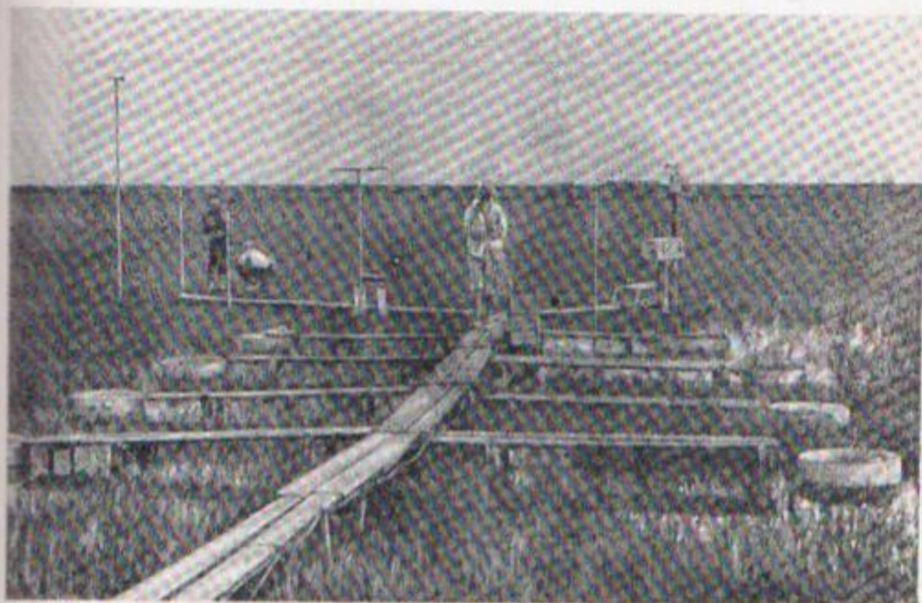
Рис. 22. Общий вид экспериментальной тепловоднобалансовой площадки на рисовом поле.
