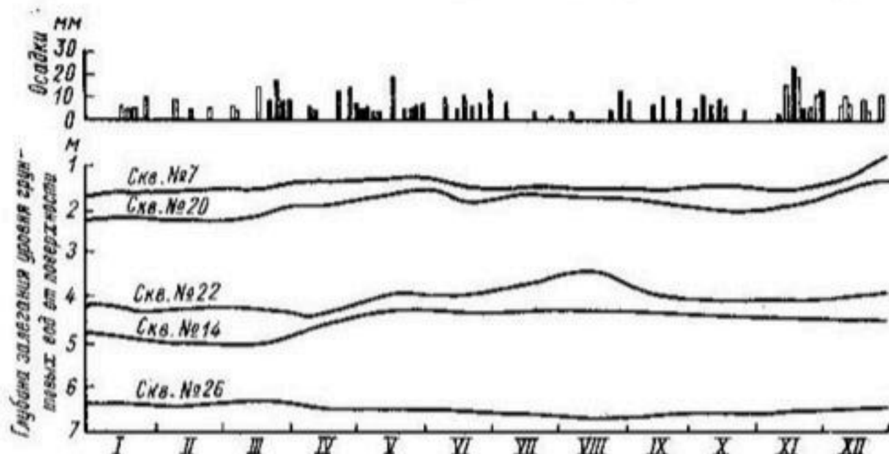
Рис. 60. Изменение уровней грунтовых вод на различных глубинах (под воздействием инфильтрации талых, дождевых и поливных вод). Рыбиче-Задонский поднобалансовый участок Нижнедонской оросительной системы, 1961 г.
