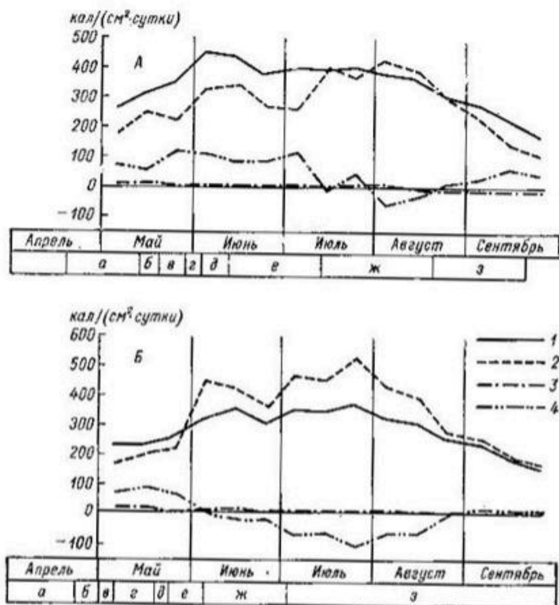
Рис. 31. Графики хода среднепентадных величин составляющих теплового баланса на полях Арысь-Туркестанского массива, занятых хлопчатником (А), и Таласского орошаемого массива, занятых сахарной свеклой (Б), 1968 г.
