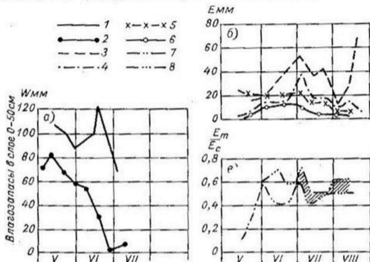
Рис. 21. График хода по времени элементов водного баланса на орошаемых и неорошаемых землях на кукурузном поле. Пос. Восход., Ростовской области, 1957 г.
