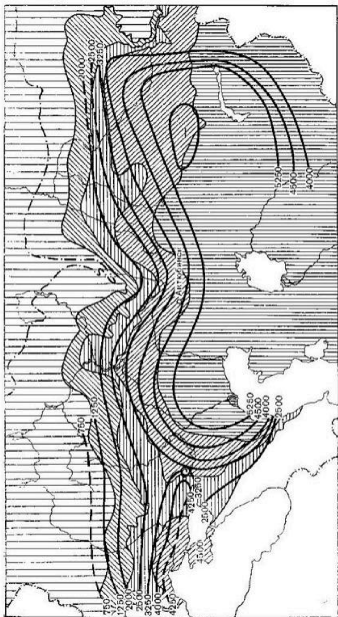
Рис. 88. Схематическая карта изолиний среднеемноголетних величин недостатка водопотребления кукурузы за период вегетации
