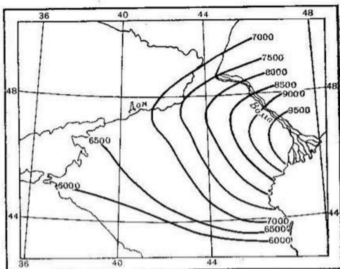
Рис. 90. Схематическая карта изолиний среднегодовых величин недостатка водопотребления риса за период вегетации.
