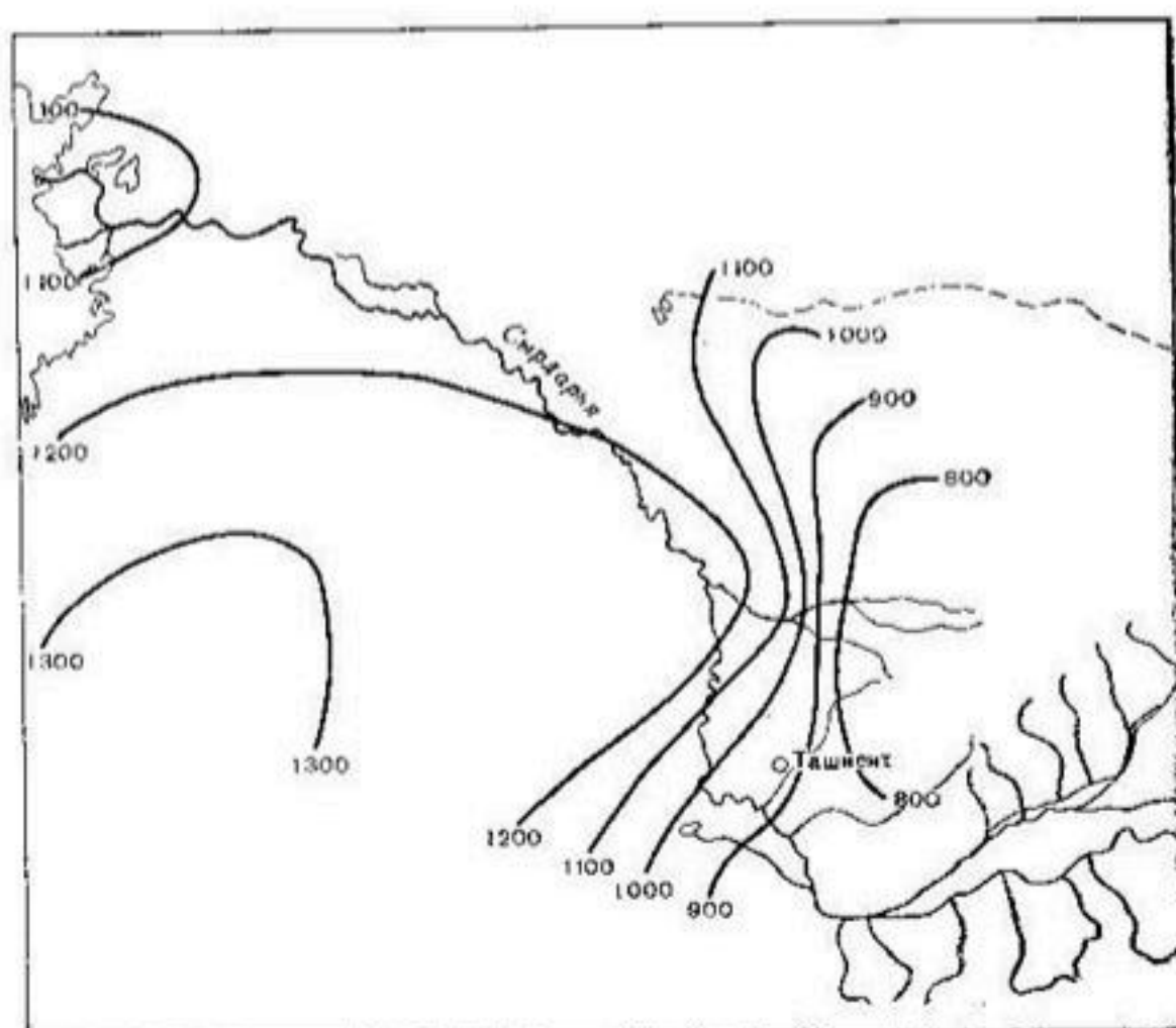
Рис. 91. Среднегодовые величины недостатков водопотребления за период вегетации хлопчатника (мм).
