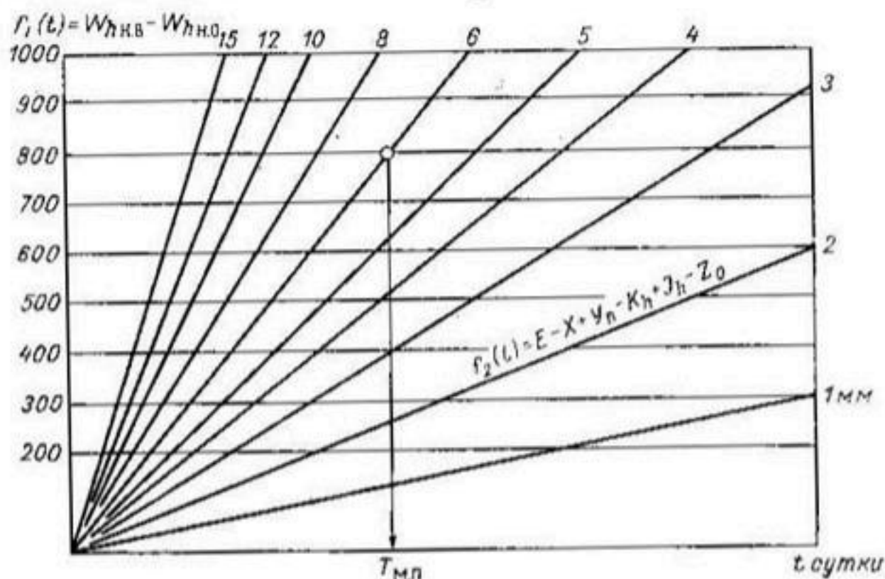
Рис. 105. Номограмма для определения продолжительности межполивного периода T_{м.п} и корректировки сроков полива для оросительных систем Ростовской и Волгоградской областей и Северного Кавказа.
