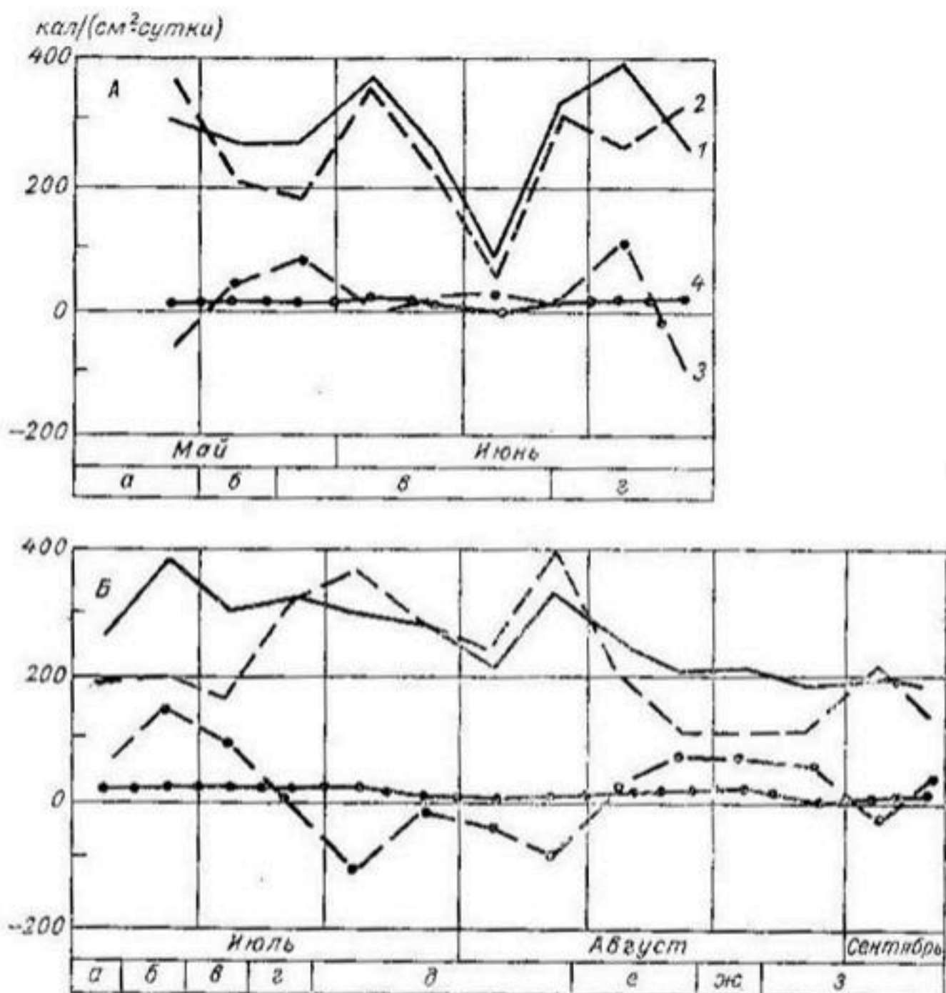
Рис. 29. Графики хода средиепентадных величин составляющих теплового баланса на полях, занятых озимой пшеницей (А) и кукурузой (Б). Свх «Изобильненский», Ставропольского края, 1966 г.
