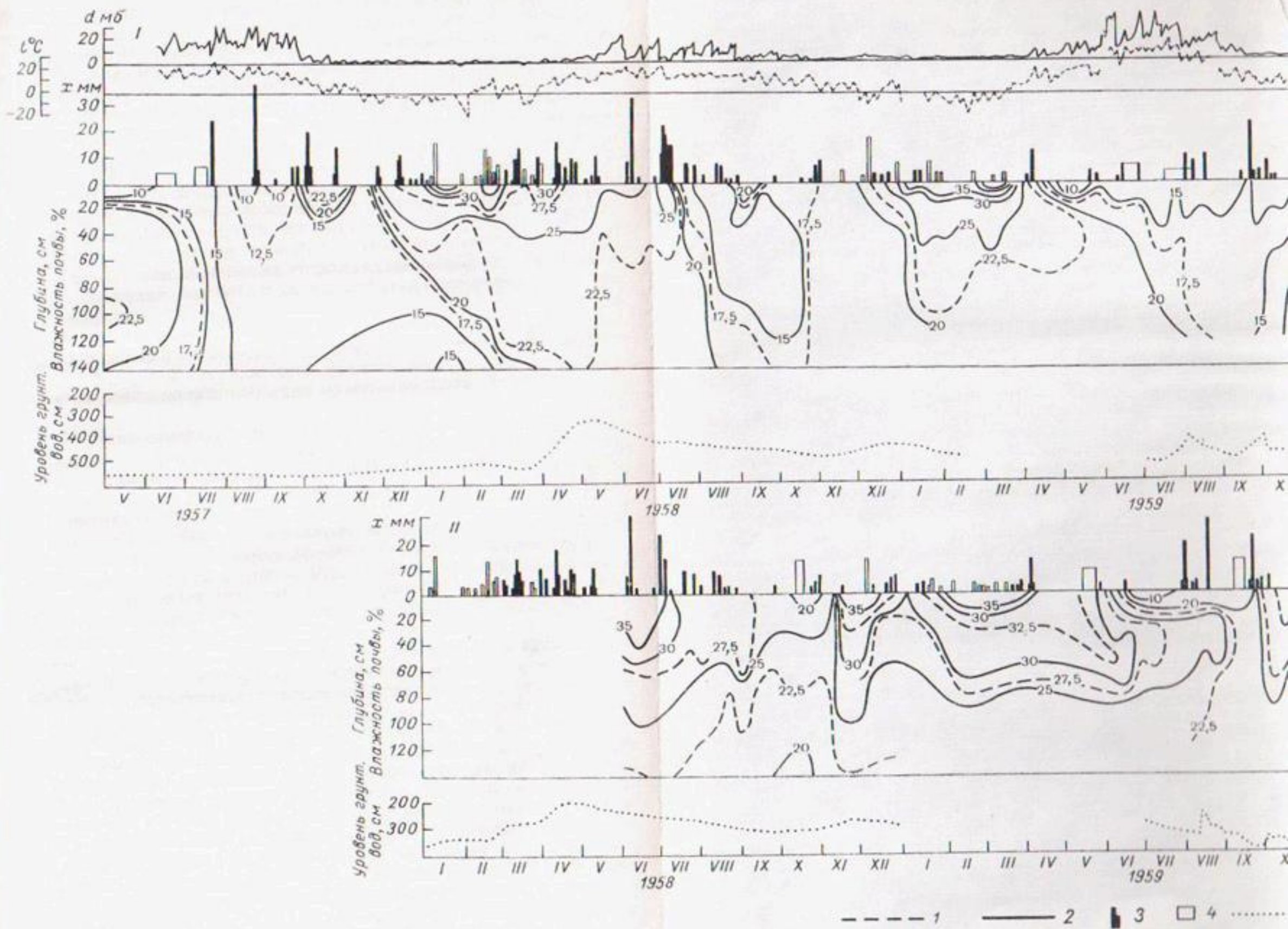
Рис. 107. Хроноизоплеты влажности суглинчатых почво-грунтов на полях I и II, а также ход температуры (I) и дефицита влажности воздуха (II), режим осадков (3),
