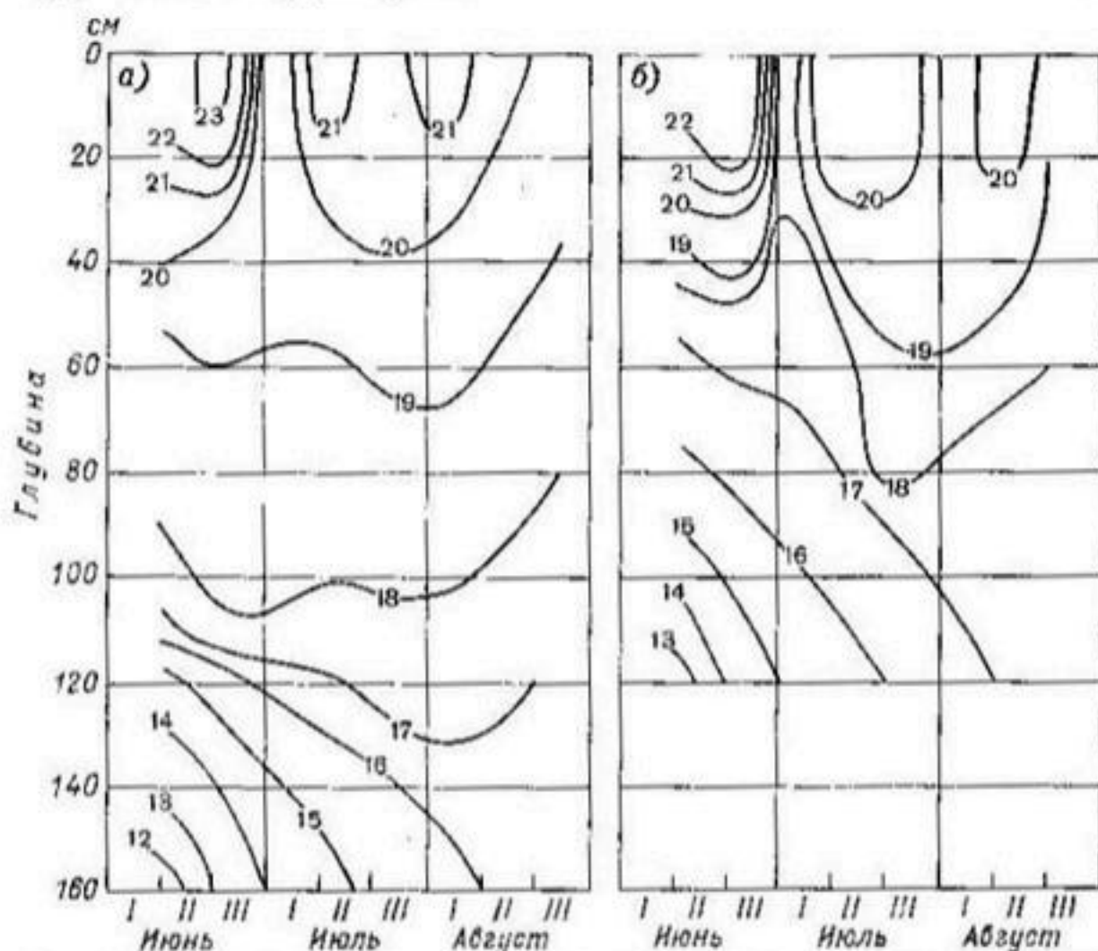
Рис. 14. Термонизоплеты в монолите лизиметра с глубиной залегания грунтовых под 2,0 м (а) и в поле (б). Заволжская опытно-мелиоративная станция, 1969 г.
