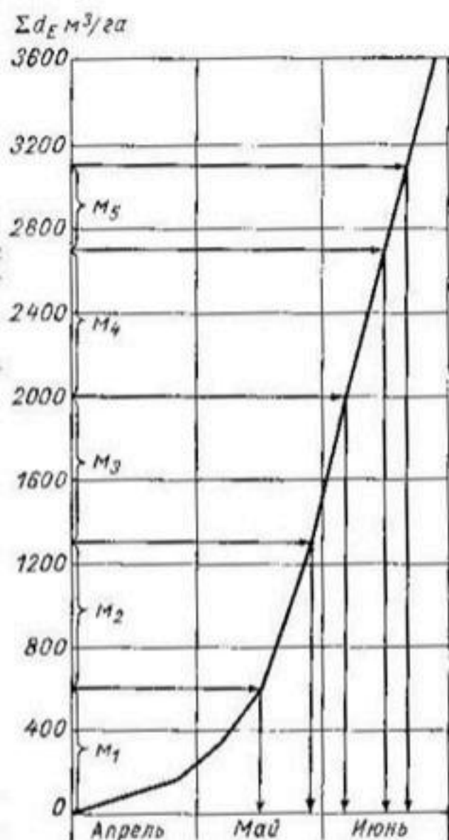
Рис. 104. Интегральная кривая декадных величин недостатков водопотребления озимой пшеницы на агрометстанции «Зимовники» (Ростовская область, 1950 г.) и схема определения сроков полива.
