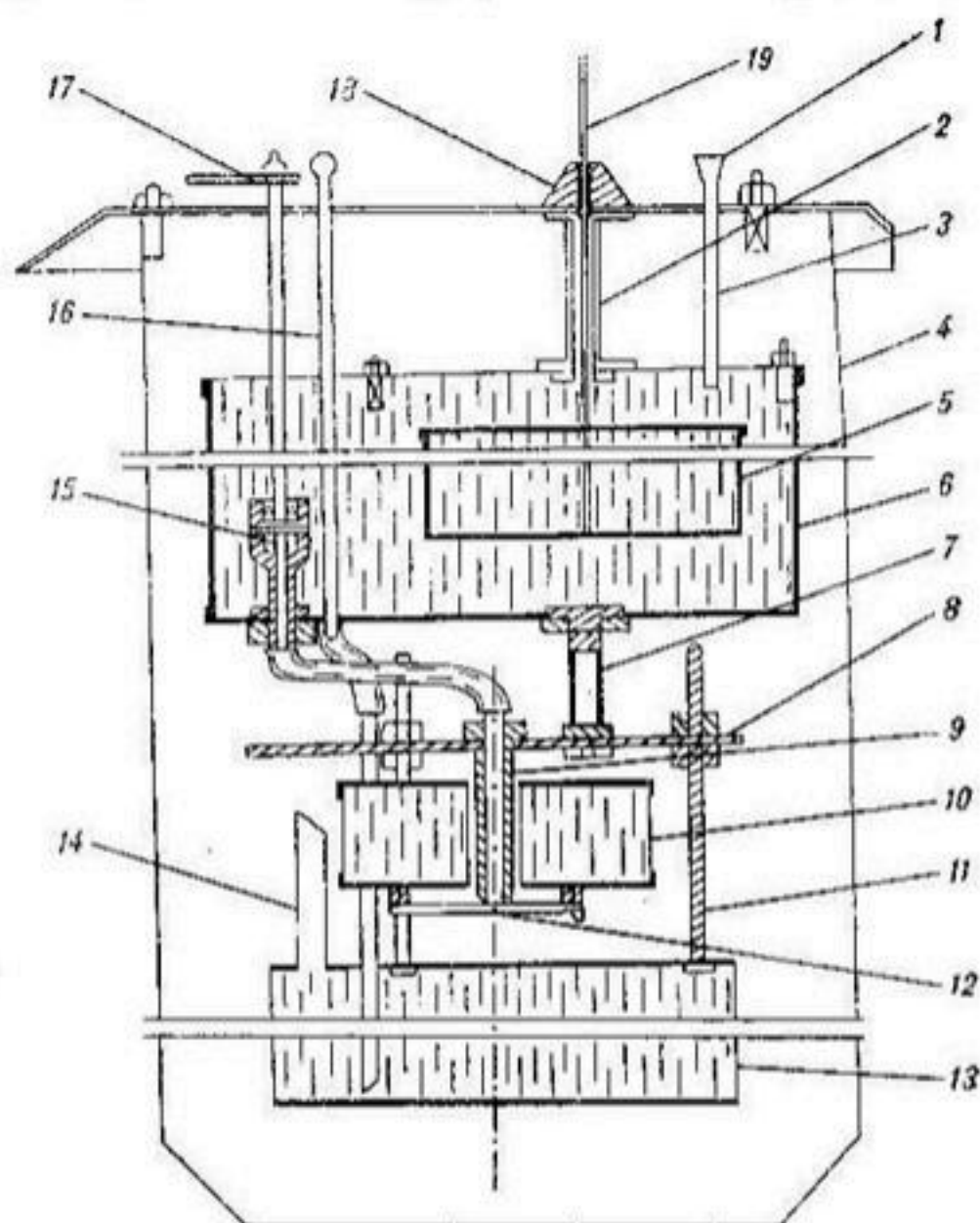
Рис. 11. Схематический разрез водорегулирующего устройства.
