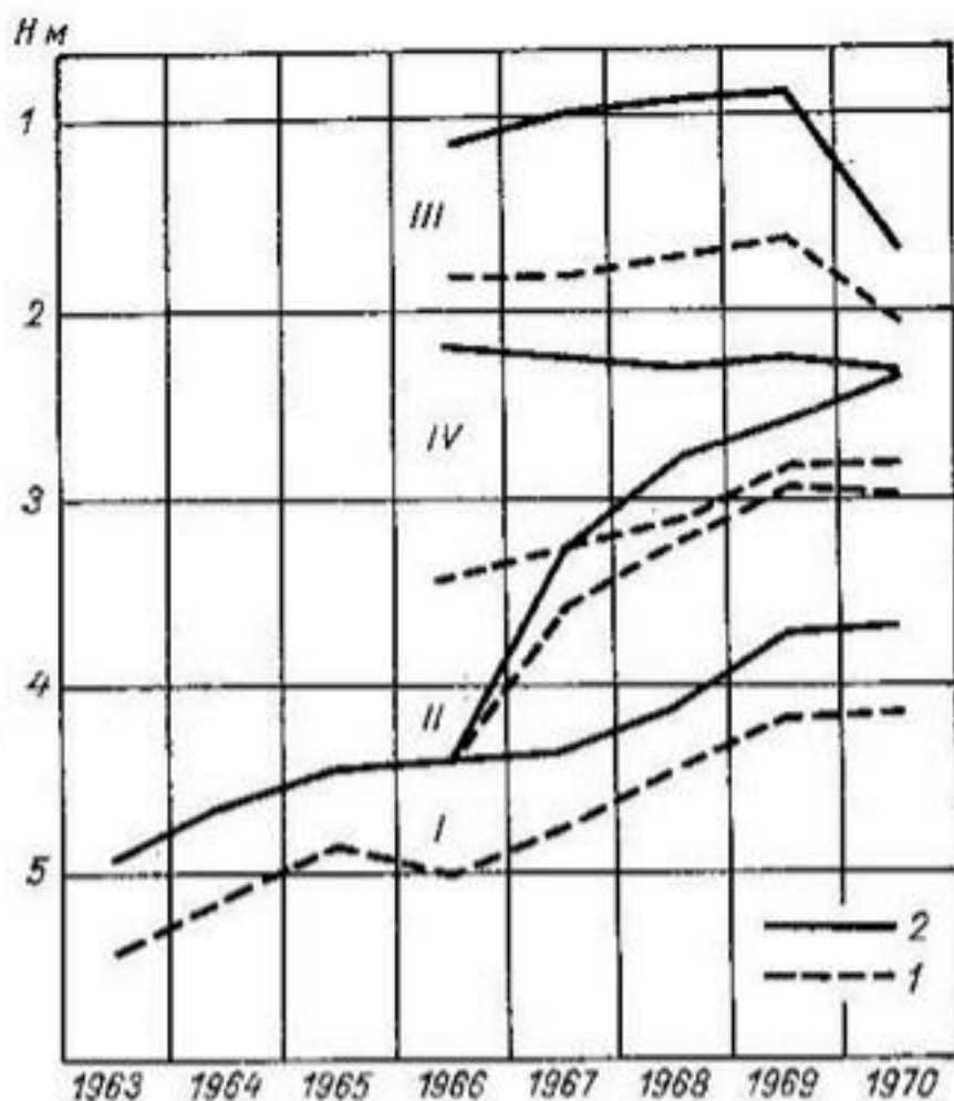
Рис. 68. Изменение максимальных (1) и минимальных (2) уровней грунтовых вод на различных участках Арысь-Туркестанской оросительной системы. Участки: I — междуречье Бугунь—Чаян; II — междуречье Чаян—Мынбулак; III — Мынбулак—Икансу; IV — Икансу—Чага.
