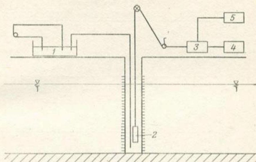
Рис. 4.2.1. Схема установки для запуска трассерной волны.
