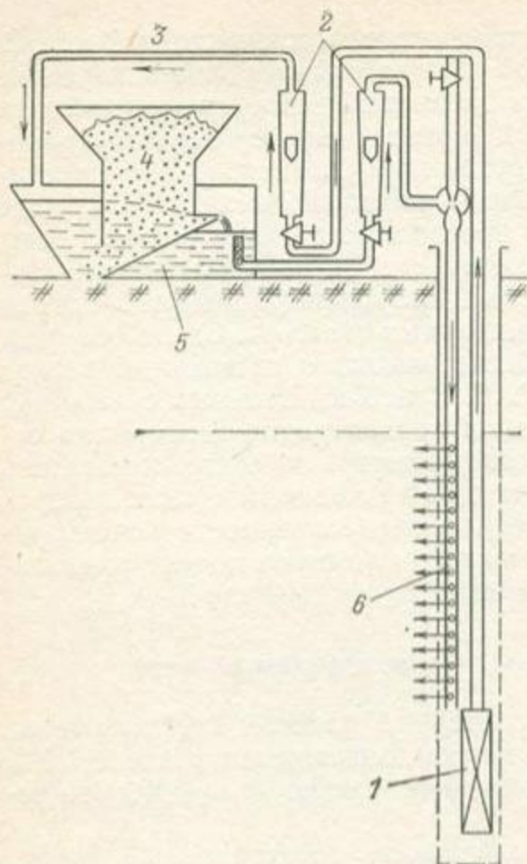
Рис. 4.2.18. Одоскважинный геозлектрический метод: устройство для запуска трассера.
