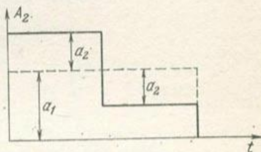
Рис. 5.4.2. Импульсная переходная характеристика
