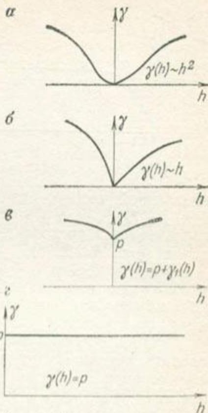
Рис. 7.2.1
