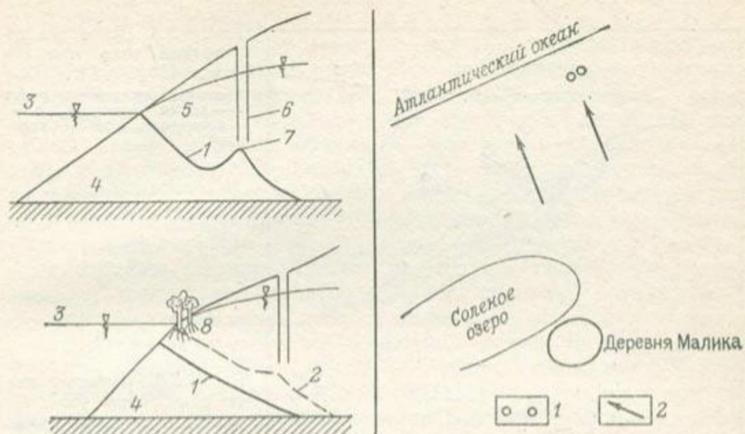
Рис. 6.3.1. Внедрение соленой воды в прибрежный водоносный горизонт. 1 — до откачки; 2 — после откачки; 3 — море; 4 — соленый «язык»; 5 — водоносный горизонт; 6 — откачивающая скважина; 7 — образование конуса; 8 — корни
