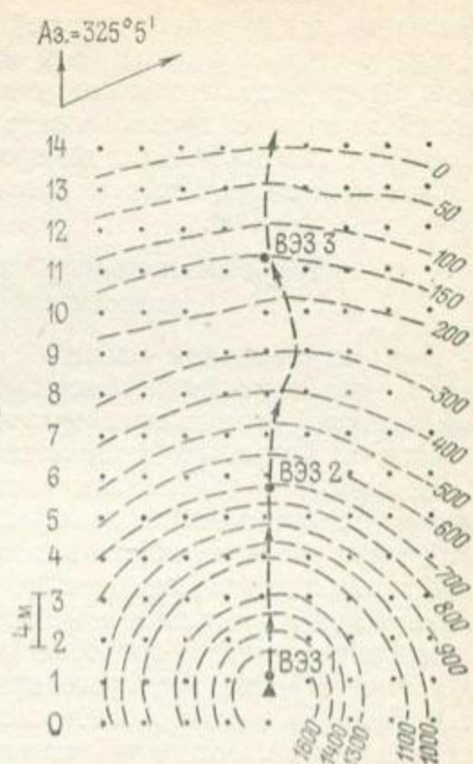
Рис. 4.2.29. План распределения электрических потенциалов. Условные обозначения аналогичны рис. 4.2.28
