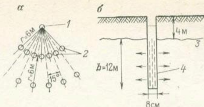
Рис. 4.2.15. План расположения (а) и конструкция (б) скважины при проведении многоскважинного эксперимента в рейнском водоносном горизонте.
