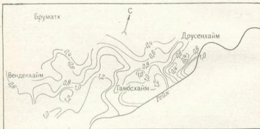
Рис. 4.3.2. План распределения проводимости (в 10^{-1} м²/с) [71]
