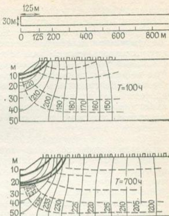
Рис. 6.1.15. Рассчитанная интрузия соленых вод для 1975 г.
