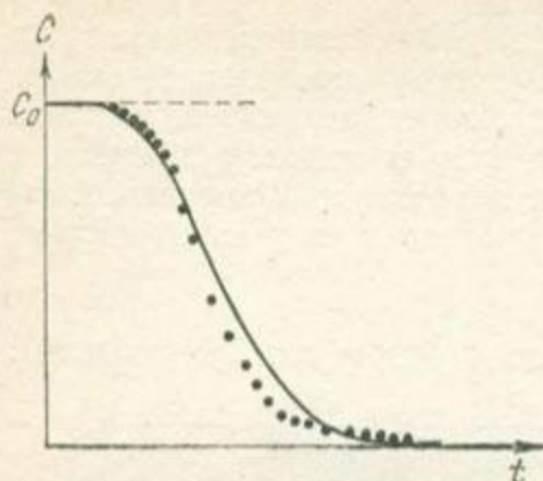
Рис. 2.3.1. Сравнение расчетной кривой Шейдггера с экспериментальными результатами
