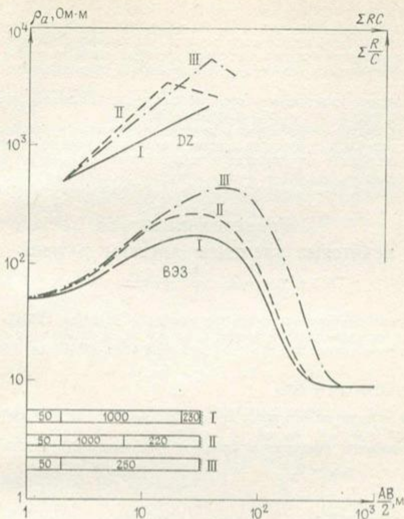
П.2.8. Кривые электрического зондирования (ВЭЗ) и кривые суммарного сопротивления (DZ).
