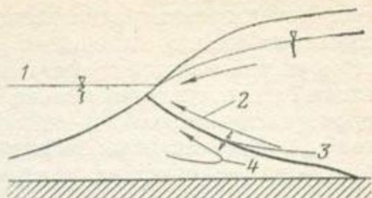
Рис. 6.3.6. Обратная дисперсия при движении пресной воды к морю.
