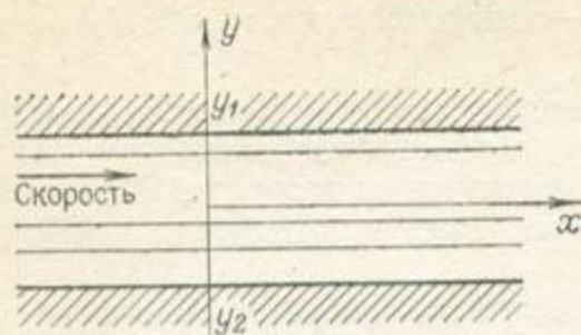
Рис. 2.5.1. Система координат
