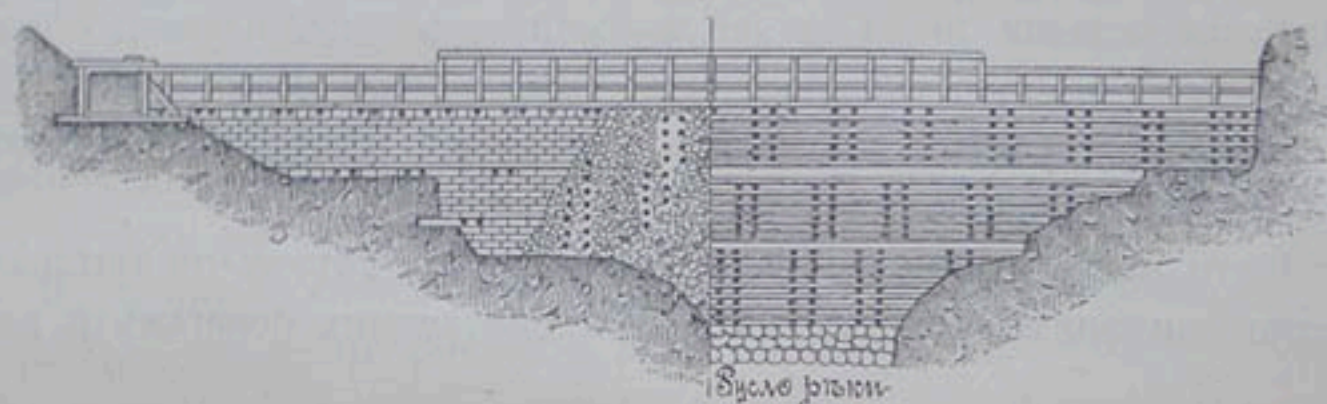
Черт. 22. — Продольное сѣченіе.
