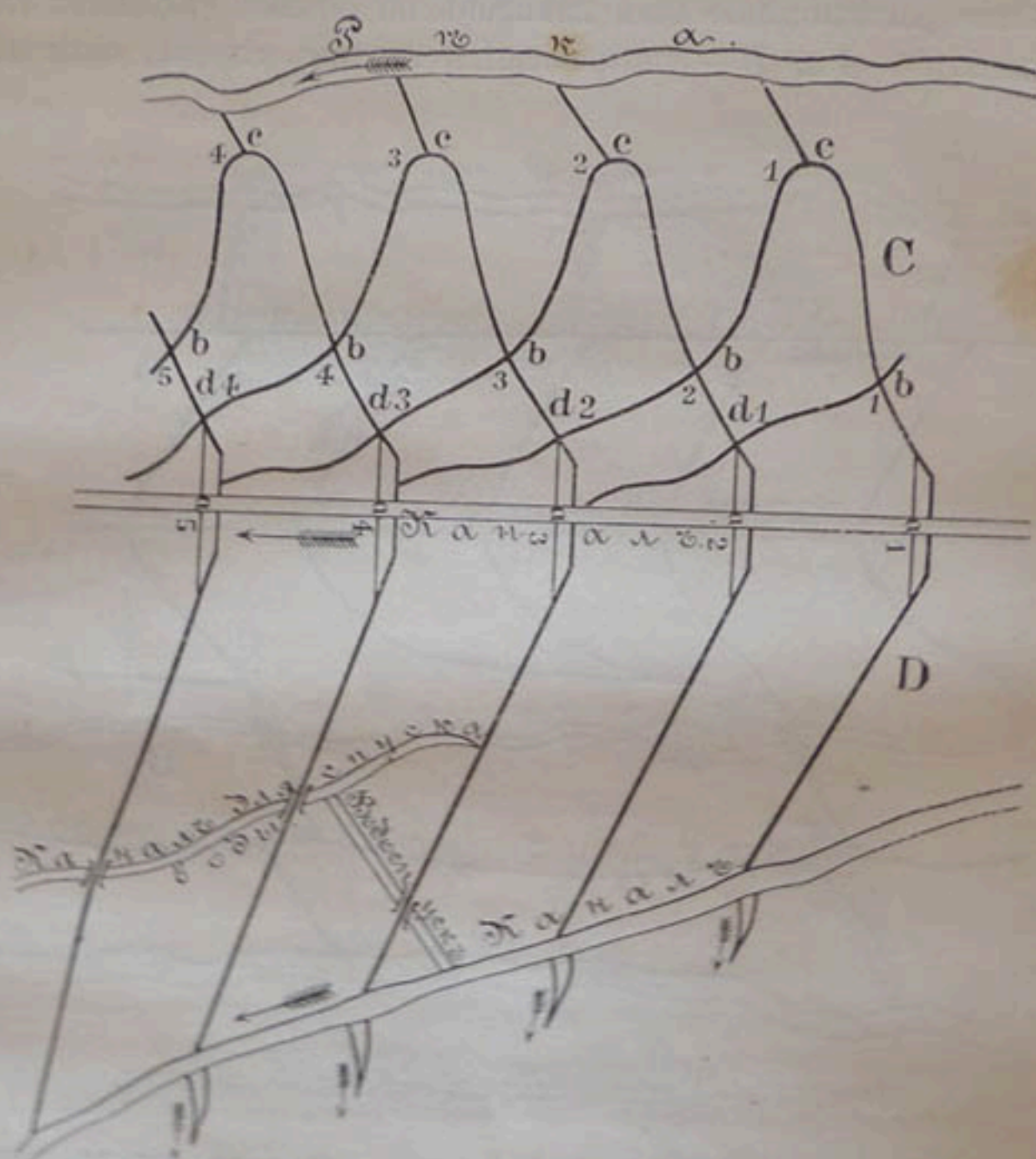
Черт. 148. — Планъ распределительной системы.
