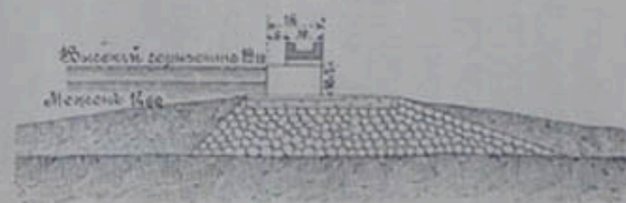
Черт. 34. — Поперечное сѣченіе по АВ.
