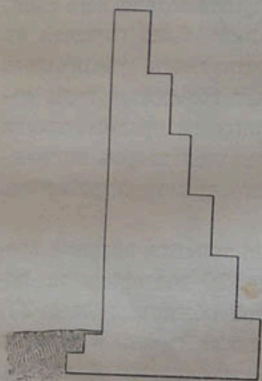
Черт. 140. — Поперечное сѣченіе подпорной стѣнки.
