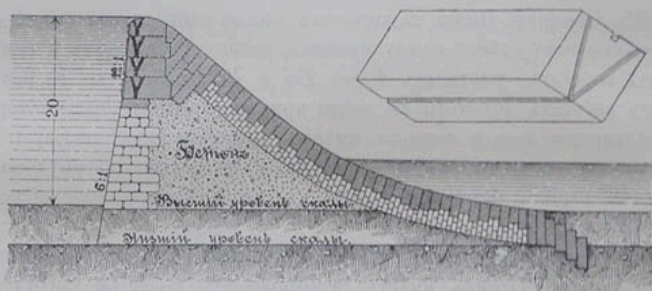
Черт. 46. — Плотина канала Хенаресь.
