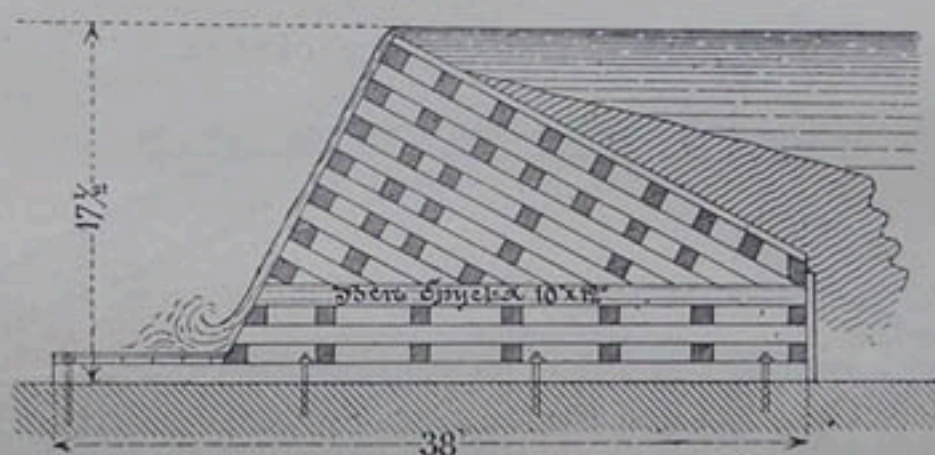
Черт. 21. — Поперечное сѣченіе плотины на р. Беар.
