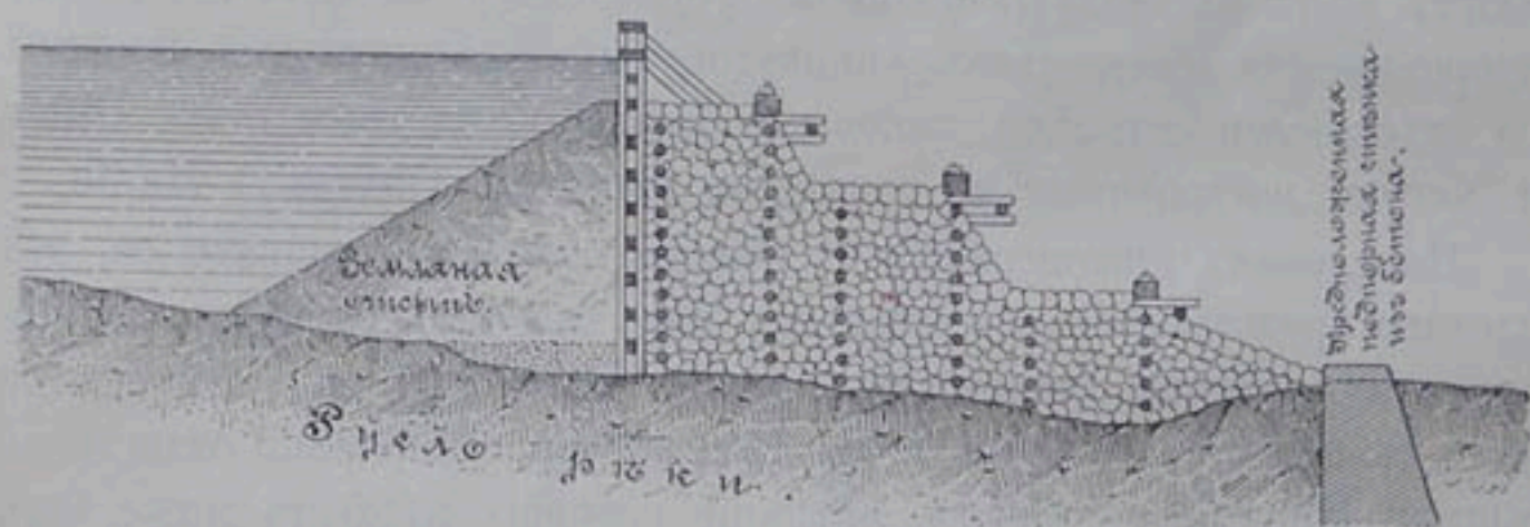
Черт. 24. — Сѣченіе по срединѣ ряжей.
