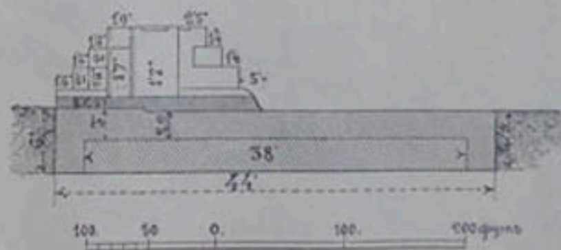
Черт. 30. — Сѣченіе по срединѣ пролета и боковой видъ быка.
