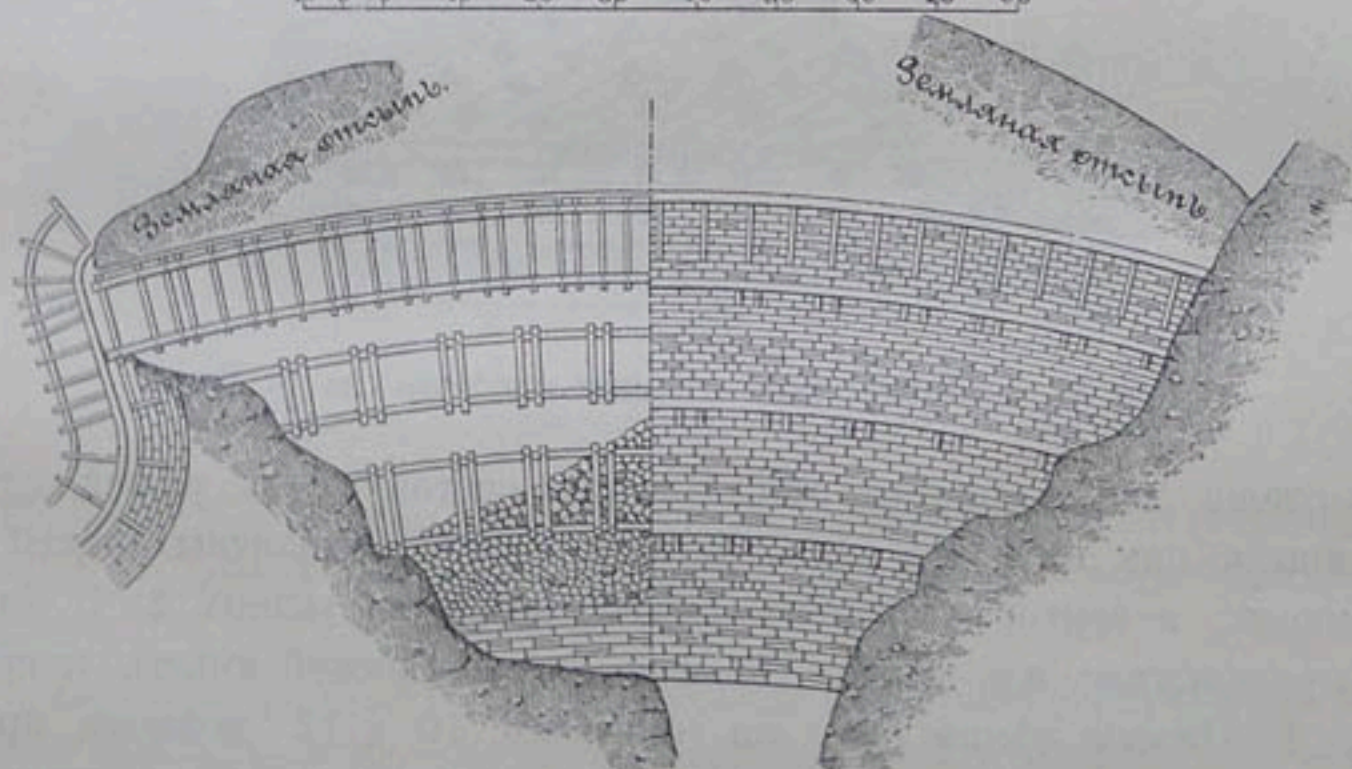
Черт. 23. — Планъ и горизонтальное сѣченіе.
