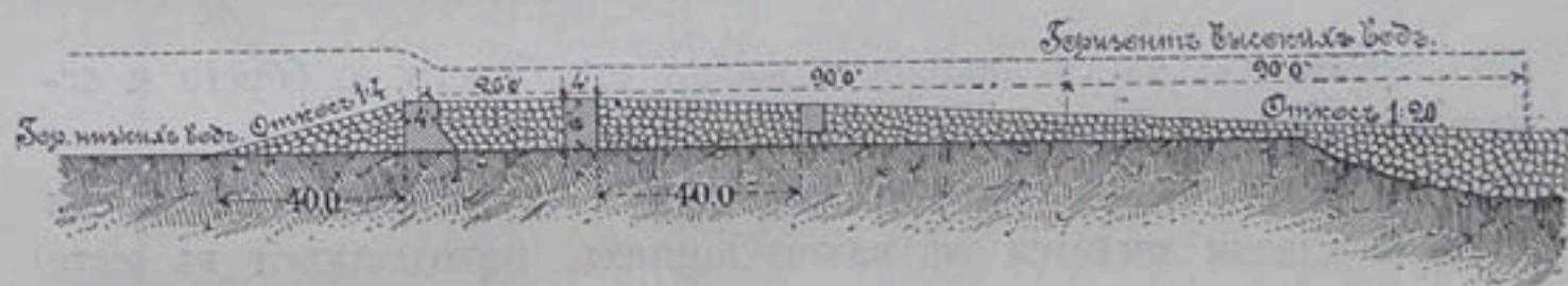
Черт. 39. — Плотина Okhla на Агрскомъ каналѣ.
