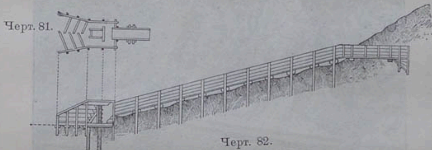
Перепадъ Big Drop на каналѣ Grand River.
