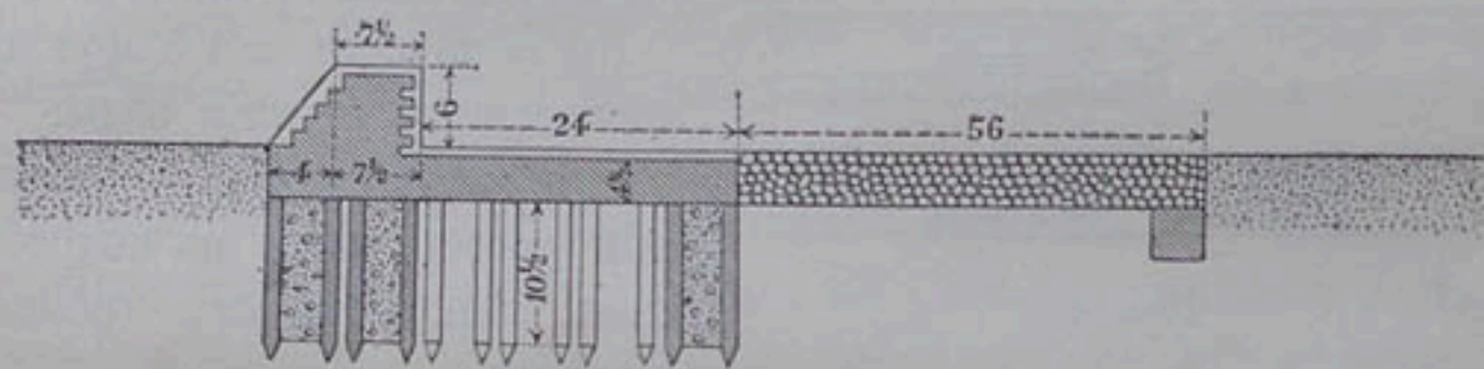
Черт. 41. — Аникутъ Streeviguntum .
