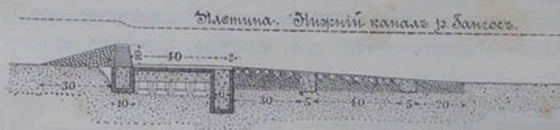
Черт. 43. — Плотина Нарора, нижній каналъ рѣки Гангеса.
