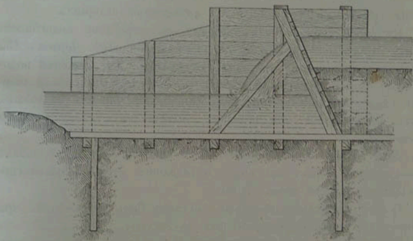
Черт. 131. — Деревянный перепадъ на каналѣ Calloway
