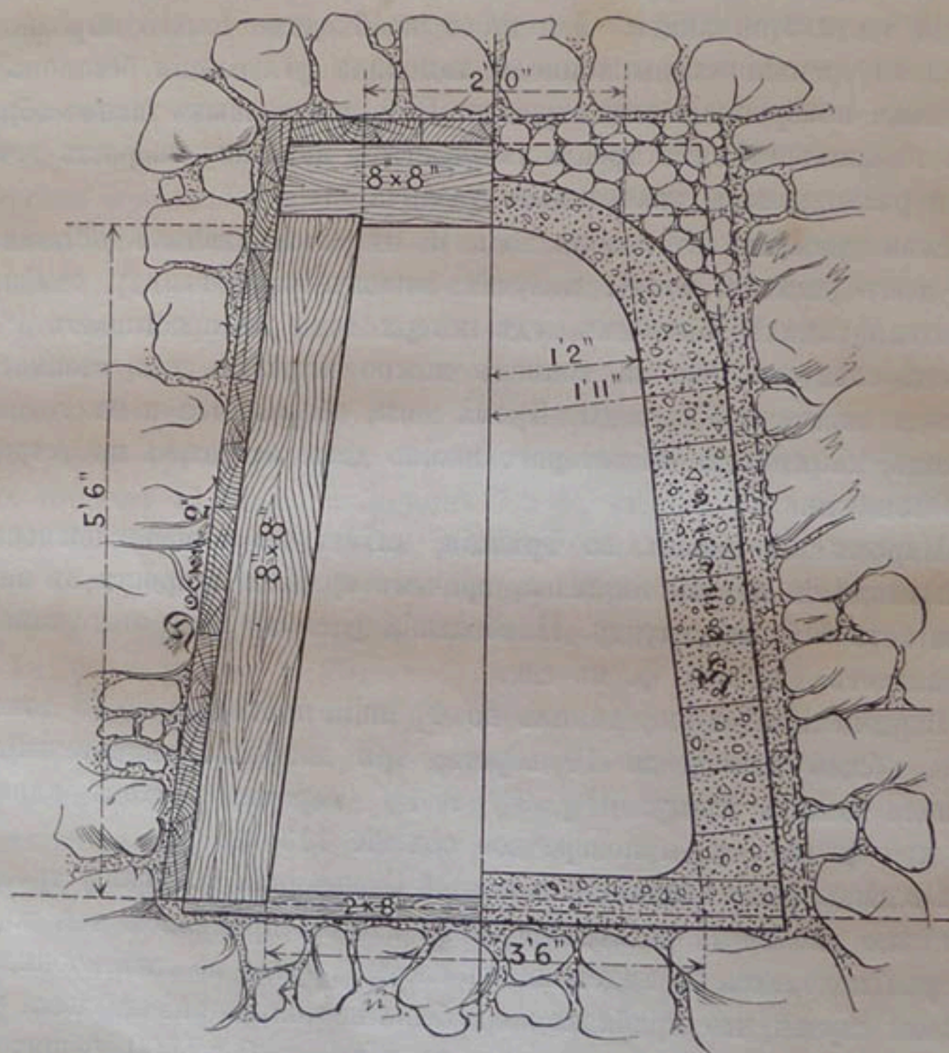
Черт. 139. — Поперечное сѣченіе тоннеля Санъ-Антоніо.
