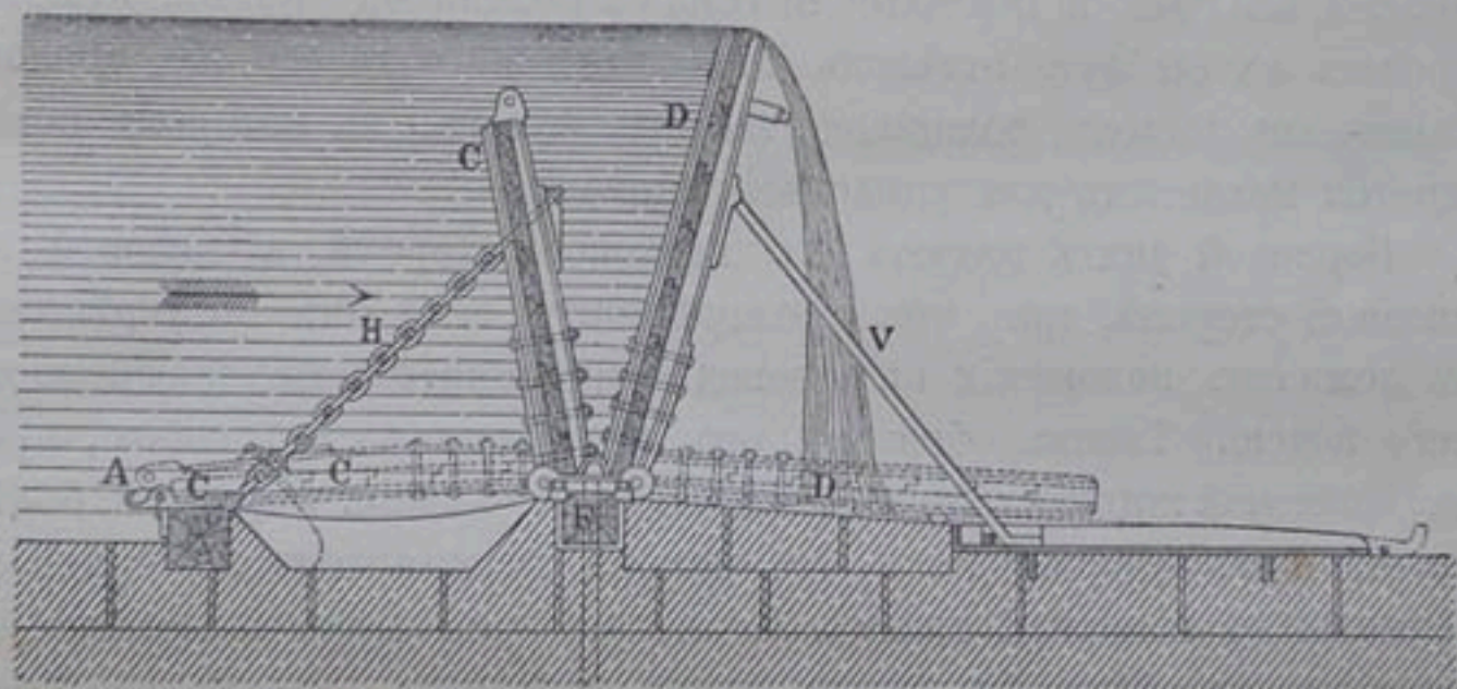
Черт. 66. — Затворы плотины Маханудди.
