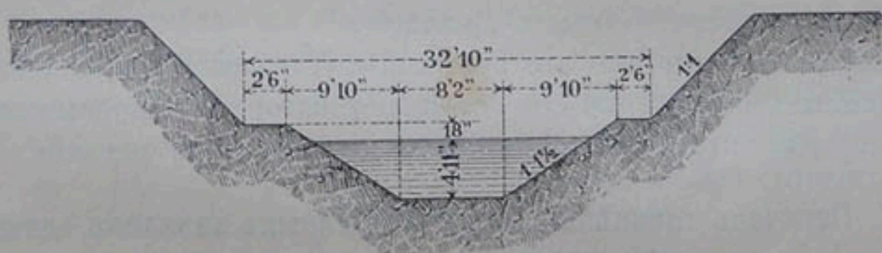
Черт. 9. — Каналь Хенаресъ въ Испаніи.
