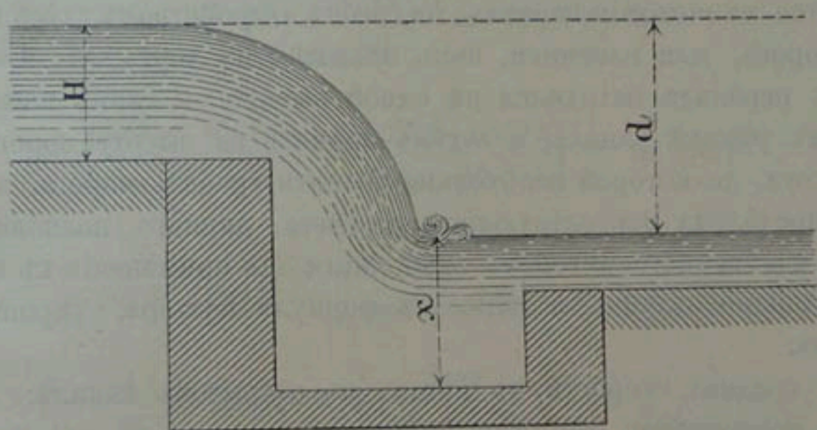
Черт. 119. — Продольное сѣченіе водослива съ водобойнымъ колодцемъ.
