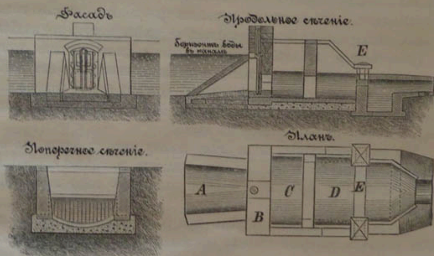
Черт. 168. — Типъ модуля на каналѣ Henares.
