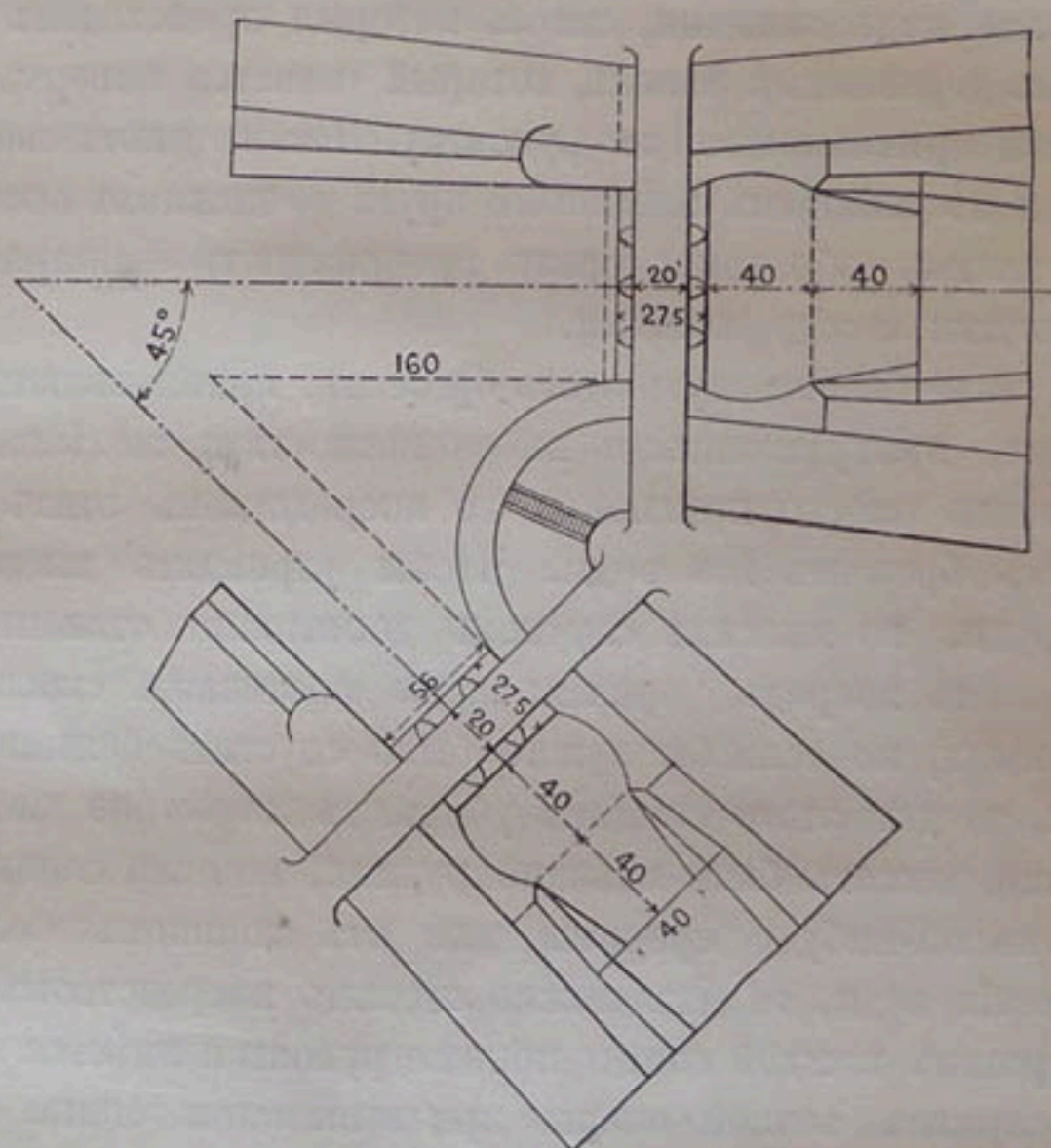
Черт. 137. — Вѣтвь Kotluh канала Sutlej.
