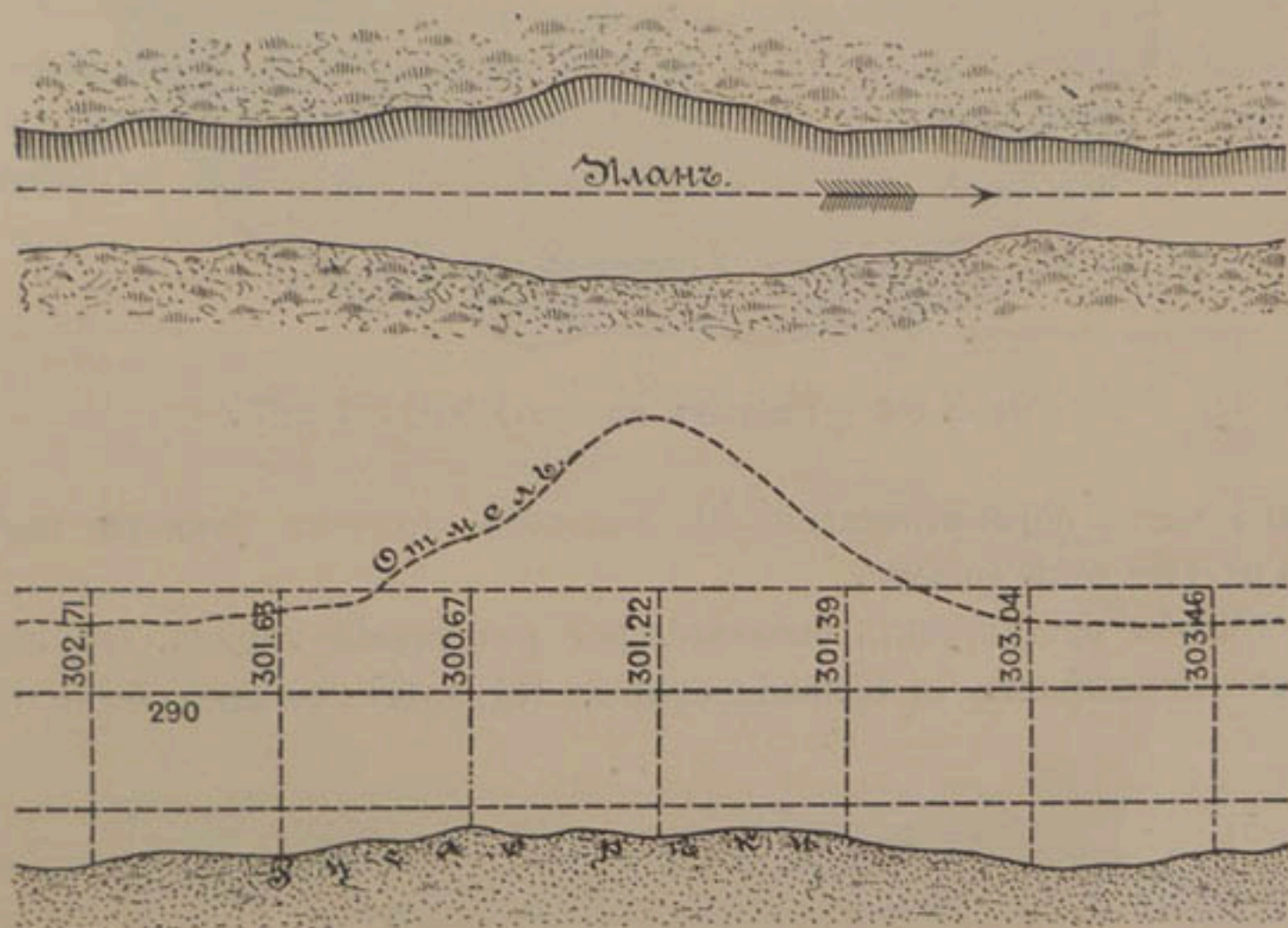
Черт. 104 и 105. — Уширеніе Гангесскаго канала у Toghulpoor.
