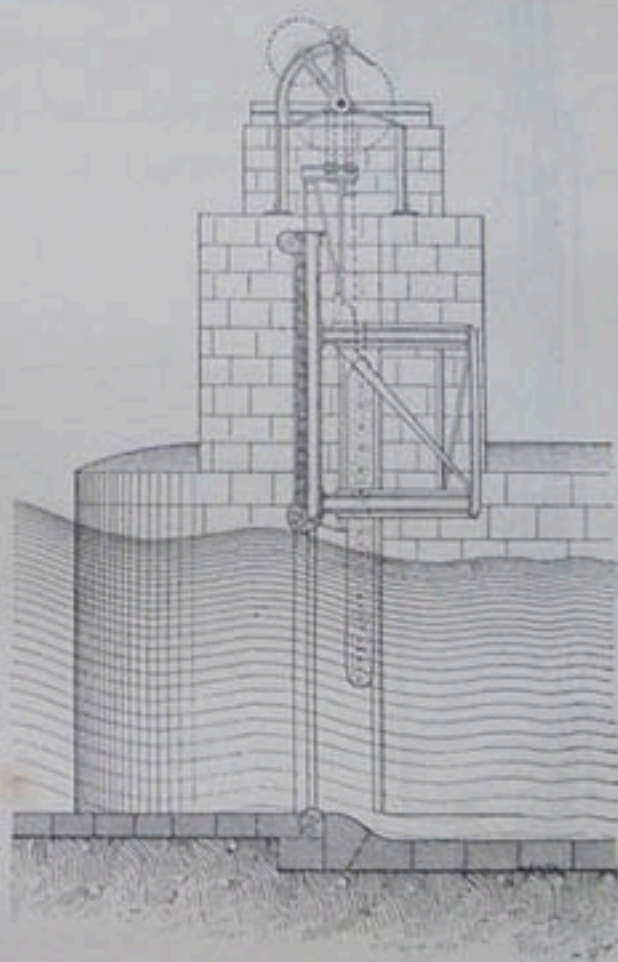
Черт. 77. — Поперечное сѣченіе при открытыхъ воротахъ.
