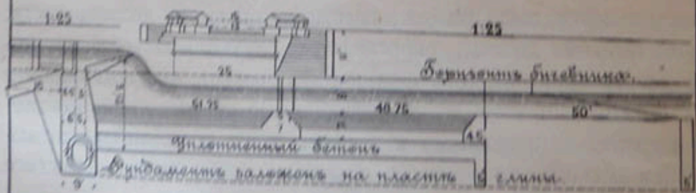
Черт. 120.—Вертикальный водосливъ на каналѣ Barge Doab.
