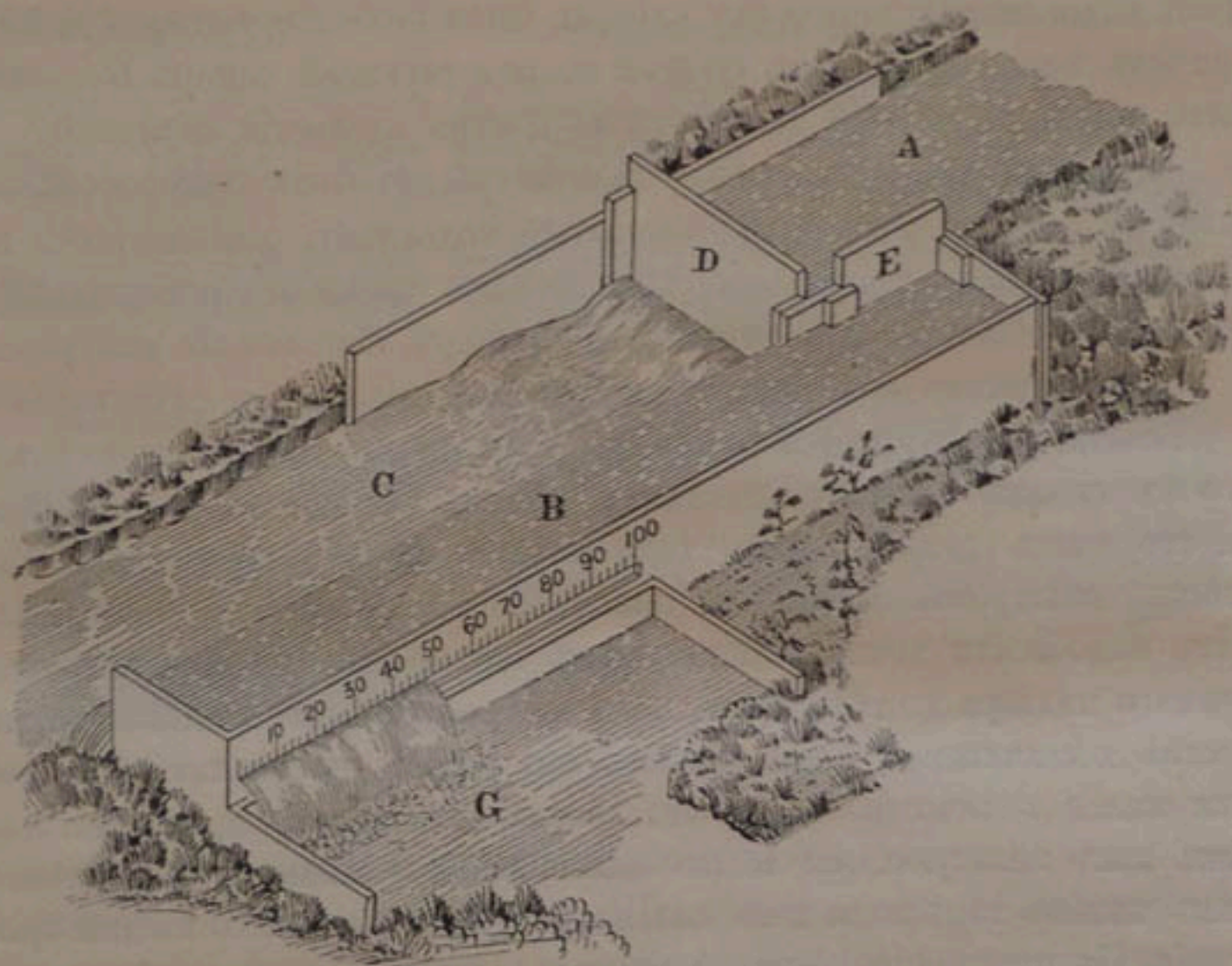
Черт. 167. — Видъ модуля А. Д. Фута.
