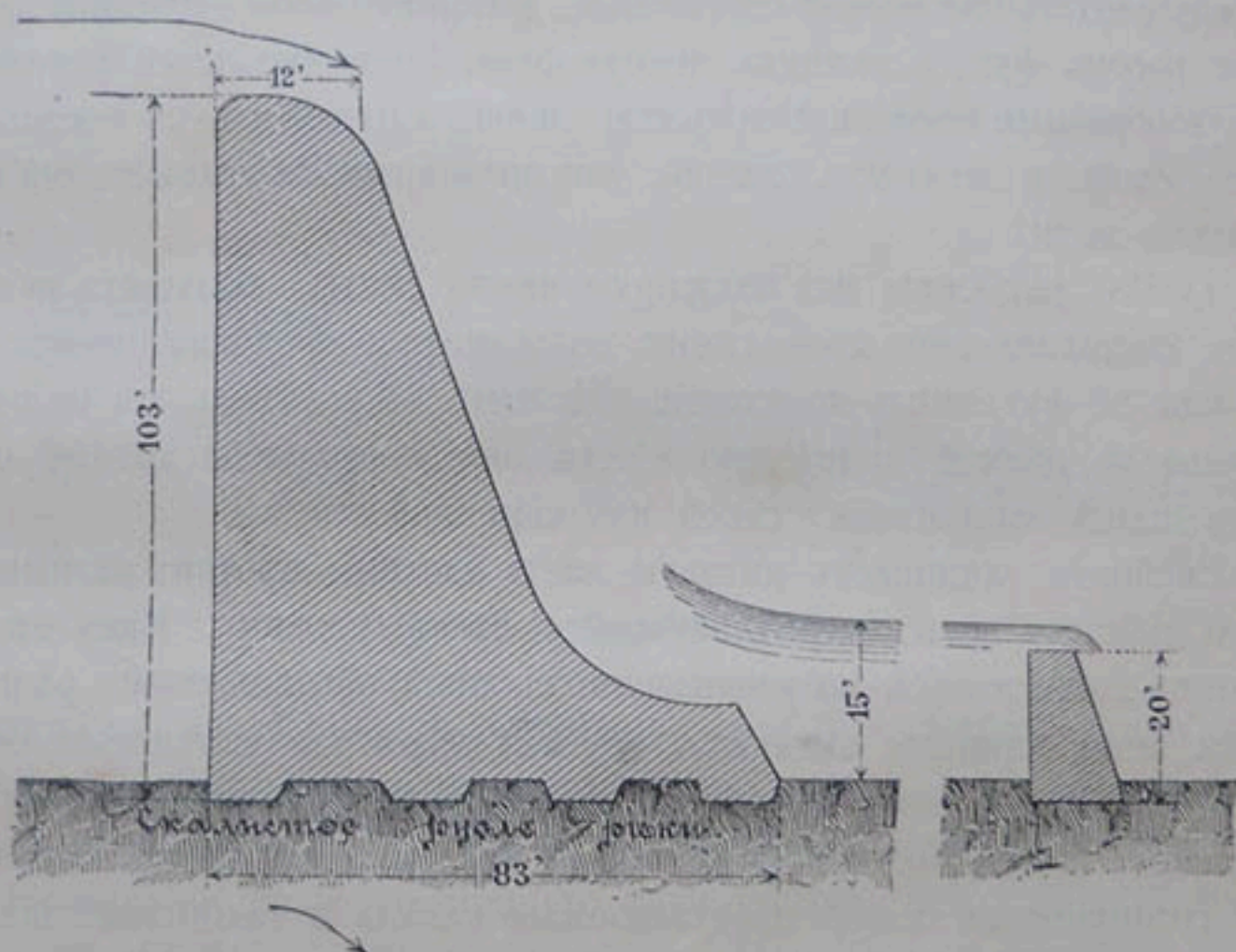
Черт. 45. — Поперечное сѣченіе плотины Turlock.
