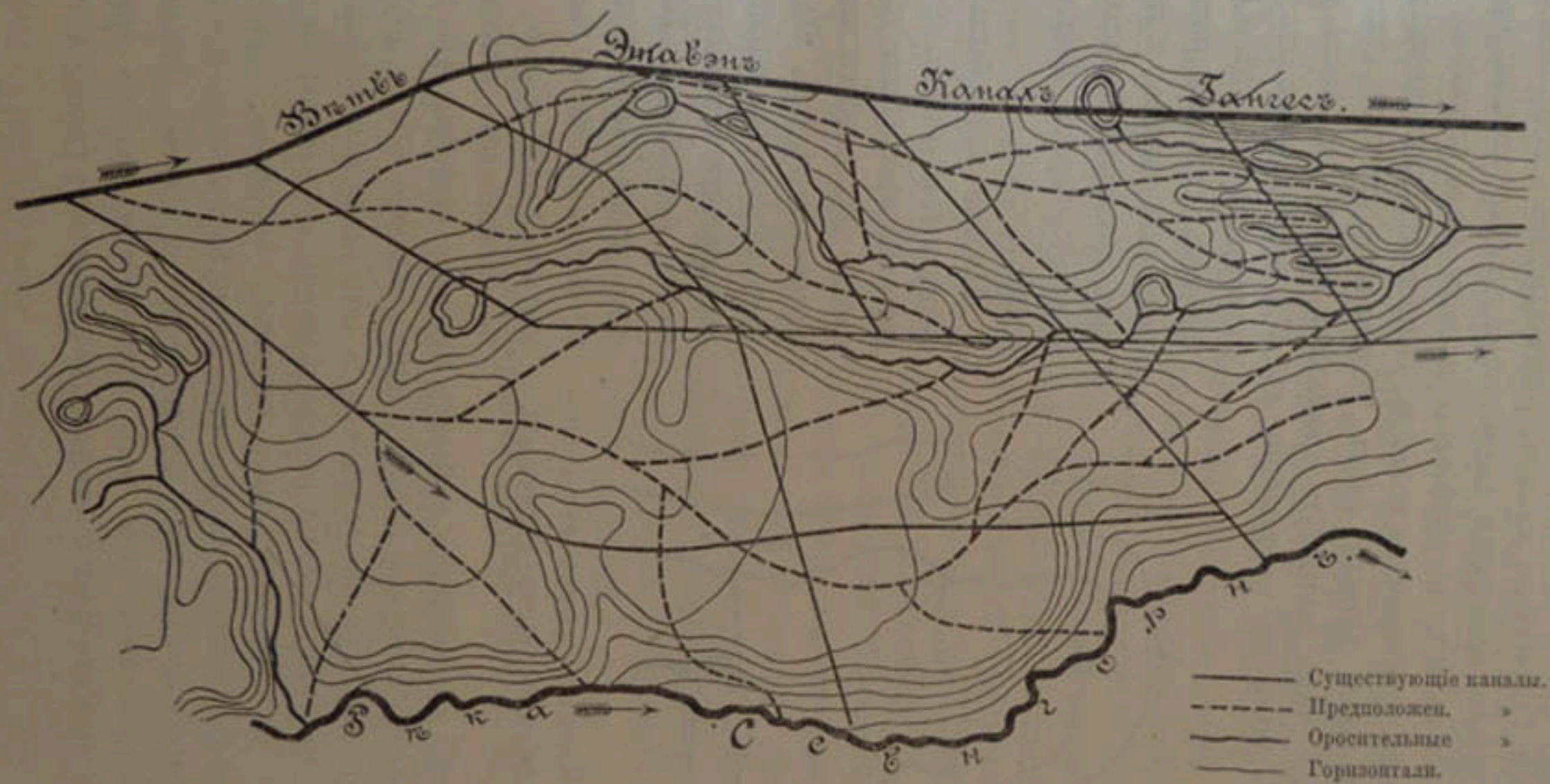
Черт. 142. — Планъ расположенія каналовъ распредѣлителей.
