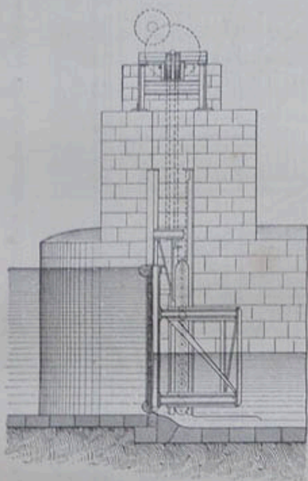
Черт. 76. — Поперечное сѣченіе при закрытыхъ воротахъ.
