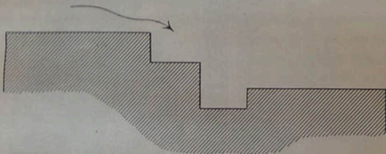
Черт. 113. — Сѣченіе водослива съ вертикальными уступами.
