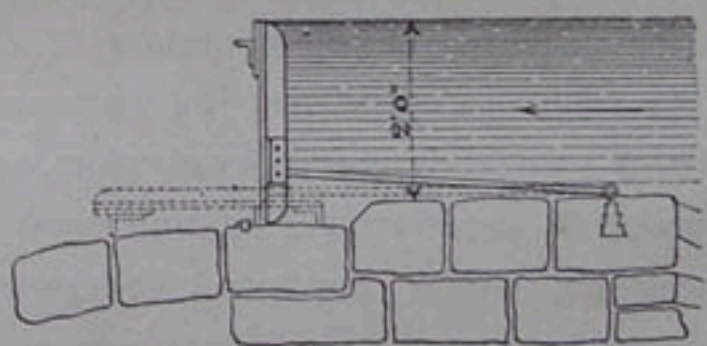
Черт. 38. — Откидной щитъ на плотинѣ Sone Weir .
