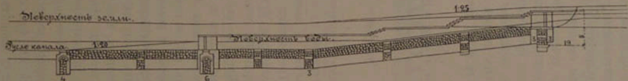
Черт. 132. — Водоспускъ на каналѣ Bagee Doab.
