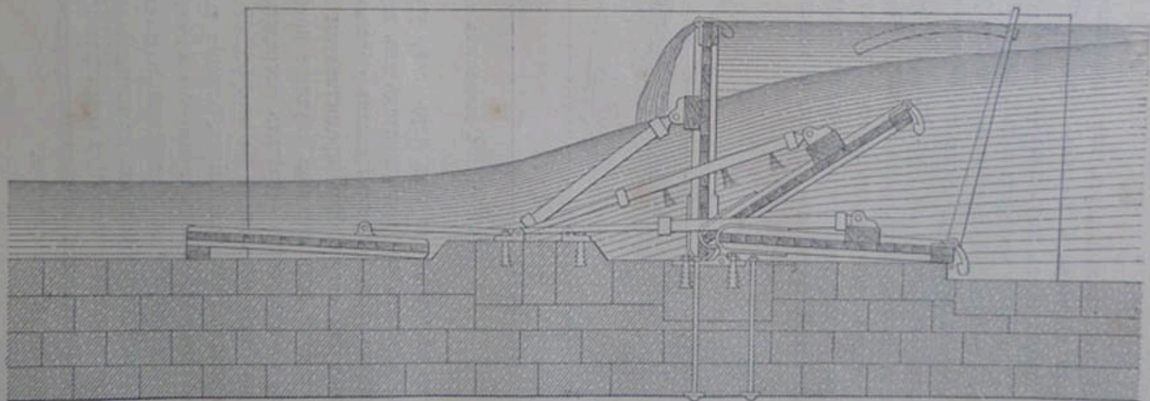
Черт. 73. — Поперечное сѣченіе по срединѣ пролета.
