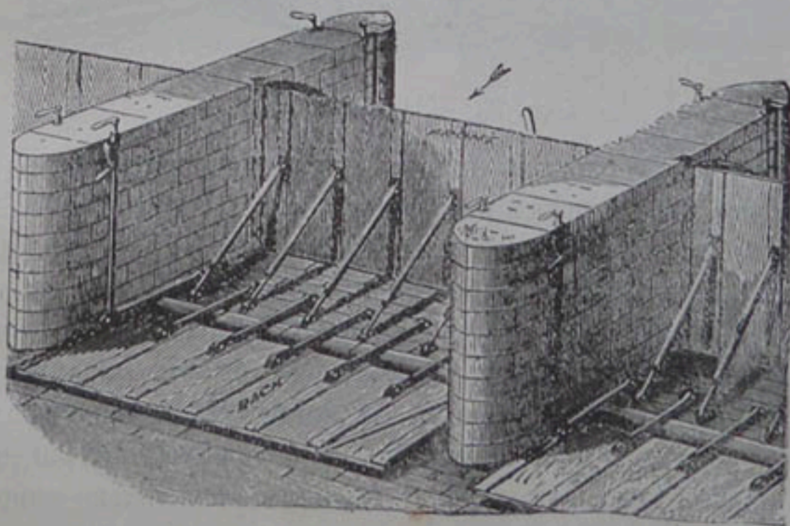
Черт. 69. — Пролетъ закрытъ.
