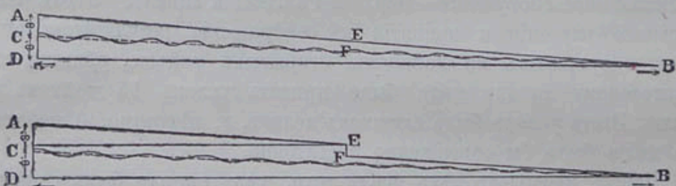
Черт. 102 и 103. — Пониженіе дна въ каналахъ.
