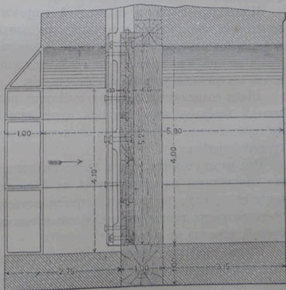
Черт. 63. — Затворы Хенаресскаго канала.
