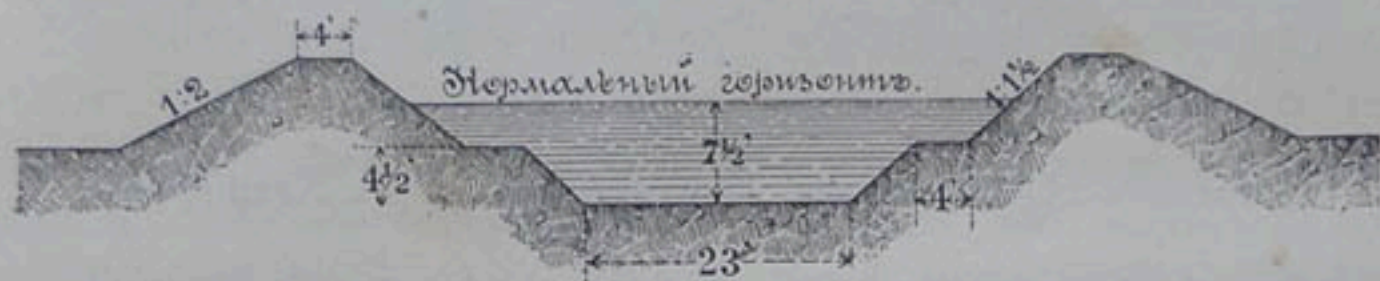
Черт. 8. — Каналь Нира въ Индіи.
