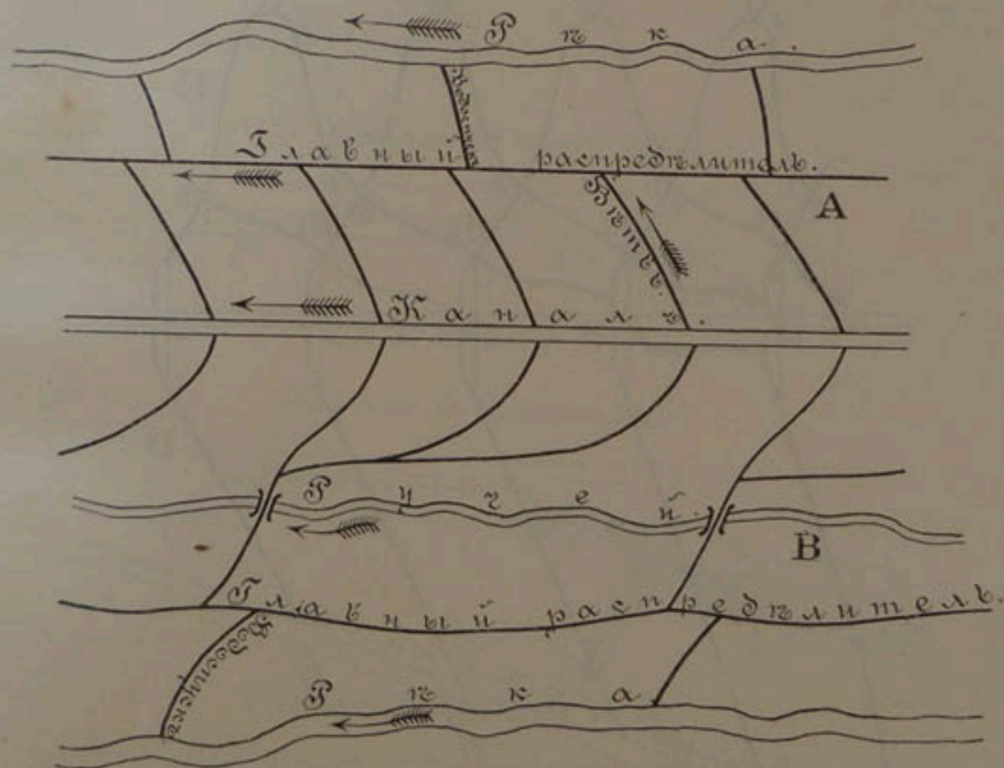
Черт. 147. — Планъ распредѣлительной системы.
