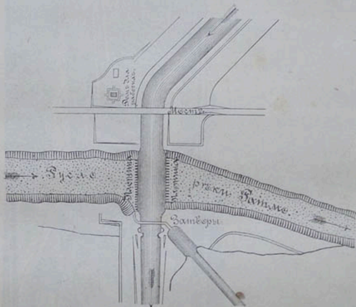
Черт. 93. — Планъ пересѣченія Гангесскаго канала р. Rutmoor близъ Dhunowree.
