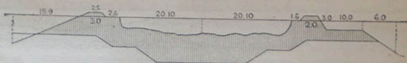
Черт. 107. — Наносы въ каналѣ Eastern Jumna.
