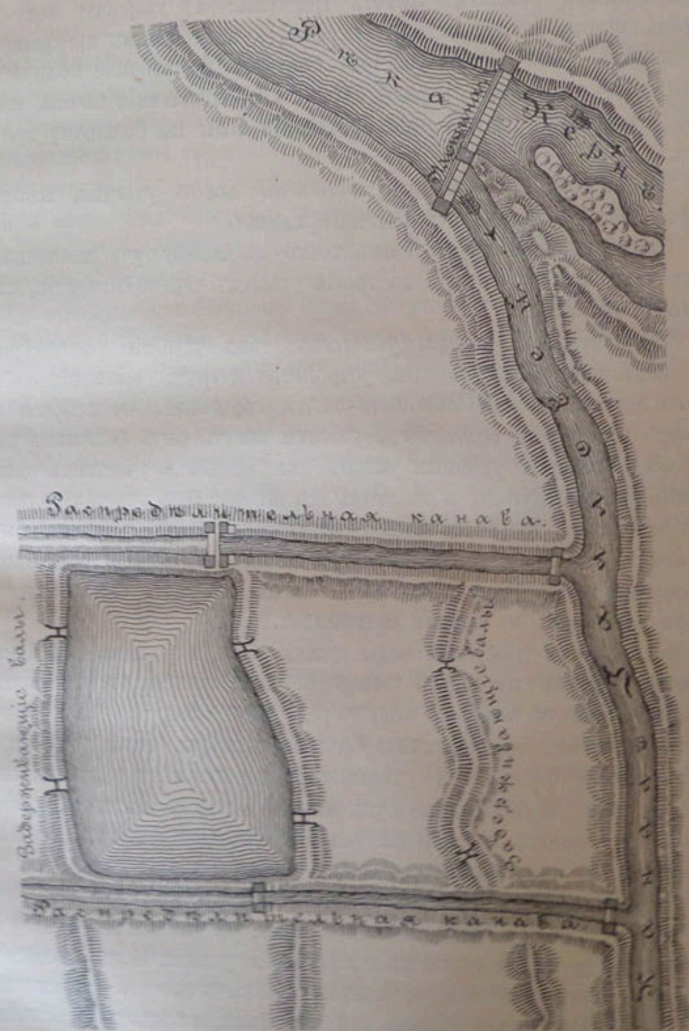
Черт. 136. — Общий видъ оросительной системы.
