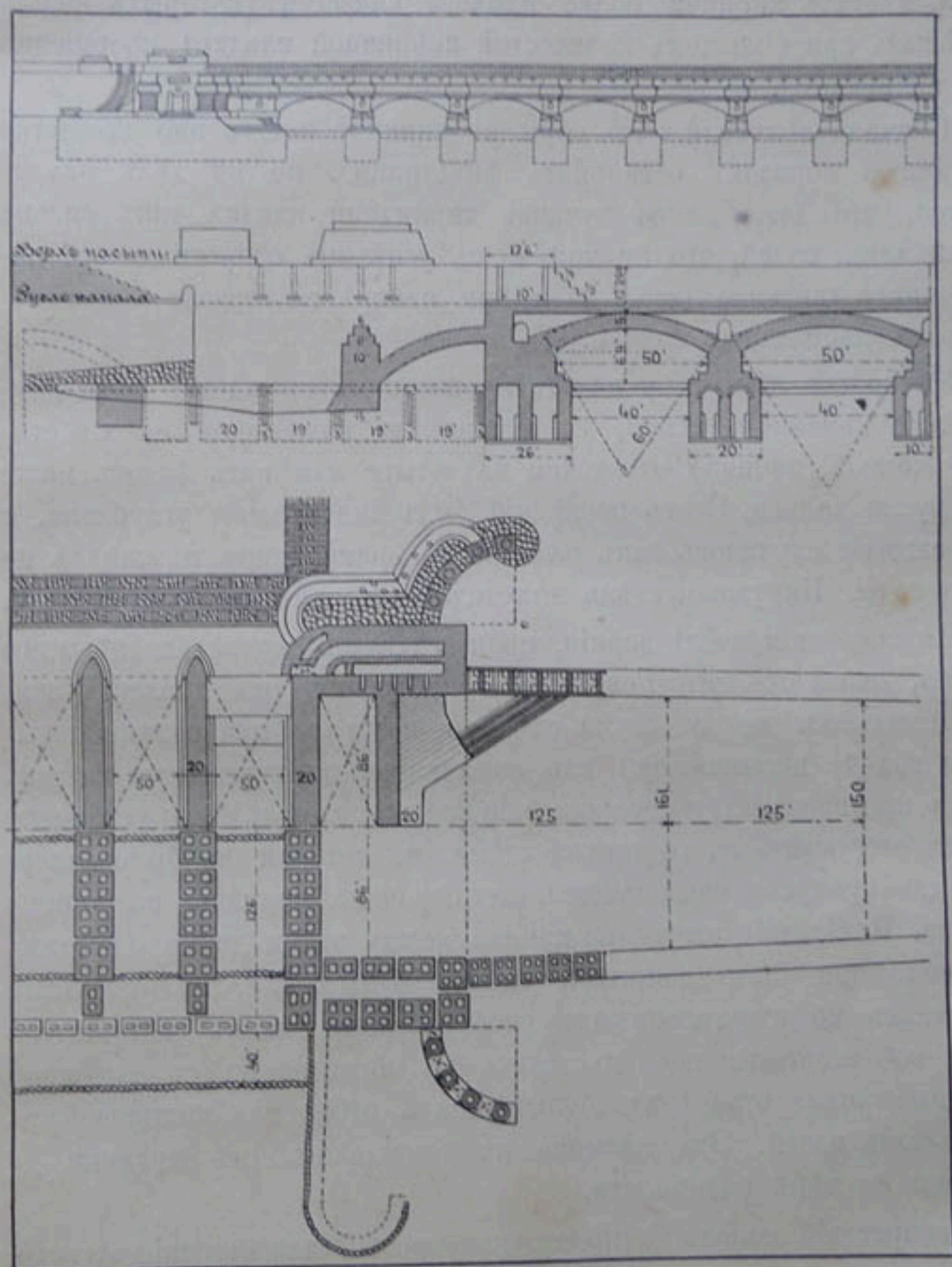
Черт. 89. — Каналь Солани.
