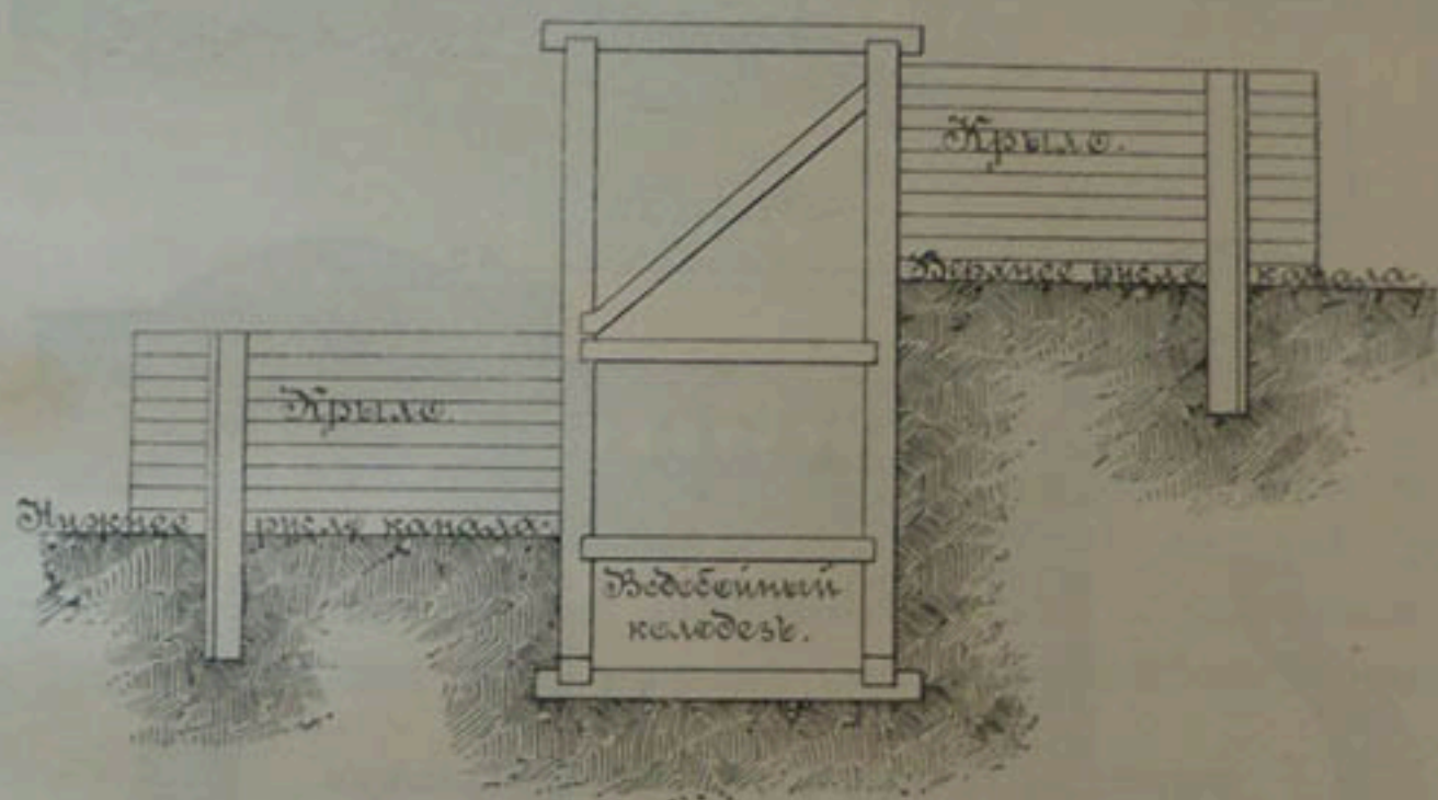
Черт. 118. — Пролонное сѣченіе деревяннаго водослива съ водобойнымъ колодеземъ.
