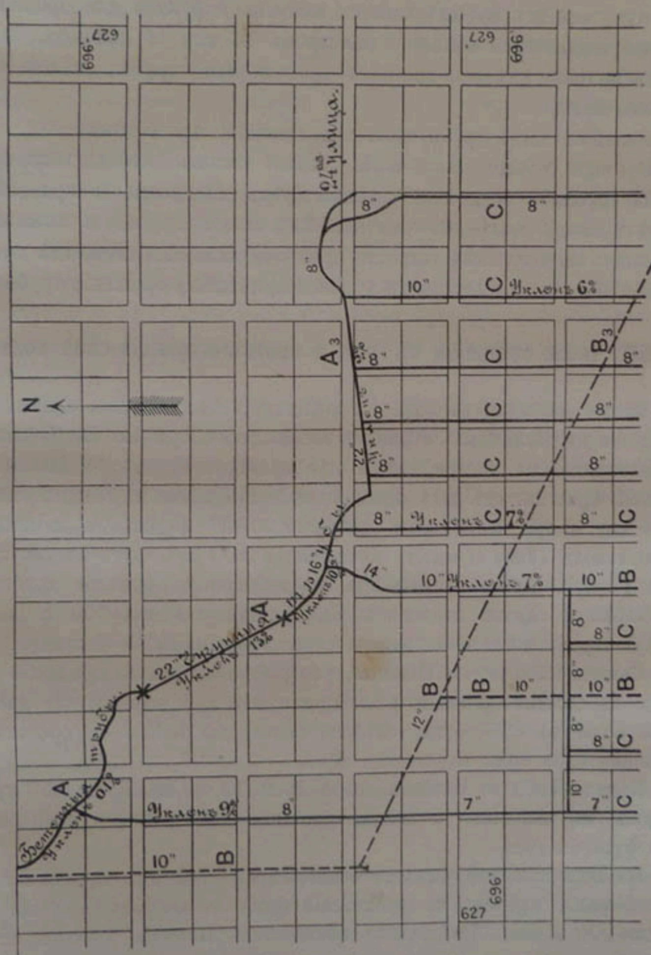
Черт. 166. — Планъ системы орошенія трубами.
