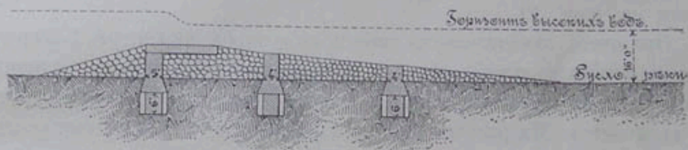
Черт. 37. — Плотина у Dehree Sone Canals.
