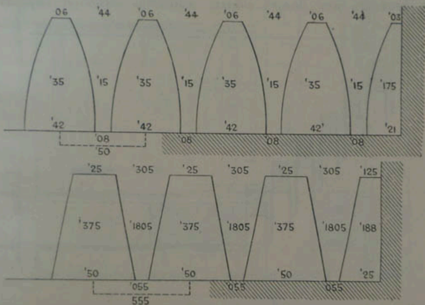
Черт. 125 и 126. — Планъ вертикальных затворовъ.
