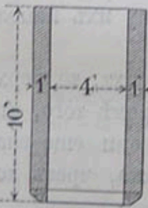
Сѣченіе по АВ.
