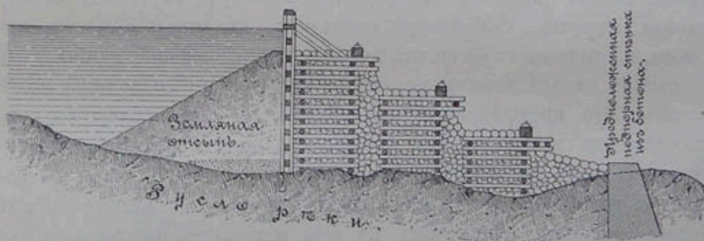
Черт. 25. — Сѣченіе у концовъ ряжей.
