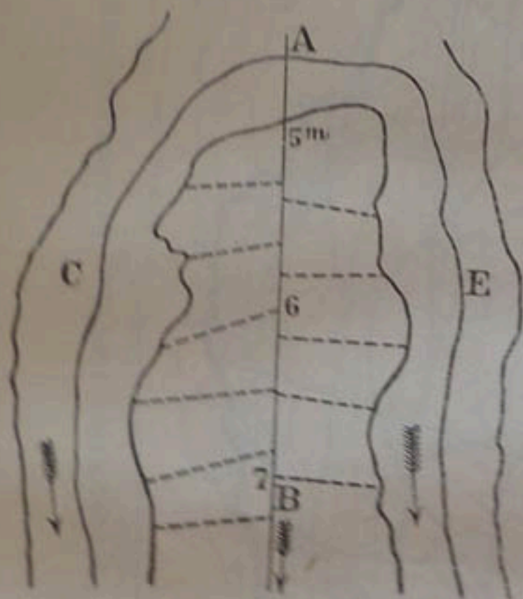
Черт. 143. — Планъ съ указаніемъ расположенія каналовъ распределителей.
