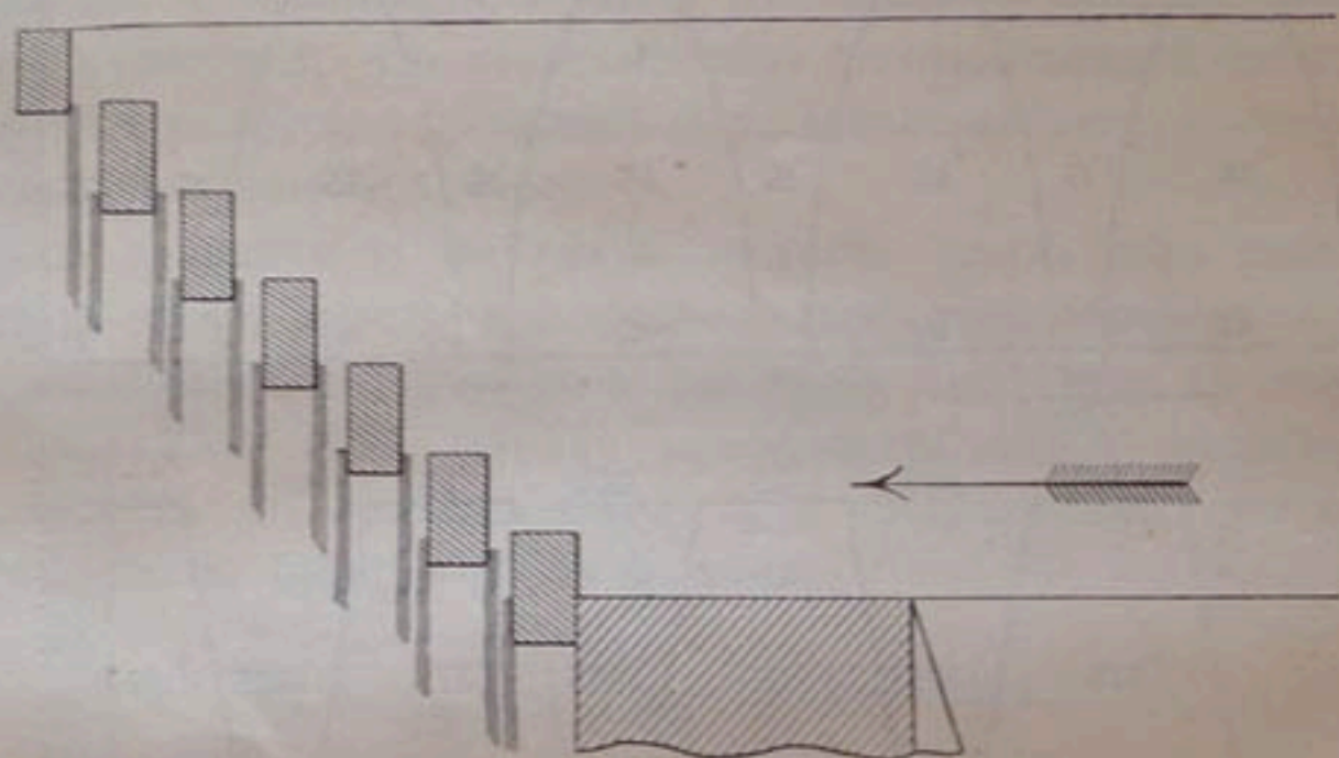
Черт. 127. — Сѣченіе плотины съ горизонтальными брусъями.
