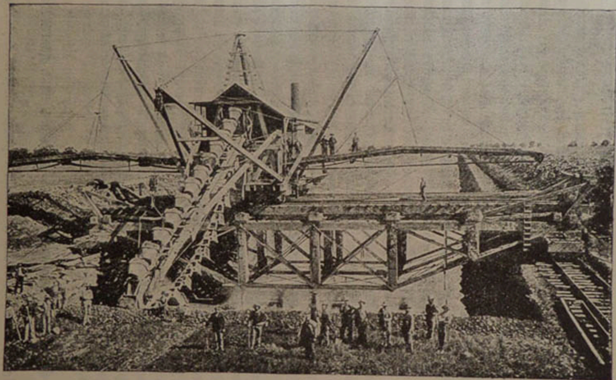
Черт. 158. — Землечерпательница Общества Jan-Francisco Bridge Company.
