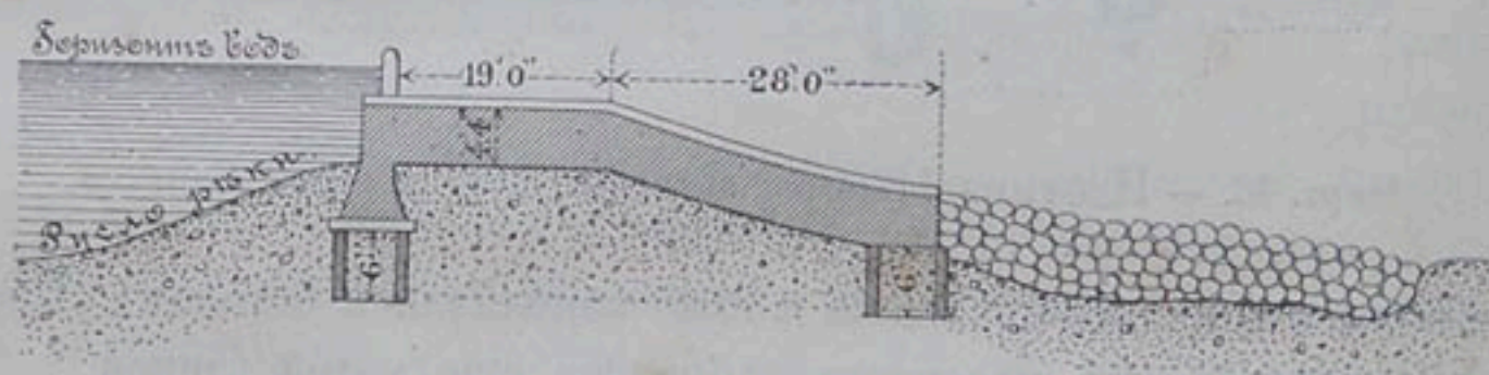
Черт. 44. — Аникутъ Годавери.
