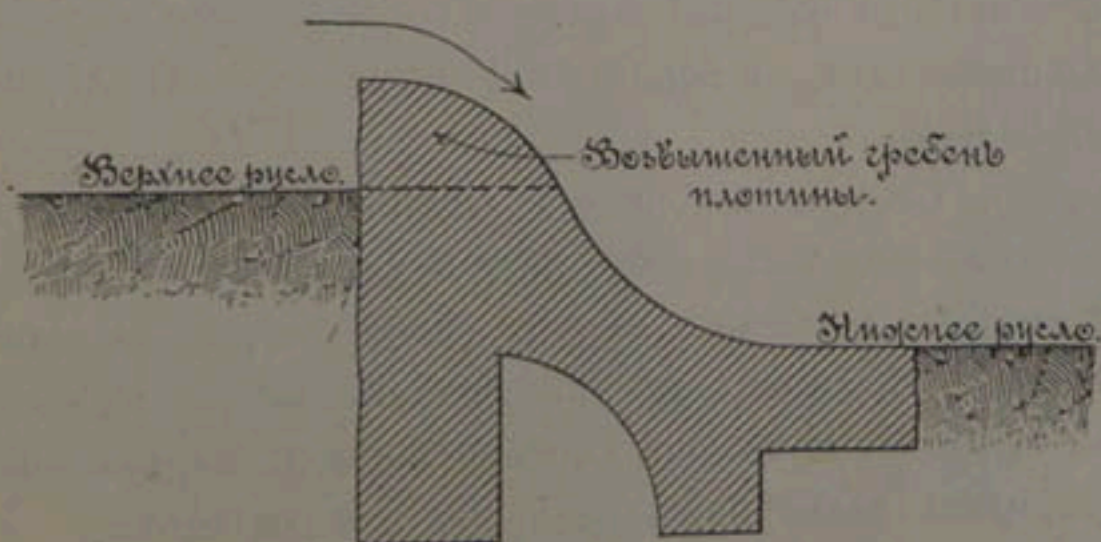
Черт. 110. — Сѣченіе водослива Огес.
