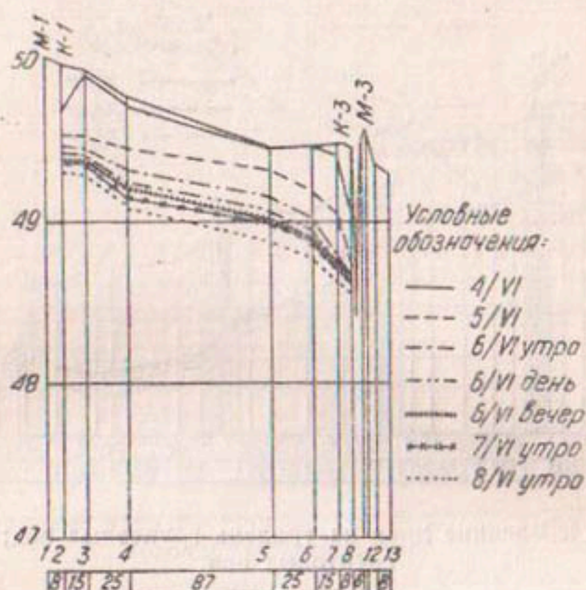
Рис. 16. Влияние дрен на уровень грунтовых вод; спад грунтовых вод после полива дренированного участка.
