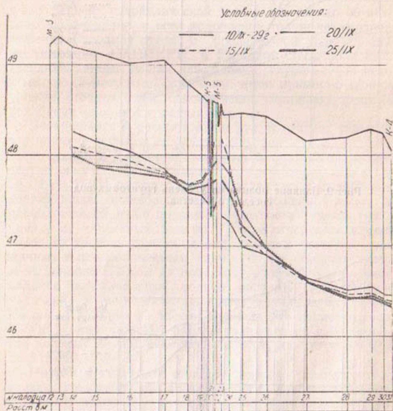
Рис. 11. Влияние оросителей на уровень грунтовых вод.
