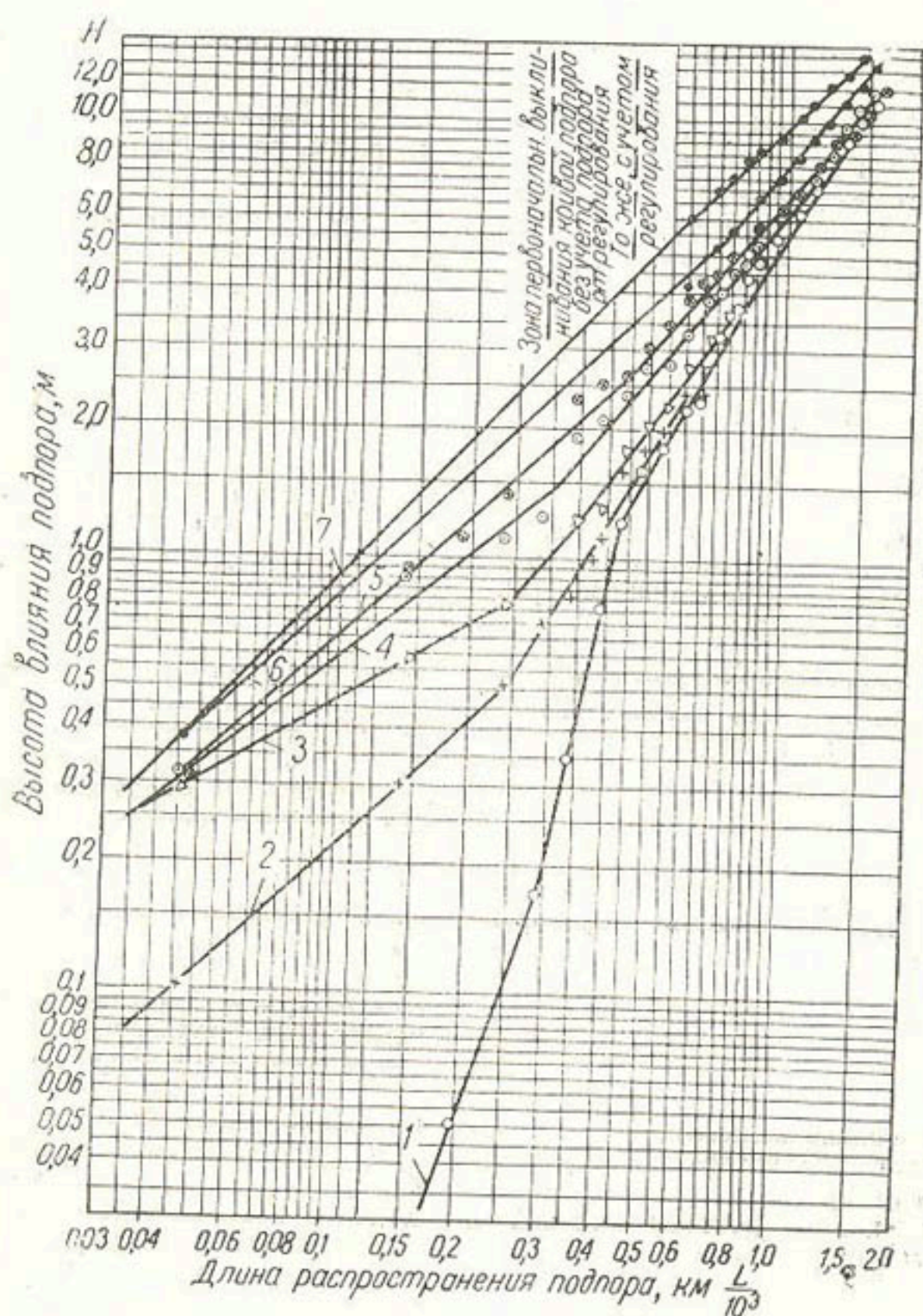
Рис. 53. Кривые изменения горизонтов воды в подпертом бьефе при среднепаводковом расходе ( Q = 160 \text{ м}^3/\text{сек} ) по мере его формирования; I_0 = 0,0034 , \Delta H = 3,80 \text{ м} , подпертый бьеф руслового типа зарегулирован, B = 30-60 \text{ м} (модель).
