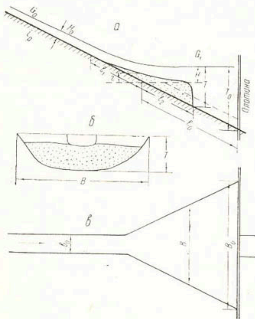
Рис. 43. Расчетная схема. а — продольный разрез, б — поперечный разрез, в — план.
