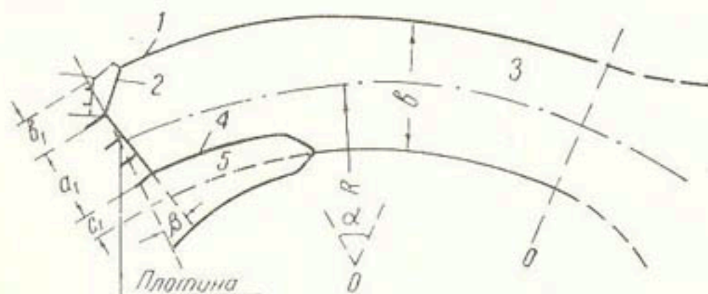
Рис. 4. Принципиальная схема водозабора ферганского типа. 1 — урез воды при расчетном расходе, 2 — водоприемный порог, 3 — подводящее русло, 4 — катастрофический волослив; 5 — траншейный сброс; относительные фронтальности: a = a_1/B (на рисунке — ошибочно b ) плотины, b = b_1/B водоприемного порога, c = c_1/B сбросного волослива; \alpha — угол поворота подводящего русла, \beta — угол шитового сброса (отклонение фронта плотины от л к подводящему руслу).
