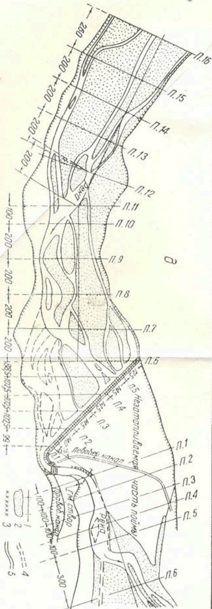
Рис. 45. Сарат-Курганский гидроузел.
