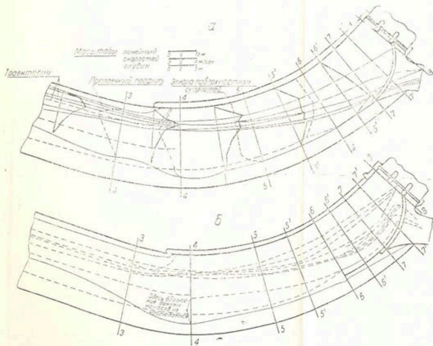
Рис. 38. План траекторий поверхностных струй и эпюры поверхностных скоростей в подводящем русле (а), направление глубинных токов (б), профили горизонтов воды и дна (в).
