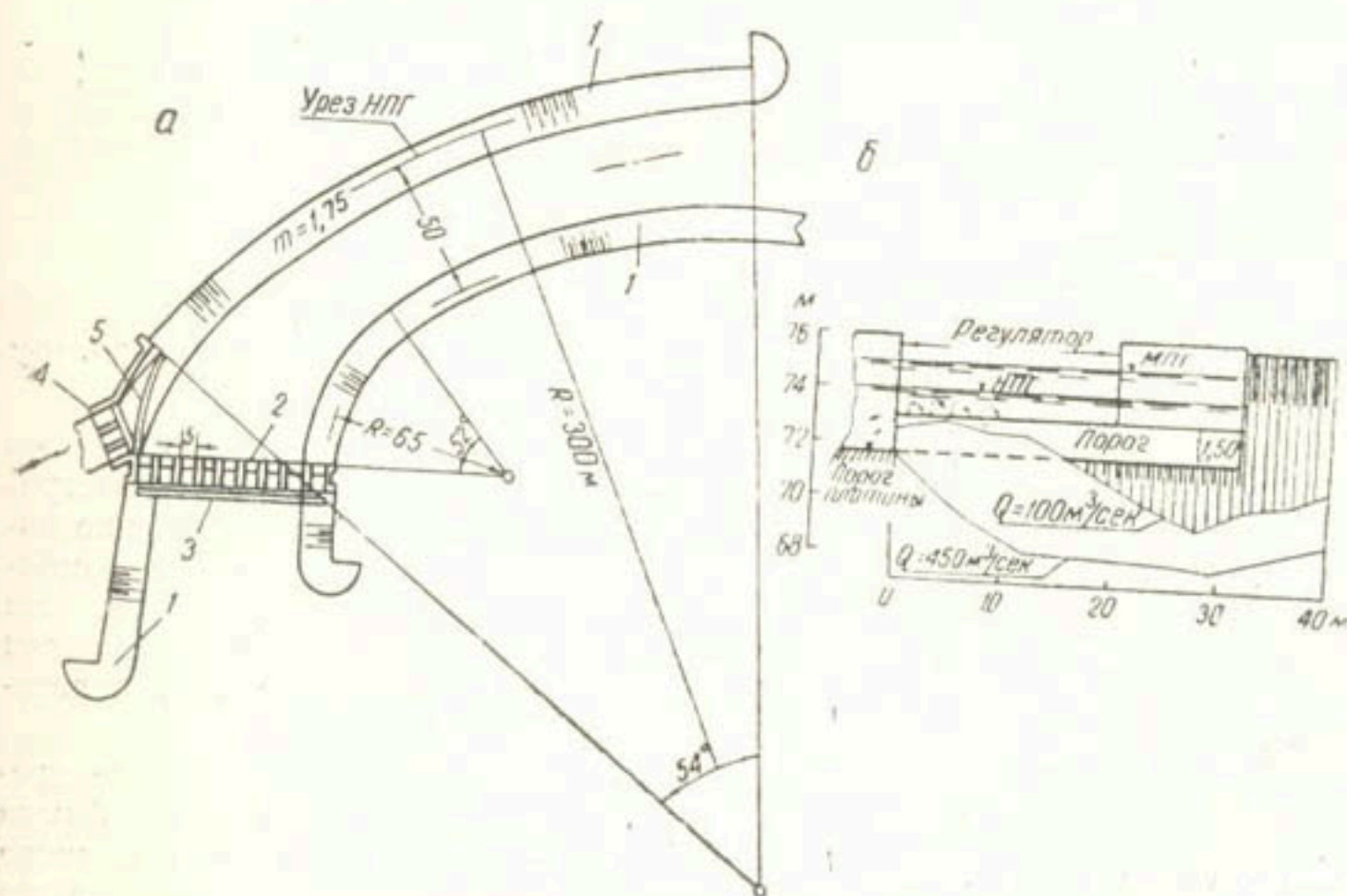
Рис. 17. Плотина Арысь-Туркестанского канала на р. Арысь. а — план: 1 — струенаправляющие дамбы, 2 — плотина, 3 — предохранительная плоскость, 4 — регулятор, 5 — водоприемный порог. б — профили для перекладки водоприемника с повышенным прямоугольным порогом (движение напоров через порог показано пунктирными стрелками).
