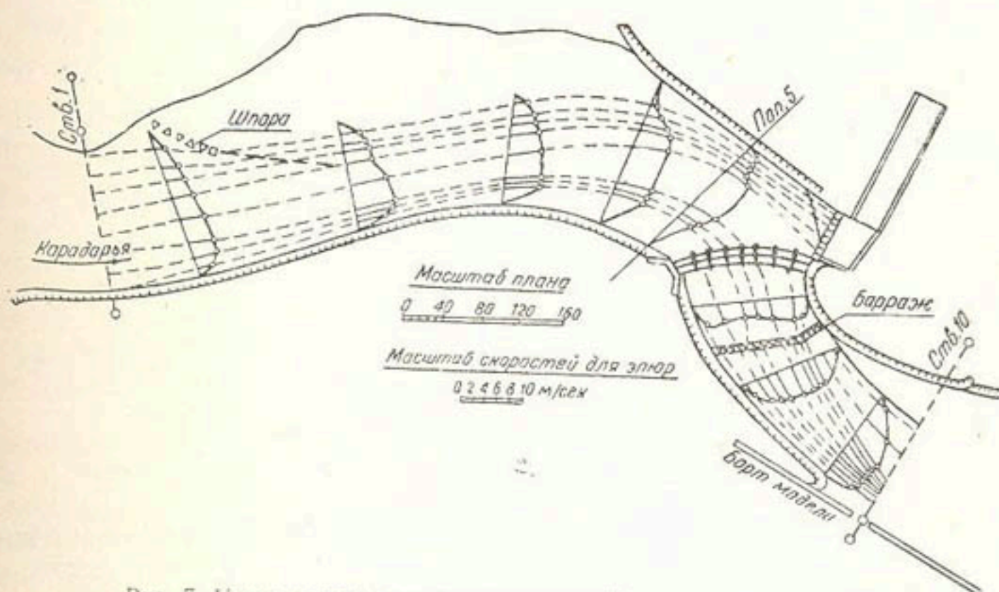
Рис. 7. Направление поверхностных струй и эюры скоростей при Q = 150 \text{ м}^3/\text{сек.} ; водозабор 230 \text{ м}^3/\text{сек.}
