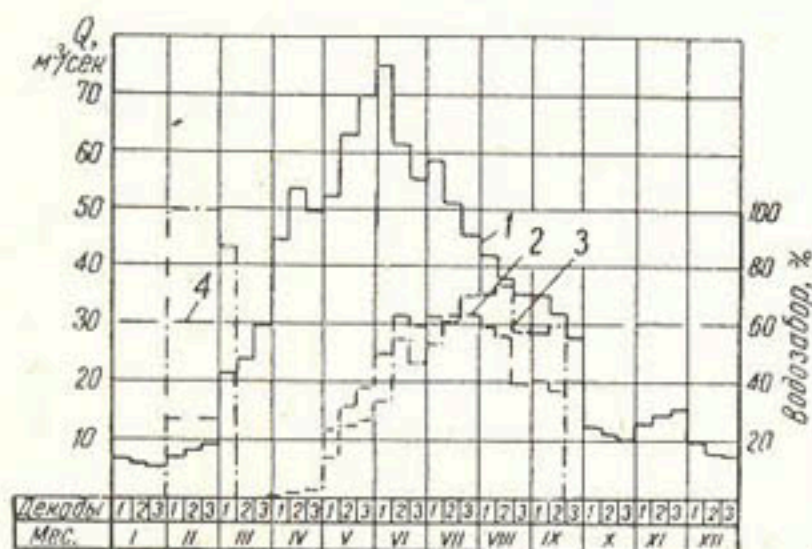
Рис. 29. Гидрографы р. Каратаг с подпитыванием из р. Дюшамбинки и водозабор в Тупалангский канал на гидроузле.
