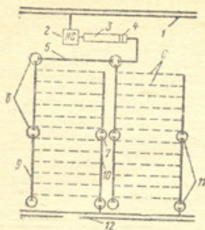
Рис. 2. Схема системы двустороннего действия с подачей воды через истоки дрен: 1 — водонесущий; 2 — насосная станция; 3 — отстойник; 4 — керамзитовый фильтр; 5 — распределительный трубопровод; 6 — приемные колодцы; 7 — сбросные дрены; 8 — регулирующие дрены; 9 — увлажнительный коллектор; 10 — сбросной коллектор; 11 — клапаны; 12 — открытый коллектор
