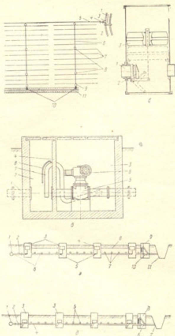
Рис. 8. Схемы автоматизации системы двустороннего действия: а — схема системы регулирования уровня грунтовых вод дренажной сетью; 1 — водонепроницаемая перегородка; 2 — низконапорное сооружение.
