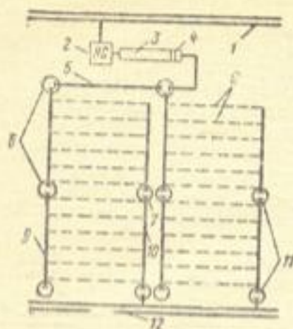
Рис. 2. Схема системы двустороннего действия с подачей воды через источник дрена: 1 — водонесущий; 2 — насосная станция; 3 — отстойник; 4 — керамзитовый фильтр; 5 — распределительный трубопровод; 6 — приемные колодцы; 7 — сбросные дренажи; 8 — регулирующие; 9 — увлажнительный коллектор; 10 — сбросной коллектор; 11 — клапаны; 12 — открытый коллектор
