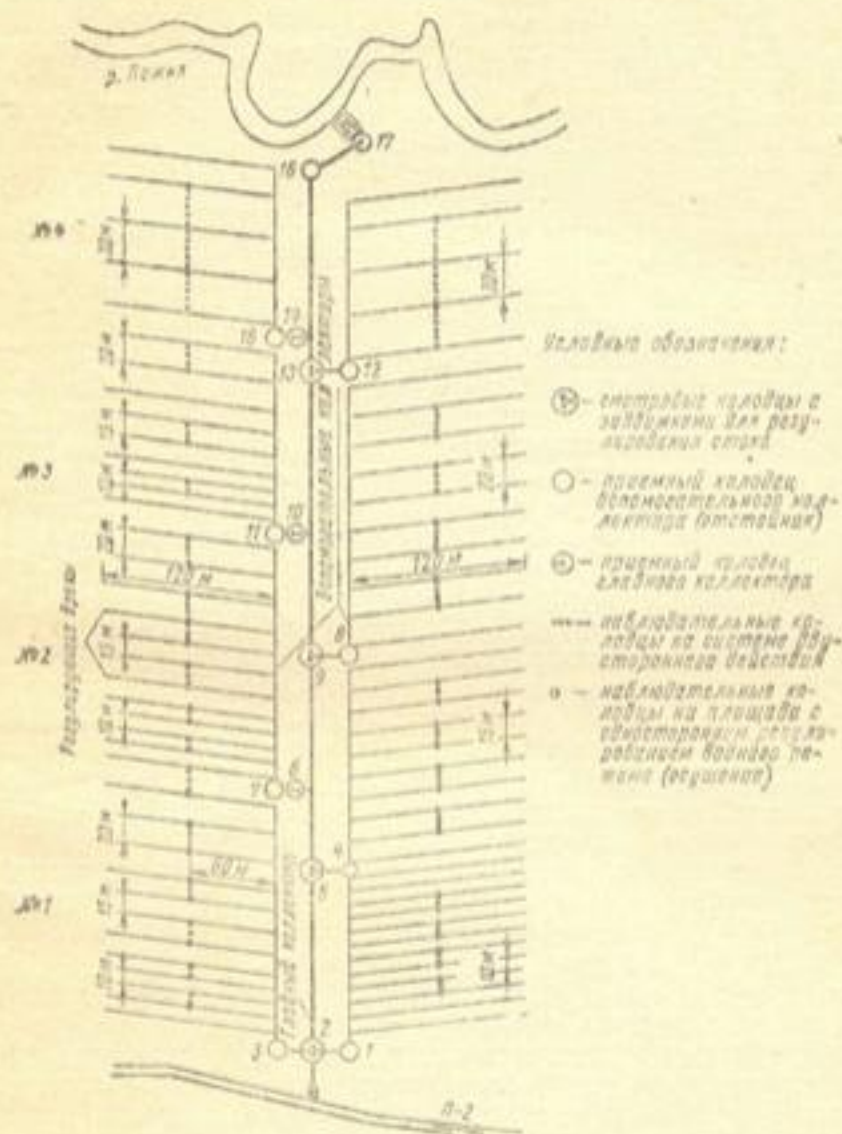
Рис. 3. План системы двустороннего регулирования водного режима почв в совхозе «Клементьевское» Можайского района Московской области
