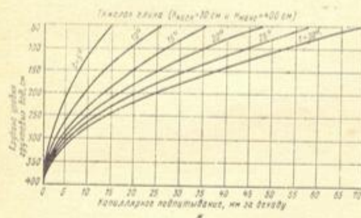
Рис. 4. Объем капиллярного подпитывания почвы при h_{\text{корн}} = 30 см: а — песок, H_{\text{макс}} = 50 см; б — супесь, H_{\text{макс}} = 100 см; в — легкий суглинок, торф, H_{\text{макс}} = 150 см; г — средний суглинок, H_{\text{макс}} = 200 см; д — тяже- лый суглинок, H_{\text{макс}} = 250 см; е — легкая глина, H_{\text{макс}} = 300 см; ж — тяжелая глина, H_{\text{макс}} = 400 см
