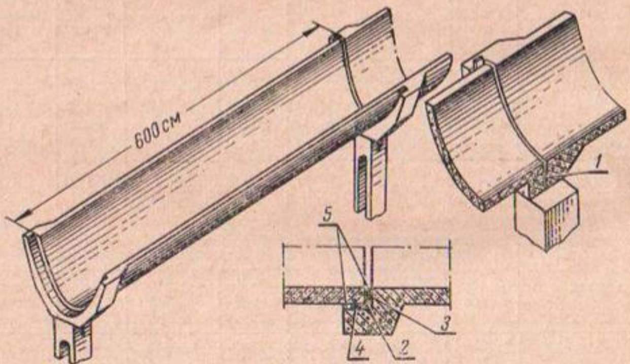
Рис. 52. Конструкции лотков:
