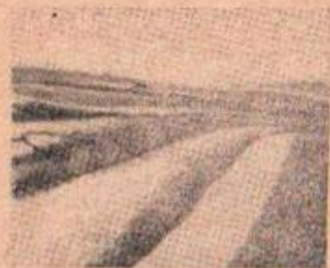
Рис. 63. Участок канала с деформированной облицовкой.
