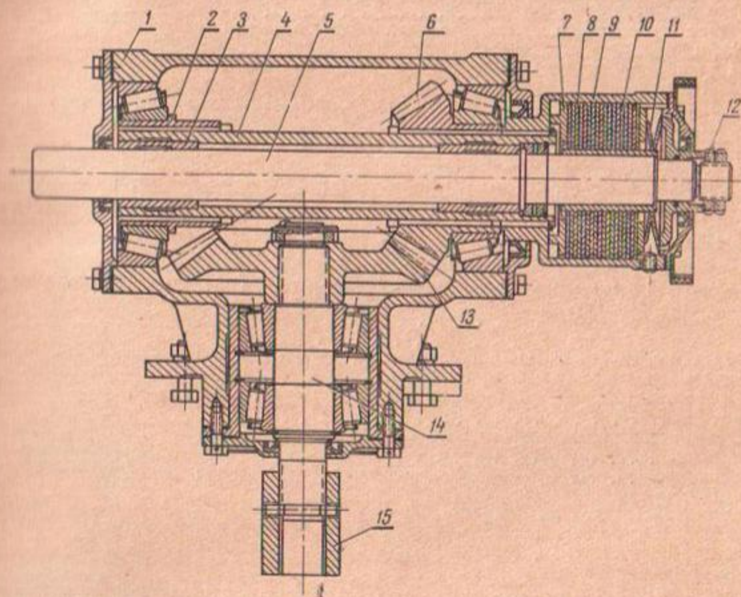
Рис. 10. Конический редуктор:
