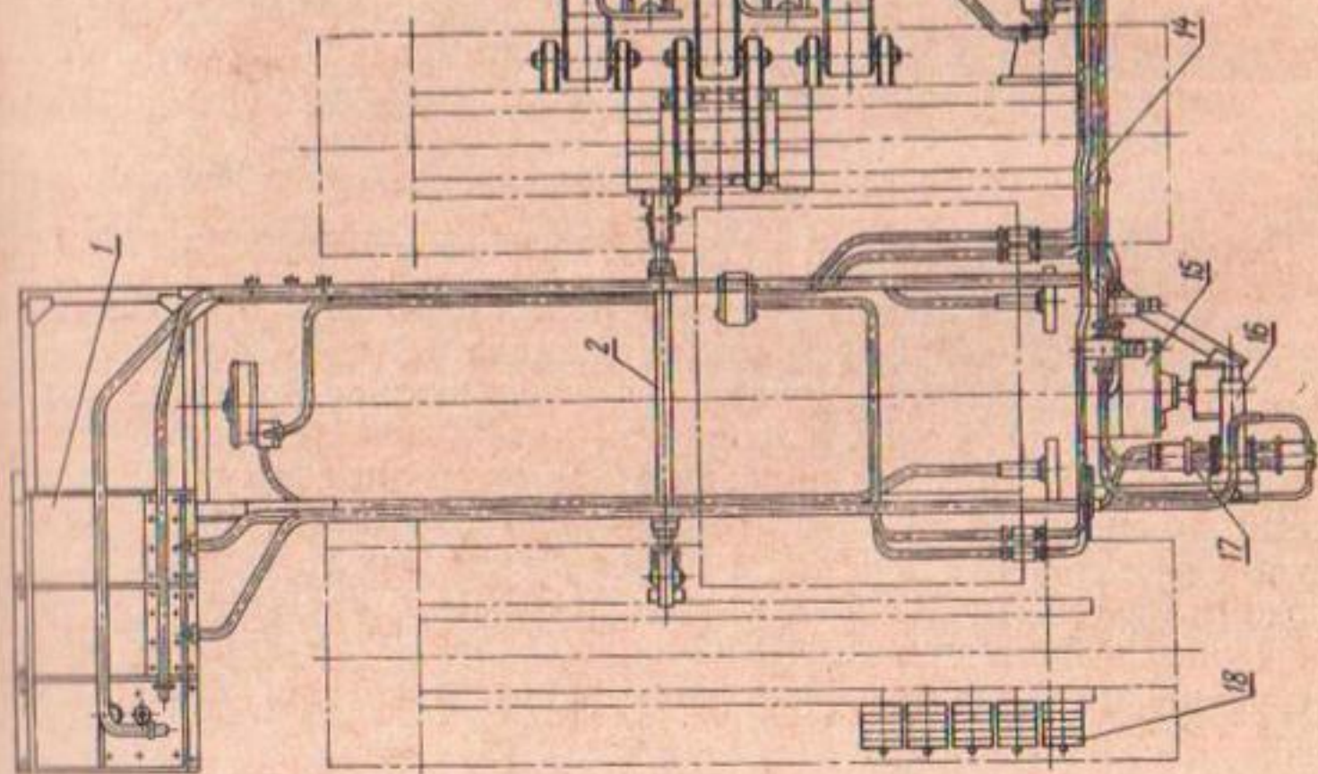
Рис. 24. Конструкция навесного рабочего оборудования каналоочистителя КОБ-1,5;
