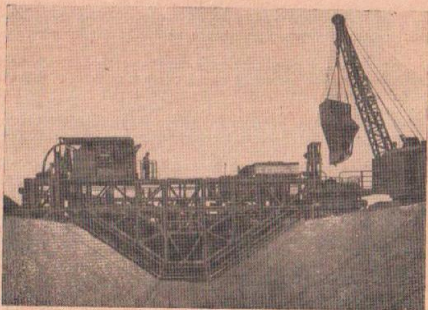
Рис. 56. Бетоноукладчик Д-655.
