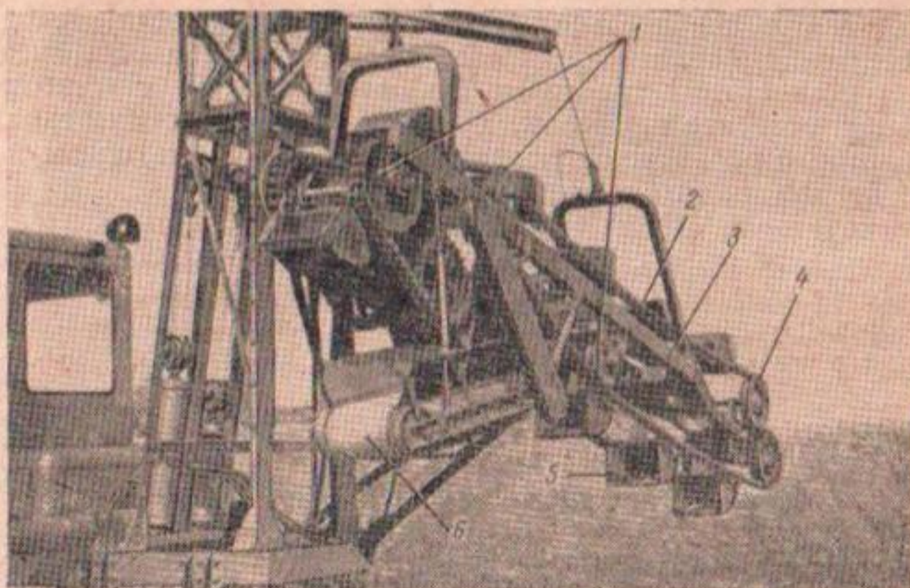
Рис. 27. Рабочее оборудование многоковшового экскаватора ЭМ-152А: 1 — обводные ролики; 2 — цепь; 3 — ковшовая рама; 4 — планирующее звено; 5 — ковши; 6 — транспортер.
