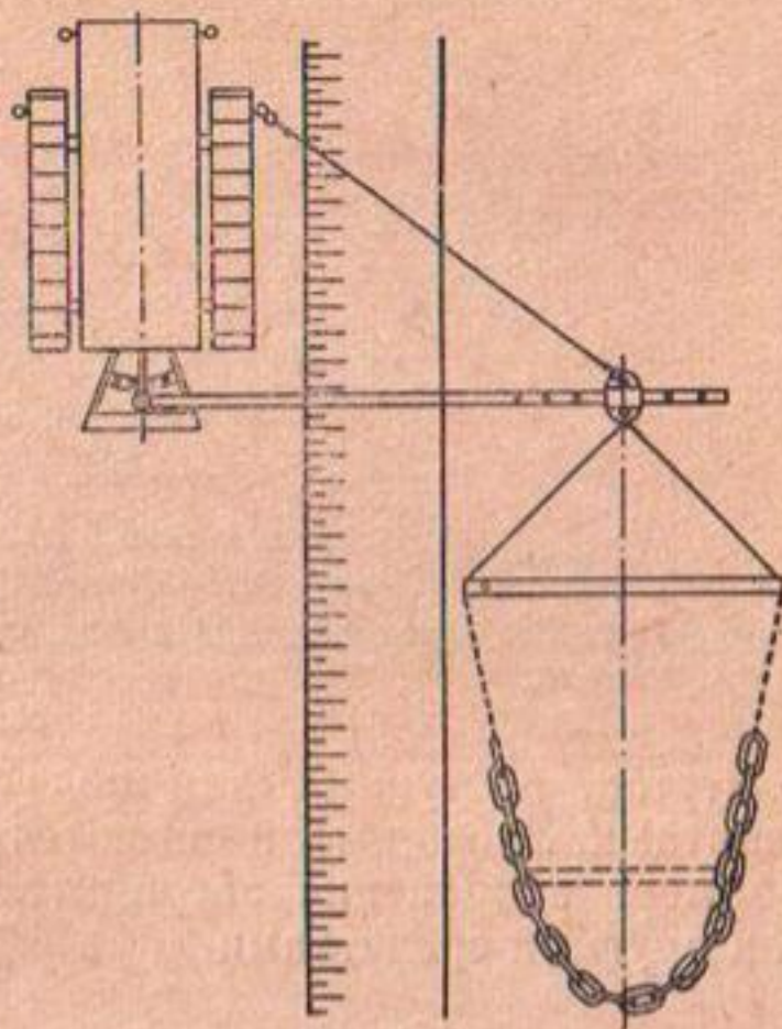
Рис. 37. Цепная драга для среза растительности на дне канала.
