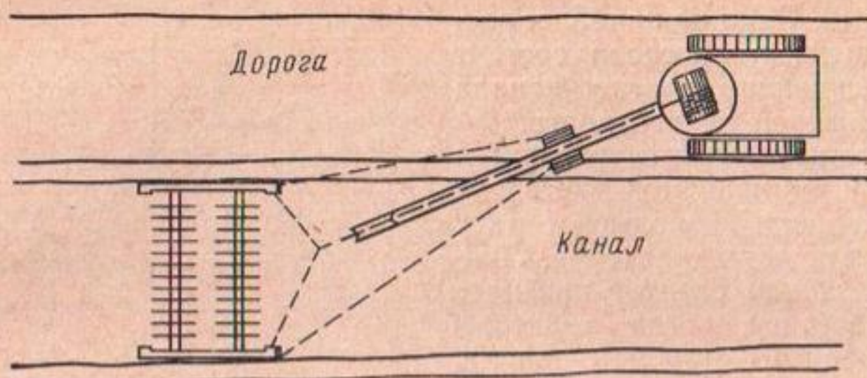
Рис. 38. Дискосая драга для срезки растительности на дне канала.
