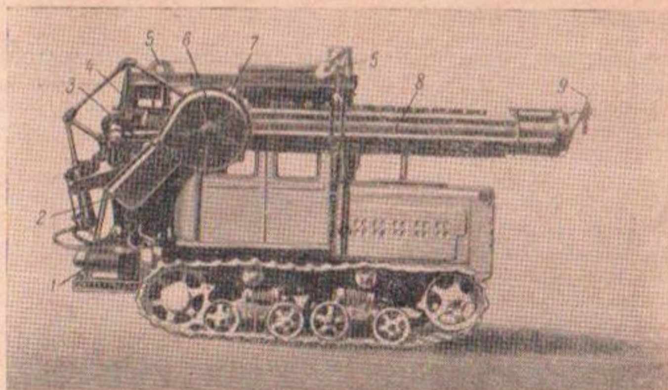
Рис. 28. Общий вид шнекового каналаочистителя КШБ-2,4:
