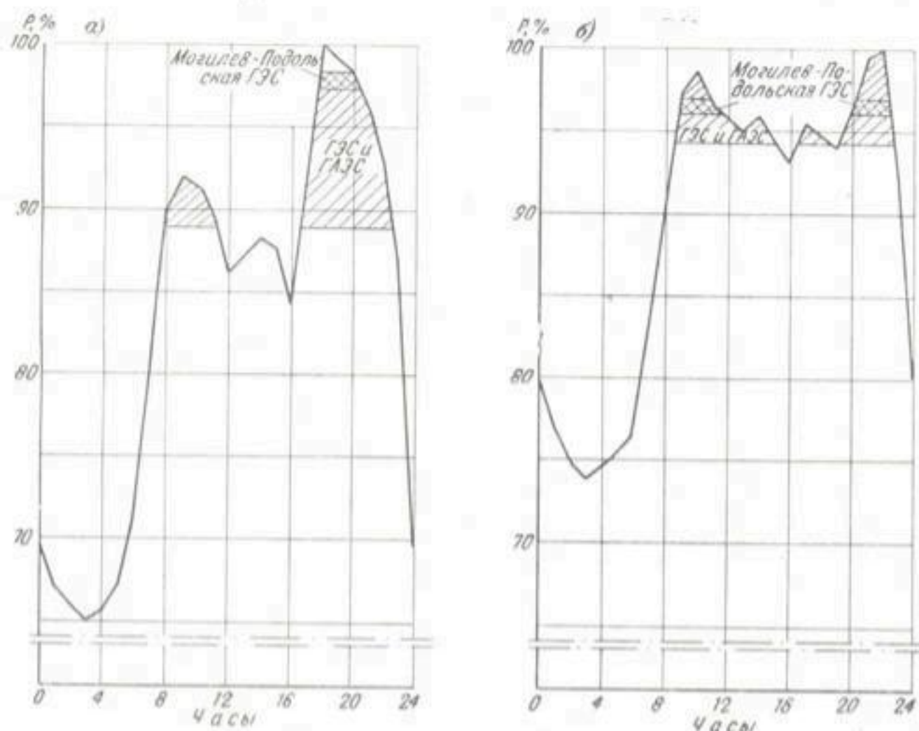
Рис. 1. Использование мощности Могилев-Подольской ГЭС в суточном графике нагрузки Объединенной энергосистемы Юга:
