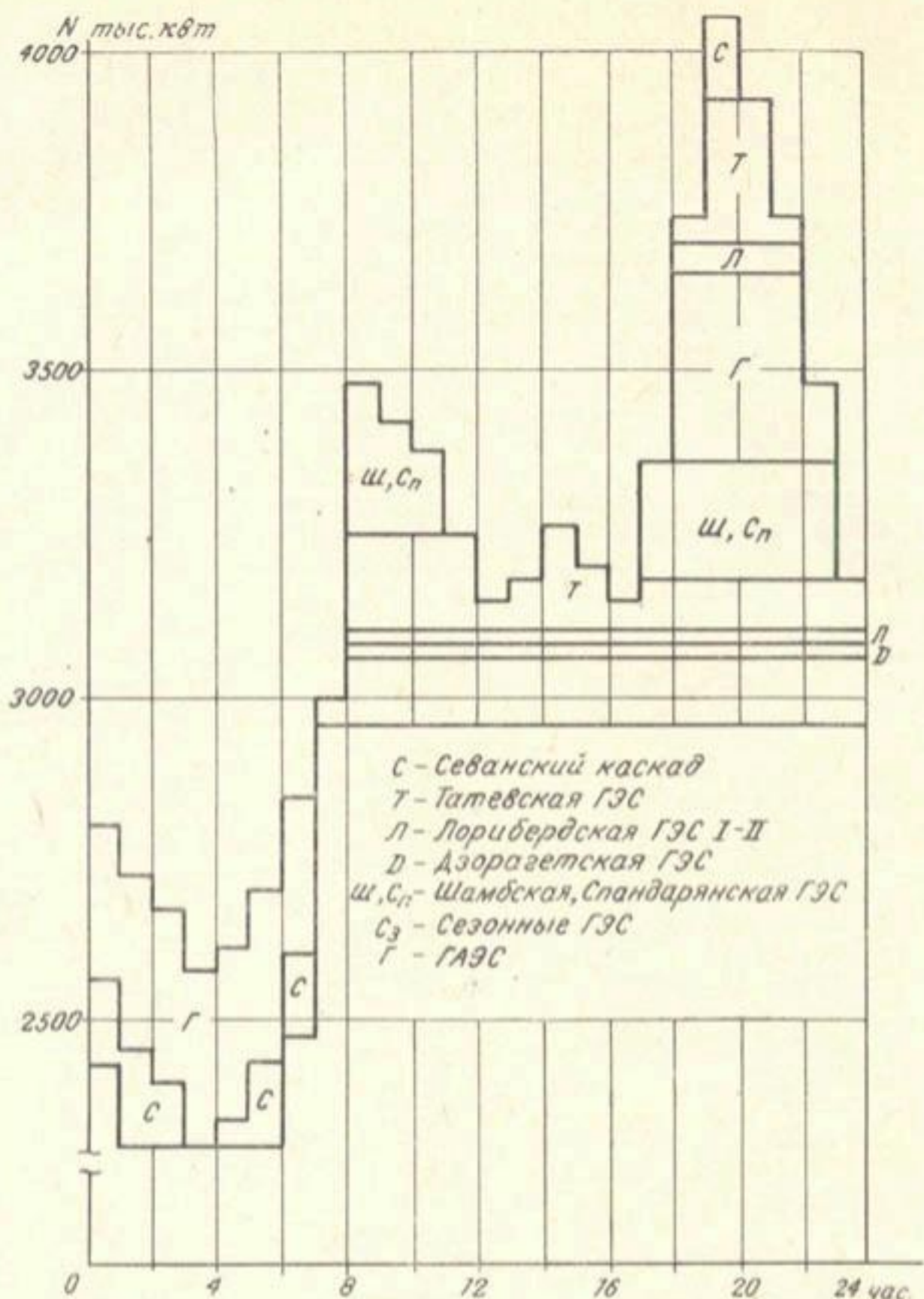
Рис. 1. Покрывание суточного графика нагрузки Армянской энергосистемы в перспективе, зима.
