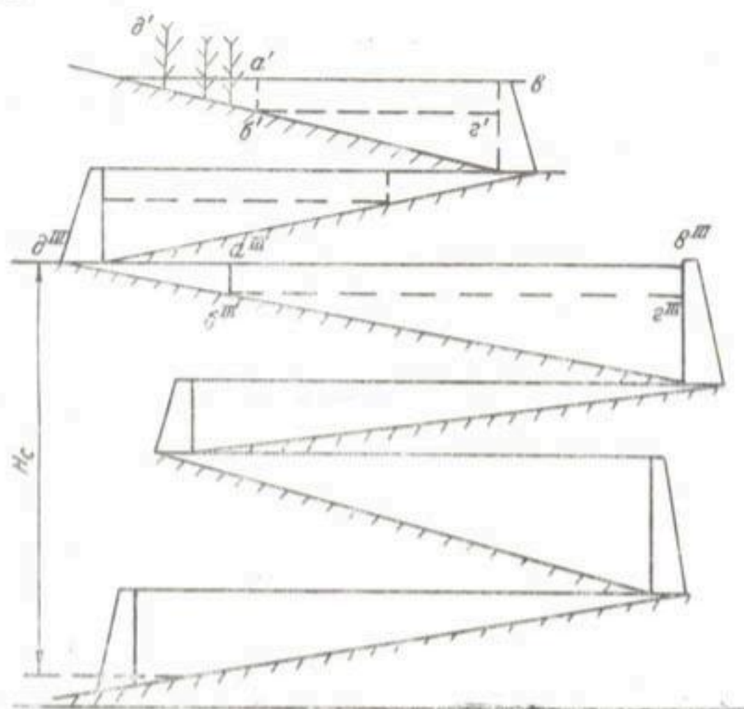
Схема выбора НПУ гидроузлов каскада.
