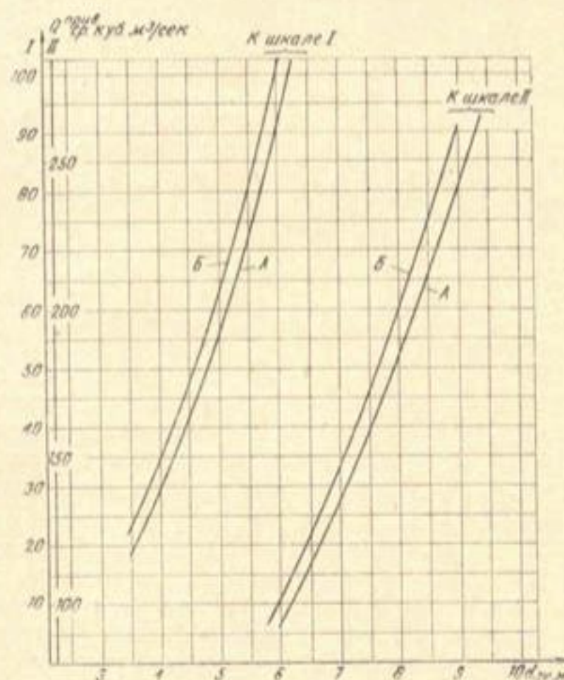
Рис. 4. Зависимость между Q_{ср.куб.} и экономическим диаметром туннеля:
