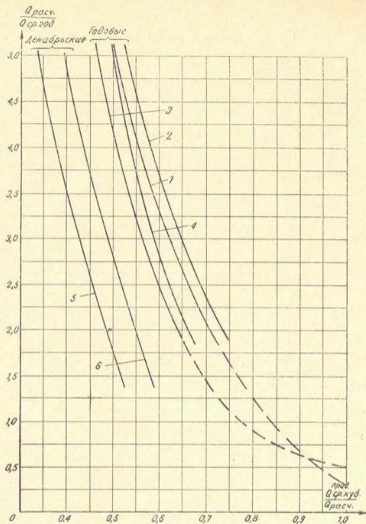
Рис. 1. Расчетные кривые для определения приведенных среднекубических расходов:
