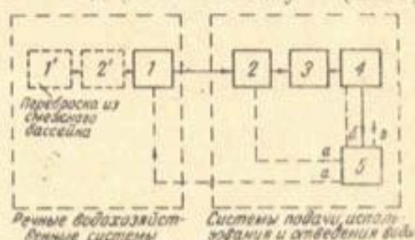
Рис. 1. Регулирование и территориальное перераспределение стока.
