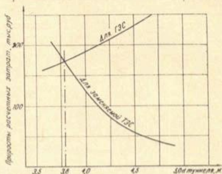
Рис. 3. Определение d_{э\kappa} построением кривых приростов расчетных затрат.
