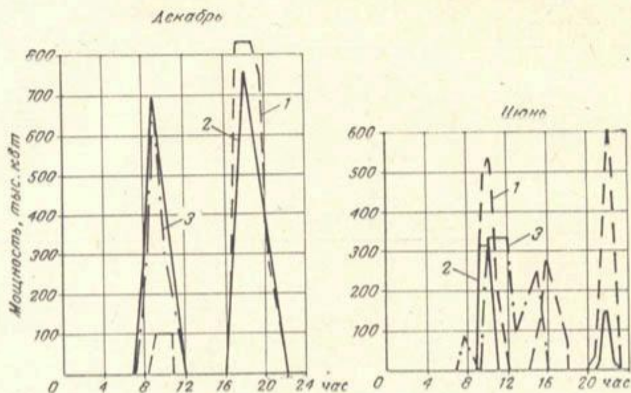
Проектный и фактический режим работы Плявиньской ГЭС (маловодный год):
