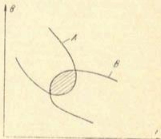
Рис. 2. Области оптимальных параметров канала.
