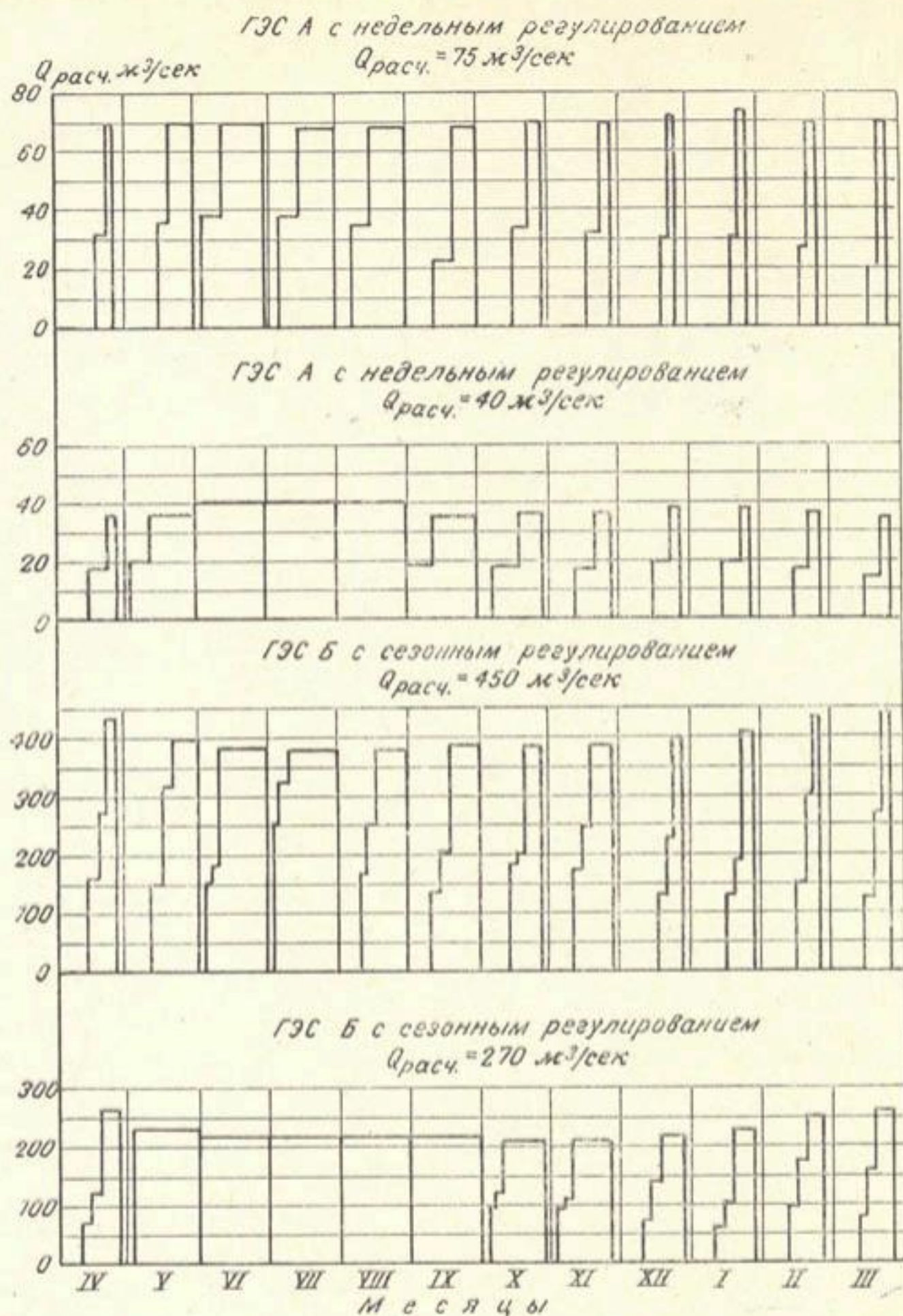
Рис. 2. Суточные режимы ГЭС.
