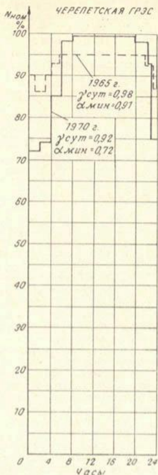
Зимние суточные графики нагрузок ГРЭС.
