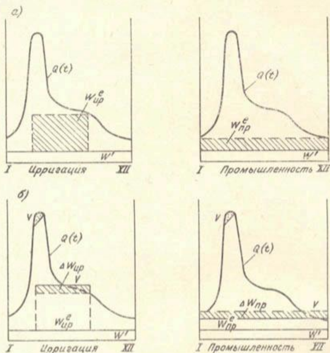
Рис. 2. К определению расчетной отдачи реки:
