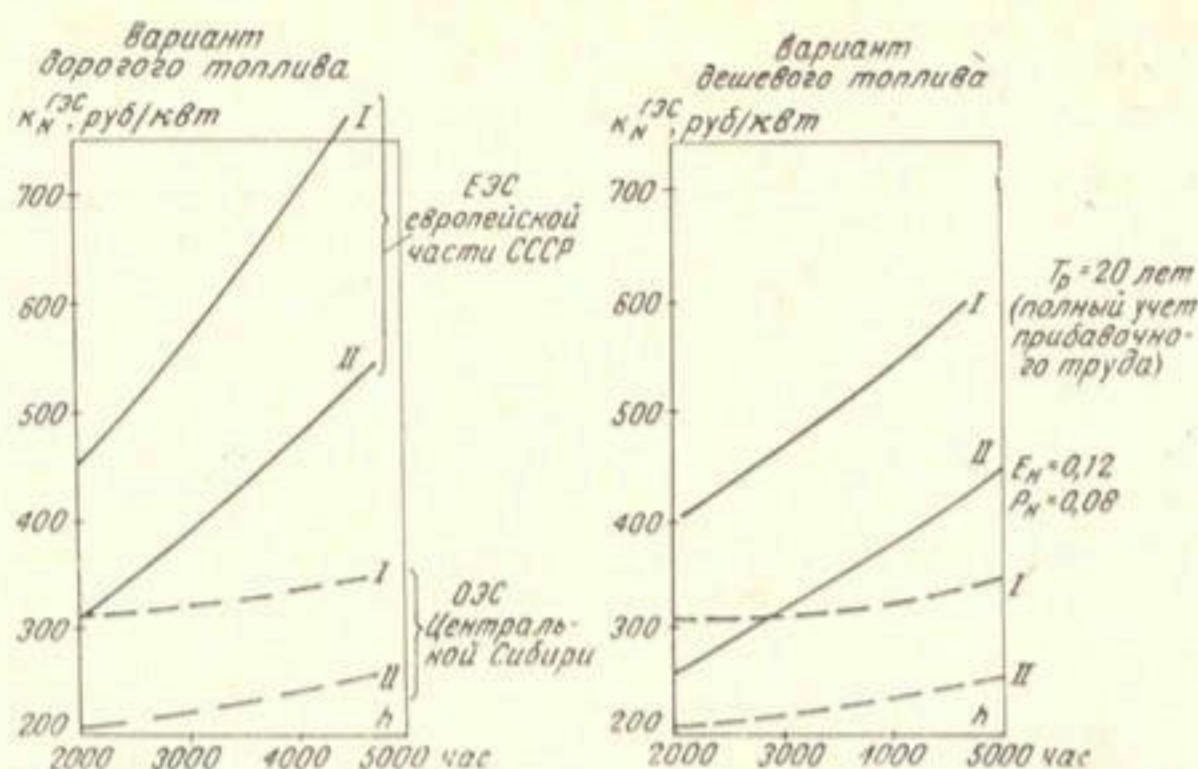
Рис. 4. Влияние затрат на топливо, числа часов использования и критерия экономичности на допустимые капиталовложения в ГЭС.
