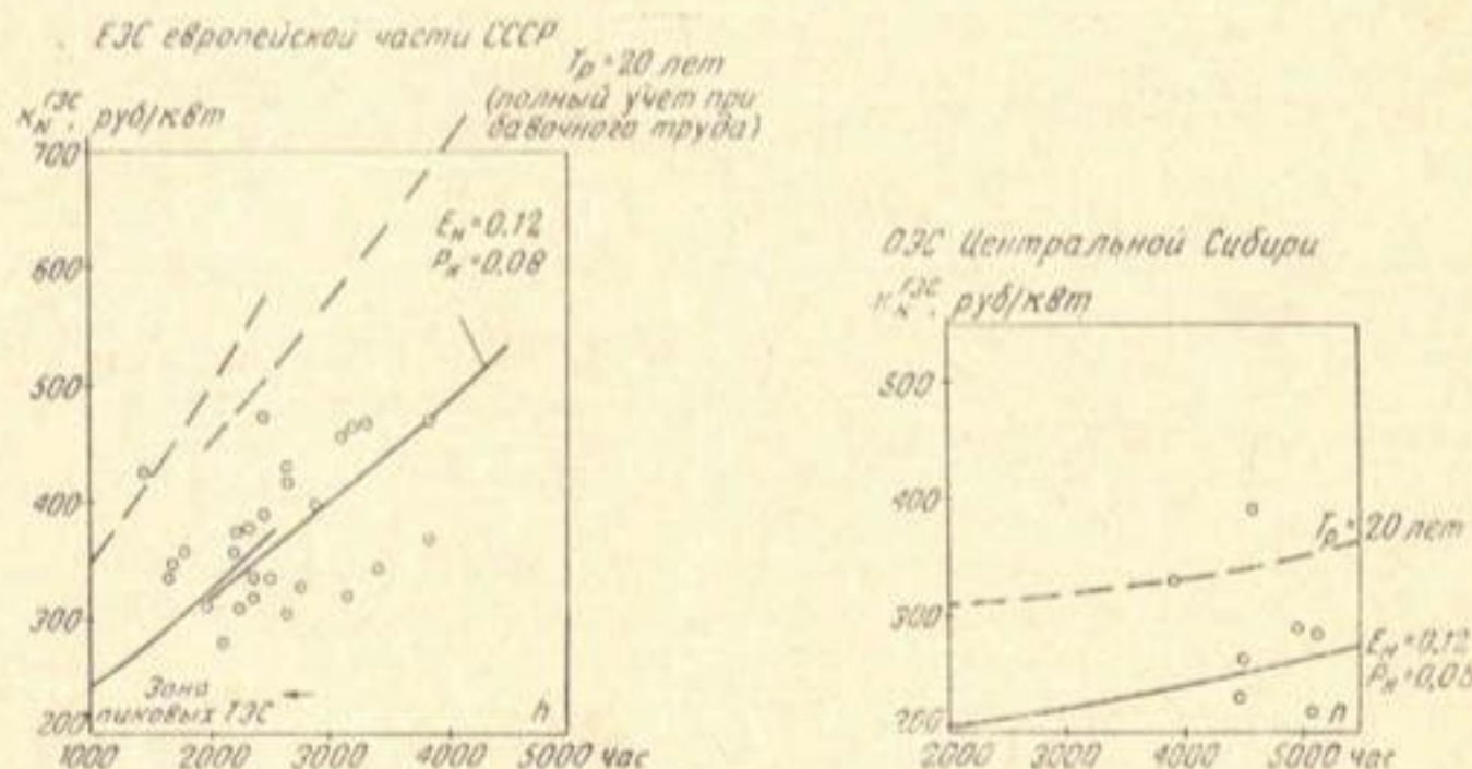
Рис. 3. Экономически допустимые капиталовложения на строительство ГЭС. Точками обозначены удельные капиталовложения по ряду строящихся и проектируемых ГЭС.
