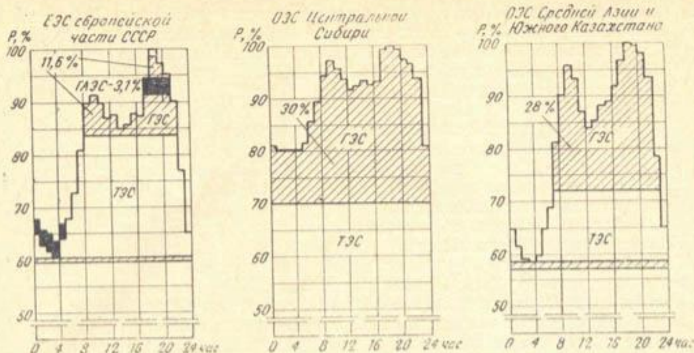
Рис. 1. Удельный вес ГЭС в покрытии пиковой части графиков нагрузки основных энергосистем СССР.
