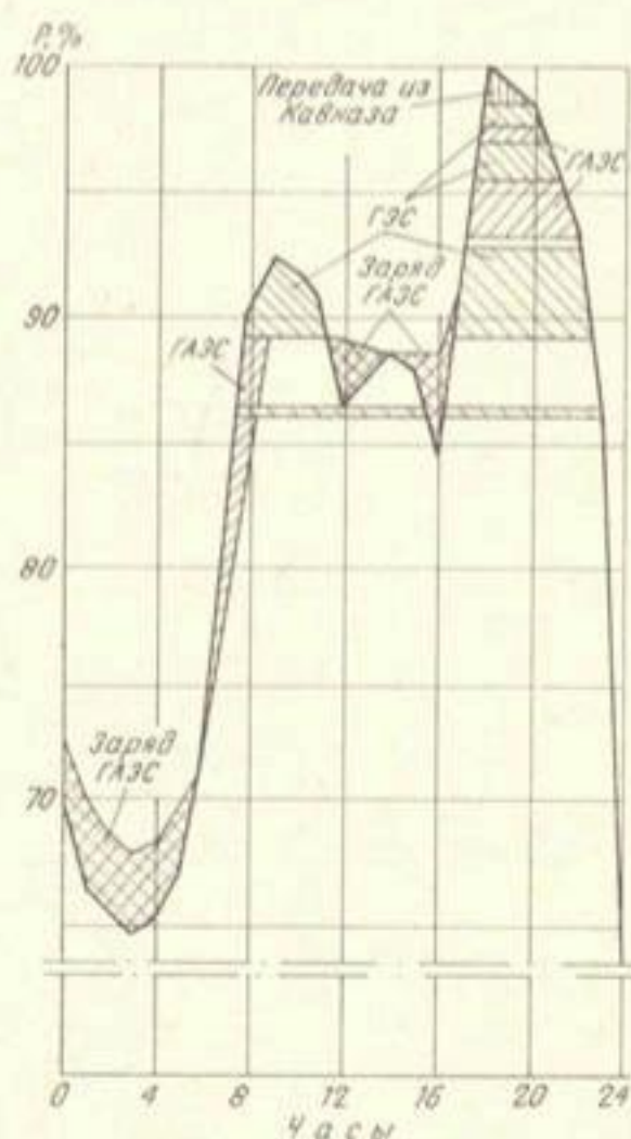
Покрывание суточного графика нагрузки ОЭС Юга за максимальный день (зима).
