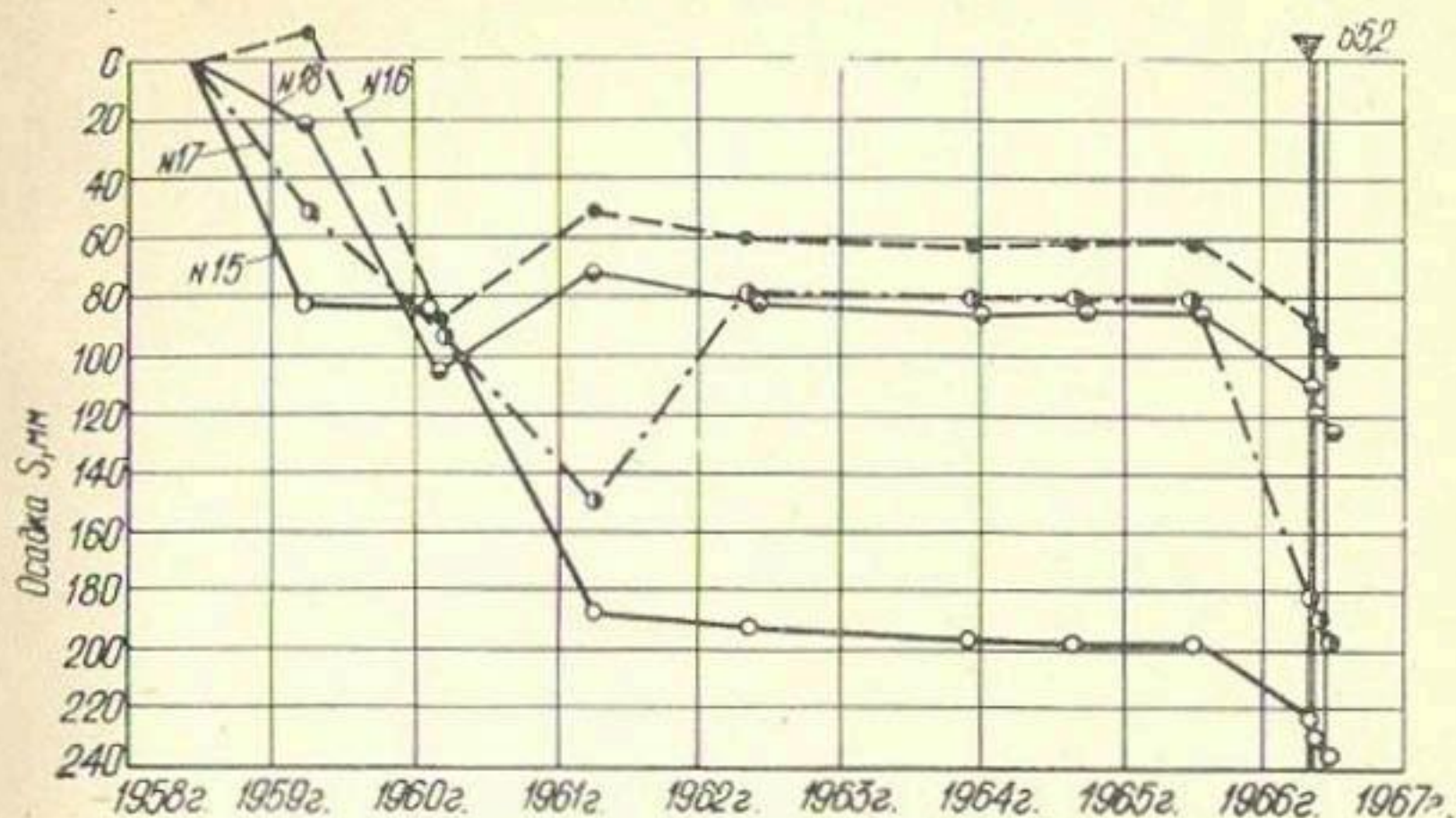
Рис. 1.15. Осадки гребня Шейхантаурской плотины по реперам 15—18 до и после землетрясений 26/IV и 9—10/V 1966 г.
