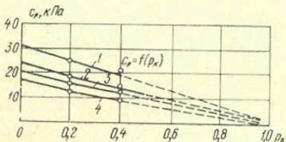
Рис. V.14. Зависимость сцепления на разрыв смеси c_p^{cm} от \rho_k при постоянных значениях плотности и влажности мелкозема 1 — \rho_{sk} = 1.7 г/см 3 ; W = 15\% ; 2 — \rho_{sk} = 1.6 г/см 3 ; W = 15\% ; 3 — \rho_{sk} = 1.7 г/см 3 ; W = 18\% ; 4 — \rho_{sk} = 1.6 г/см 3 ; W = 18\%
