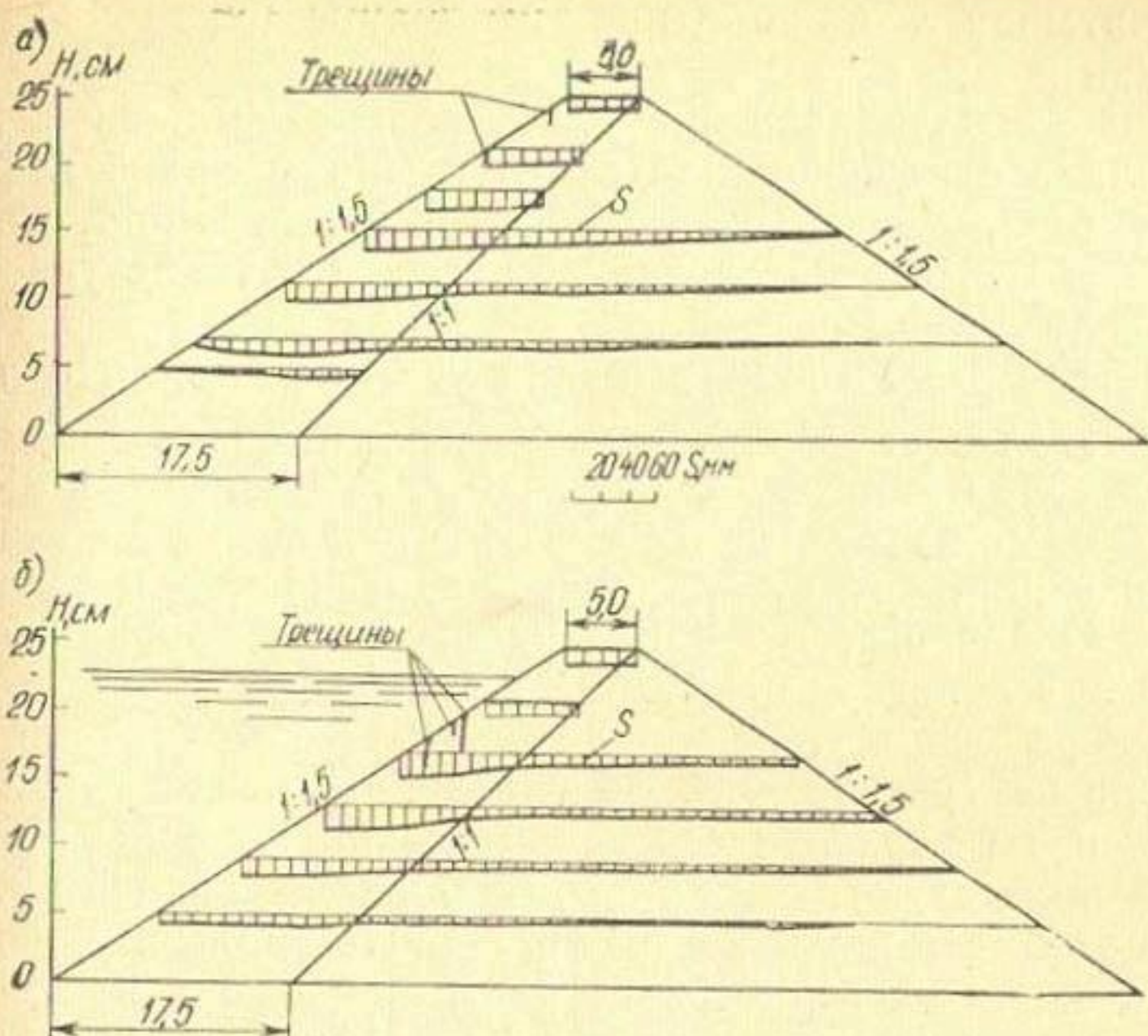
Рис. IV.13. Распределение вертикальных перемещений в поперечном сечении моделей плотин с экраном при отсутствии воды (а) и наличии воды в верхнем бьефе (б) для случая E_a < E_{пр}
