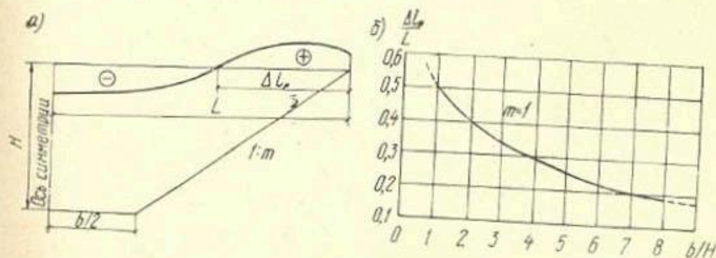
Рис. III.10. Схема определения параметров деформаций (а) и график изменения относительных размеров зон растяжений \Delta l_p/L в зависимости от отношения b/H при m=1 (б)
