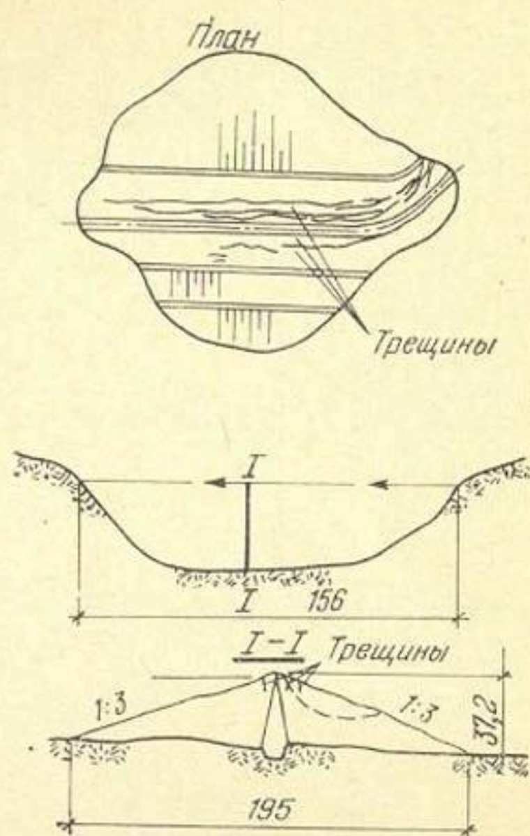
Рис. I.10. Плотина Оно
