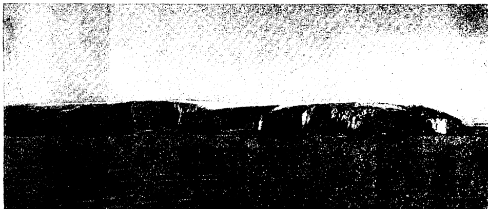
Рис. 26. Северный обрывистый берег оз. Балхаш
