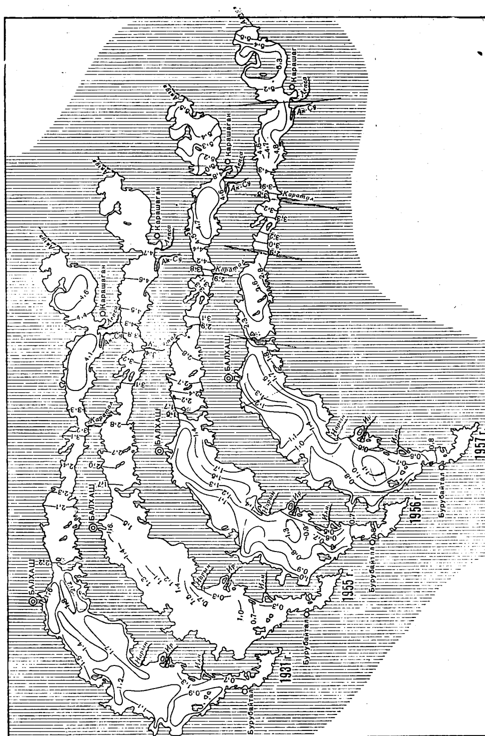
Рис. 55. Распределение минерализации в оз. Балхаш (в г/кг)
