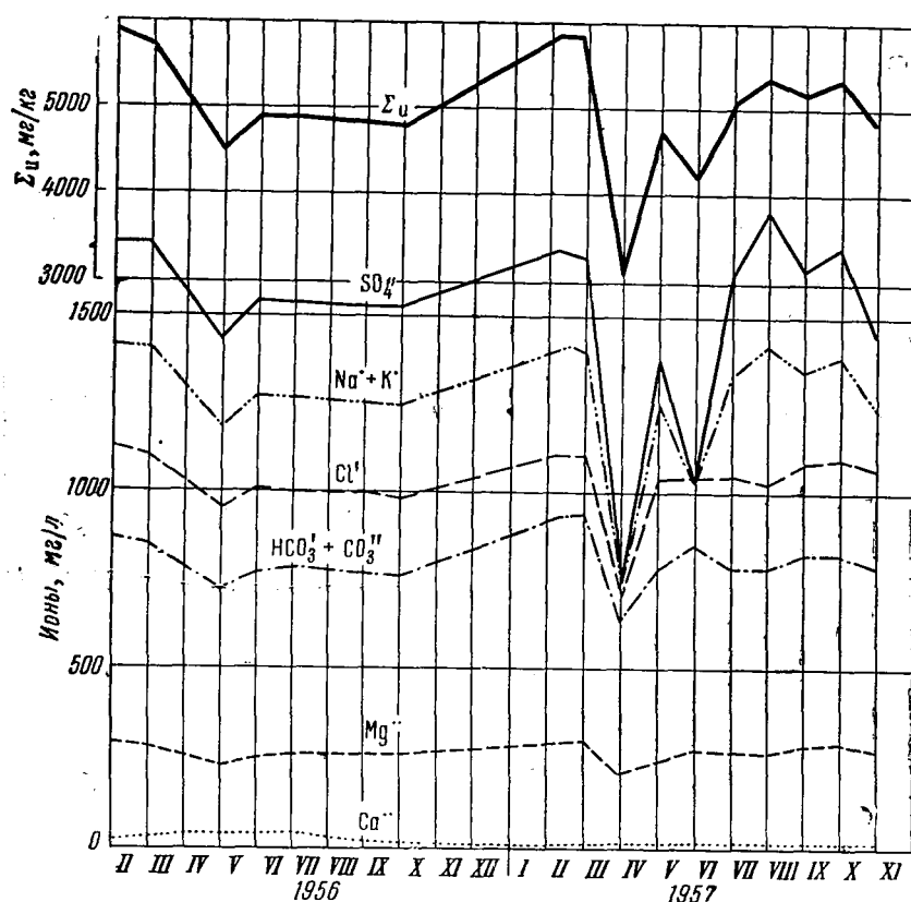
Рис. 63. Режим главных ионов и минерализации воды оз. Балхаш в заливе Карашаган (1956—1957 гг.)
