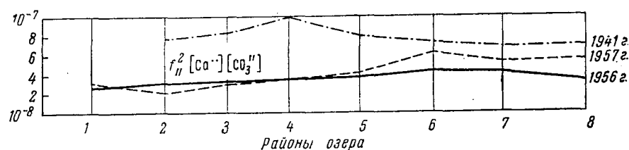
Рис. 71. Характер изменения произведений активностей \text{Ca}^{2+} и \text{CO}_3^{2-} по длине озера
