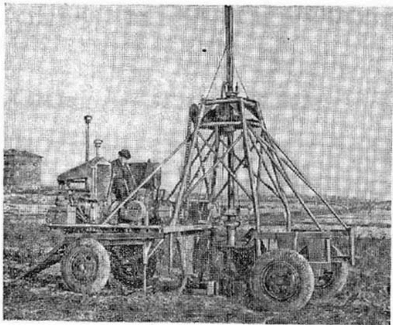
Агрегат КШК-30 для устройства шахтных колодцев.
