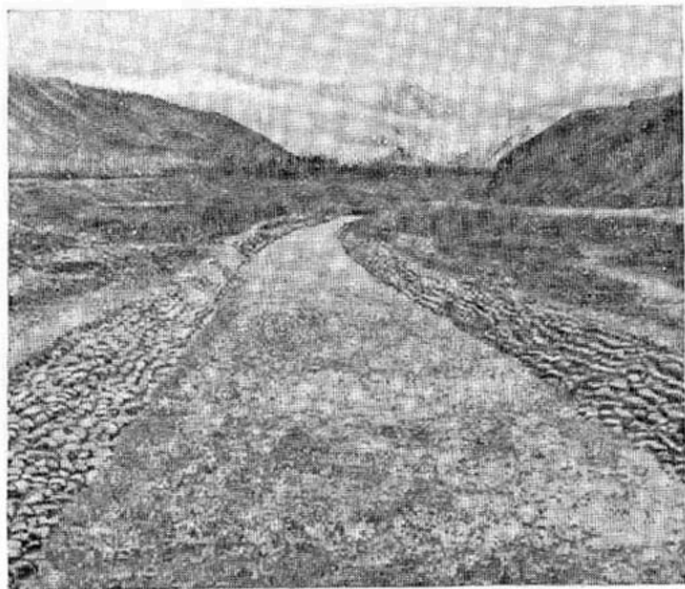
Каменистая отмостка каналов в Киргизской ССР.
