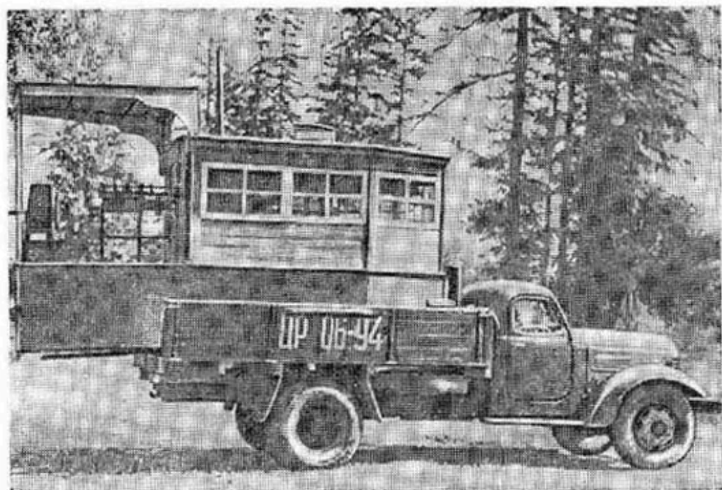
Землесосная установка 4ПЗУ-ВНИИГиМ. Транспортирование установки на автомашине ЗИС-150.
