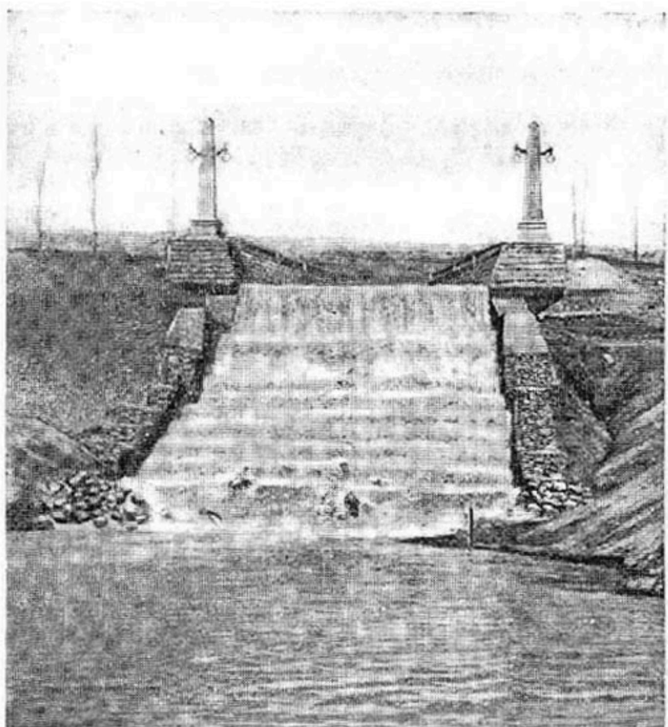
Концевой сброс верхнего магистрального канала в Тбилисское водохранилище.
