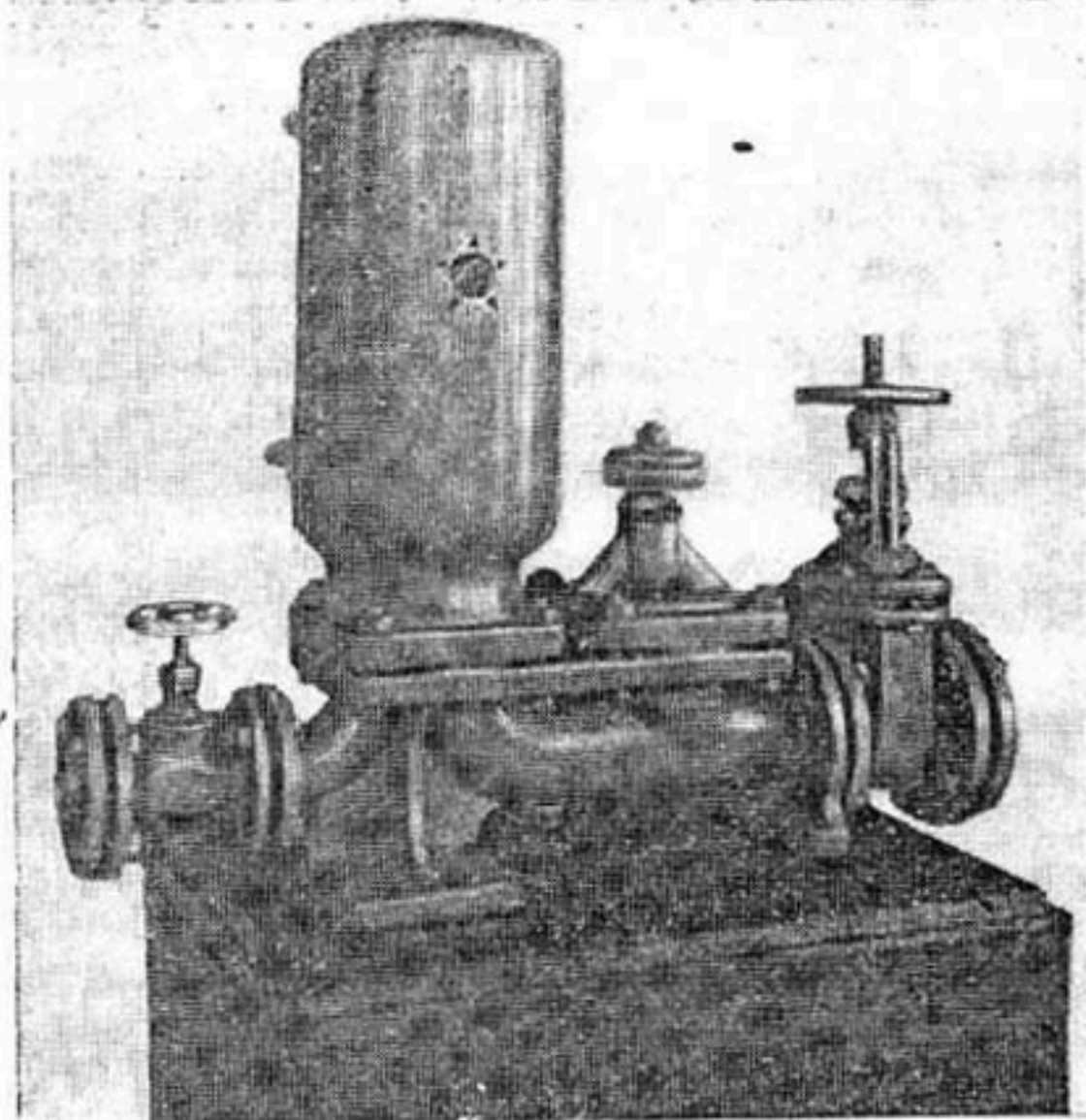
Гидравлический таран.
