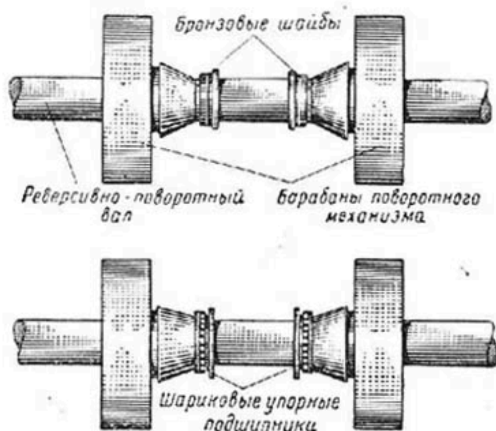
Ревверсивно-поворотный механизм экскаватора.
