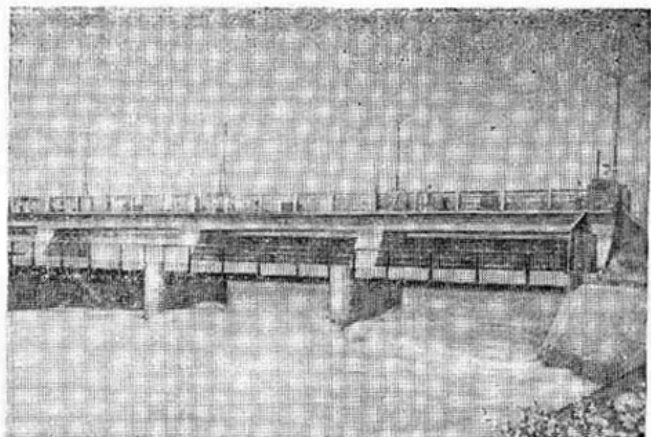
Главное сооружение Большого Гиссарского канала.
