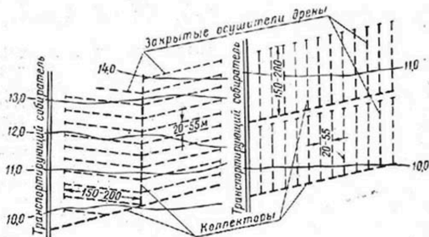
Схема расположения сети закрытого дренажа: слева—поперечный дренаж; справа—продольный дренаж.
