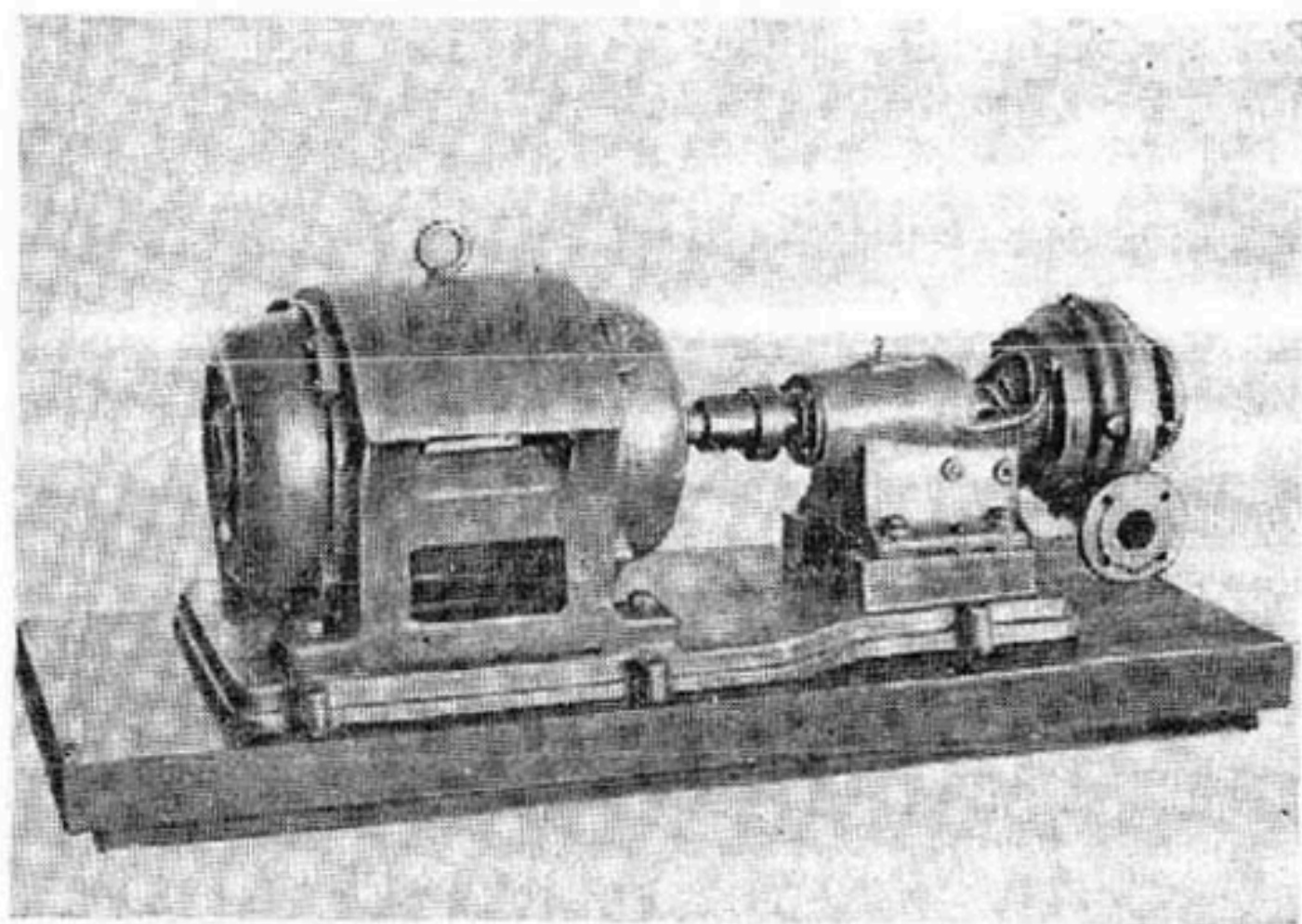
Центробежный консольный насос.
