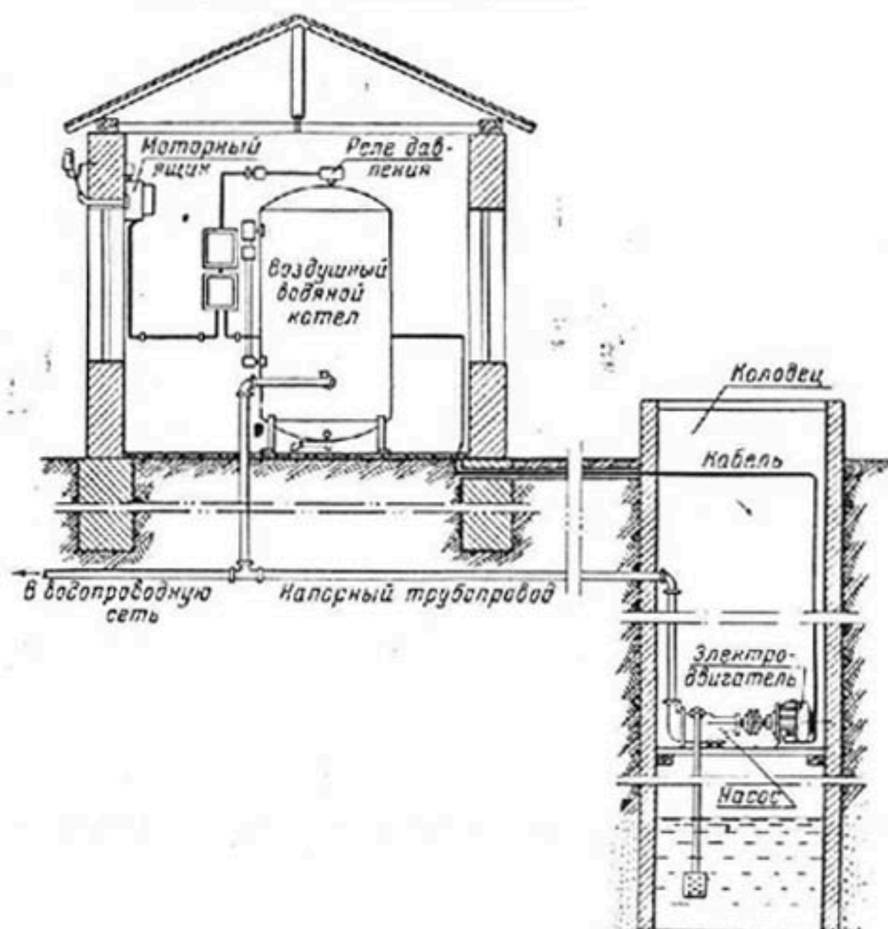
Безбашенная водокачка ВЭ-2,5.
