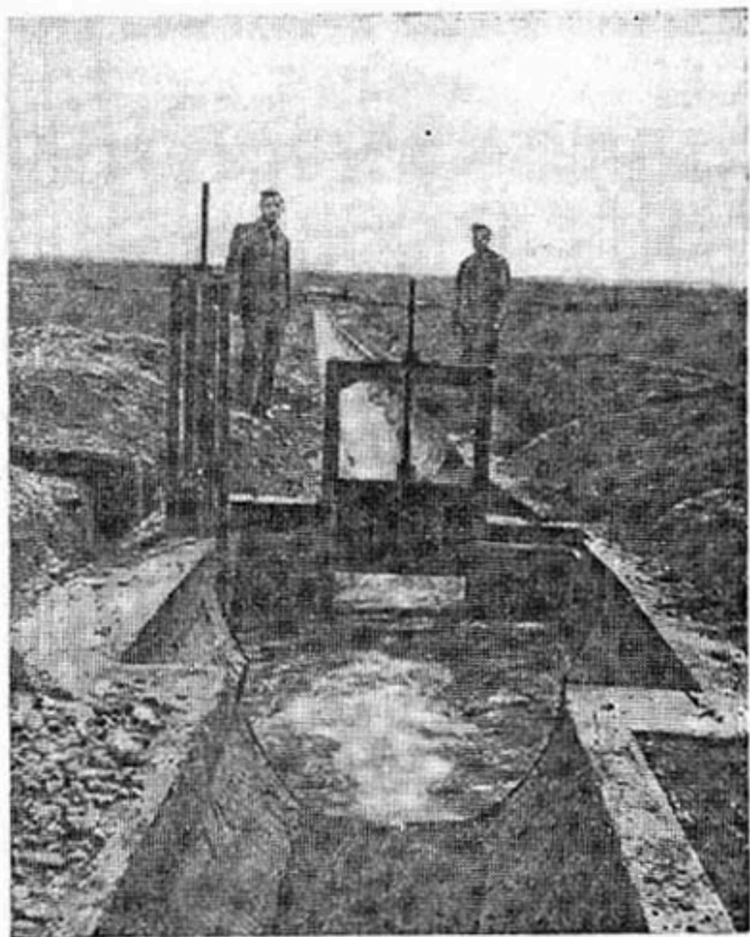
Облицовка каналов бетонными блоками-лотками (распределитель № 8 на Самгорской оросительной системе в Грузинской ССР).
