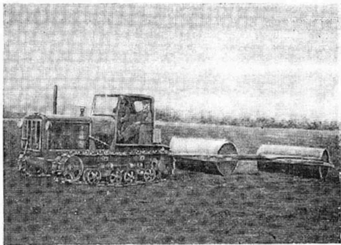
Катки КВГ-1,4 для прикатывания осушенных земель.
