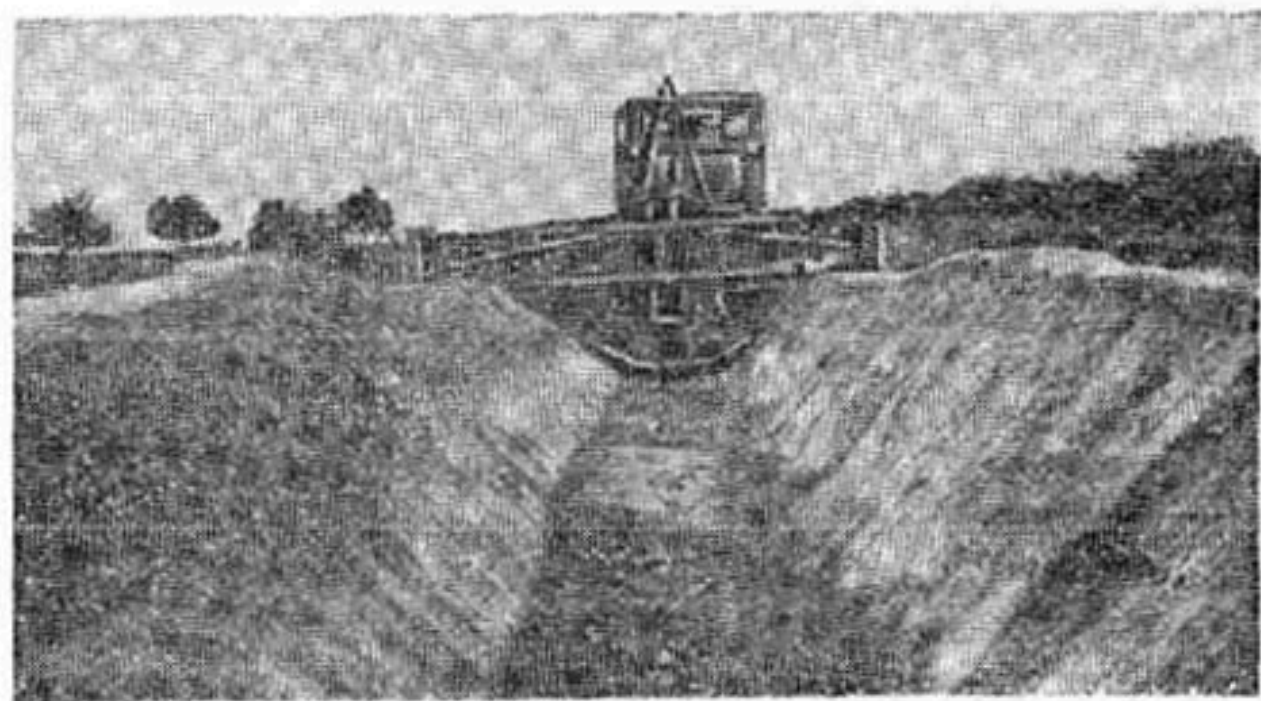
Плужный канавокопатель в работе.
