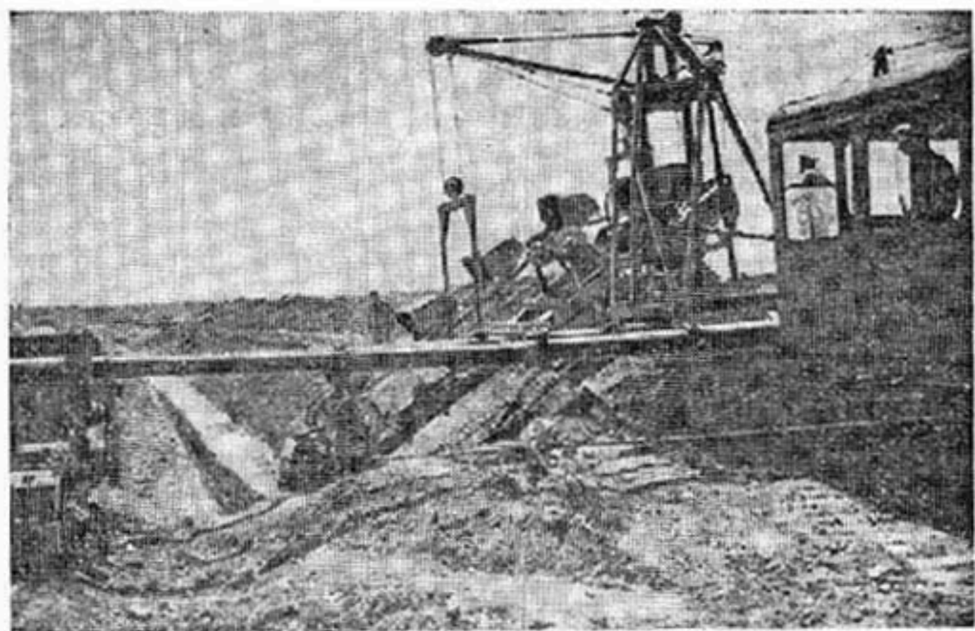
Многоковшовый мелпоративный экскаватор ЭМ-502 в работе.
