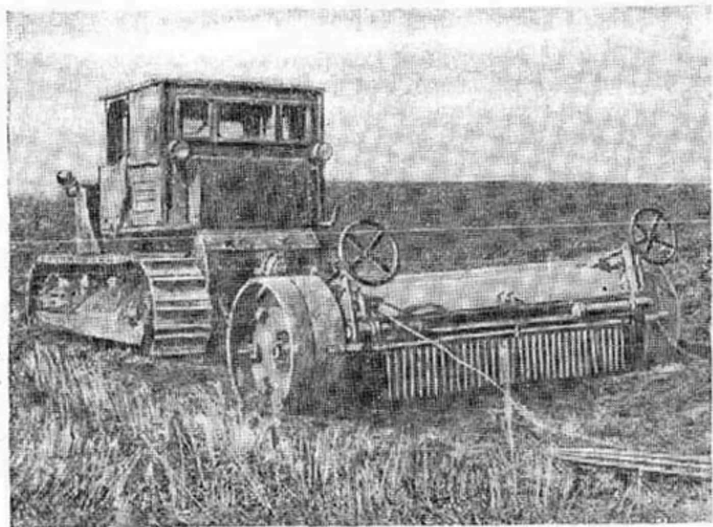
Фрезбарабаи ФБ-1,0.
