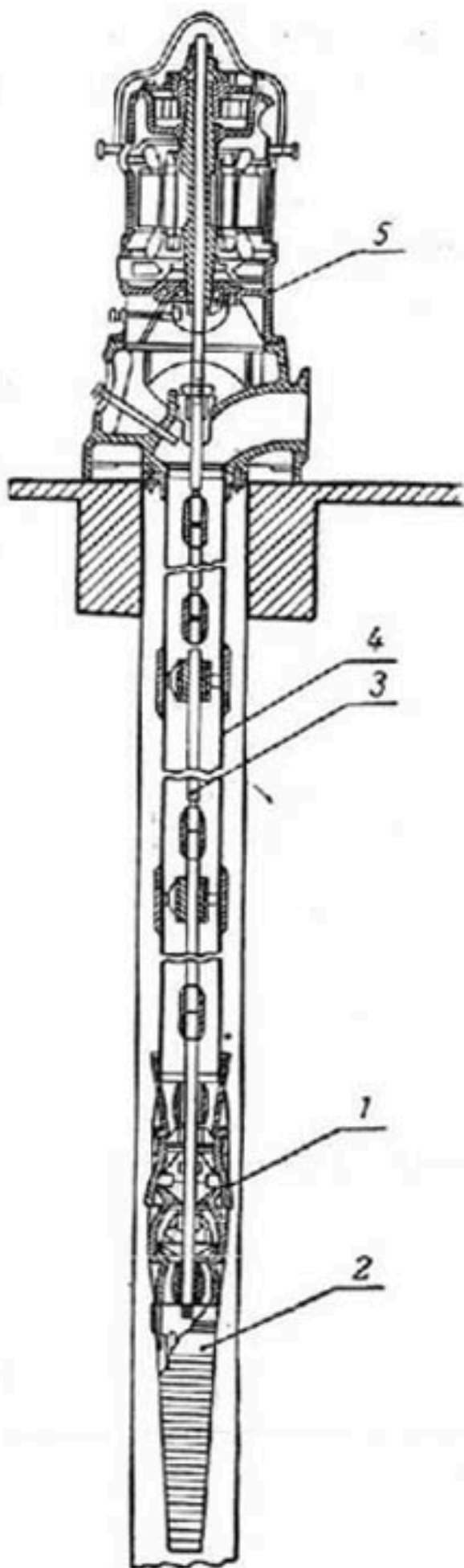
Общий вид установки насоса АТН в трубчатом колоде:
