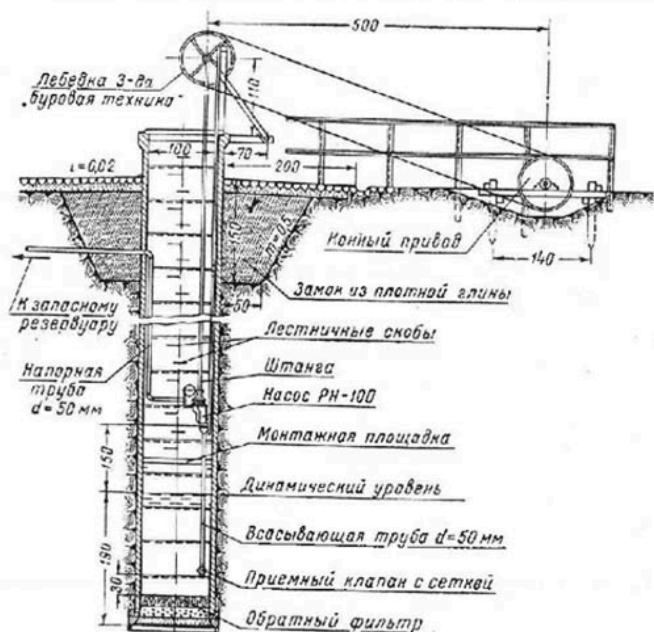
Насос РН-100 с конным приводом.
