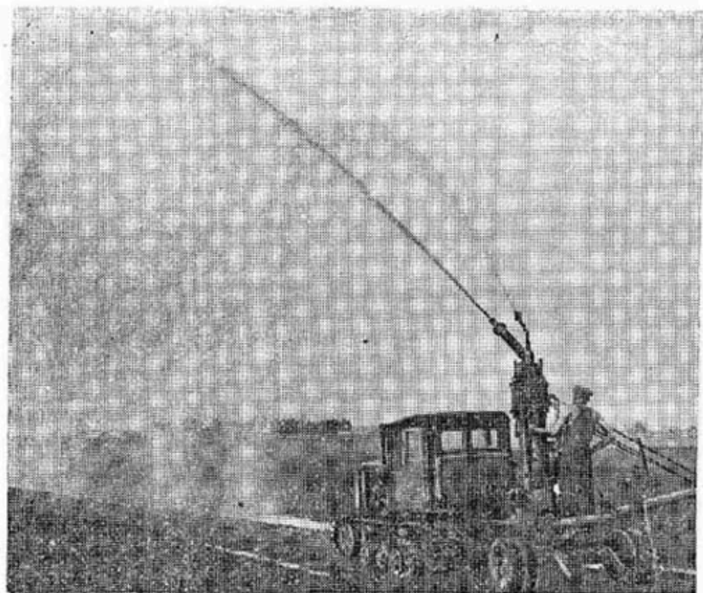
Дальноструйная дождевальная установка ДДП-30с в работе.
