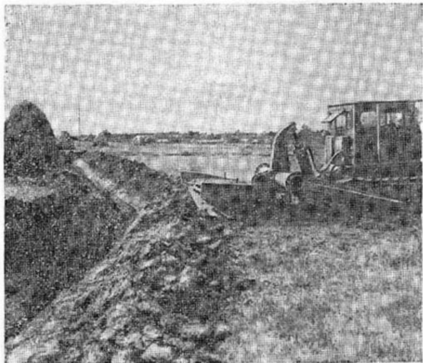
Навесная рама УМАС с канавокопателем КОР-500.
