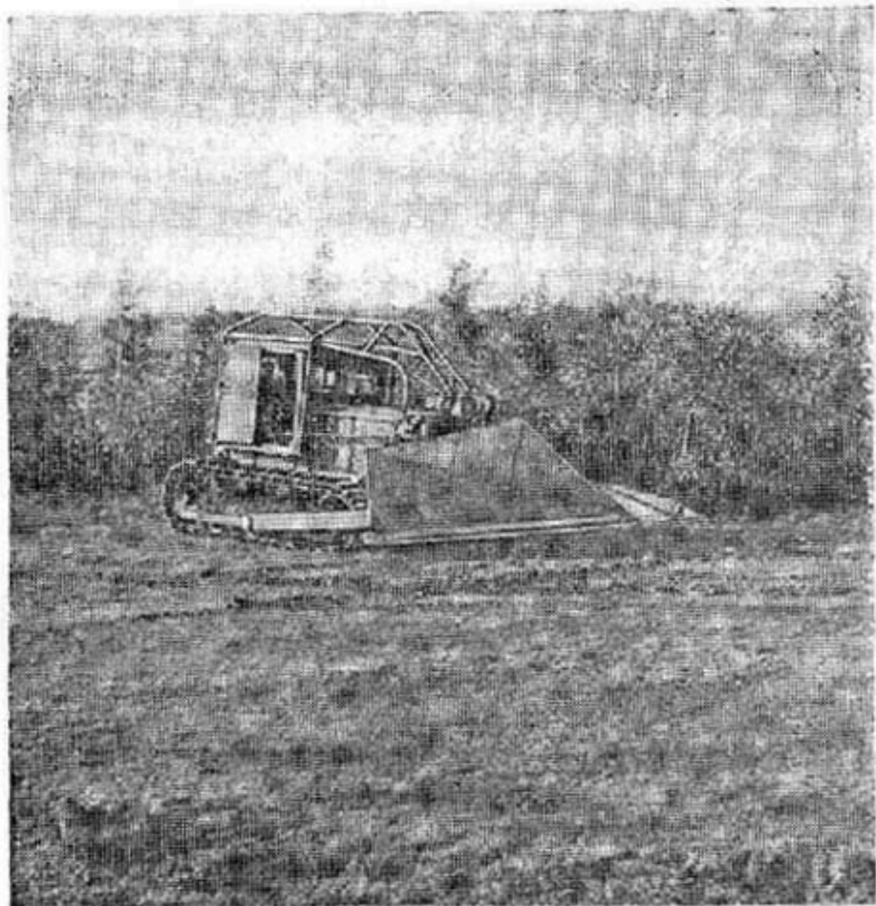
Кусторез Д-174В.
