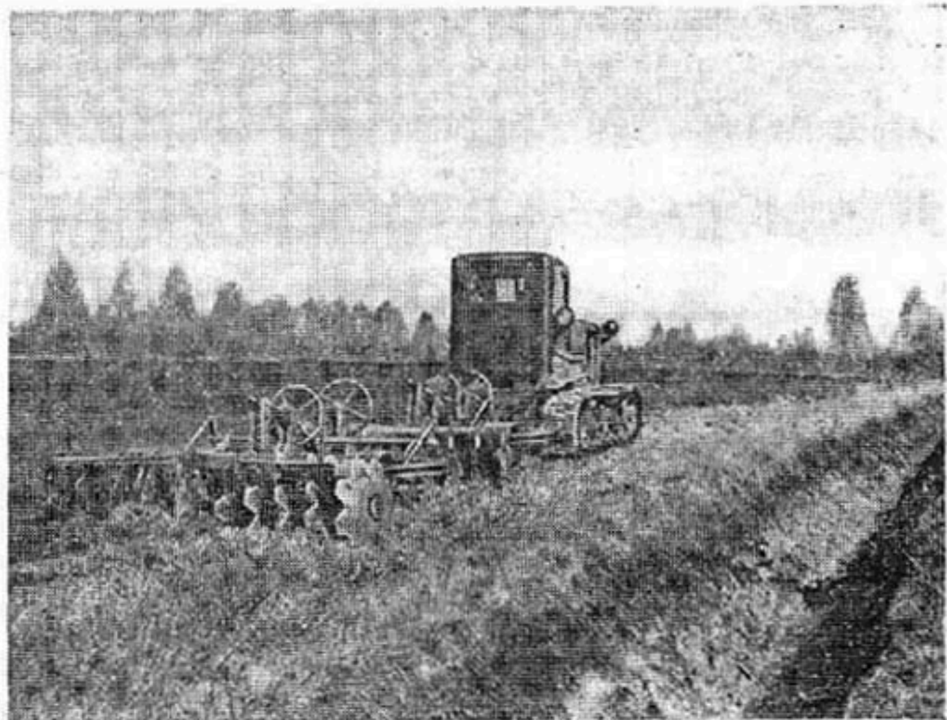
Тяжелая дисковая борона.
