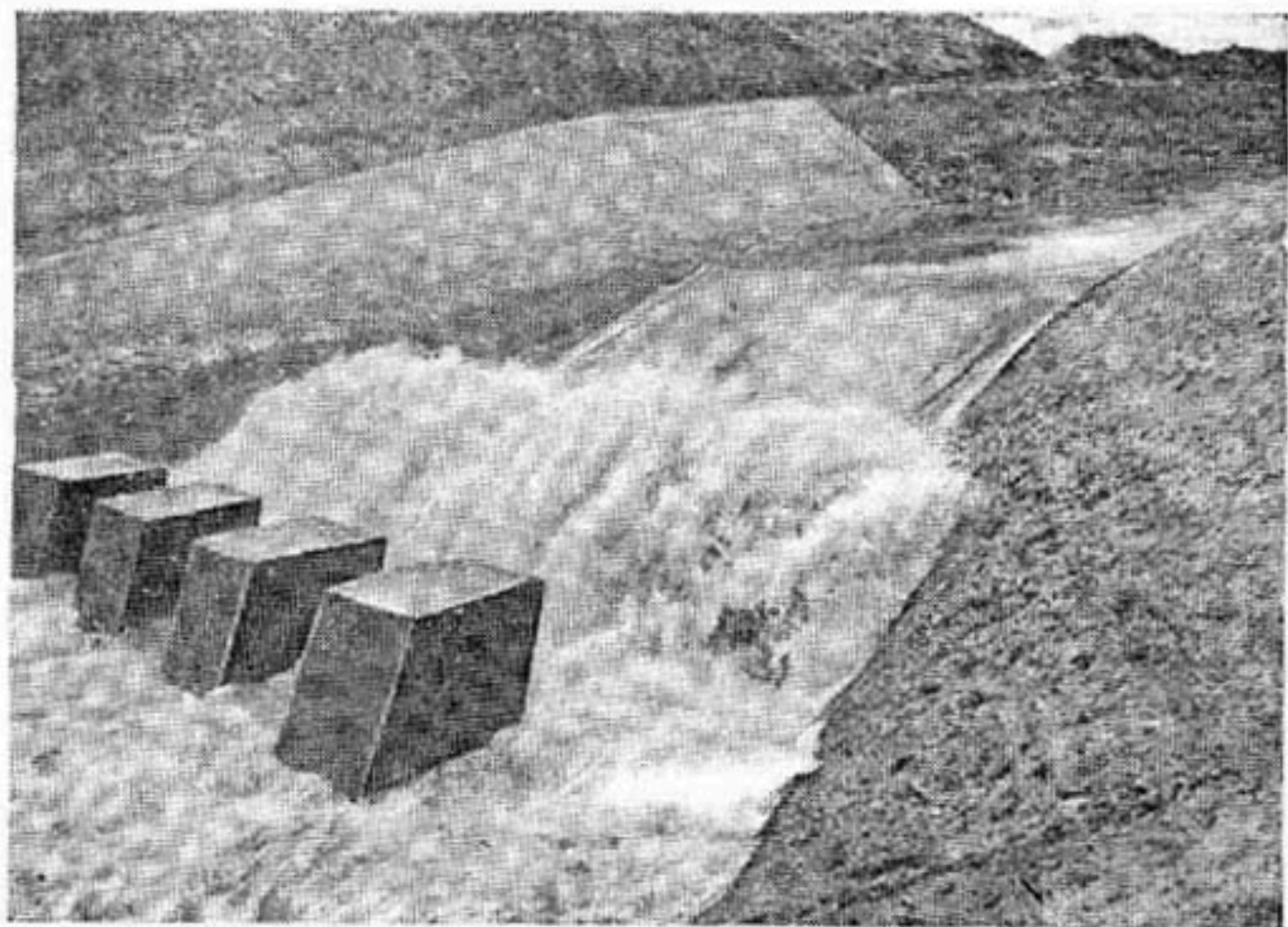
Перенад с гасителями на Северном Ферганском канале.
