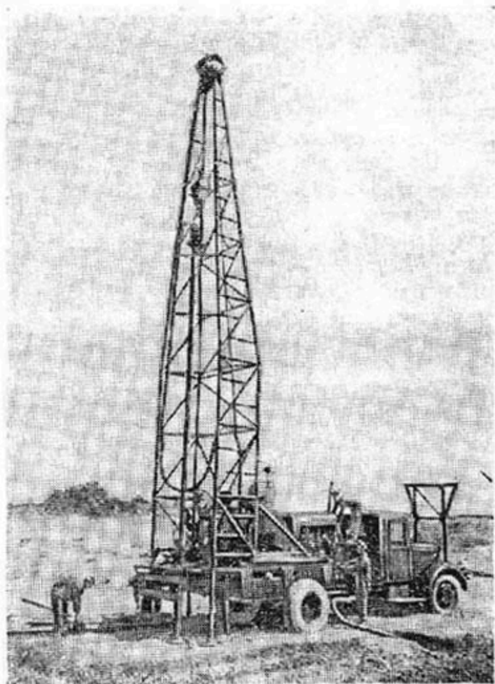
Буровой агрегат АВБ-400.
