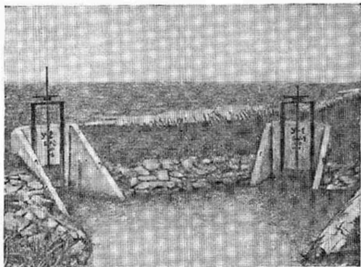
Трубчатые сборные сооружения на Ростовских оросительных системах.
