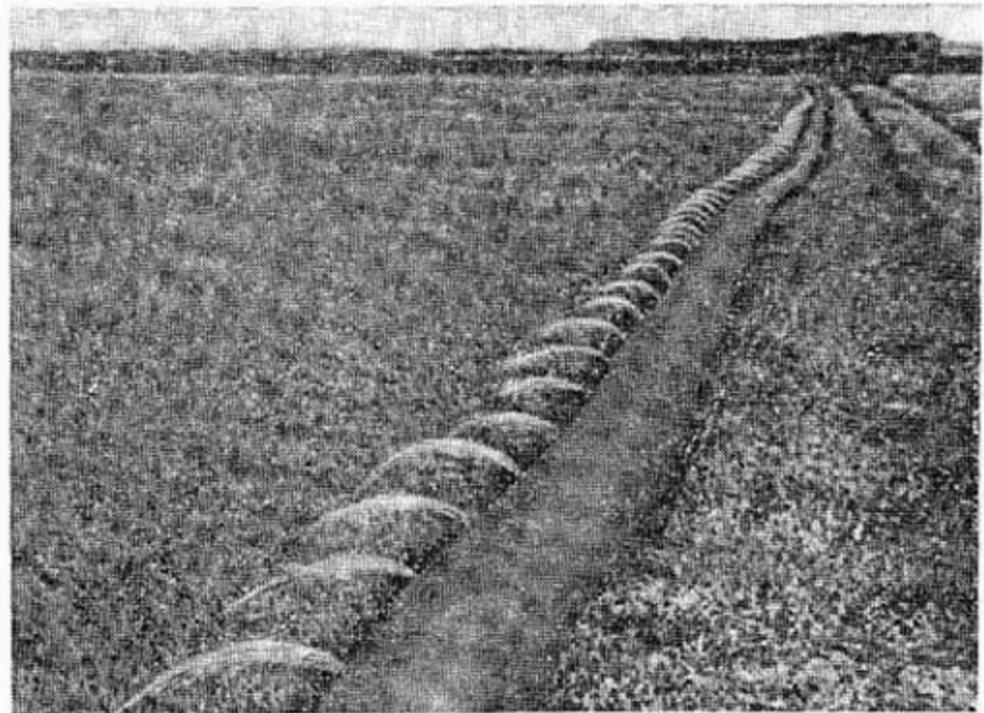
Гибкий тканевый поливной трубопровод.
