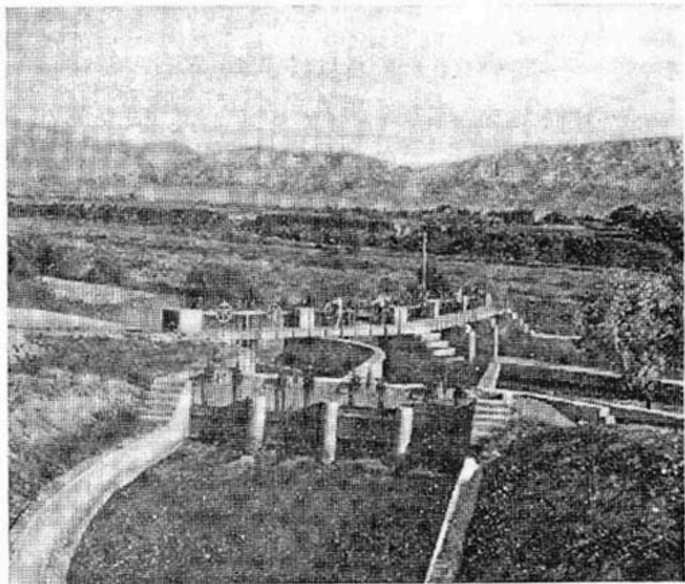
Пальманский вододелительный узел на р. Исфайраме Узбекской ССР.
