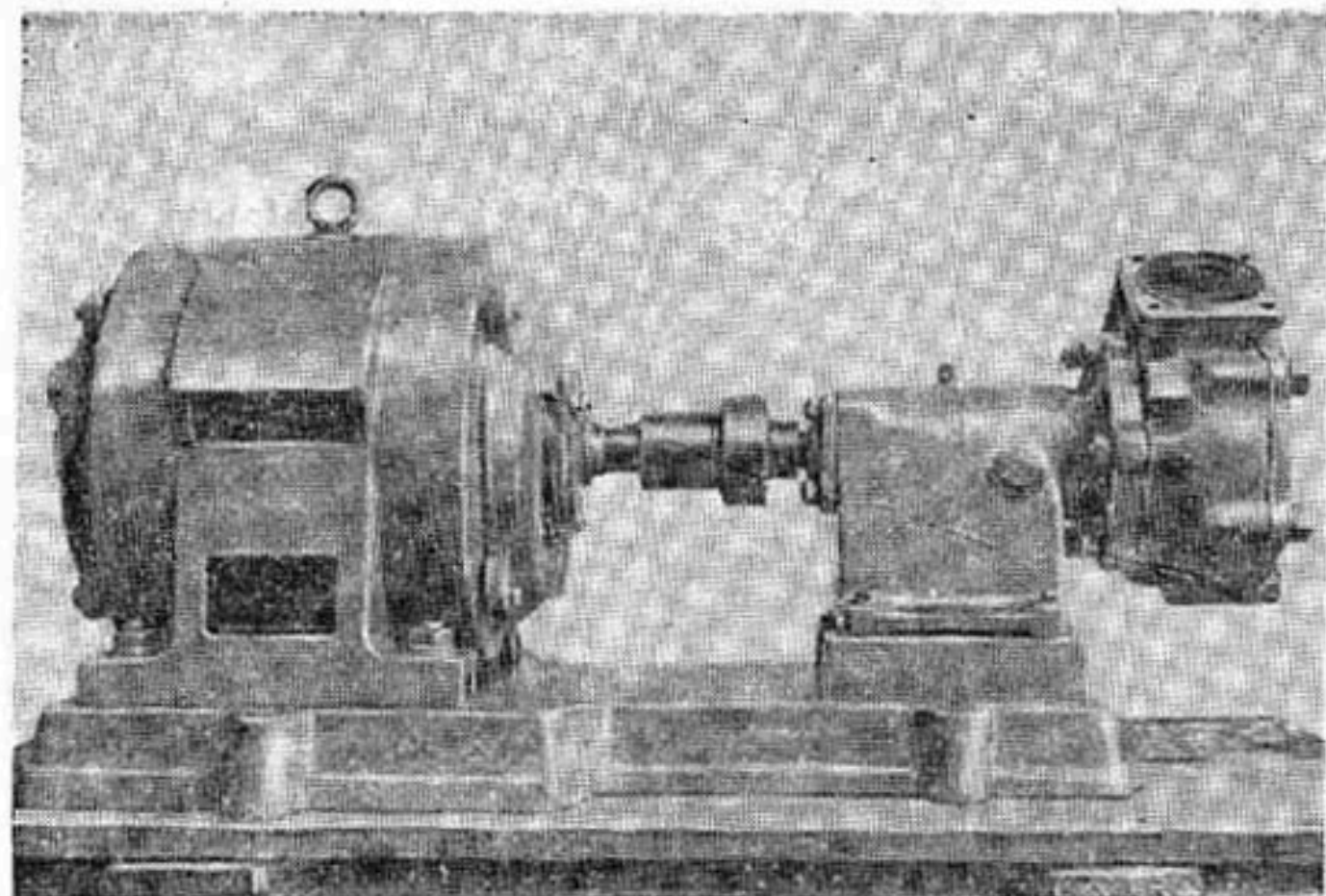
Вихревой насос 2В-1,6.
