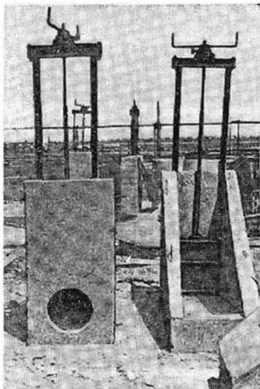
Открытые и трубчатые сборные сооружения с применением объемных блоков на Ингулецкой системе УССР.
