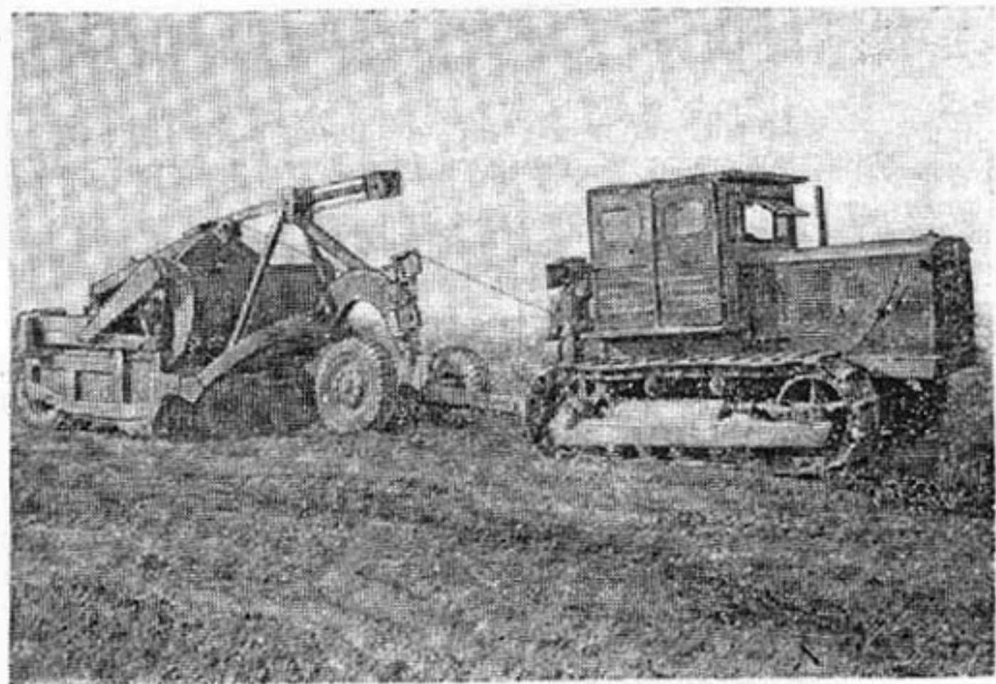
Скрепер Д-222 в работе.
