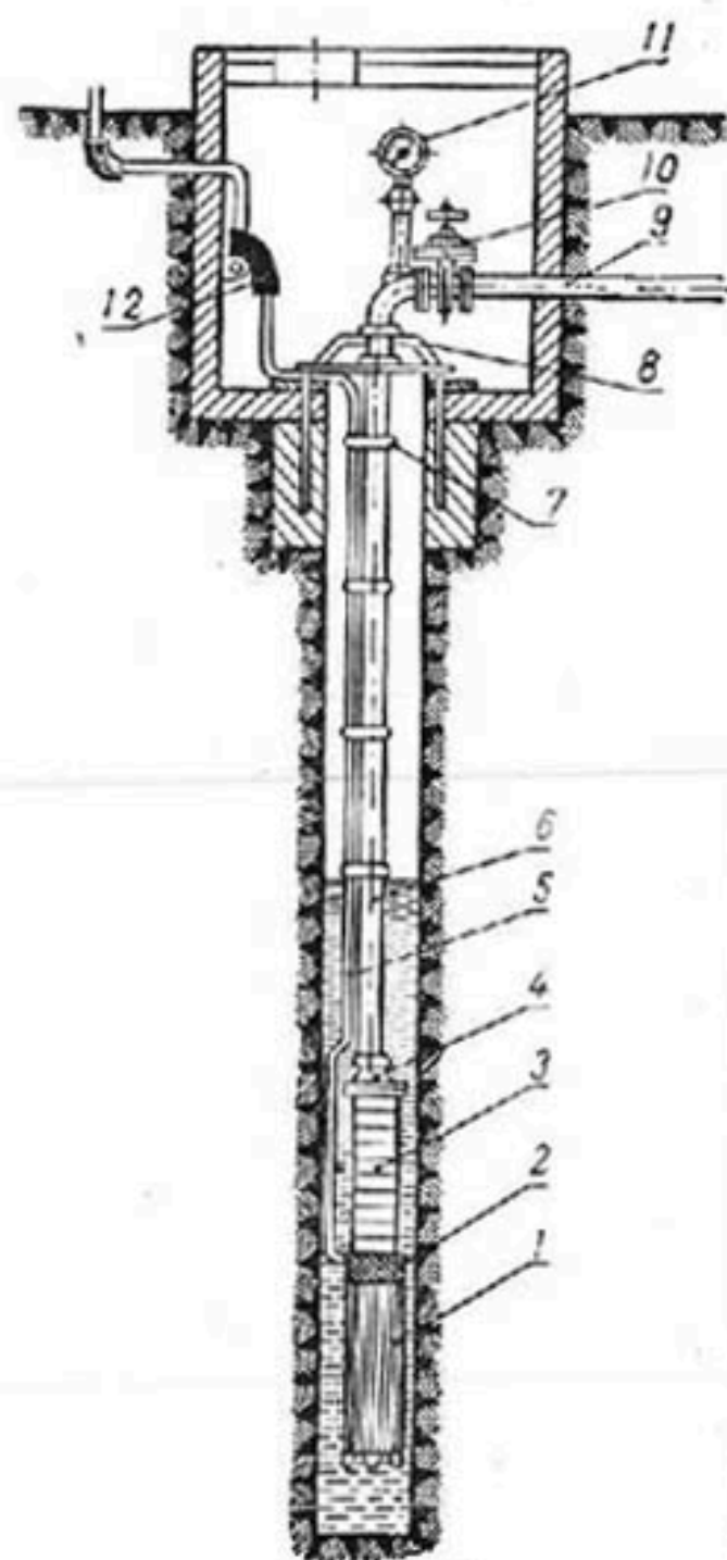
Общий вид установки погружного электронасоса АП в трубчатом колодце:
