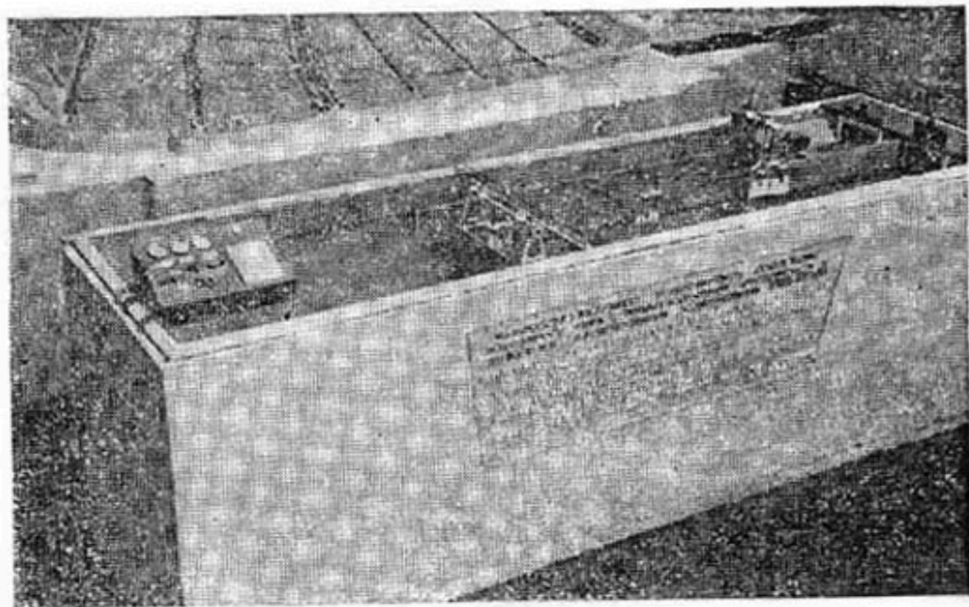
Модель наносорегулирующего водозаборного сооружения плотинного типа с многокамерным отстойником и донными промывными устройствами конструкции ВНИИГим.
