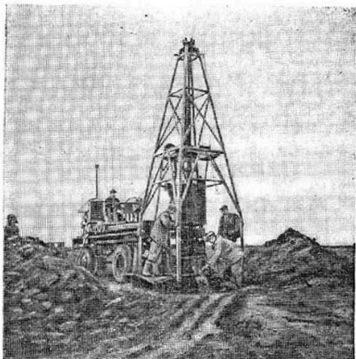
Работа агрегата КШК-25 при устройстве шахтного колодца.
