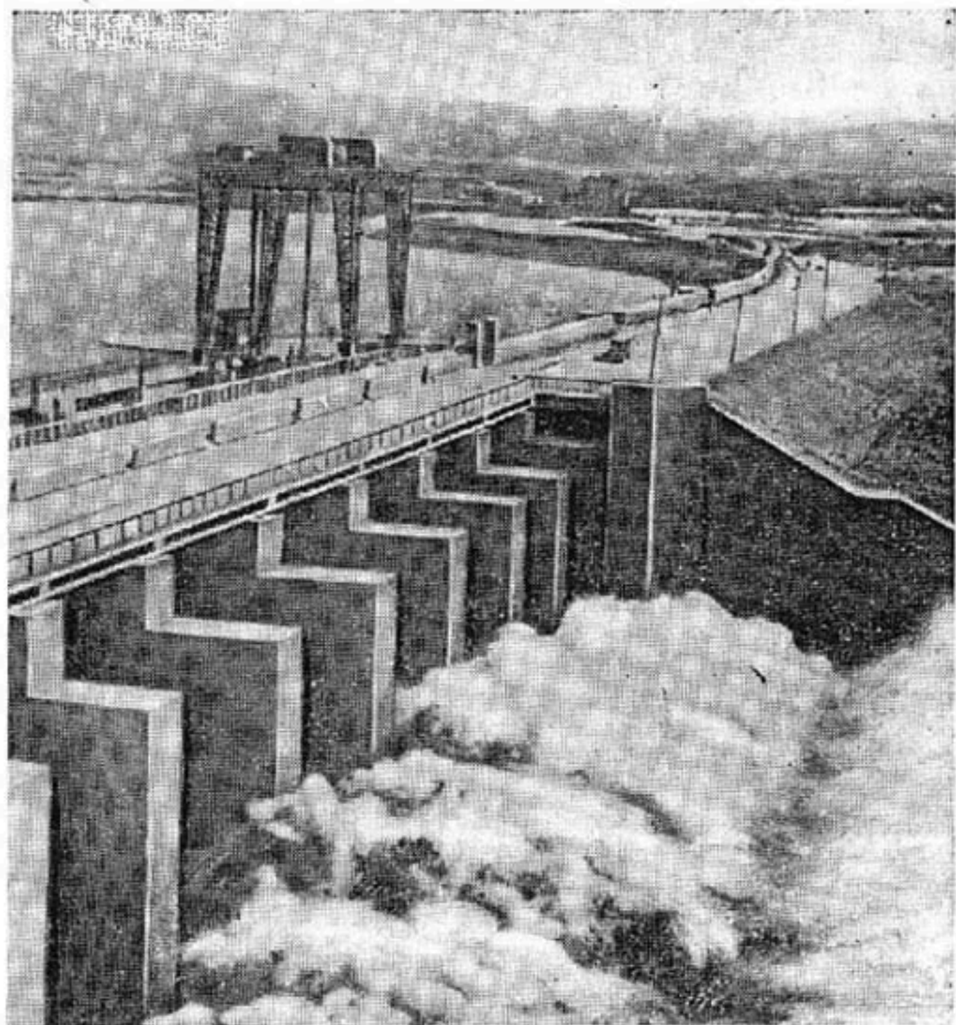
Фархадская плотина на р. Сыр-Дарье.
