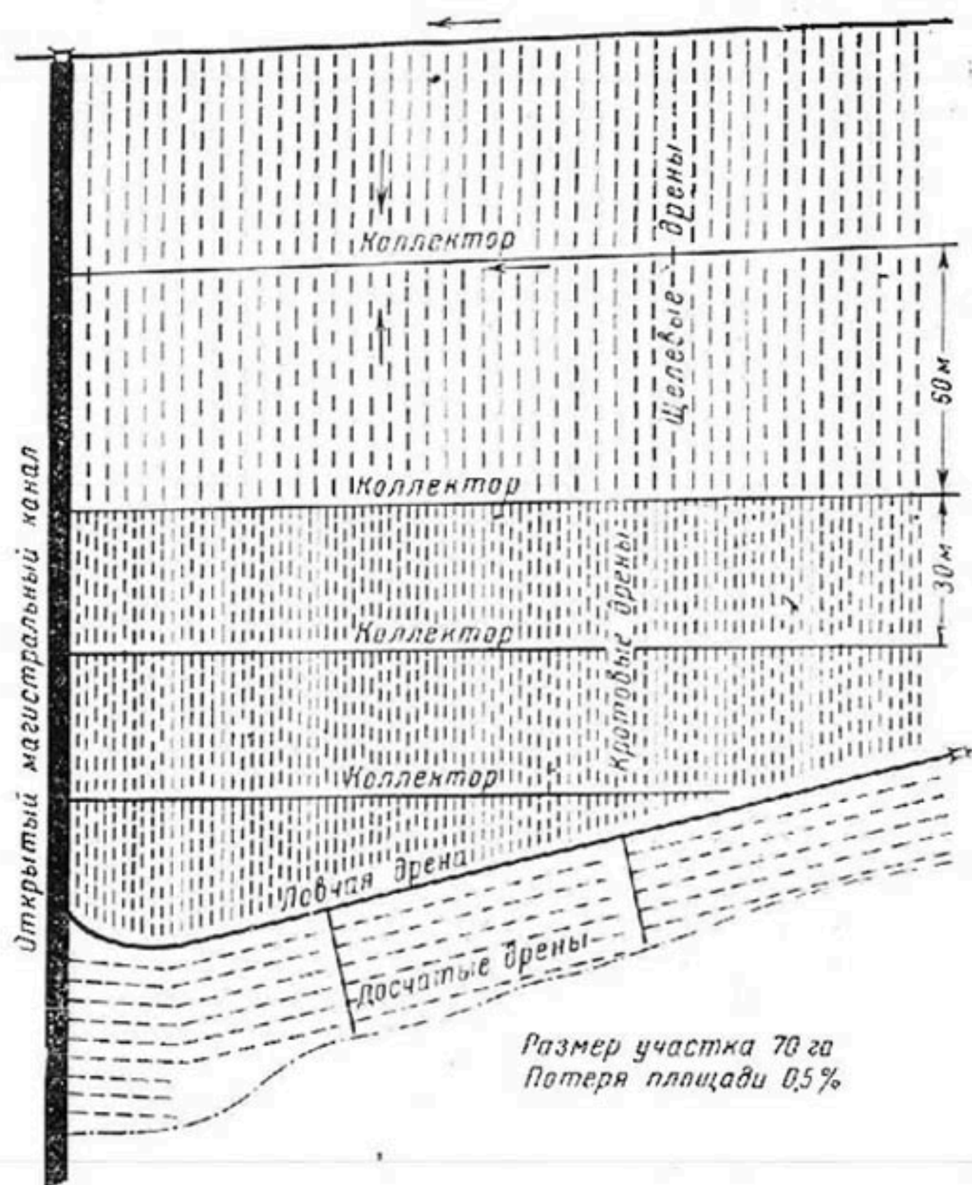
Схема осушения кротовым и щелевым дренажем.
