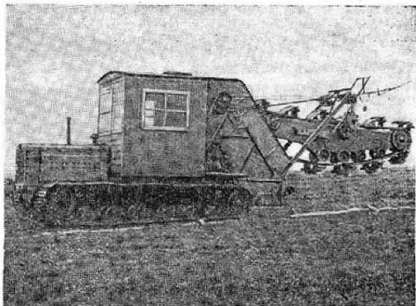
Траншейный экскаватор ЭТ-141 на нарезке траншей под гончарный дренаж.
