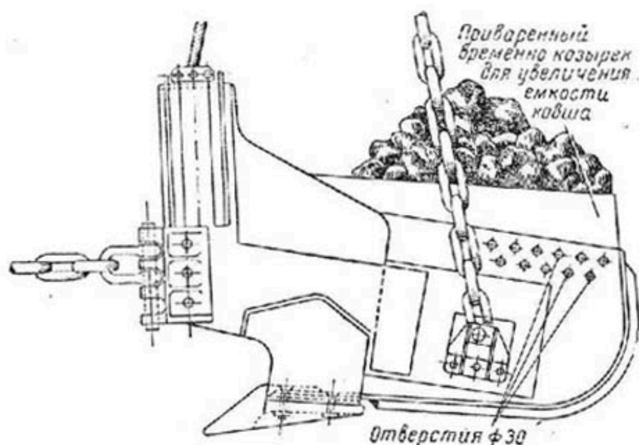
Ковш облегченной конструкции для работы во влажных грунтах.
