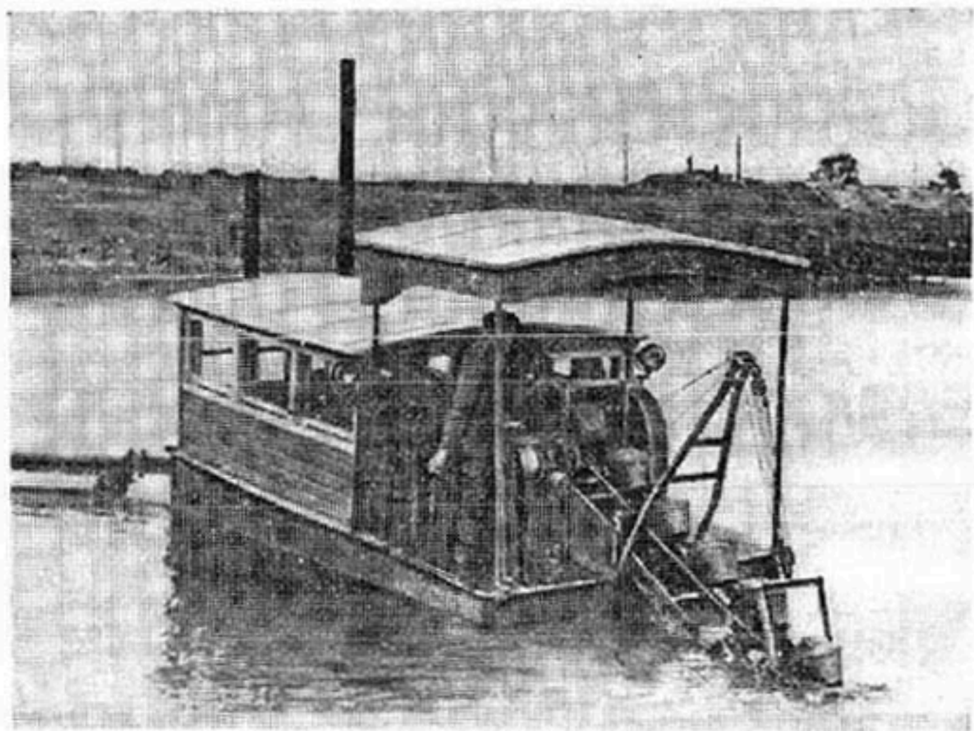
Землессосно-землечерпательная установка ЗЗУ-ВНИИГиМ на очистке пруда.
