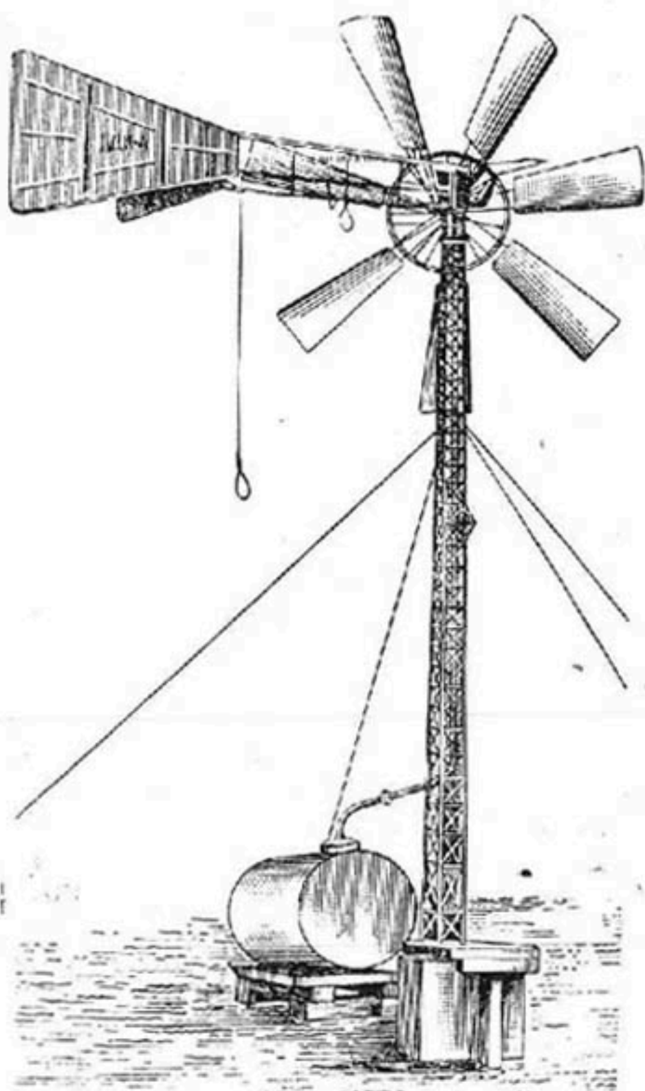
Ветронасосный агрегат ДДК-4.
