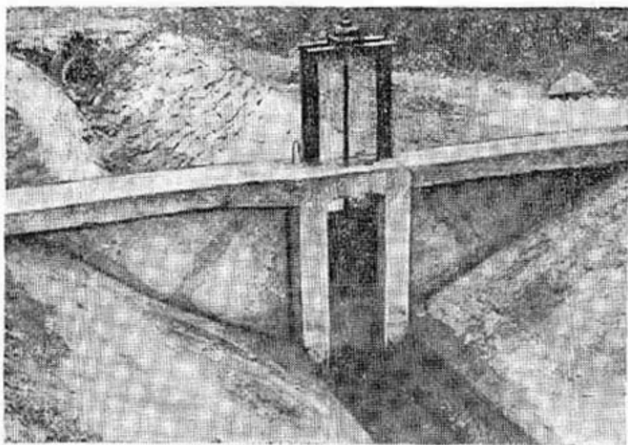
Сооружения на сети из плоских блоков на оросительной системе «Камешский Под» УССР.
