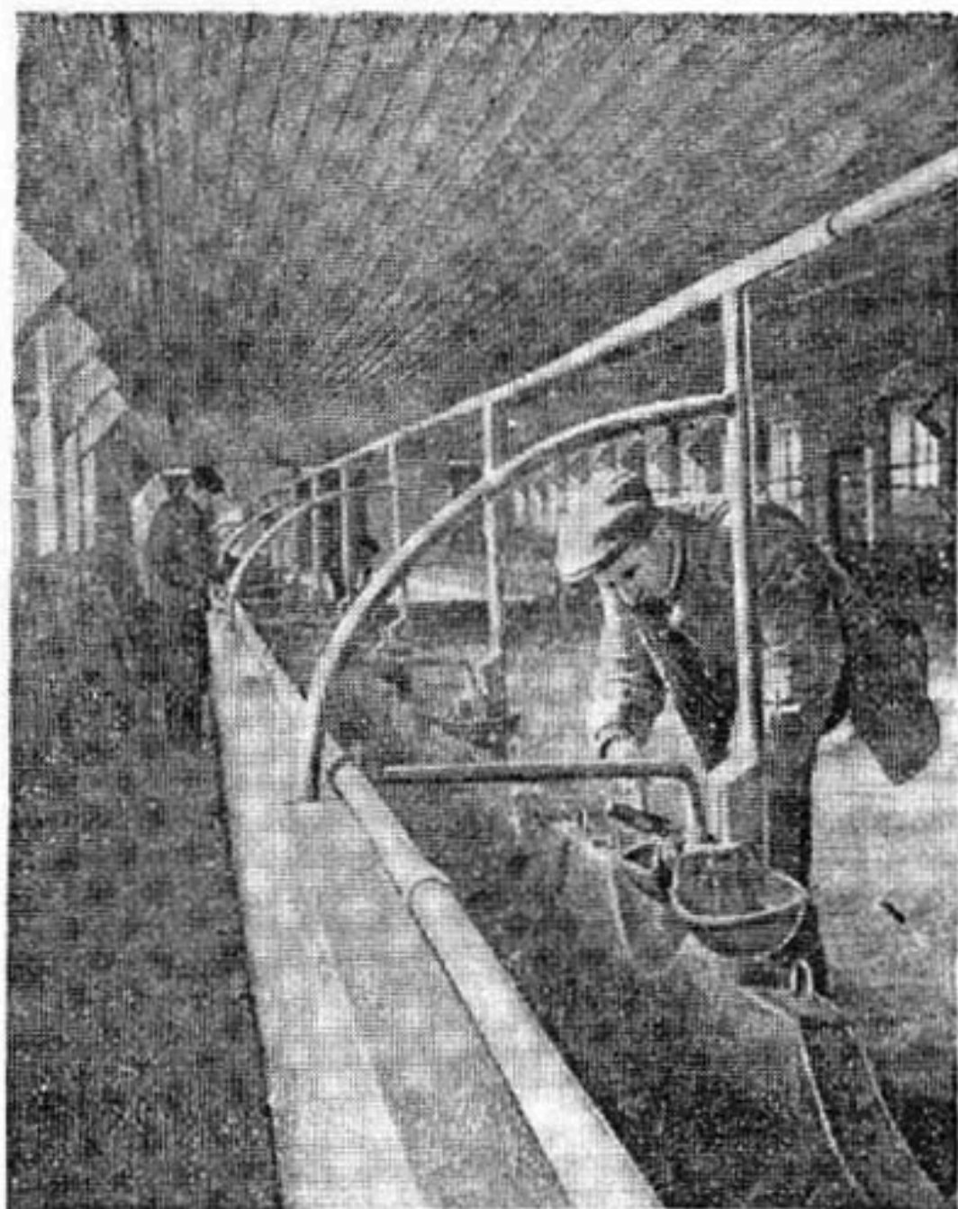
Монтаж автопоилок на животноводческой ферме.
