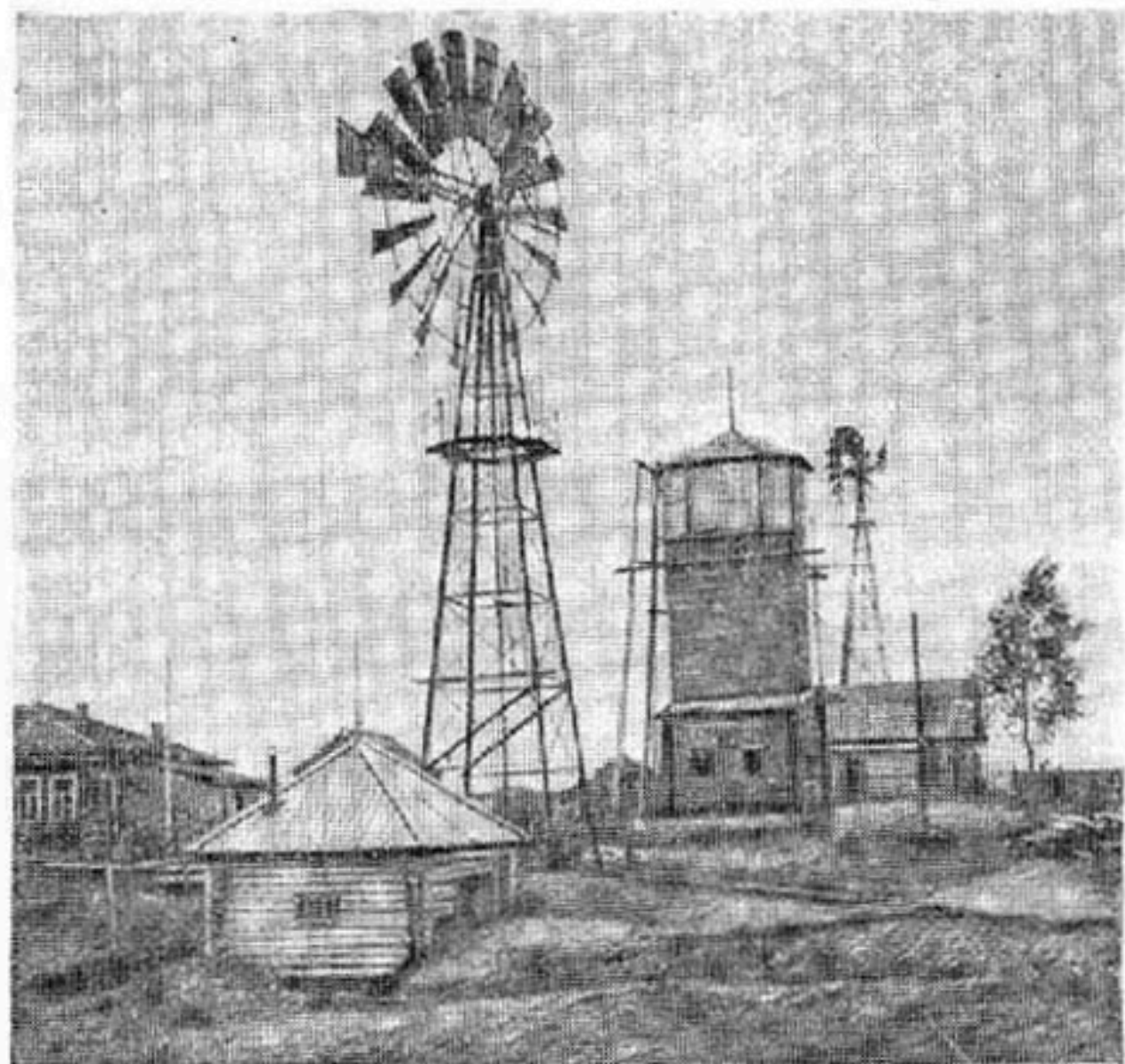
Ветродвигатель и водонапорная башня, подающие воду на водоснабжение деревни Чскоты Кировской области.
