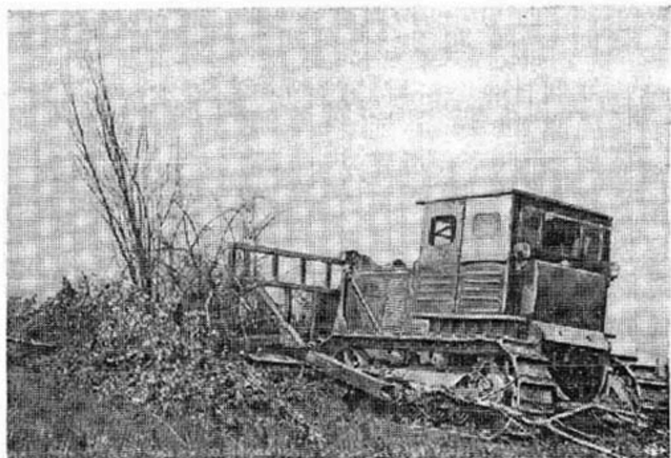
Корчеватель-собираатель Д-210В.
