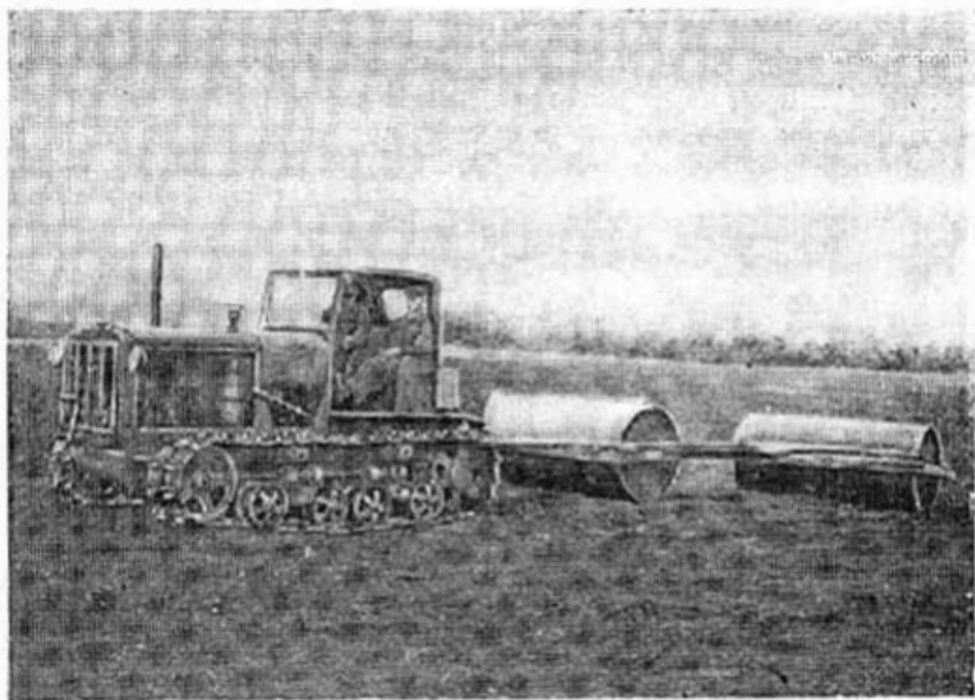
Катки KBГ-1,4 для прикатывания осушенных земель.
