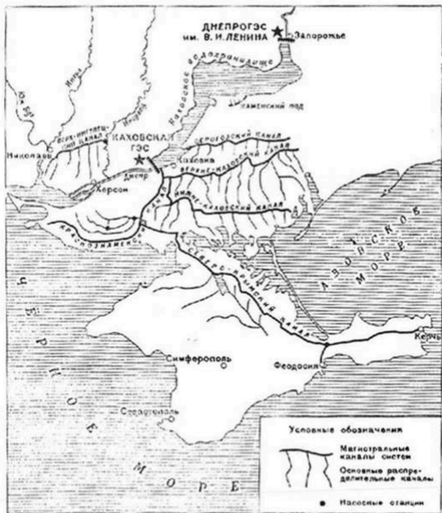
Схема орошения юга Украины на базе Каховского гидроузла.
