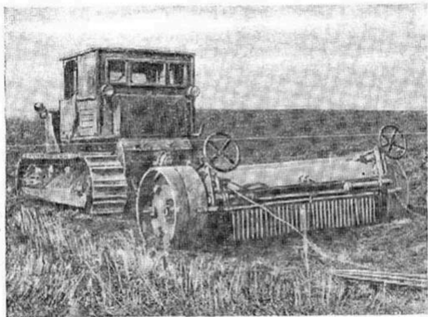
Фрезбарабаи ФБ-1,0.
