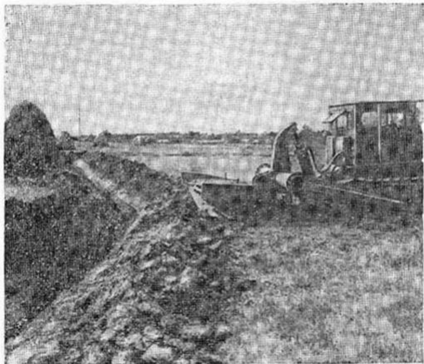
Навесная рама УМАС с кашакопателем КОР-500.
