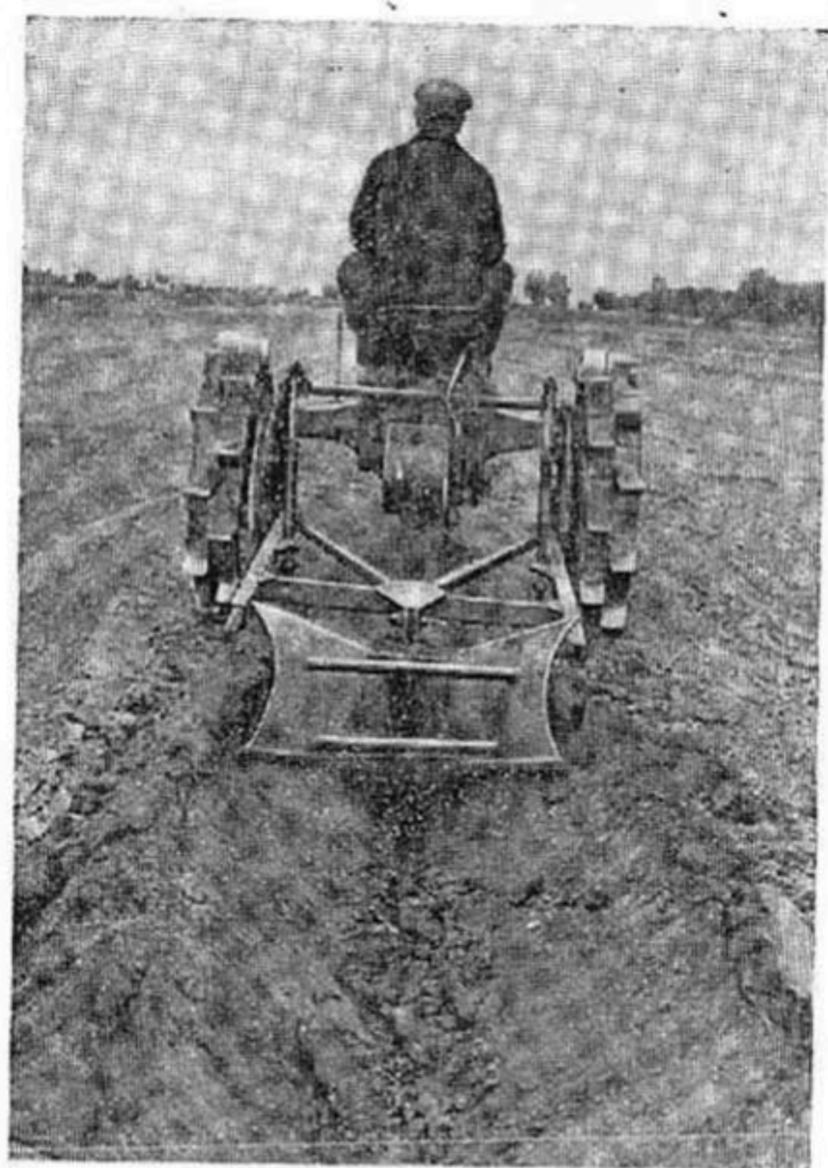
Канавокопатель КРН на парезке временных оросителей.
