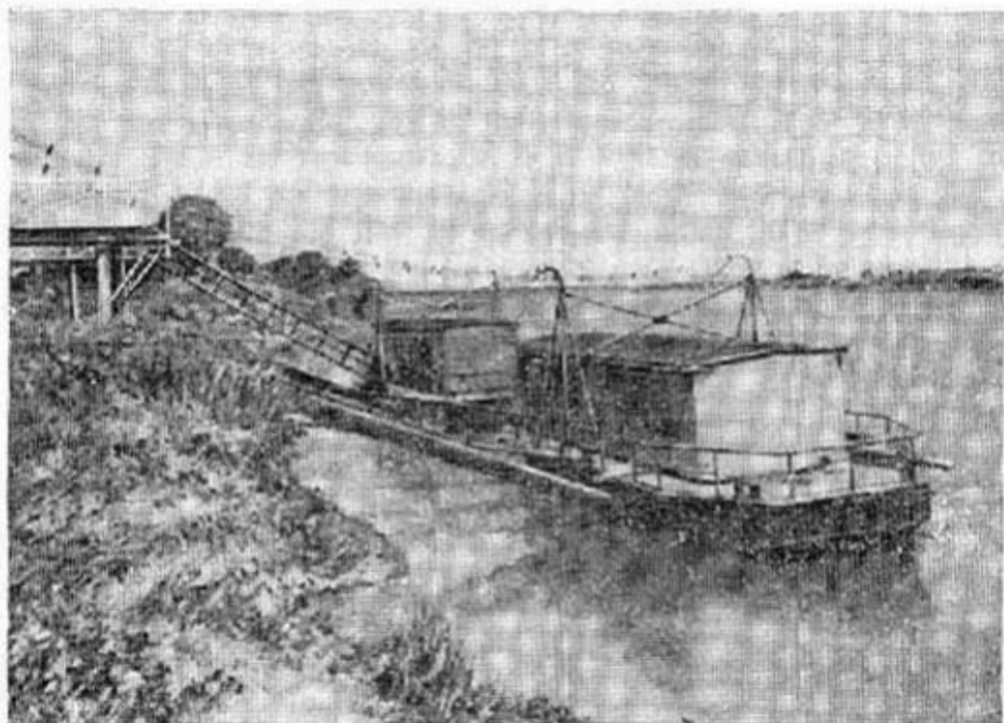
Пловучая насосная станция на р. Кура.
