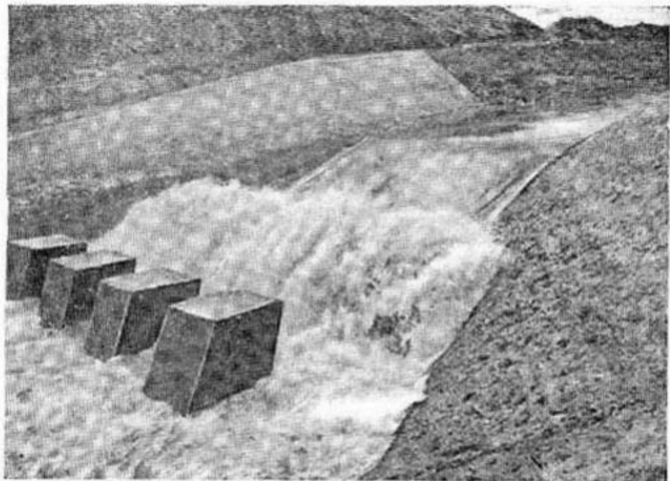
Перепад с гасителями на Северном Ферганском канале.
