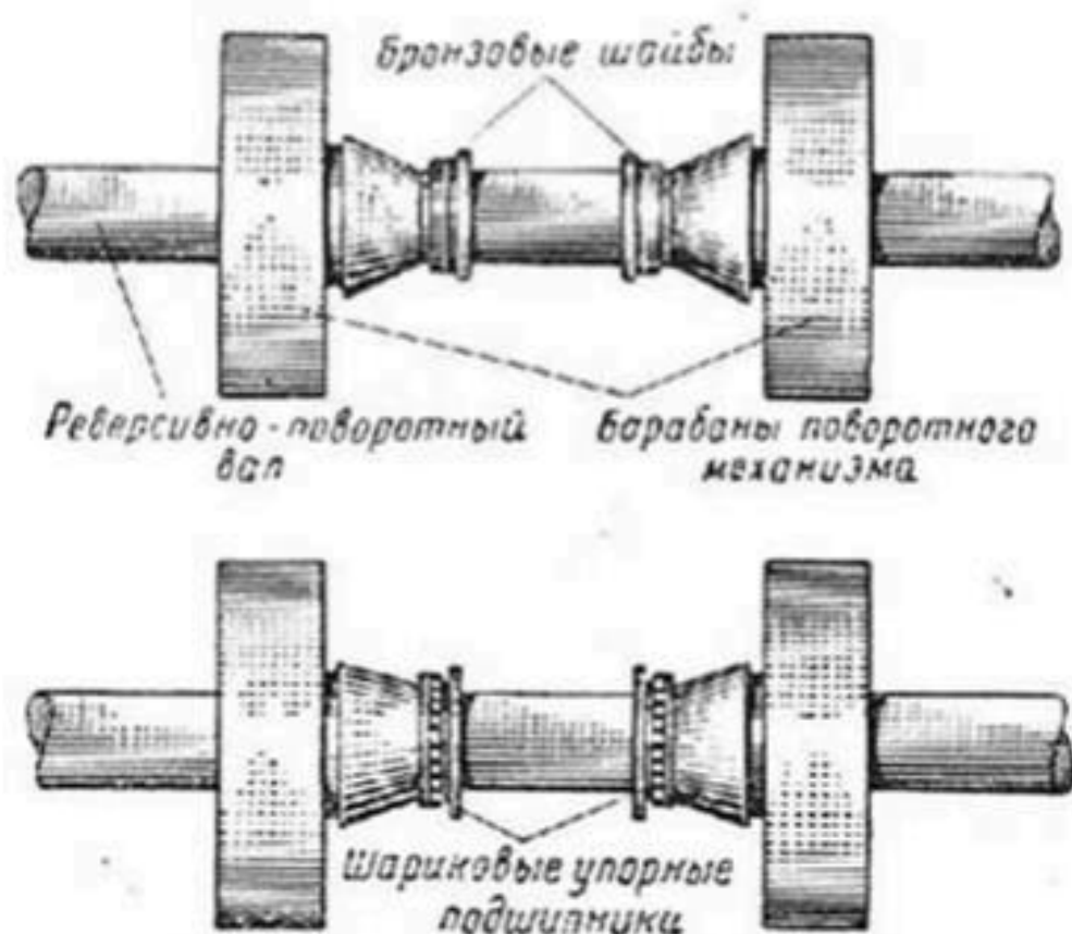
Реверсивно-поворотный механизм экскаватора.
