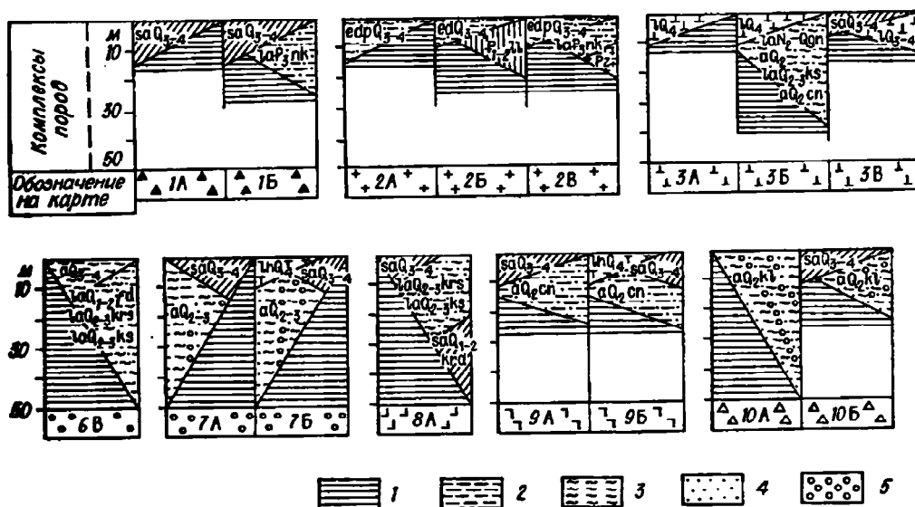
Рис. 2. Мелиорируемые комплексы пород надводноупорной
