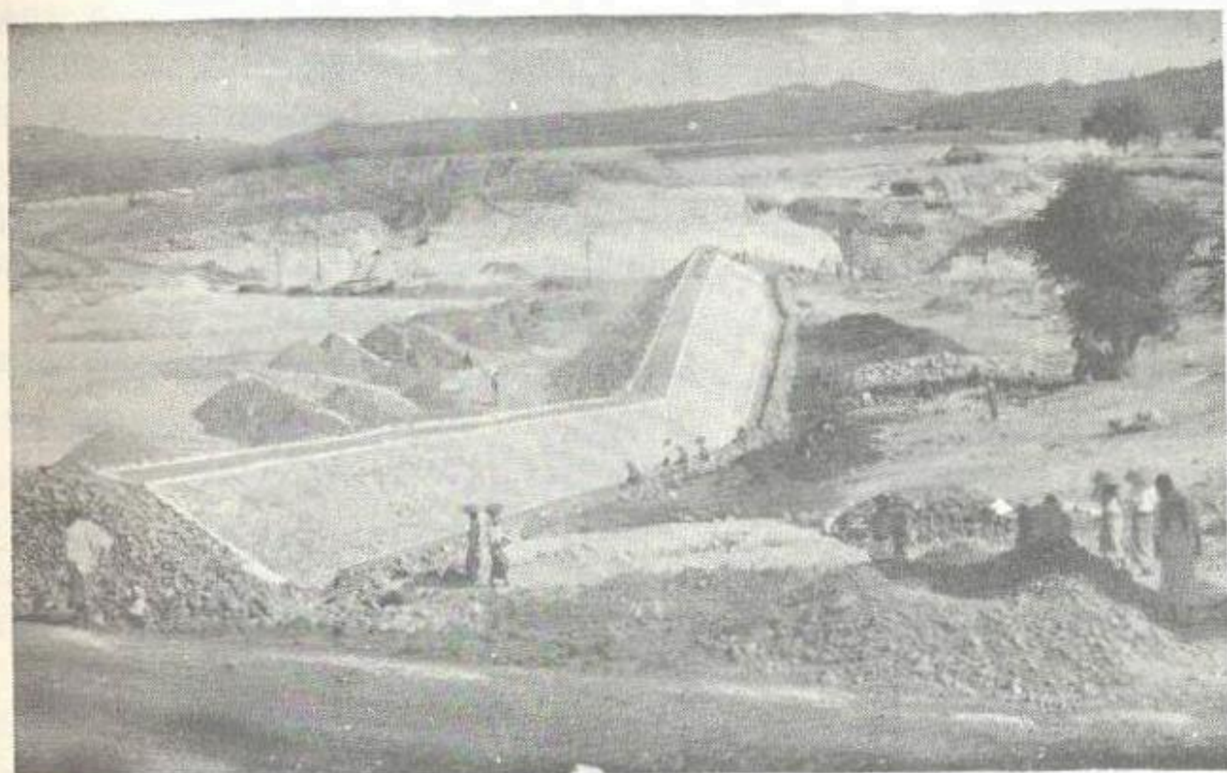
Рис. 1. Дренажная призма одной из частей плотины
